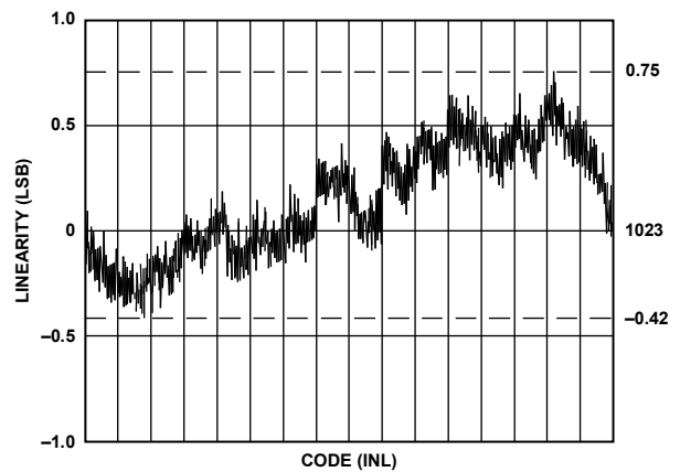
図 18. 直線性
