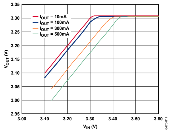
図 16. 入力電圧対出力電圧(ドロップアウト)
