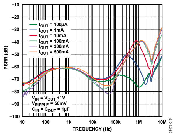
図 17. 電源除去比の周波数特性、VOUT = 2.8 V、VIN = 3.8 V
