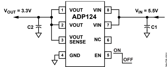
図 1. 固定出力電圧の ADP124
