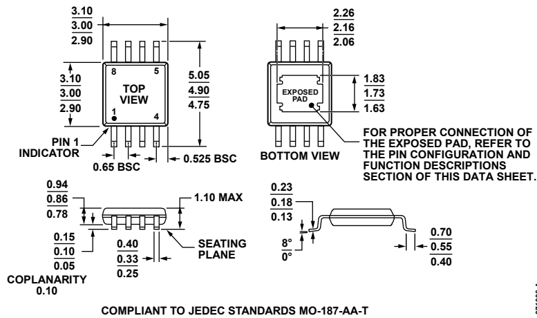
図 45. エクスポート・パッド付き 8 ピン・ミニモールド・アウトライン・パッケージ [MINI_SO_EP] (RH-8-1) 寸法: mm
