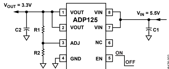
図 2. 調整可能出力電圧の ADP 125
