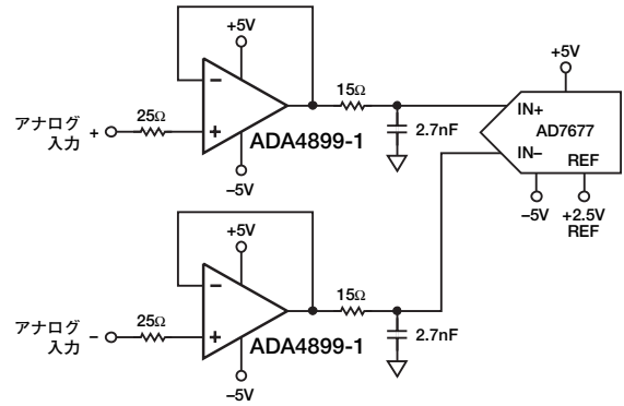
図49. シングルエンド入力のADCドライバ
