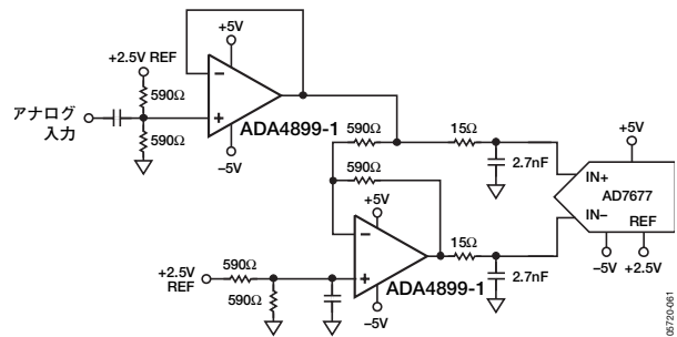
図50. シングルエンド/差動変換ADCドライバ
