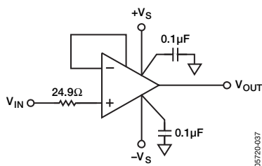
図46. ユニティ・ゲイン回路図
