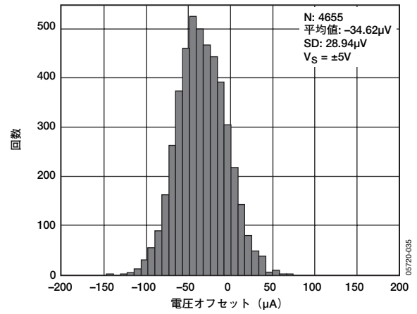
図39. 入力オフセット電圧の分布 ( V_S=\pm 5V )
