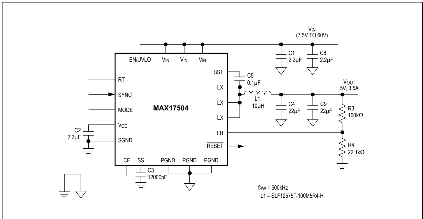
图3. 5V输出典型应用电路
