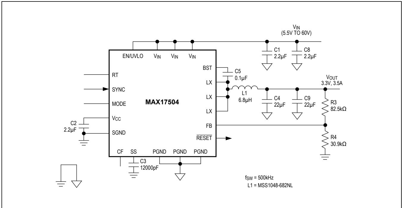
图4. 3.3V输出典型应用电路
