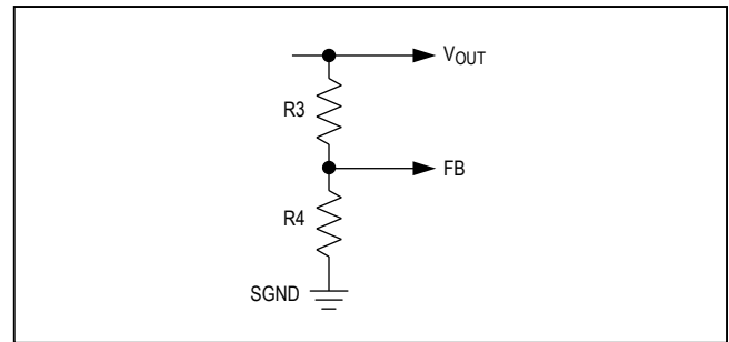
图2. 设置输出电压
