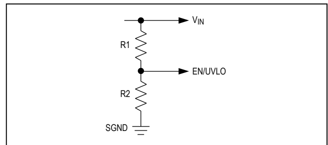
图1. 设置输入欠压锁定
