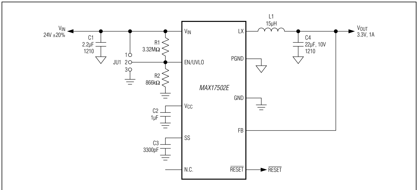
图3. MAX17502E应用电路(3.3V输出, 1A最大负载电流, 600kHz开关频率)
