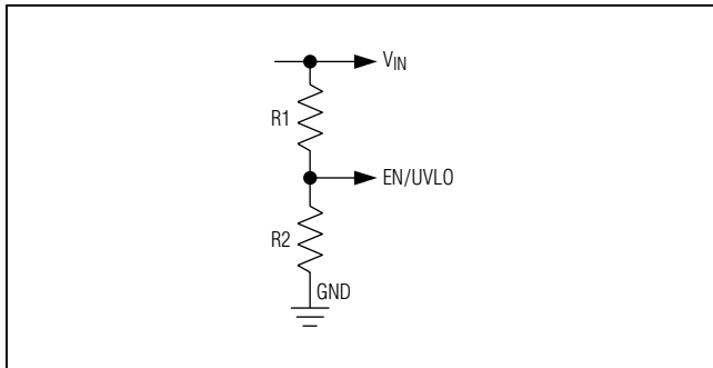
图1. 可调节UVLO网络
