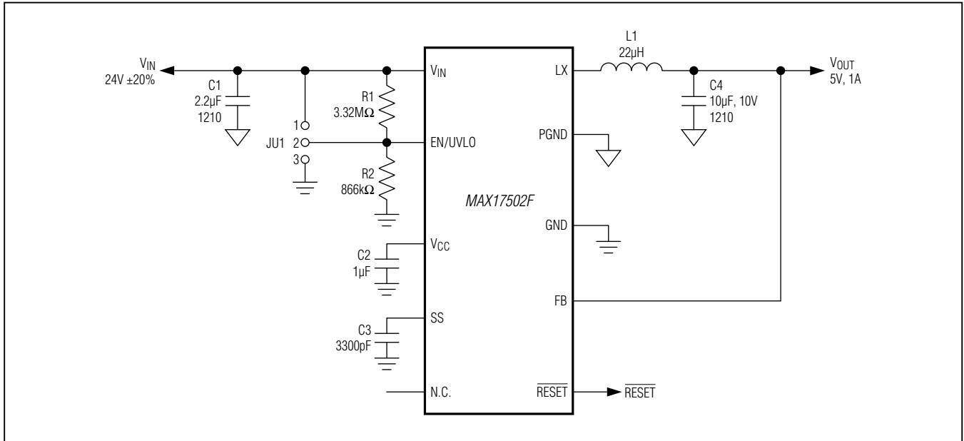
图2. MAX17502F应用电路(5V输出, 1A最大负载电流, 600kHz开关频率)
