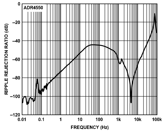
图79. ADR4550纹波抑制比与频率的关系
