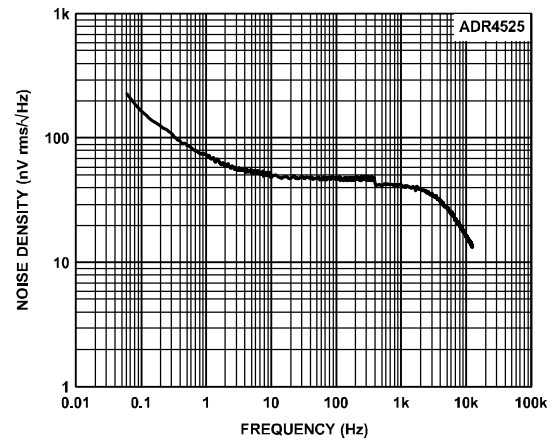
图25. ADR4525输出噪声谱密度
