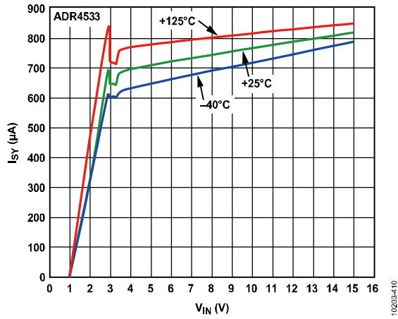
图50. ADR4533电源电流与电源电压的关系
