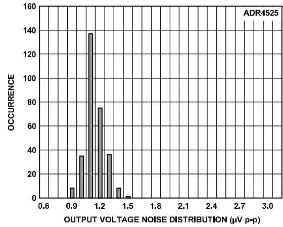
图24. ADR4525输出电压噪声 (最大幅度从0.1 Hz到10 Hz)
