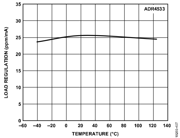
图47. ADR4533负载调整率与温度的关系 (源电流)
