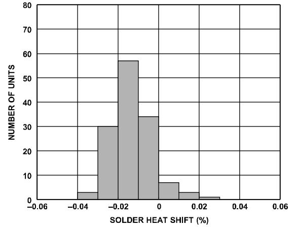
图29. ADR4525焊接热阻变化 (3 × 回流)
