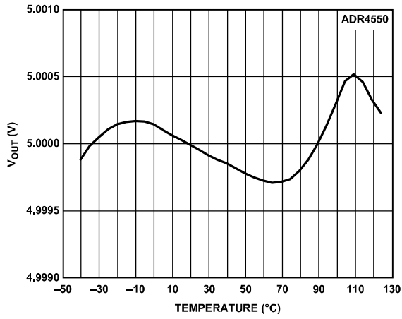
图70. ADR4550 B级输出电压与温度的关系
