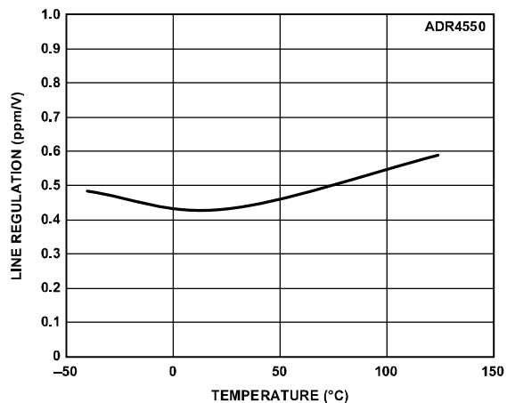
图75. ADR4550线性调整率与温度的关系
