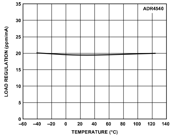
图60. ADR4540负载调整率与温度的关系 (源电流)
