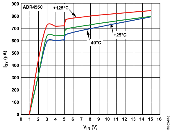
图76. ADR4550电源电流与电源电压的关系
