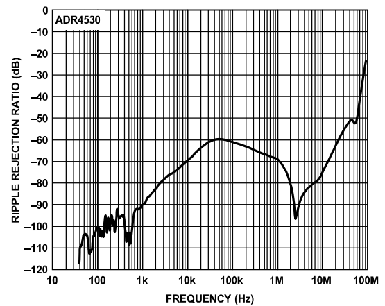
图40. ADR4530纹波抑制比与频率的关系
