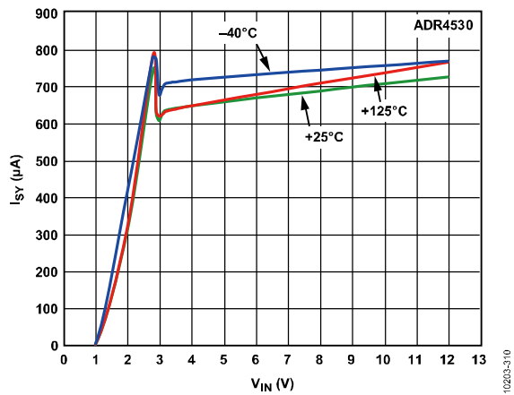
图37. ADR4530电源电流与电源电压的关系
