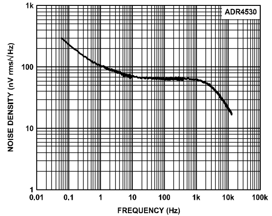
图39. ADR4530输出噪声谱密度
