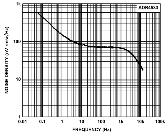
图52. ADR4533输出噪声谱密度
