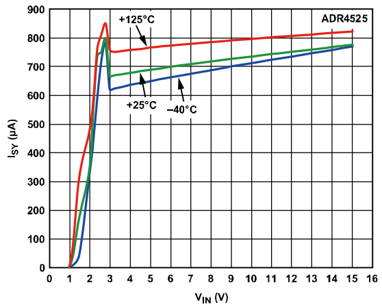
图23. ADR4525电源电流与电源电压的关系
