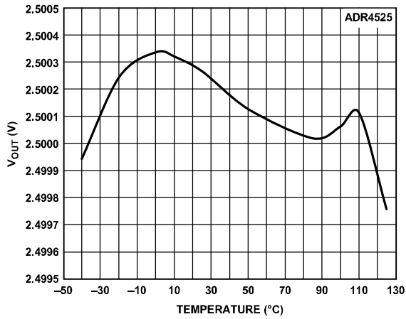
图16. ADR4525 B级输出电压与温度的关系
