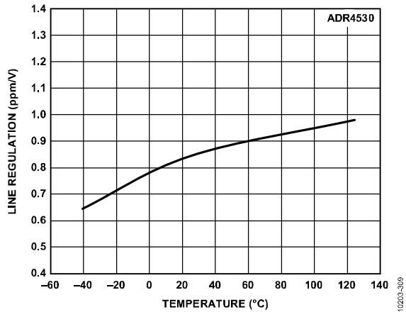
图36. ADR4530线性调整率与温度的关系
