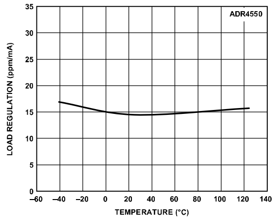
图73. ADR4550负载调整率与温度的关系 (源电)
