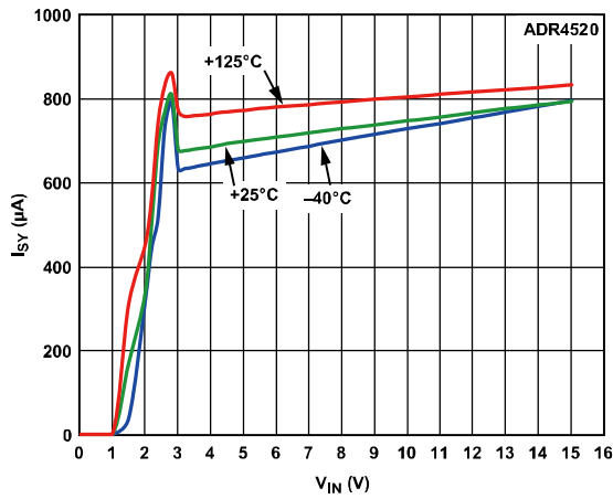
图9. ADR4520电源电流( I_{SV} )与电源电压的关系
