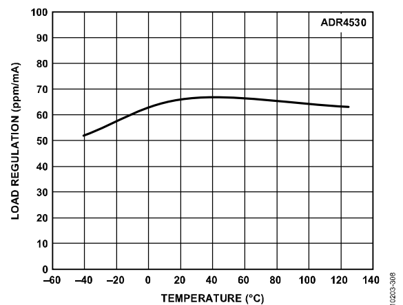
图35. ADR4530负载调整率与温度的关系 (吸电流)
