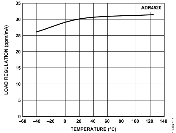
图6. ADR4520负载调整率与温度的关系 (源电流)
