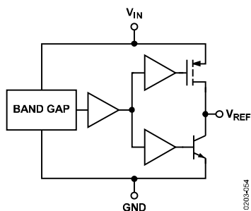
图83. ADR4520/ADR4525/ADR4530/ADR4533/ADR4540/ADR4550简化原理示意图
