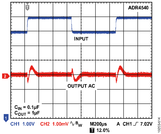
图67. ADR4540线路瞬态响应
