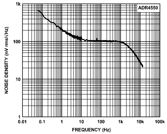
图78. ADR4550输出噪声谱密度
