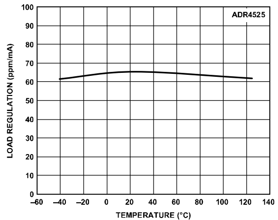
图21. ADR4525负载调整率与温度的关系 (吸电流)
