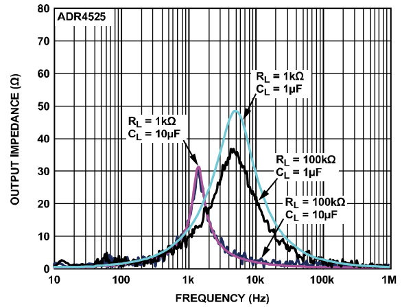
图28. ADR4525输出阻抗与频率的关系
