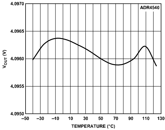
图57. ADR4540 B级输出电压与温度的关系
