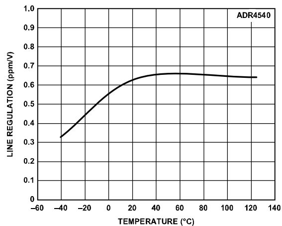
图62. ADR4540电源电压调整率与温度的关系
