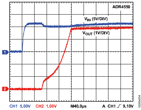
图71. ADR4550输出电压启动响应
