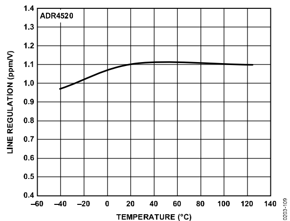
图8. ADR4520线性调整率与温度的关系
