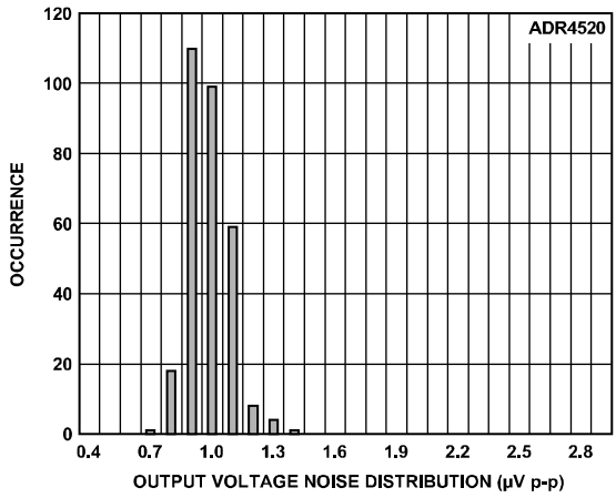
图10. ADR4520输出电压噪声 (最大幅度从0.1 Hz到10 Hz)
