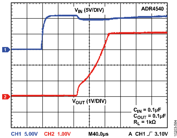
图58. ADR4540输出电压启动响应
