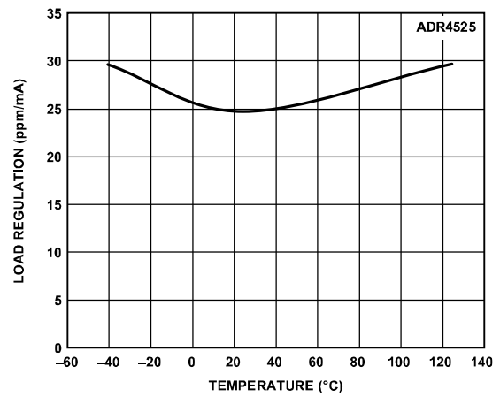
图20. ADR4525负载调整率与温度的关系 (源电流)
