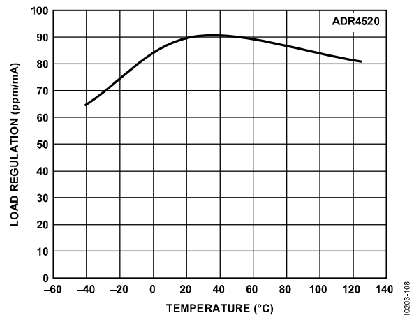
图7. ADR4520负载调整率与温度的关系 (吸电流)
