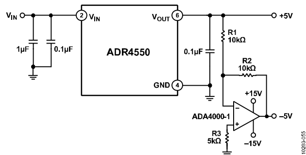
图84. ADR4550双极性输出基准电压源
