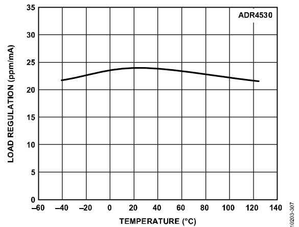
图34. ADR4530负载调整率与温度的关系 (源电流)
