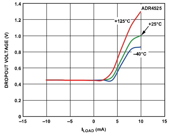
图19. ADR4525压差与负载电流的关系
