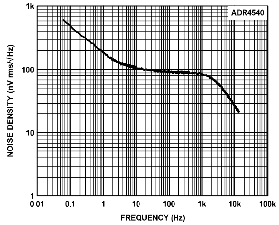
图65. ADR4540输出噪声谱密度
