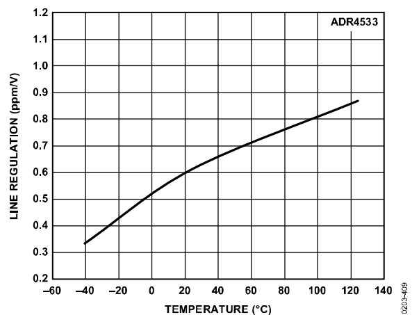
图49. ADR4533线性调整率与温度的关系
