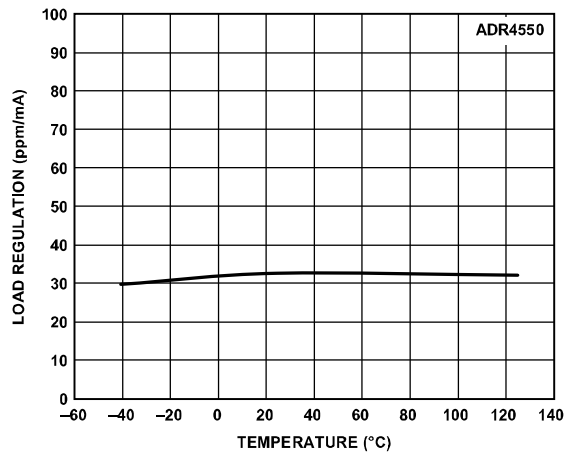
图74. ADR4550负载调整率与温度的关系 (吸电)
