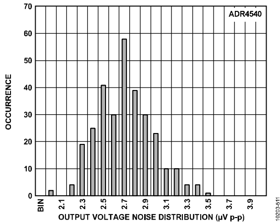
图64. ADR4540输出电压噪声 (最大幅度从0.1 Hz到10 Hz)
