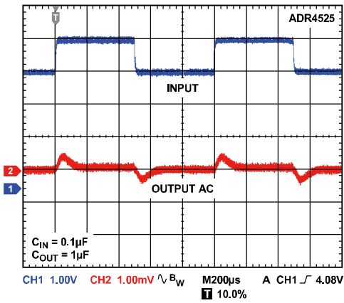
图27. ADR4525线路瞬态响应
