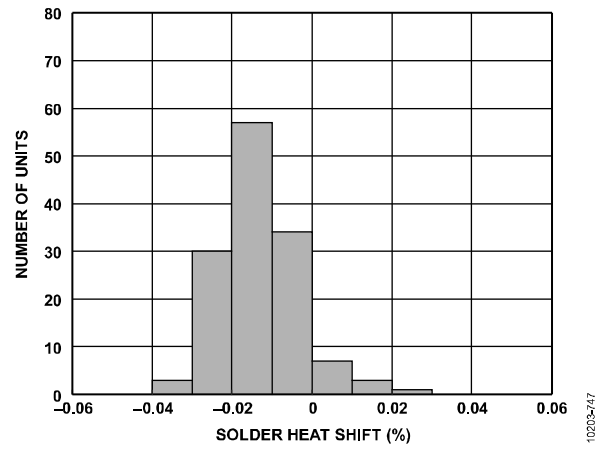
图43. ADR4530焊接热阻变化 (3 × 回流)
