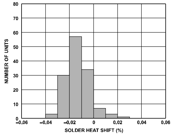
图82. ADR4550焊接热阻变化 (3 × 回流)
