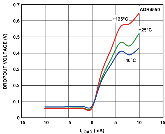
图72. ADR4550压差与负载电流的关系
