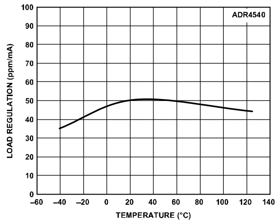
图61. ADR4540负载调整率与温度的关系 (吸电流)
