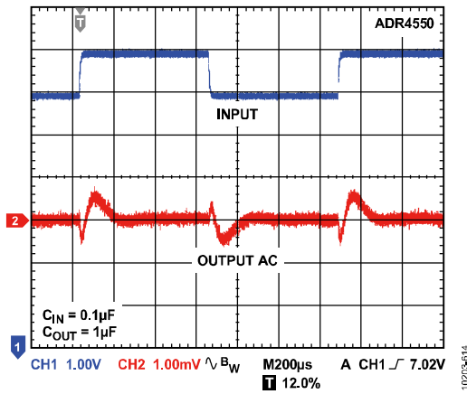
图80. ADR4550线路瞬态响应
