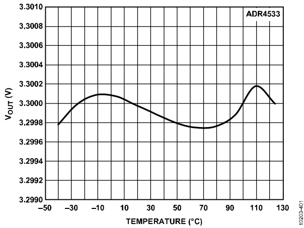
图44. ADR4533 B级输出电压与温度的关系
