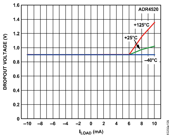
图5. ADR4520压差与负载电流的关系
