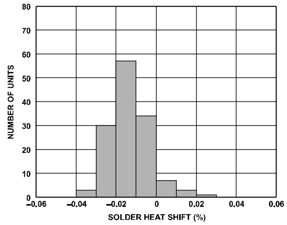
图69. ADR4540焊接热阻变化 (3 × 回流)
