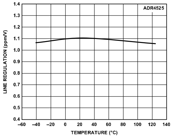
图22. ADR4525线性调整率与温度的关系
