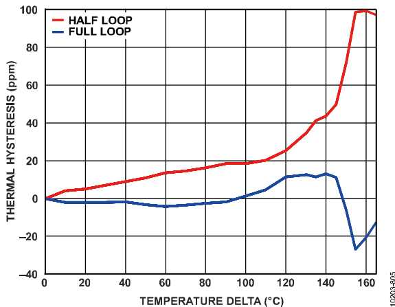
图92. 温度范围不断提高的热滞
