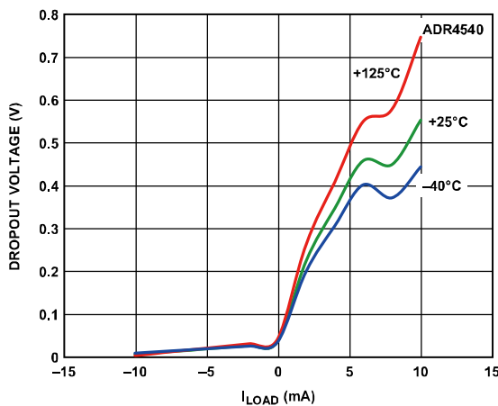
图59. ADR4540压差与负载电流的关系
