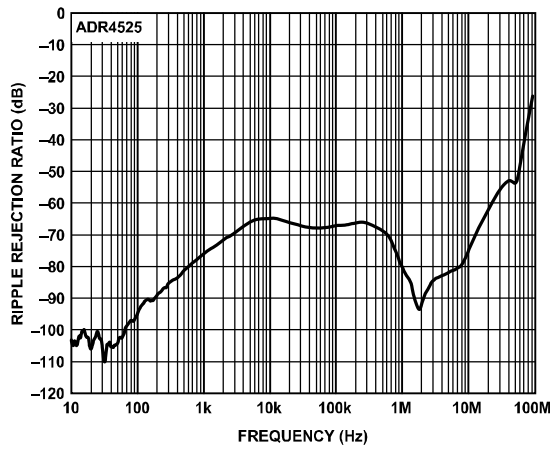
图26. ADR4525纹波抑制比与频率的关系
