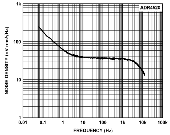
图11. ADR4520输出噪声谱密度
