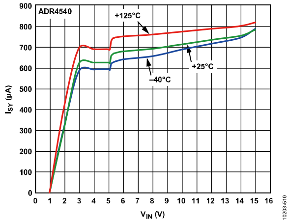
图63. ADR4540电源电流与电源电压的关系
