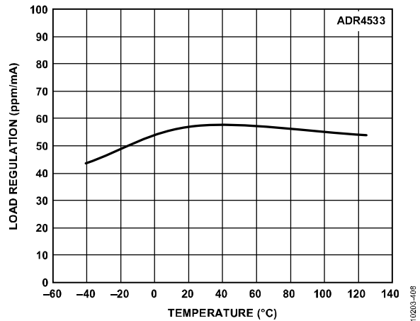
图48. ADR4533负载调整率与温度的关系 (吸电流)
