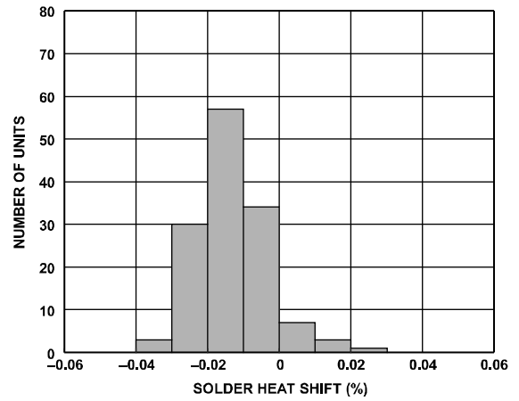
图15. ADR4520焊接热阻变化 (3 × 回流)
