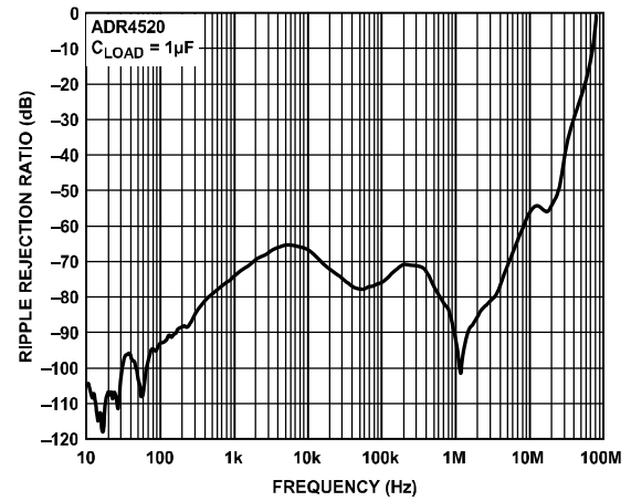
图12. ADR4520纹波抑制比与频率的关系
