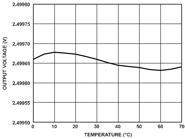
图17. ADR4525 C级输出电压与温度的关系
