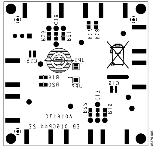
図 6. ボード組立図一回路面
