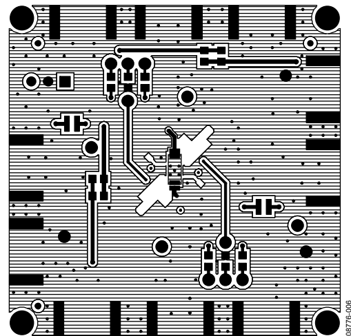
図 7. ボードのレイアウト・パターン一回路面
