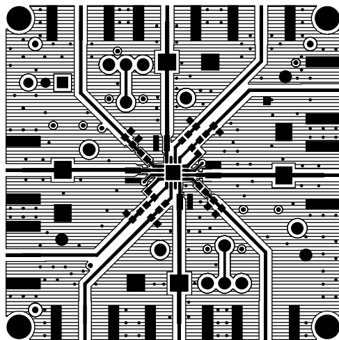
図 5. ボードのレイアウト・パターン一部品面
