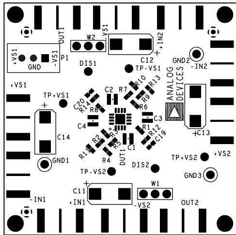
図 4. ボード組立図一部品面
