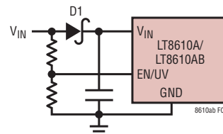
図3. 逆入力保護
