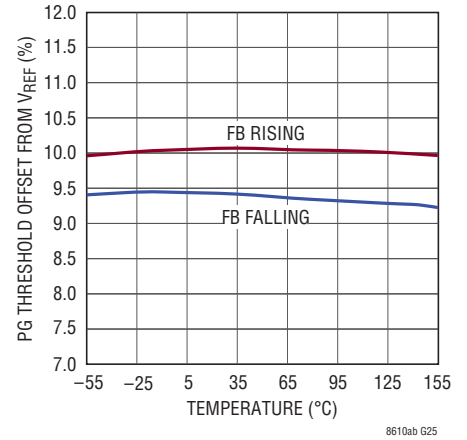
PGピンの“H”しきい値
