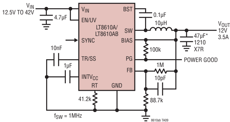
12V 降圧コンバータ
