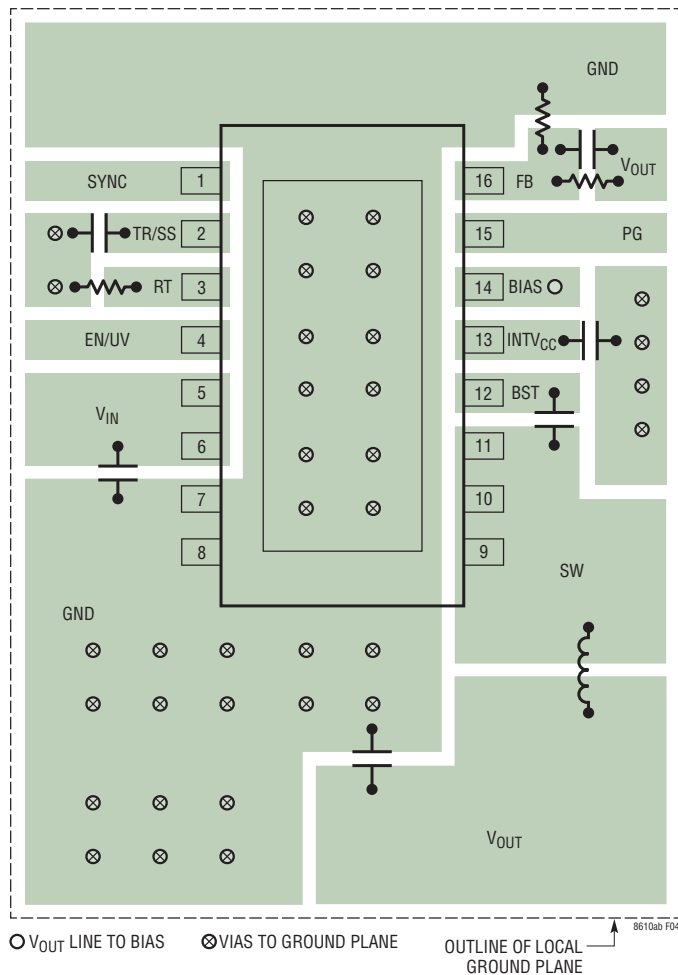
図4. LT8610A/LT8610ABの推奨PCBレイアウト
