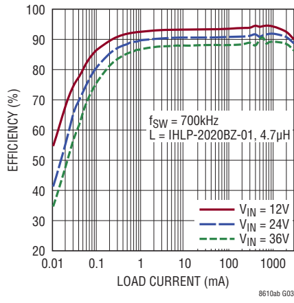
5V出力時のLT8610ABの効率
