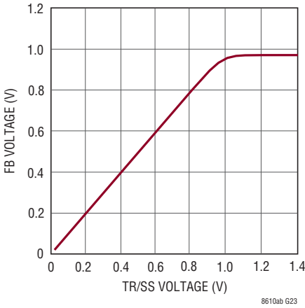
ソフトスタートおよび トラッキングの電圧
