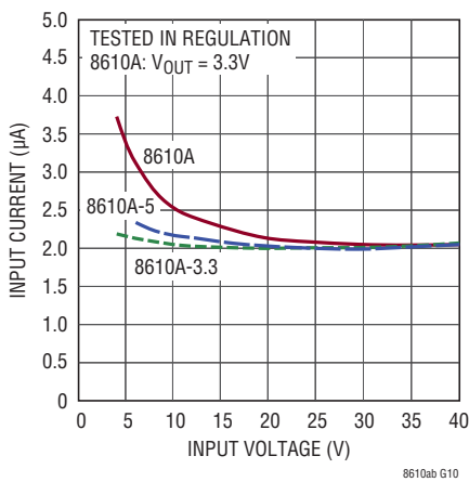
LT8610A 無負荷時電源電流
