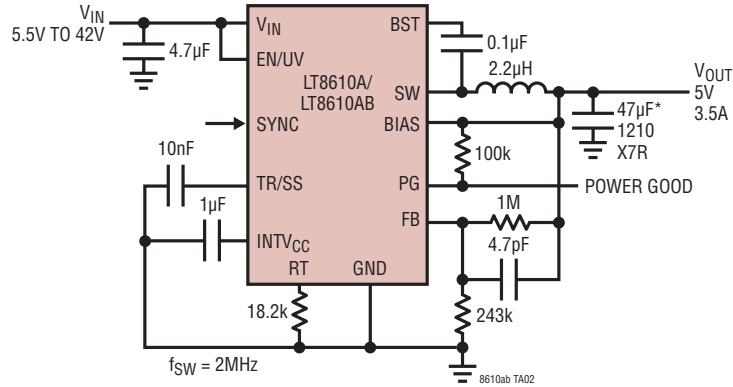
5V/2MHz 降圧コンバータ
