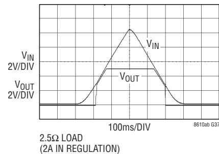
起動時のドロップアウト性能
