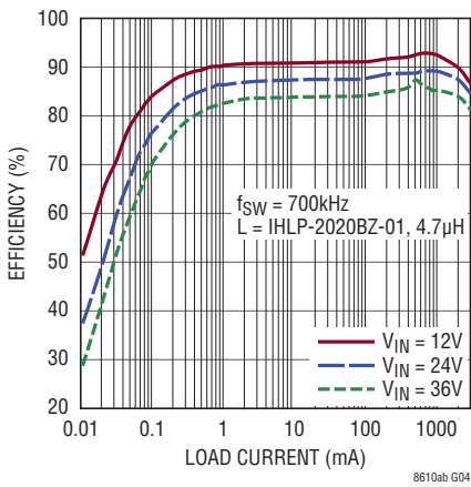
3.3V出力時のLT8610ABの効率
