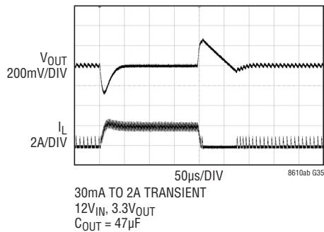
LT8610A/LT8610ABの トランジェント応答
