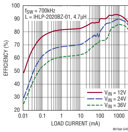
3.3V出力時のLT8610Aの効率
