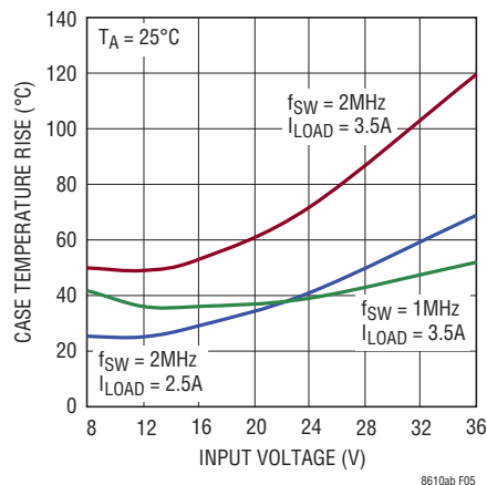
図5. LT8610ABのケース温度の上昇
