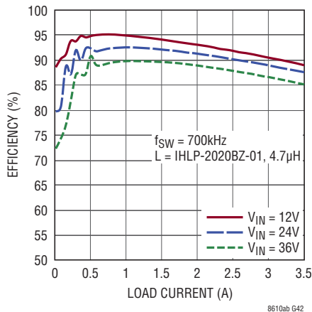
5V出力時のLT8610Aの効率
