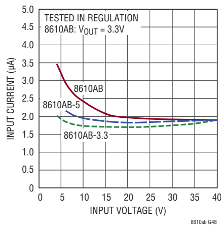
LT8610AB 無負荷時電源電流
