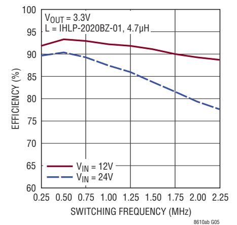
LT8610A/LT8610ABの効率と 1A時の周波数
