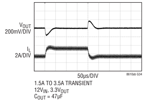
LT8610A/LT8610ABの トランジェント応答
