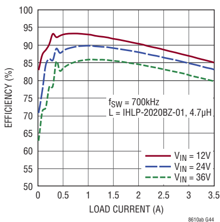
3.3V出力時のLT8610Aの効率
