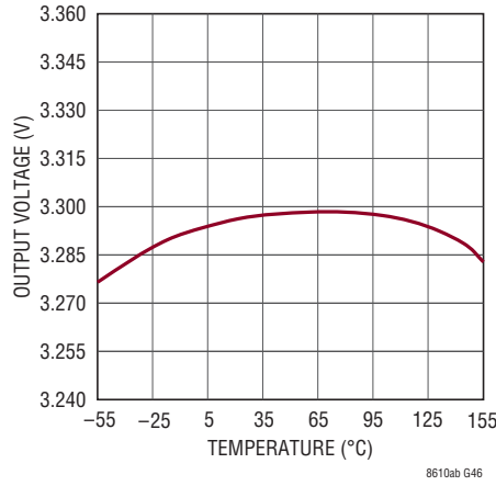
LT8610A-3.3出力電圧
