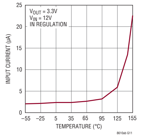
無負荷時電源電流
