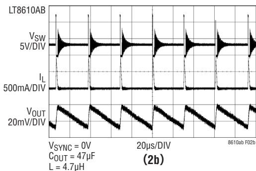
図2. LT8610A (2a)およびLT8610AB (2b)のBurst Mode動作
