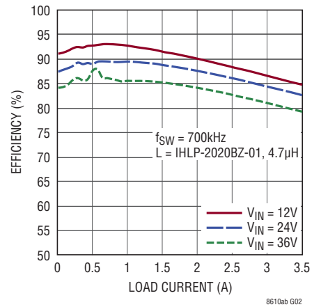
3.3V出力時のLT8610ABの効率
