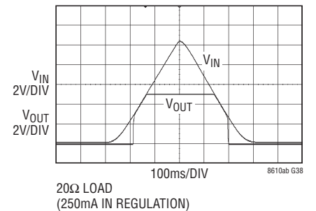
起動時のドロップアウト性能
