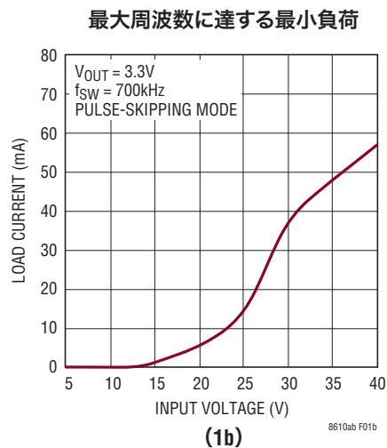
図1. スwitchング周波数と負荷情報: Burst Mode動作の場合(1a)およびパルス・スキップ・モードの場合(1b)
