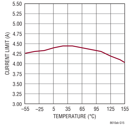
下側FETの電流制限
