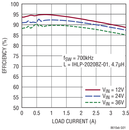
5V出力時のLT8610ABの効率
