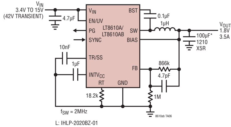
1.8V/2MHz 降圧コンバータ
