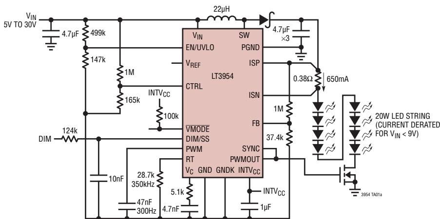
効率が 95% の内部 PWM 調光付き 20W 昇圧型 LED ドライバ
