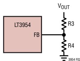
図 2. 昇圧型 LED ドライバまたは SEPIC 型 LED ドライバでの帰還抵抗の接続
