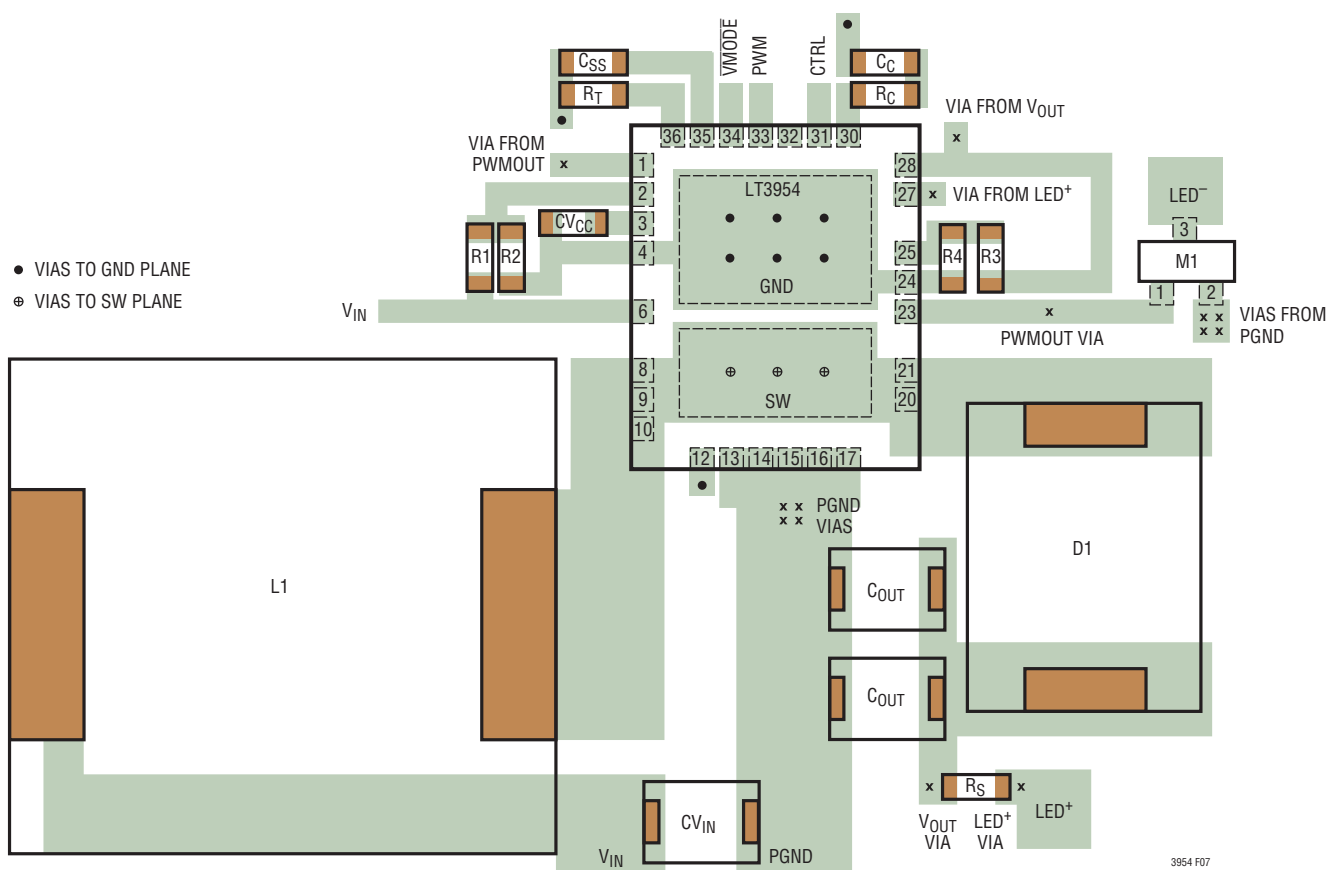
図7.昇圧コンバータの推奨レイアウト
