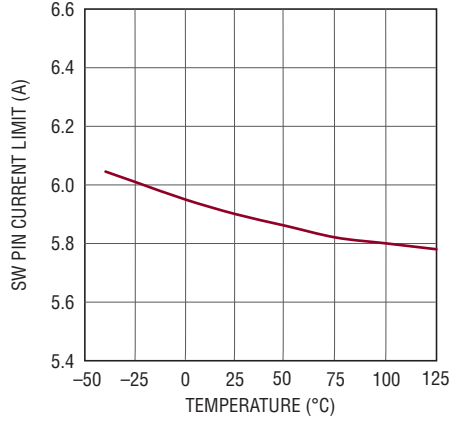
SWピンの電流制限と温度
