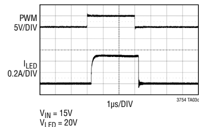
120Hzでの3000:1 PWM調光
