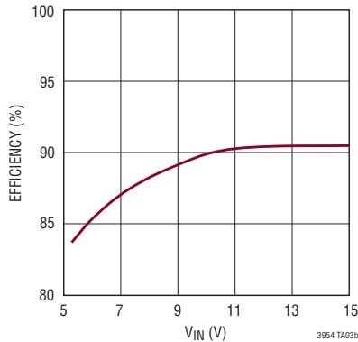
効率と V_{IN}
