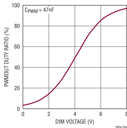
図4.PWMOUTピンのデューティ比とDIM/SSピンの電圧(R DIM = 124k)
