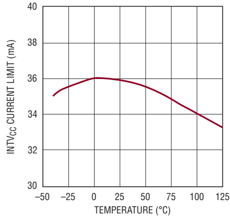
INTV CC ピンの電流制限と温度
