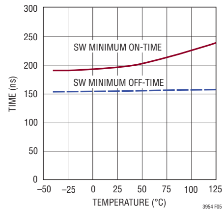
図5. スイッチの標準的な最小オン時間および最小オフ時間でのパルス幅と温度
