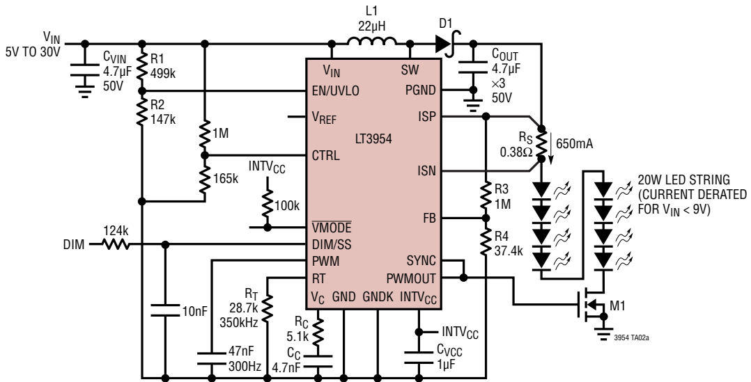
効率が95%の内部PWM調光付き20W昇圧型LEDドライバ
