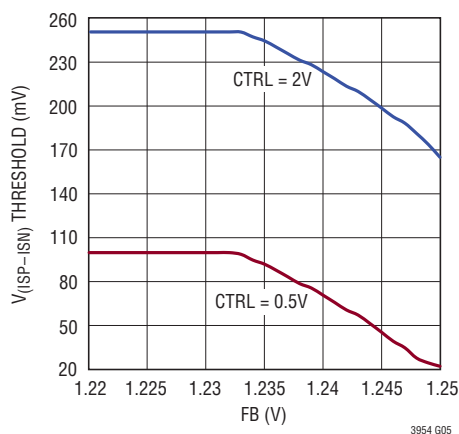
V_{(ISP-ISN)} のしきい値とFBの電圧
