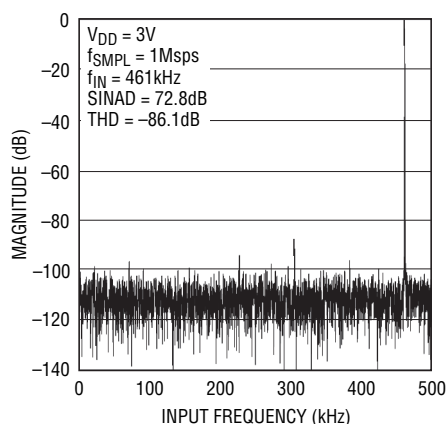
461kHz正弦波の8192ポイントの FFTプロット
