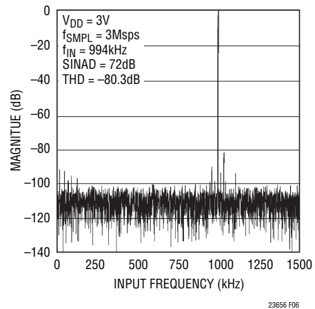
図6. LTC2366のFFTプロット
