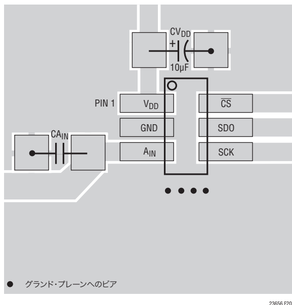
図20. 電源の接地方法
