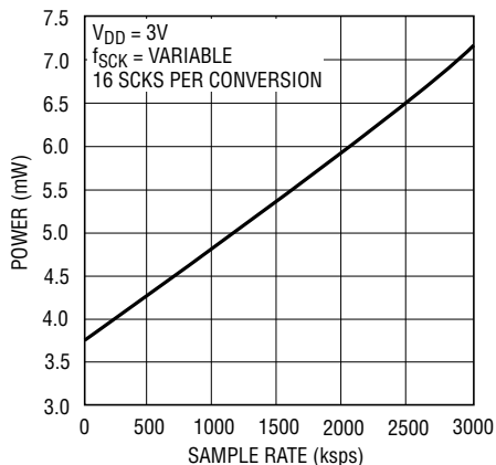
図16. デバイスが連続してパワーアップした状態に留まる際の電力消費とサンプリング・レート
