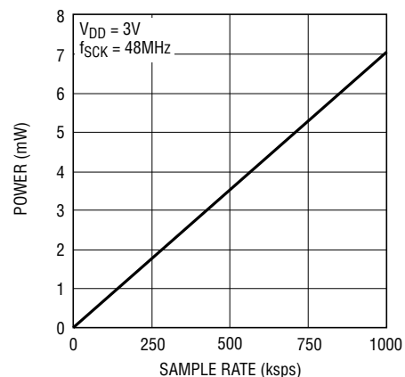
図17. 変換を行わないときはデバイスがスリープ・モードに移行する場合の電力消費とサンプリング・レート
