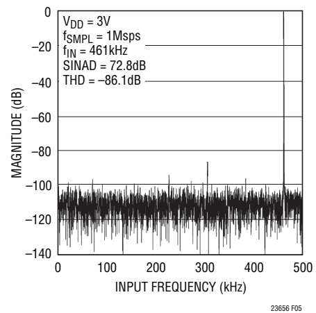
図5. LTC2365のFFTプロット
