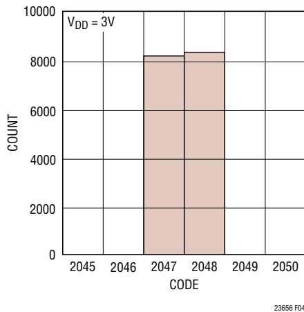
図4. 16384回の変換のヒストグラム
