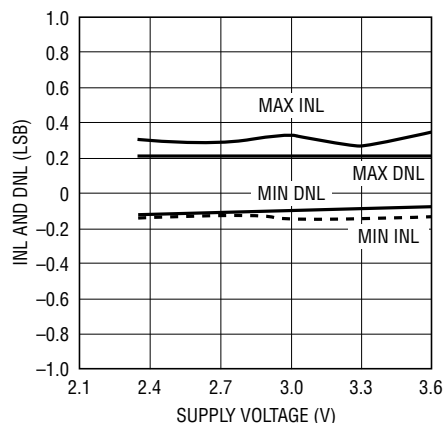
積分非直線性 および微分非直線性と電源電圧
