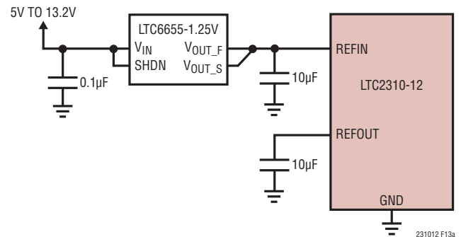
図13a. 外部REFIN電圧を使用したLTC2310-12
