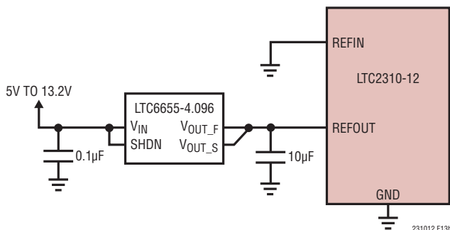
図 13b. 外部 REFOUT 電圧を使用した LTC2310-12
