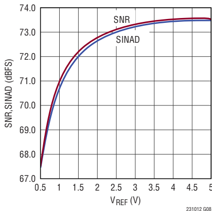
SNR, SINADとリファレンス電圧、 (f_{IN} = 500\text{kHz})
