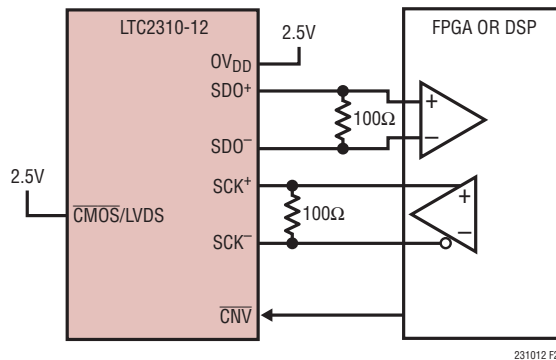
図22. LVDSインタフェースを使用するLTC2310-12
