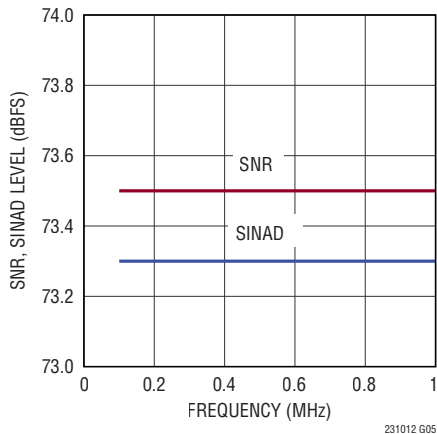
SNR, SINADと入力周波数 (100kHz ~ 1MHz)
