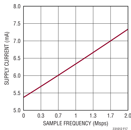
図17. LTC2310-12の電源電流とサンプリング・レート
