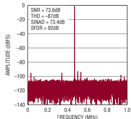
32k ポイントの FFT ( f_{SAMPL} = 2\text{Msps} , f_{IN} = 500\text{kHz} )
