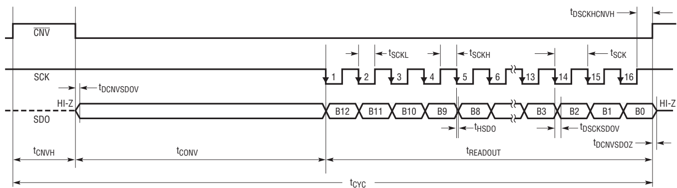
図21. LTC2310-12のタイミング図、CMOS、LVDS I/Oモード
