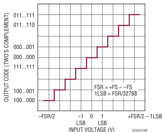
図2. LTC2310-12の伝達関数
