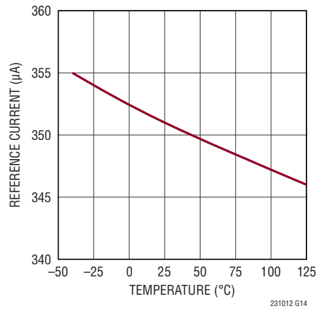
IREFOUTと温度、VREF = 4.096V
