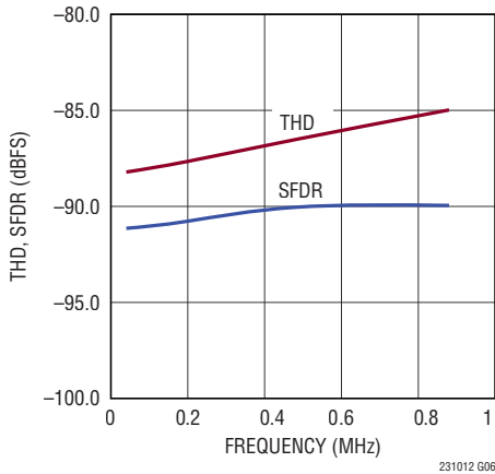
THDおよび高調波と周波数 (100kHz ~ 1MHz)
