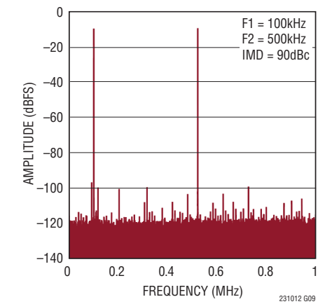
8kポイントのFFT、IMD、 f_{SAMPL} = 2\text{Mpsps} 、 A_{IN}^+ = 100\text{kHz} 、 A_{IN}^- = 500\text{kHz}
