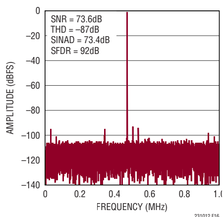
図16. LTC2310-12の32kポイントのFFT
