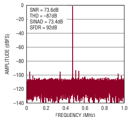
32k ポイントの FFT ( f_{SAMPL} = 2 Msps, f_{IN} = 500 kHz)
