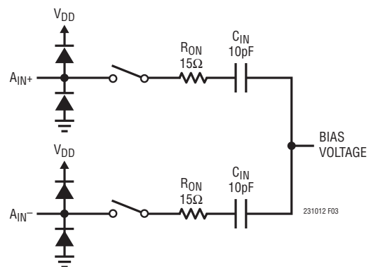
図3. LTC2310-12の差動アナログ入力の等価回路
