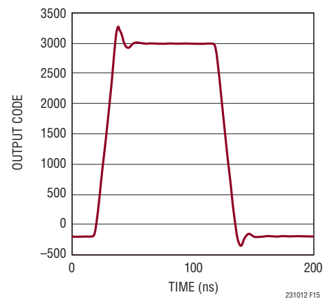
図 15. LTC2310-12 のトランジェント応答
