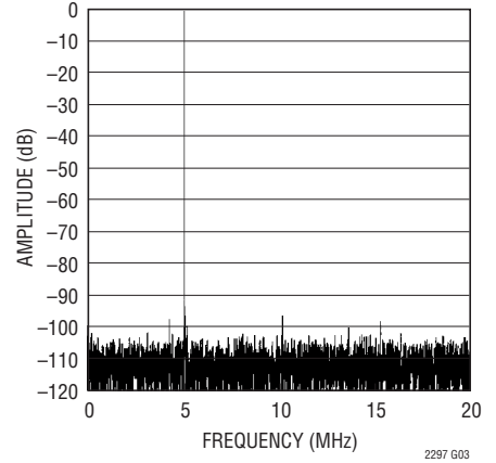
LTC2297: 8192 ポイントの FFT、 f_{IN} = 5\text{MHz} 、-1dB、2V レンジ、 40Msps
