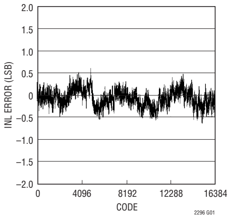
LTC2296: 標準的な INL、2Vレンジ、25Mps
