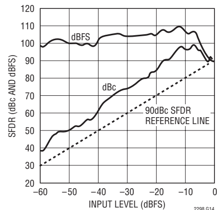
LTC2298: SFDRと入力レベル、 f_{IN} = 30\text{MHz} 、2Vレンジ、65Msps
