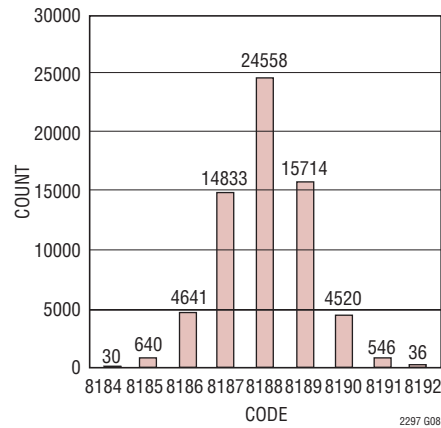
LTC2297: 接地入力時の ヒストグラム、40Msps
