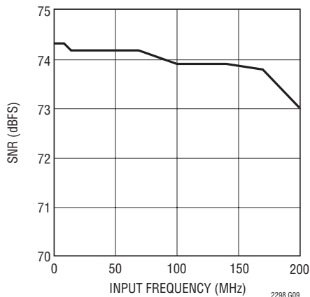
LTC2298: SNRと入力周波数、-1dB、2Vレンジ、65Msps
