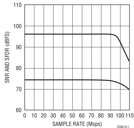
LTC2298: SNRおよびSFDRとサンプル・レート、2Vレンジ、 f_{IN} = 5\text{MHz} 、-1dB
