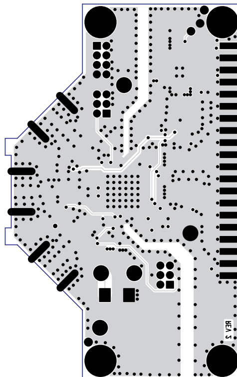
底面
