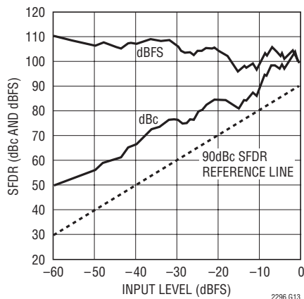
LTC2296: SFDRと入力レベル、 f_{IN} = 5\text{MHz} 、2Vレンジ、25Msps
