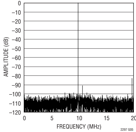
LTC2297: 8192 ポイントの FFT、 f_{IN} = 70\text{MHz} 、-1dB、2V レンジ、 40Msps
