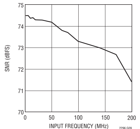
LTC2296: SNRと入力周波数、 -1\text{dB} 、 2\text{V} レンジ、 25\text{Mpsps}
