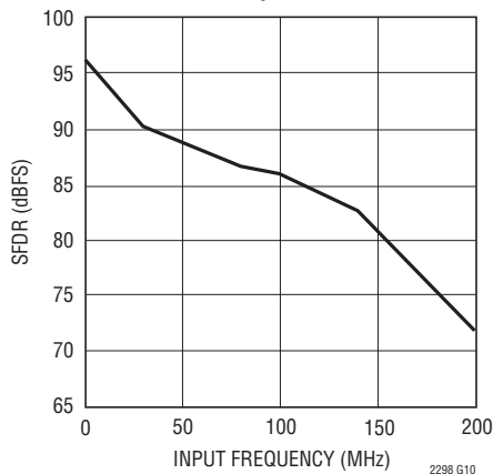
LTC2298: SFDRと入力周波数、-1dB、2Vレンジ、65Msps
