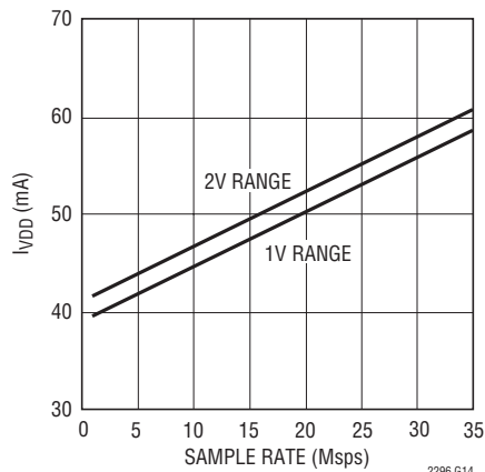
LTC2296: I_{VDD} とサンプル・レート、 5MHzの正弦波入力、-1dB
