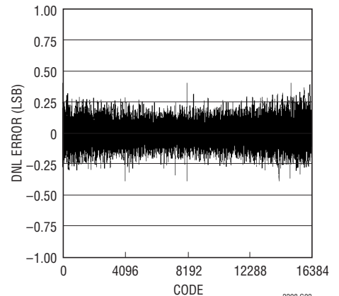
LTC2298: 標準的な DNL、 2Vレンジ、65Msps
