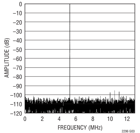
LTC2296: 8192ポイントのFFT、 f_{IN} = 5\text{MHz} 、-1dB、2Vレンジ、25Mps
