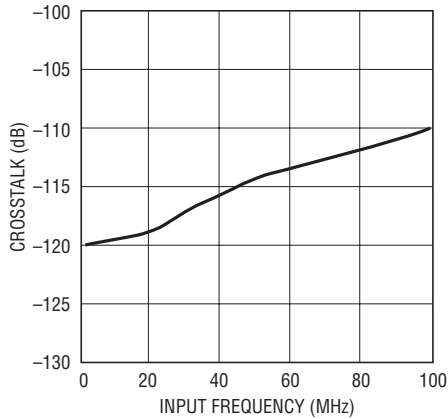
LTC2298/LTC2297/LTC2296: クロストークと入力周波数
