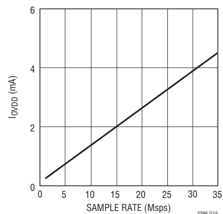
LTC2296: I_{VDD} とサンプル・レート、 5MHzの正弦波入力、-1dB、 V_{DD} = 1.8\text{V}
