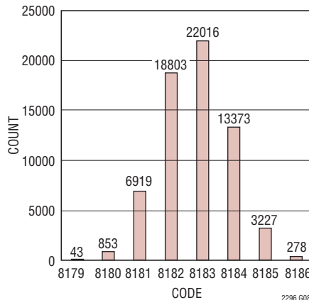
LTC2296: 接地入力時の ヒストグラム、 25\text{Mpsps}
