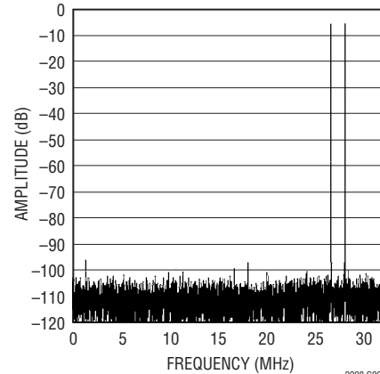
LTC2298: 8192ポイントの2トーン FFT、 f_{IN} = 28.2\text{MHz} および 26.8\text{MHz} 、 -1\text{dB} 、2Vレンジ、65Msps
