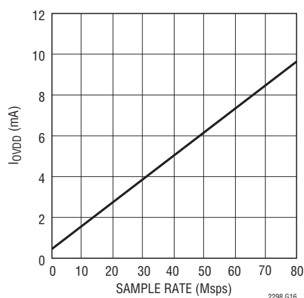
LTC2298: I_{OVD} とサンプル・レート、5MHzの正弦波入力、-1dB、 O_{VDD} = 1.8\text{V}
