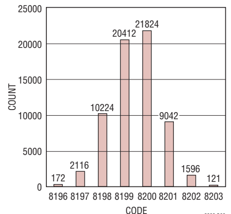
LTC2298: 接地入力時のヒストグラム、 65Msps
