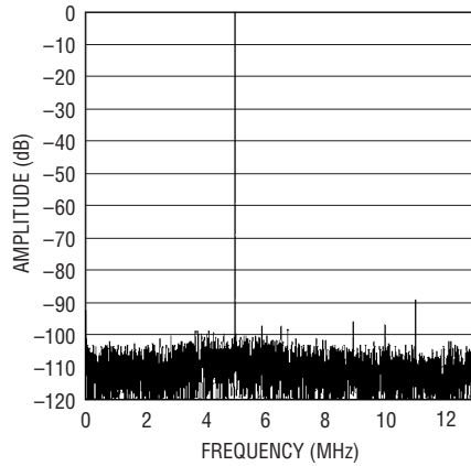
LTC2296: 8192ポイントのFFT、 f_{IN} = 70\text{MHz} 、 -1\text{dB} 、 2\text{V} レンジ、 25\text{Mpsps}
