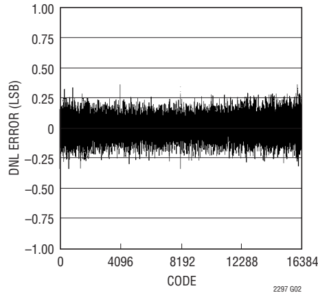
LTC2297: 標準的な DNL、 2V レンジ、40Msps
