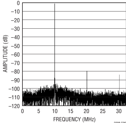
LTC2298: 8192ポイントのFFT、 f_{IN} = 140\text{MHz} 、 -1\text{dB} 、2Vレンジ、 65Msps
