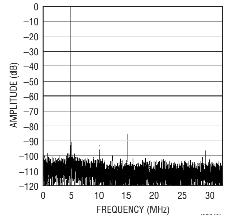
LTC2298: 8192ポイントのFFT、 f_{IN} = 70\text{MHz} 、 -1\text{dB} 、2Vレンジ、 65Msps
