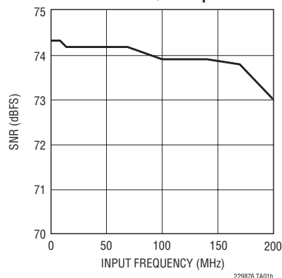
LTC2298: SNRと入力周波数、-1dB、2Vレンジ、65Msps
