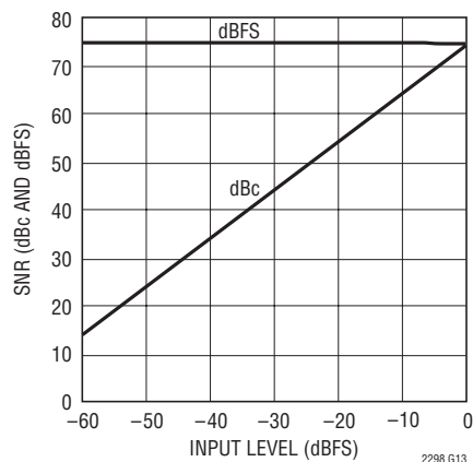
LTC2298: SNRと入力レベル、 f_{IN} = 30\text{MHz} 、2Vレンジ、65Msps
