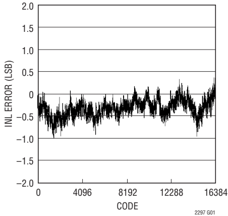
LTC2297: 標準的な INL、 2V レンジ、40Msps
