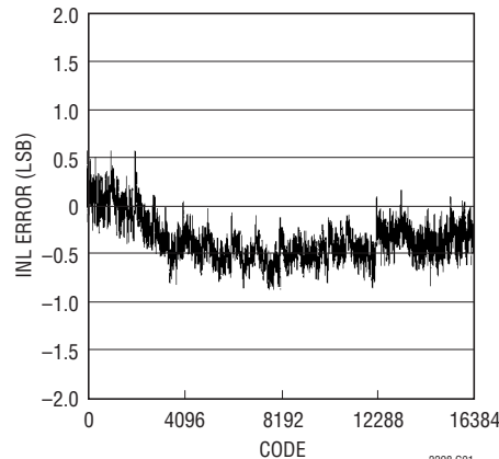
LTC2298: 標準的な INL、 2Vレンジ、65Msps
