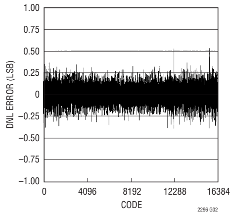
LTC2296: 標準的な DNL、2Vレンジ、25Mps
