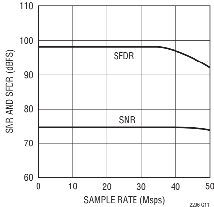
LTC2296: SNRおよびSFDRと サンプル・レート、 2\text{V} レンジ、 f_{IN} = 5\text{MHz} 、 -1\text{dB}
