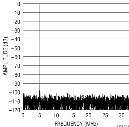
LTC2298: 8192ポイントのFFT、 f_{IN} = 5\text{MHz} 、 -1\text{dB} 、2Vレンジ、 65Msps
