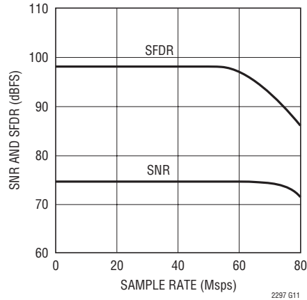
LTC2297: SNRおよびSFDRとサンプル・レート、2Vレンジ、 f_{IN} = 5\text{MHz} 、-1dB
