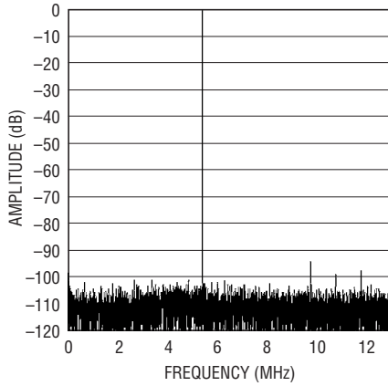
LTC2296: 8192ポイントのFFT、 f_{IN} = 30\text{MHz} 、 -1\text{dB} 、 2\text{V} レンジ、 25\text{Mpsps}
