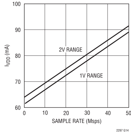
LTC2297: I_{VDD} とサンプル・レート、5MHzの正弦波入力、-1dB
