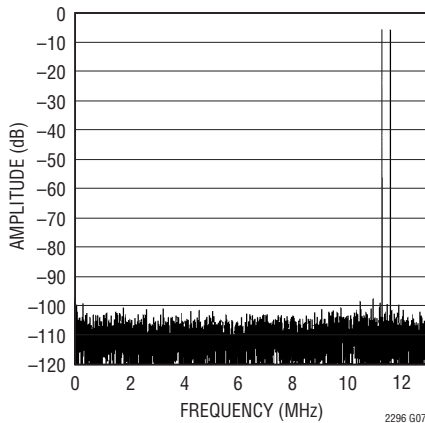
LTC2296: 8192ポイントの2トーン FFT、 f_{IN} = 10.9\text{MHz} および 13.8\text{MHz} 、 -1\text{dB} 、 2\text{V} レンジ、 25\text{Mpsps}
