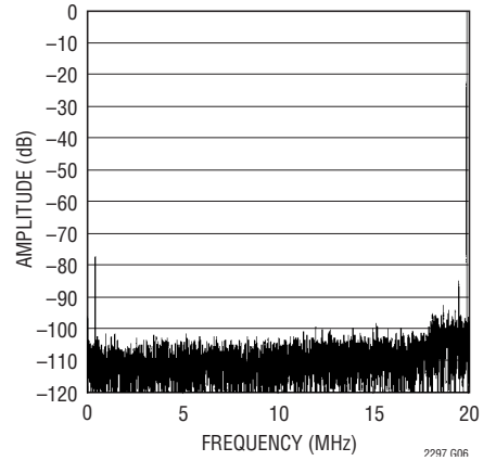
LTC2297: 8192 ポイントの FFT、 f_{IN} = 140\text{MHz} 、-1dB、2V レンジ、 40Msps
