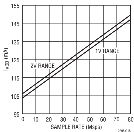
LTC2298: I_{VDD} とサンプル・レート、5MHzの正弦波入力、-1dB
