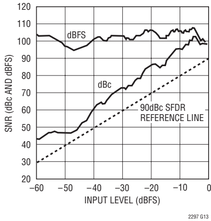
LTC2297: SFDRと入力レベル、 f_{IN} = 5\text{MHz} 、2Vレンジ、40Mps
