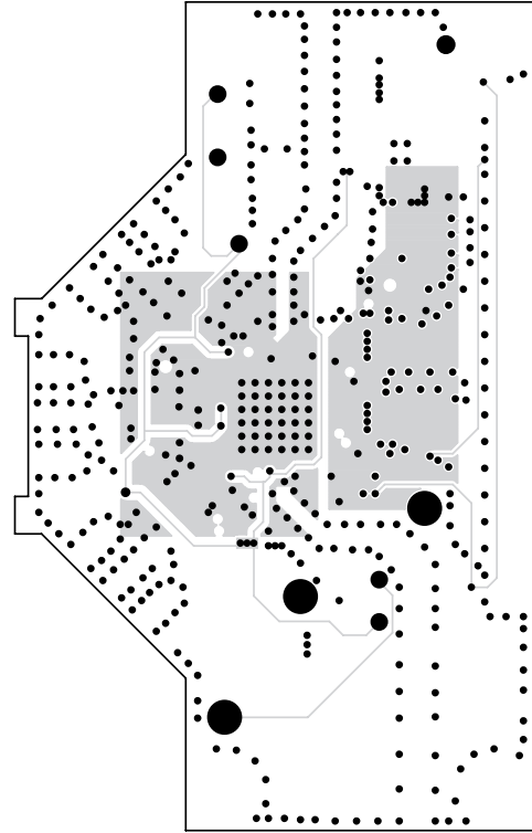
中間層 3 電源
