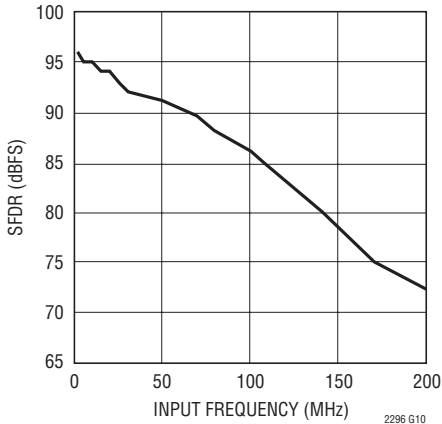
LTC2296: SFDRと入力周波数、 -1\text{dB} 、 2\text{V} レンジ、 25\text{Mpsps}
