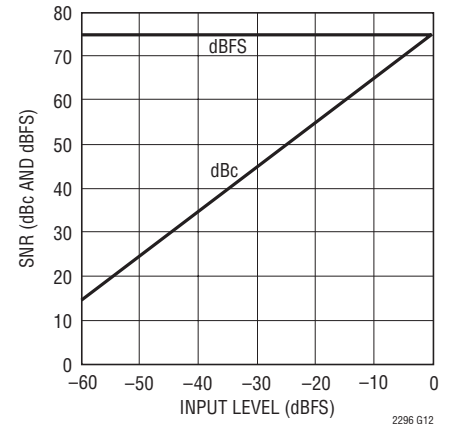
LTC2296: SNRと入力レベル、 f_{IN} = 5\text{MHz} 、 2\text{V} レンジ、 25\text{Mpsps}
