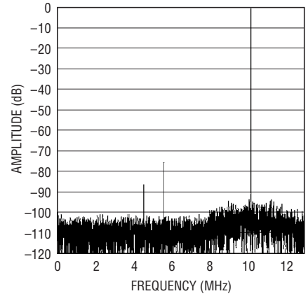
LTC2296: 8192ポイントのFFT、 f_{IN} = 140\text{MHz} 、 -1\text{dB} 、 2\text{V} レンジ、 25\text{Mpsps}
