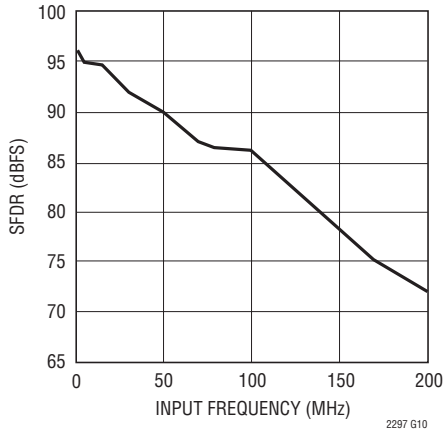
LTC2297: SFDRと入力周波数、-1dB、2Vレンジ、40Mps
