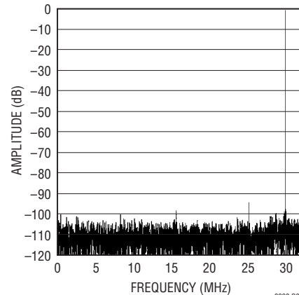
LTC2298: 8192ポイントのFFT、 f_{IN} = 30\text{MHz} 、 -1\text{dB} 、2Vレンジ、 65Msps
