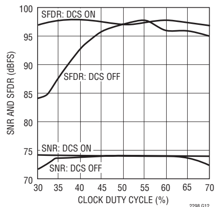
LTC2298: SNRおよびSFDRとクロック・デューティ・サイクル、65Msps
