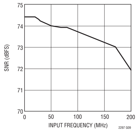
LTC2297: SNR と入力周波数、-1dB、 2V レンジ、40Msps
