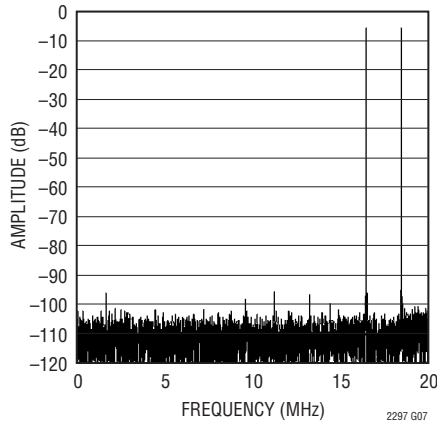
LTC2297: 8192 ポイントの 2 トーン FFT、 f_{IN} = 21.6\text{MHz} および 23.6\text{MHz} 、 -1dB、2V レンジ、40Msps
