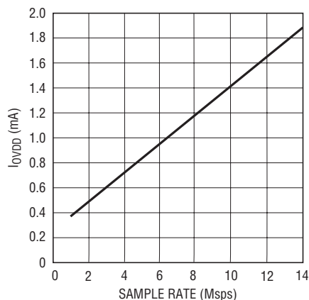
I_{OVD} とサンプル・レート、5MHzの 正弦波入力、 -1\text{dB} 、 0_{VDD} = 1.8\text{V}
