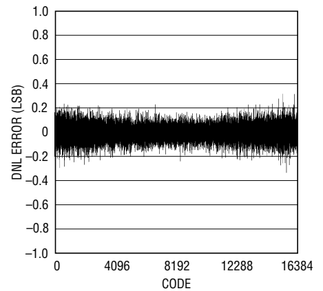
標準的なDNL、2Vレンジ
