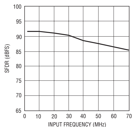
SFDRと入力周波数、 -1\text{dB} 、2Vレンジ
