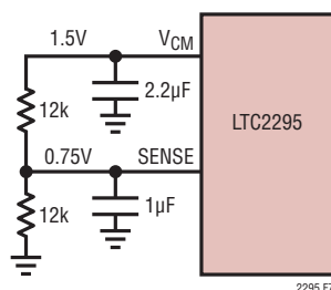
図7. 1.5VレンジのADC
