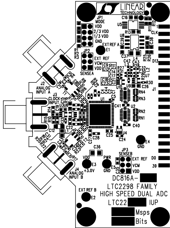
部品面シルク
