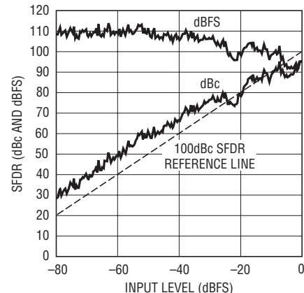
SFDRと入力レベル、 f_{IN} = 5\text{MHz} 、 2Vレンジ
