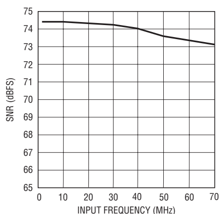
SNRと入力周波数、 -1\text{dB} 、2Vレンジ
