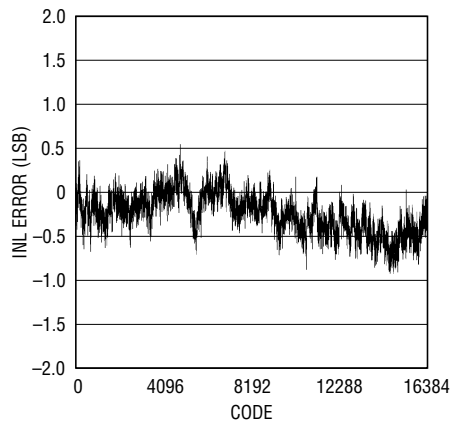
標準的なINL、2Vレンジ
