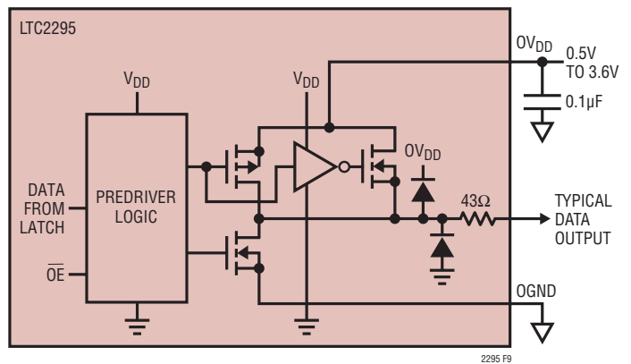
図9. デジタル出力バッファ
