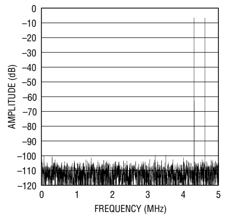
8192ポイントの2トーンFFT、 f_{IN} = 4.3\text{MHz} および 4.6\text{MHz} 、 -1\text{dB} 、2Vレンジ
