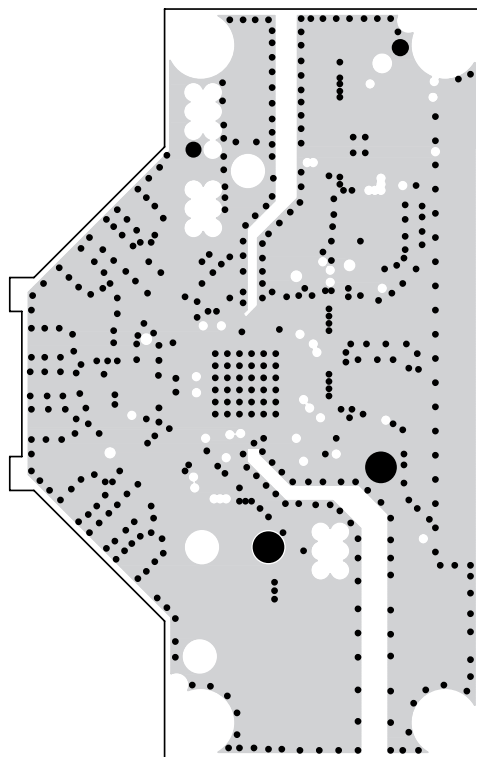
中間層3 電源
