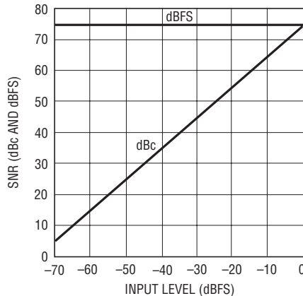
SNRと入力レベル、 f_{IN} = 5\text{MHz} 、 2Vレンジ
