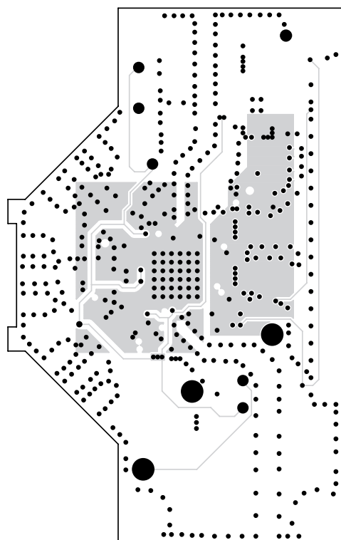
中間層3 電源
