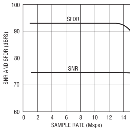
SNRおよびSFDRとサンプル・レート、 2Vレンジ、 f_{IN} = 5\text{MHz} 、 -1\text{dB}
