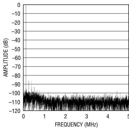
8192ポイントのFFT、 f_{IN} = 70.1\text{MHz} 、 -1\text{dB} 、2Vレンジ
