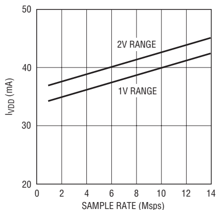
I_{VDD} とサンプル・レート、 5MHzの正弦波入力、 -1\text{dB}
