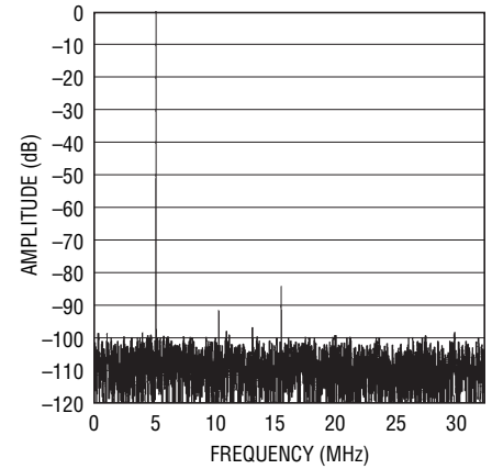
LTC2293: 8192 ポイントの FFT、 f_{IN} = 70\text{MHz} 、 -1\text{dB} 、2V レンジ、 65Msps
