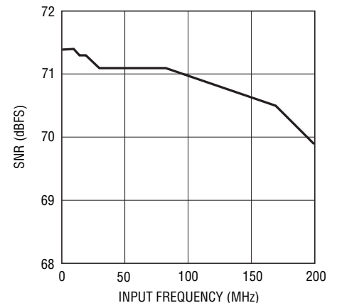
LTC2292: SNRと入力周波数、 -1\text{dB} 、2Vレンジ、40Mps
