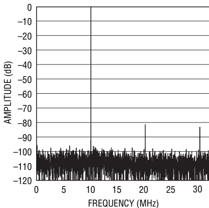
LTC2293: 8192 ポイントの FFT、 f_{IN} = 140\text{MHz} 、 -1\text{dB} 、2V レンジ、 65Msps
