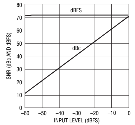
LTC2291: SNRと入力レベル、 f_{IN} = 5\text{MHz} 、 2\text{V} レンジ、 25\text{Mpsps}
