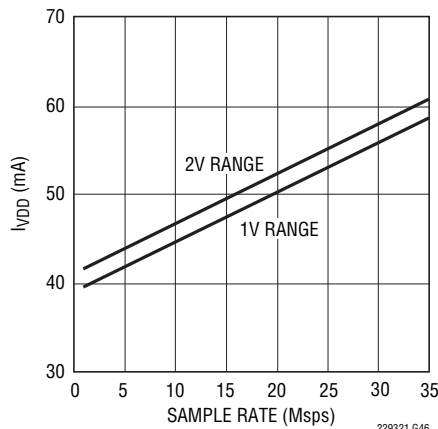
LTC2291: I_{VDD} とサンプル・レート、 5MHzの正弦波入力、-1dB
