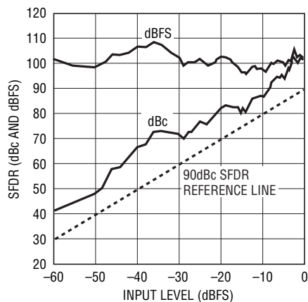
LTC2291: SFDRと入力レベル、 f_{IN} = 5\text{MHz} 、2Vレンジ、25Msps
