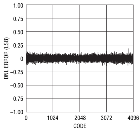
LTC2291: 標準的な DNL、2Vレンジ、25Msps
