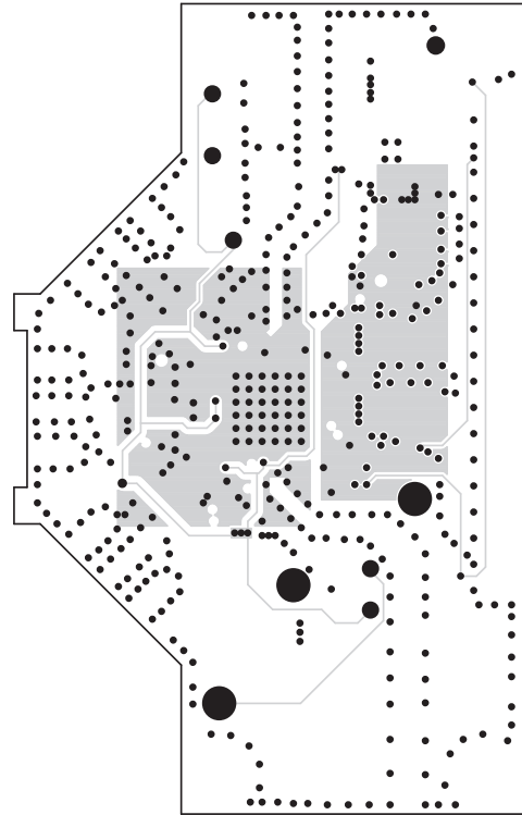
中間層 3 電源
