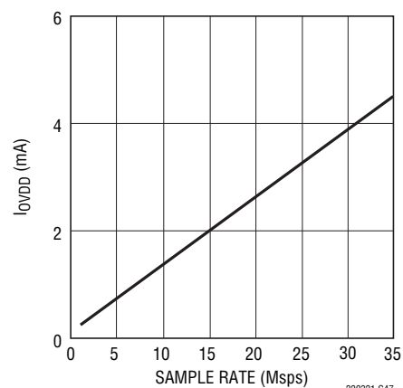
LTC2291: I_{VDD} とサンプル・レート、 5MHzの正弦波入力、-1dB、 V_{DD} = 1.8\text{V}
