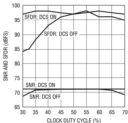
LTC2293: SNRおよびSFDRと クロック・デューティ・サイクル、 65Mpsps
