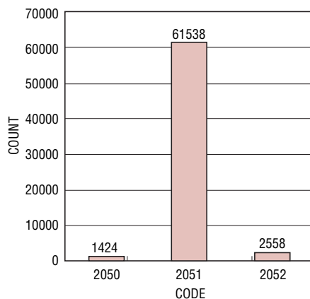
LTC2292: 接地入力時の ヒストグラム、40Mps
