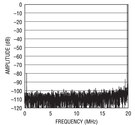
LTC2292: 8192ポイントのFFT、 f_{IN} = 140\text{MHz} 、 -1\text{dB} 、2Vレンジ、 40Mps
