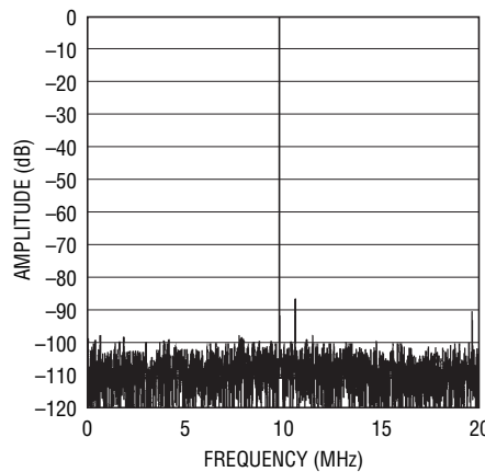
LTC2292: 8192ポイントのFFT、 f_{IN} = 70\text{MHz} 、 -1\text{dB} 、2Vレンジ、 40Mps
