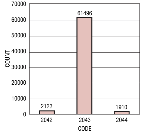
LTC2293: 接地入力時の ヒストグラム、65Msps
