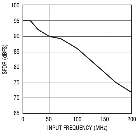
LTC2291: SFDRと入力周波数、 -1\text{dB} 、 2\text{V} レンジ、 25\text{Mpsps}
