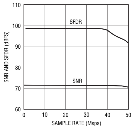
LTC2291: SNRおよびSFDRと サンプル・レート、 2\text{V} レンジ、 f_{IN} = 5\text{MHz} 、 -1\text{dB}
