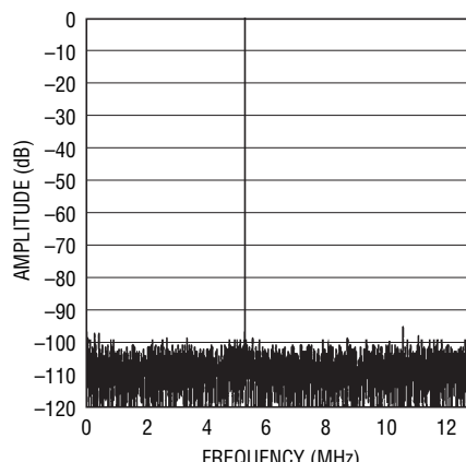
LTC2291: 8192ポイントのFFT、 f_{IN} = 5\text{MHz} 、-1dB、2Vレンジ、25Msps
