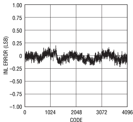
LTC2291: 標準的な INL、2Vレンジ、25Msps
