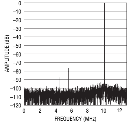
LTC2292: 8192ポイントのFFT、 f_{IN} = 140\text{MHz} 、 -1\text{dB} 、 2\text{V} レンジ、 25\text{Mpsps}
