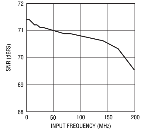
LTC2291: SNRと入力周波数、 -1\text{dB} 、 2\text{V} レンジ、 25\text{Mpsps}
