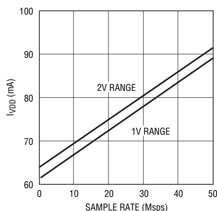
LTC2292: I_{VDD} とサンプル・レート、5MHzの正弦波入力、-1dB
