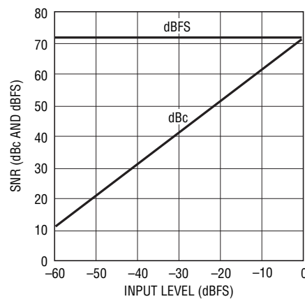
LTC2293: SNRと入力レベル、 f_{IN} = 30\text{MHz} 、2Vレンジ、 65Mpsps
