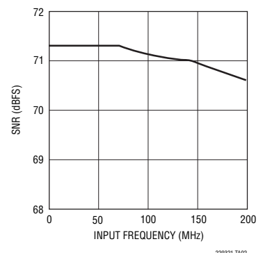
LTC2293: SNRと入力周波数、 -1dB、2Vレンジ、65Msps
