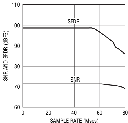
LTC2292: SNRおよびSFDRとサンプル・レート、2Vレンジ、 f_{IN} = 5\text{MHz} 、-1dB
