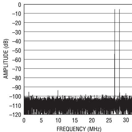
LTC2293: 8192 ポイントの 2 トーン FFT、 f_{IN} = 28.2\text{MHz} および 26.8\text{MHz} 、 -1\text{dB} 、2V レンジ、65Msps
