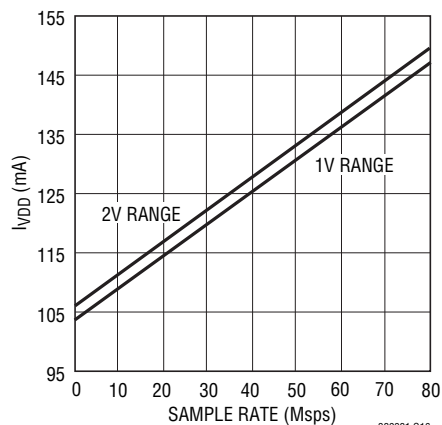
LTC2293: I_{VDD} とサンプル・レート、 5MHzの正弦波入力、-1dB
