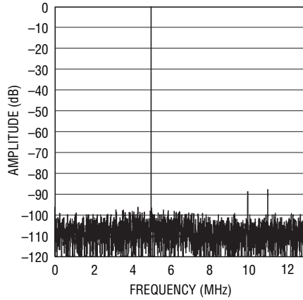
LTC2292: 8192ポイントのFFT、 f_{IN} = 70\text{MHz} 、 -1\text{dB} 、 2\text{V} レンジ、 25\text{Mpsps}
