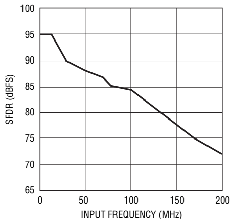
LTC2292: SFDRと入力周波数、-1dB、2Vレンジ、40Msps
