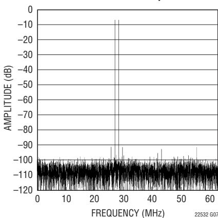
LTC2253: 8192 ポイントの 2 トーン FFT、 f_{IN} = 28.2\text{MHz} および 26.8\text{MHz} 、 -1\text{dB} 、2V レンジ、125Msps
