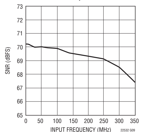
LTC2253: SNR と入力周波数、 -1\text{dB} 、2V レンジ、125Msps
