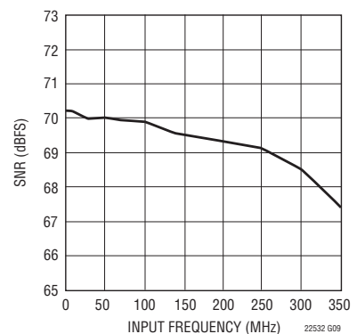
LTC2253: SNRと入力周波数、-1dB、2Vレンジ、125MSPS
