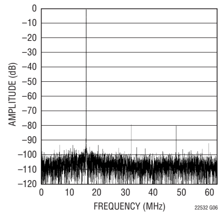
LTC2253: 8192 ポイントの FFT、 f_{IN} = 140\text{MHz} 、 -1\text{dB} 、2V レンジ、125Msps
