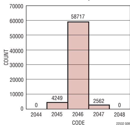
LTC2253: 接地入力時のヒストグラム、125Msps
