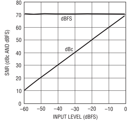
LTC2252: SNRと入力レベル、 f_{IN} = 70\text{MHz} 、2Vレンジ、105Mpsps
