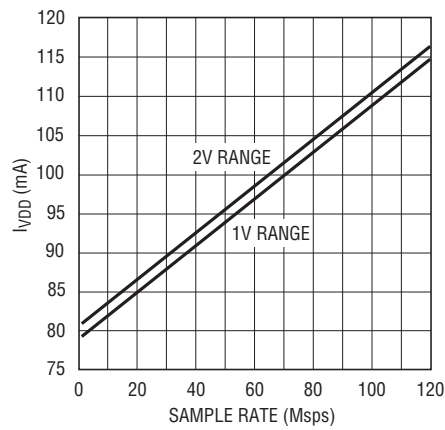
LTC2252: I_{VDD} とサンプル・レート、 5MHzの正弦波入力、-1dB
