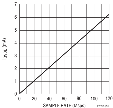
LTC2252: I_{VDD} とサンプル・レート、 5MHzの正弦波入力、-1dB、 OV_{DD} = 1.8\text{V}
