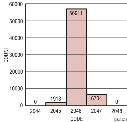
LTC2252: 接地入力時のヒストグラム、105Mps
