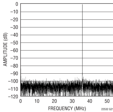
LTC2252: 8192 ポイントの FFT、 f_{IN} = 70\text{MHz} 、 -1\text{dB} 、2V レンジ、105Mps
