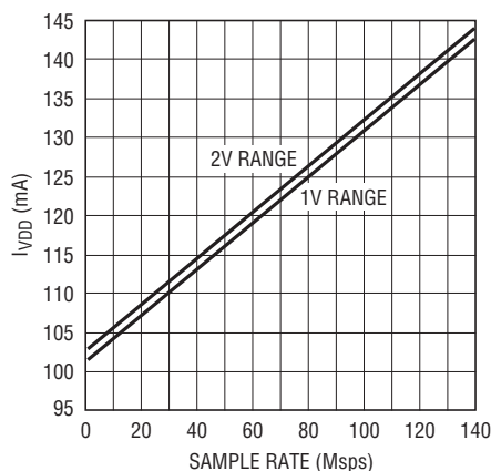
LTC2253: I_{VDD} とサンプル・レート、5MHzの正弦波入力、-1dB
