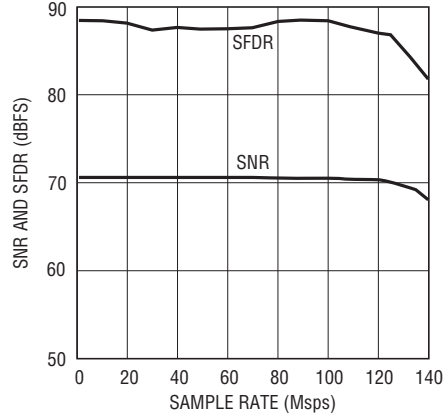
LTC2252: SNRおよびSFDRと サンプル・レート、2Vレンジ、 f_{IN} = 5\text{MHz} 、-1dB
