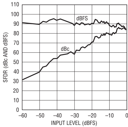
LTC2252: SFDRと入力レベル、 f_{IN} = 70\text{MHz} 、2Vレンジ、105Mpsps
