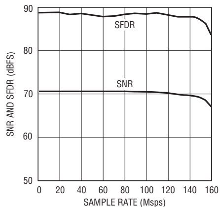
LTC2253: SNRおよびSFDRとサンプル・レート、2Vレンジ、 f_{IN} = 5\text{MHz} 、-1dB
