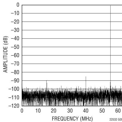
LTC2253: 8192 ポイントの FFT、 f_{IN} = 70\text{MHz} 、 -1\text{dB} 、2V レンジ、125Msps
