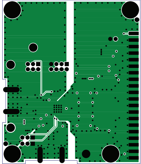
上面
