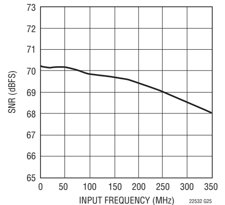
LTC2252: SNR と入力周波数、 -1\text{dB} 、2V レンジ、105Mps
