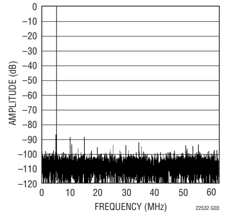
LTC2253: 8192 ポイントの FFT、 f_{IN} = 5\text{MHz} 、 -1\text{dB} 、2V レンジ、125Msps
