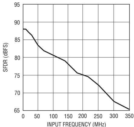
LTC2253: SFDRと入力周波数、-1dB、2Vレンジ、125Msps
