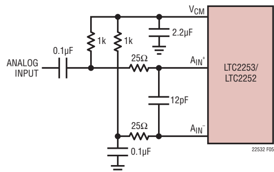
図5. シングルエンドのドライブ
