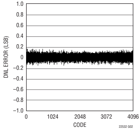
LTC2253: 標準的な DNL、2V レンジ、125Msps
