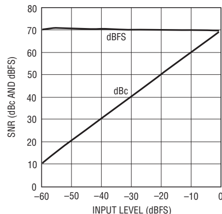
LTC2253: SNRと入力レベル、 f_{IN} = 70\text{MHz} 、2Vレンジ、125Msps
