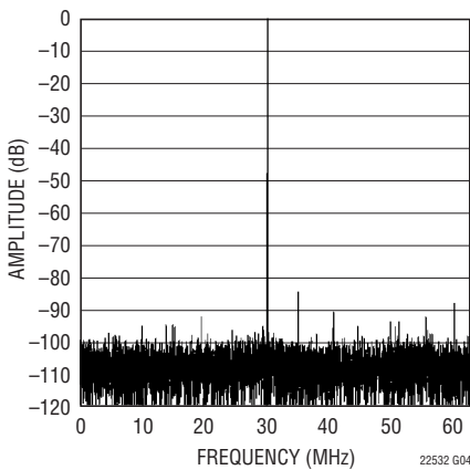
LTC2253: 8192 ポイントの FFT、 f_{IN} = 30\text{MHz} 、 -1\text{dB} 、2V レンジ、125Msps
