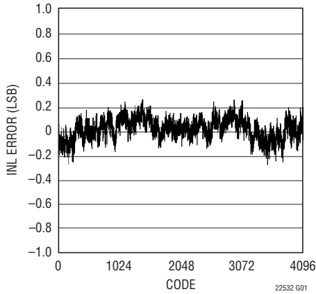
LTC2253: 標準的な INL、2V レンジ、125Msps
