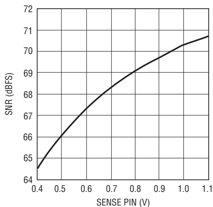
LTC2253: SNRとSENSEの電圧、 f_{IN} = 5\text{MHz} 、-1dB
