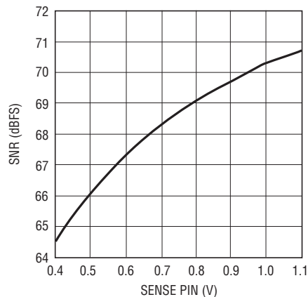
LTC2252: SNRとSENSEの電圧、 f_{IN} = 5\text{MHz} 、-1dB
