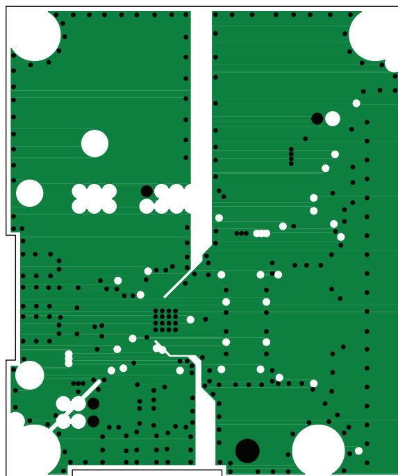
中間層2 GND
