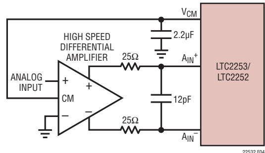
図4. アンプを使った差動ドライブ
