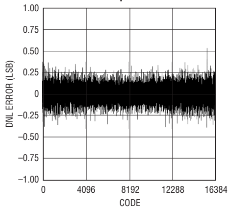
LTC2246: 標準的な DNL、 2Vレンジ、25Mps
