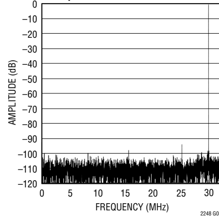
LTC2248: 8192ポイントのFFT、 f_{IN} = 30\text{MHz} 、 -1\text{dB} 、 2\text{V} レンジ、 65\text{Msps}
