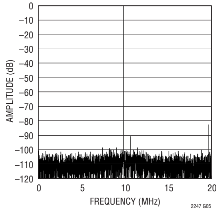
LTC2247: 8192ポイントのFFT、 f_{IN} = 70\text{MHz} 、 -1\text{dB} 、 2\text{V} レンジ、 40\text{Msps}
