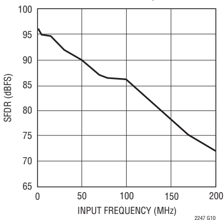
LTC2247: SFDRと入力周波数、 -1\text{dB} 、 2\text{V} レンジ、 40\text{Msps}
