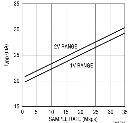
LTC2246: I_{VDD} とサンプル・レート、 5MHzの正弦波入力、-1dB
