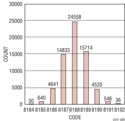
LTC2247: 接地入力時の ヒストグラム、 40\text{Msps}
