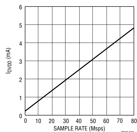
LTC2248: I_{OVD} とサンプル・レート、 5MHzの正弦波入力、 -1\text{dB} 、 O_{VDD} = 1.8\text{V}
