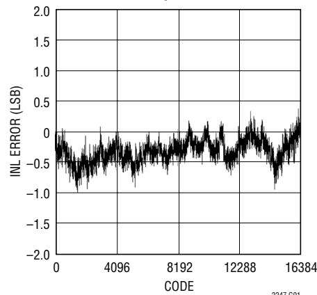
LTC2247: 標準的な INL、 2Vレンジ、40MSPS
