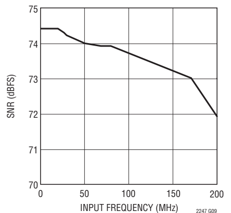
LTC2247: SNRと入力周波数、 -1\text{dB} 、 2\text{V} レンジ、 40\text{Msps}
