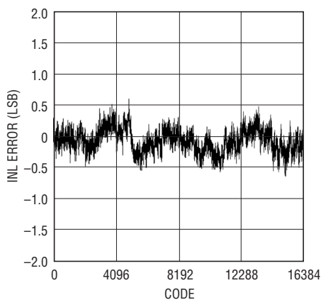
LTC2246: 標準的な INL、 2Vレンジ、25Mps
