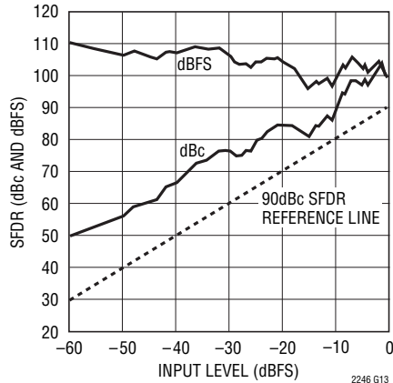
LTC2246: SFDRと入力レベル、 f_{IN} = 5\text{MHz} 、2Vレンジ、25Msps
