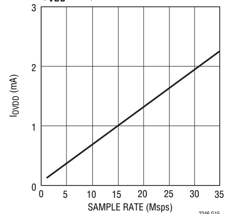
LTC2246: I_{OVD} とサンプル・レート、 5MHzの正弦波入力、-1dB、 O_{VDD} = 1.8\text{V}
