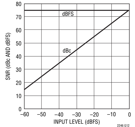
LTC2246: SNRと入力レベル、 f_{IN} = 5\text{MHz} 、2Vレンジ、25Msps
