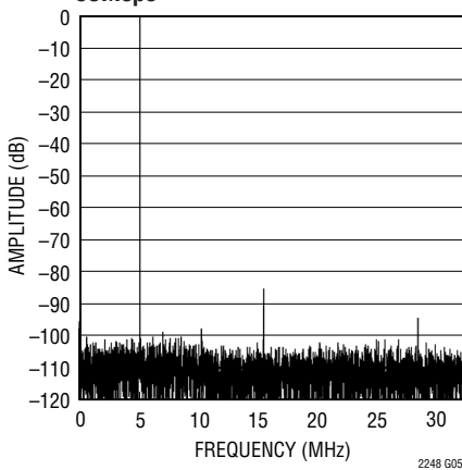
LTC2248: 8192ポイントのFFT、 f_{IN} = 70\text{MHz} 、 -1\text{dB} 、 2\text{V} レンジ、 65\text{Msps}
