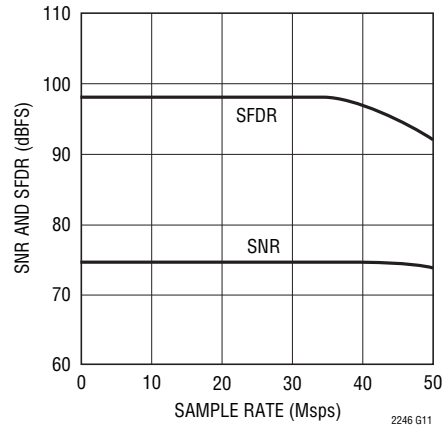
LTC2246: SNRおよびSFDRと サンプル・レート、2Vレンジ、 f_{IN} = 5\text{MHz} 、-1dB
