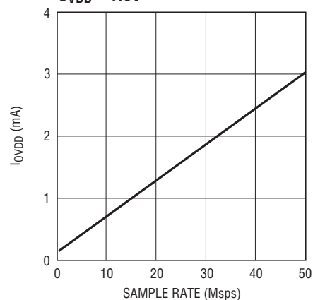
LTC2247: I_{VDD} とサンプル・レート、 5MHzの正弦波入力、-1dB、 O_{VDD} = 1.8\text{V}
