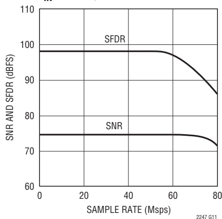
LTC2247: SNRおよびSFDRと サンプル・レート、 2\text{V} レンジ、 f_{IN} = 5\text{MHz} 、 -1\text{dB}
