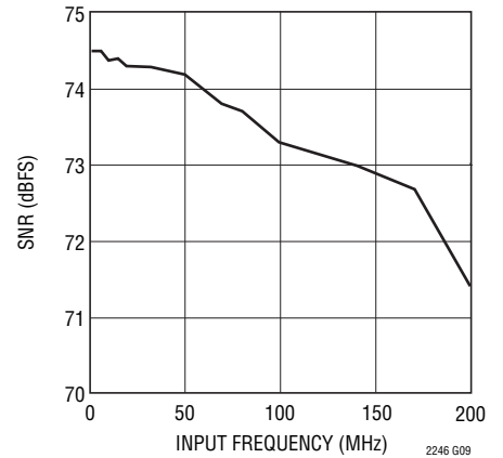
LTC2246: SNRと入力周波数、-1dB、 2Vレンジ、25Msps
