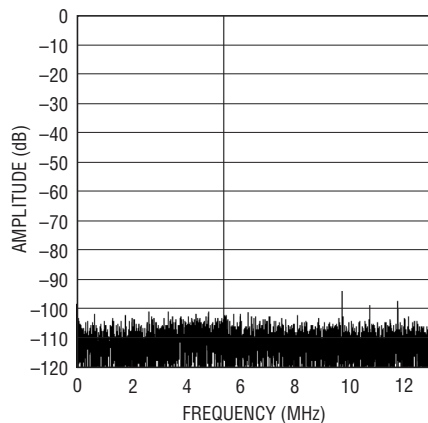
LTC2246: 8192ポイントのFFT、 f_{IN} = 30\text{MHz} 、-1dB、2Vレンジ、 25Mps
