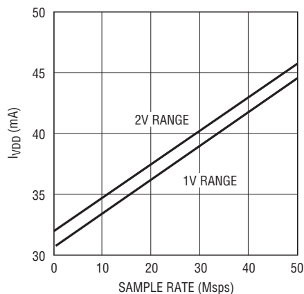
LTC2247: I_{VDD} とサンプル・レート、 5MHzの正弦波入力、-1dB
