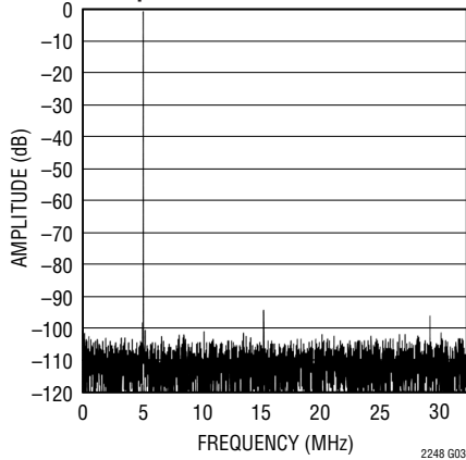
LTC2248: 8192ポイントのFFT、 f_{IN} = 5\text{MHz} 、 -1\text{dB} 、 2\text{V} レンジ、 65\text{Msps}
