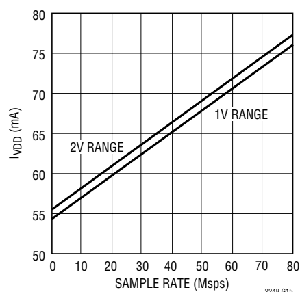
LTC2248: I_{VDD} とサンプル・レート、 5MHzの正弦波入力、 -1\text{dB}
