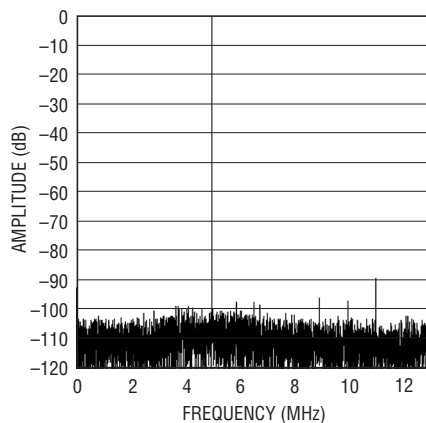
LTC2246: 8192ポイントのFFT、 f_{IN} = 70\text{MHz} 、-1dB、2Vレンジ、 25Mps
