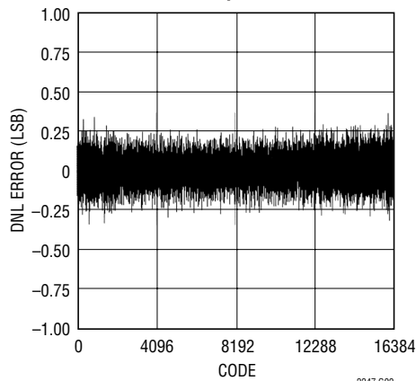
LTC2247: 標準的な DNL、 2Vレンジ、40MSPS
