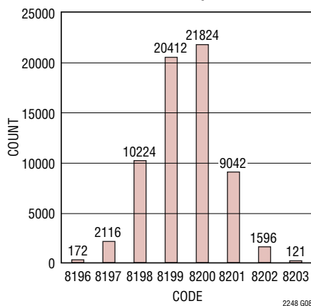
LTC2248: 接地入力時の ヒストグラム、 65\text{Msps}
