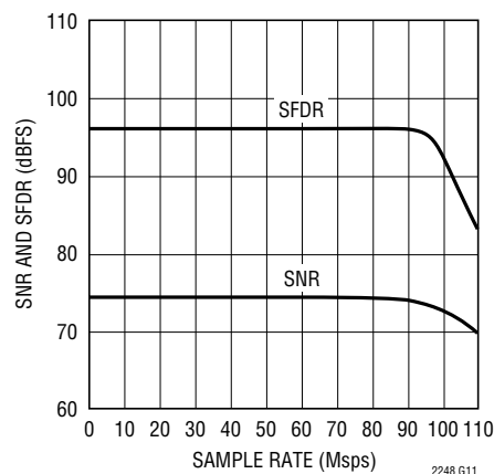
LTC2248: SNR および SFDR と サンプル・レート、2Vレンジ、 f_{IN} = 5\text{MHz} 、 -1\text{dB}
