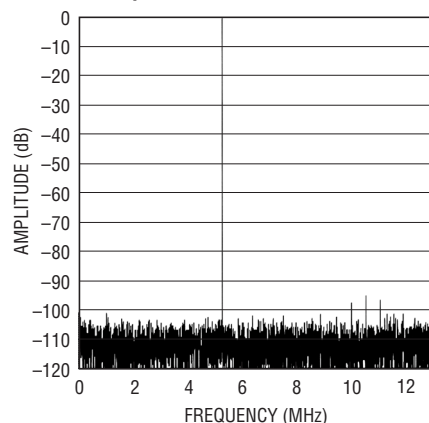
LTC2246: 8192ポイントのFFT、 f_{IN} = 5\text{MHz} 、-1dB、2Vレンジ、 25Mps
