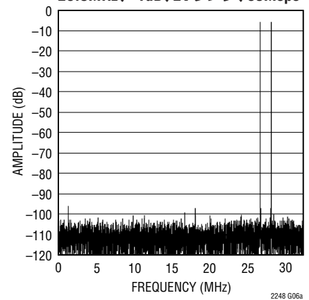
LTC2248: 8192ポイントの 2トーン FFT、 f_{IN} = 28.2\text{MHz} および 26.8\text{MHz} 、 -1\text{dB} 、 2\text{V} レンジ、 65\text{Msps}
