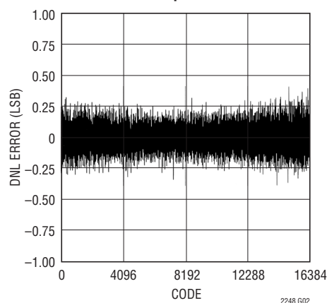
LTC2248: 標準的な DNL、 2V レンジ、65Msps
