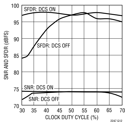
LTC2248: SNR、SFDRとクロック・ デューティ・サイクル、65MSPS
