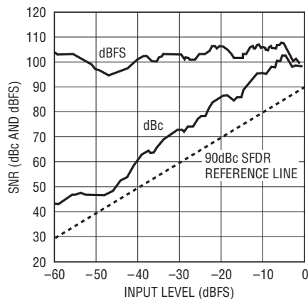
LTC2247: SFDRと入力レベル、 f_{IN} = 5\text{MHz} 、2Vレンジ、40Mps
