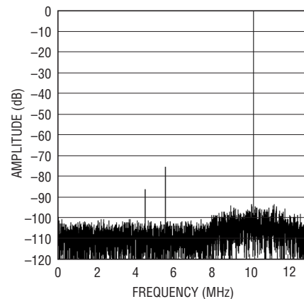
LTC2246: 8192ポイントのFFT、 f_{IN} = 140\text{MHz} 、-1dB、2Vレンジ、 25Mps
