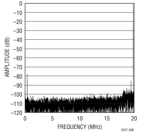
LTC2247: 8192ポイントのFFT、 f_{IN} = 140\text{MHz} 、 -1\text{dB} 、 2\text{V} レンジ、 40\text{Msps}
