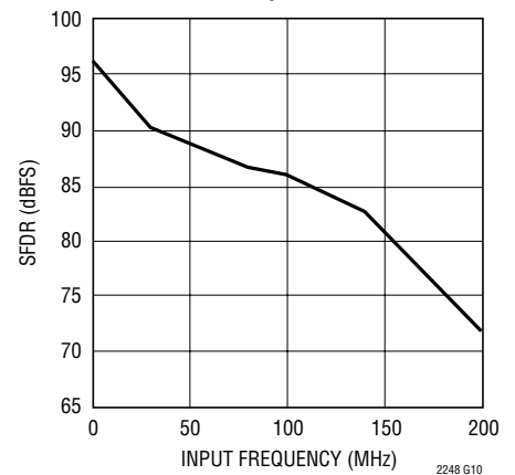
LTC2248: SFDRと入力周波数、 -1\text{dB} 、 2\text{V} レンジ、 65\text{Msps}
