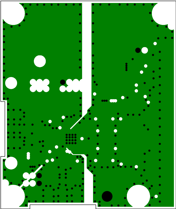
中間層 2 GND
