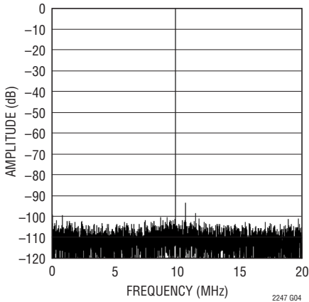
LTC2247: 8192ポイントのFFT、 f_{IN} = 30\text{MHz} 、 -1\text{dB} 、 2\text{V} レンジ、 40\text{Msps}
