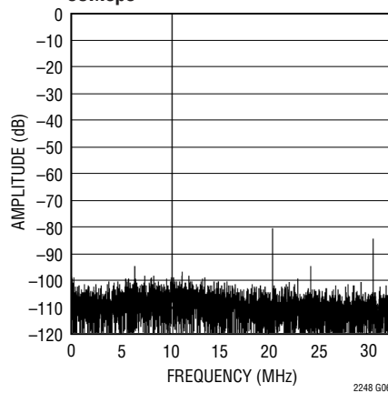
LTC2248: 8192ポイントのFFT、 f_{IN} = 140\text{MHz} 、 -1\text{dB} 、 2\text{V} レンジ、 65\text{Msps}
