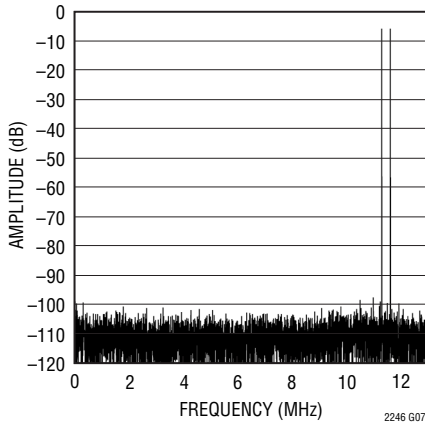
LTC2246: 8192ポイントの2トーン FFT、 f_{IN} = 10.9\text{MHz} および 13.8\text{MHz} 、 -1dB、2Vレンジ、25Msps
