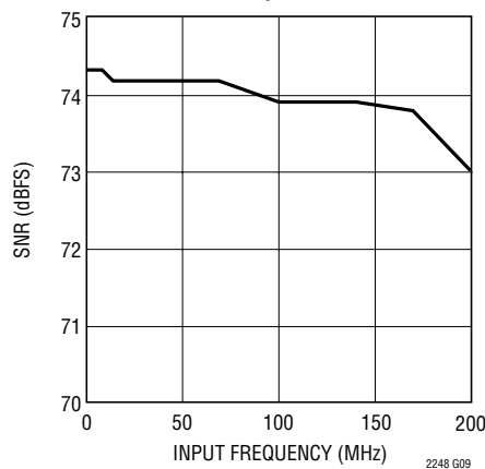
LTC2248: SNRと入力周波数、 -1\text{dB} 、 2\text{V} レンジ、 65\text{Msps}
