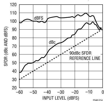
LTC2248: SFDRと入力レベル、 f_{IN} = 30\text{MHz} 、2Vレンジ、65MSPS
