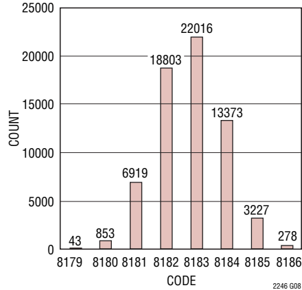
LTC2246: 接地入力時の ヒストグラム、25Msps
