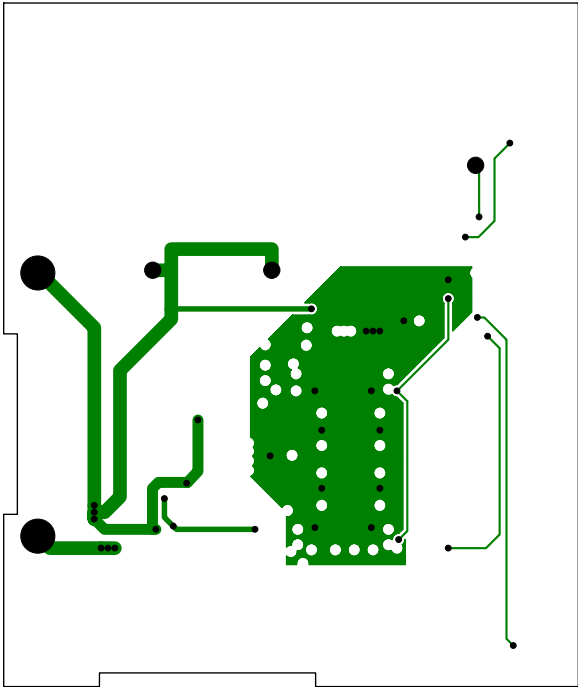
中間層 3 電源
