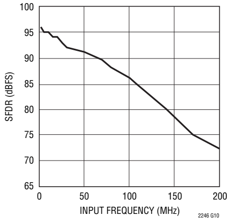
LTC2246: SFDRと入力周波数、 -1dB、2Vレンジ、25Msps
