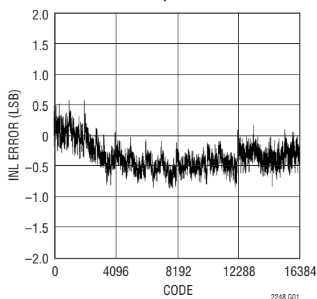
LTC2248: 標準的な INL、 2V レンジ、65Msps
