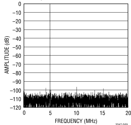
LTC2247: 8192 ポイントの FFT、 f_{IN} = 5\text{MHz} 、 -1\text{dB} 、2Vレンジ、 40MSPS
