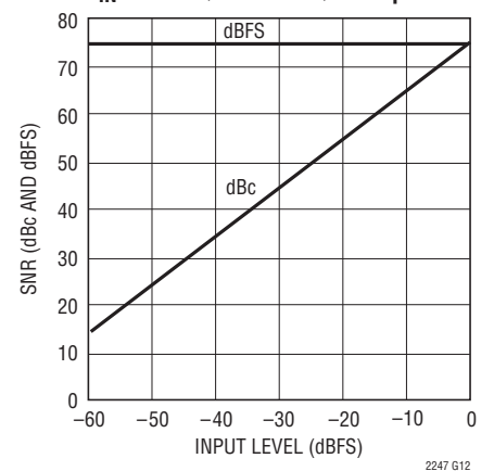
LTC2247: SNRと入力レベル、 f_{IN} = 5\text{MHz} 、 2\text{V} レンジ、 40\text{Msps}
