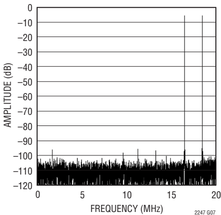
LTC2247: 8192ポイントの2トーン FFT、 f_{IN} = 21.6\text{MHz} および 23.6\text{MHz} 、 -1\text{dB} 、 2\text{V} レンジ、 40\text{Msps}
