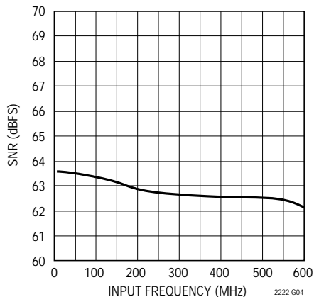
LTC2222 : SNRと入力周波数、 - 1dB、1Vレンジ
