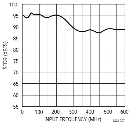
LTC2222 : SFDR (HD4+) と入力 周波数、- 1dB、2Vレンジ
