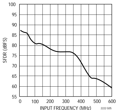
LTC2222 : SFDR (HD2とHD3) と 入力周波数、- 1dB、2Vレンジ
