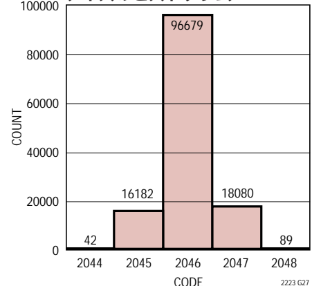
LTC2222 : ノイズのヒストグラム
