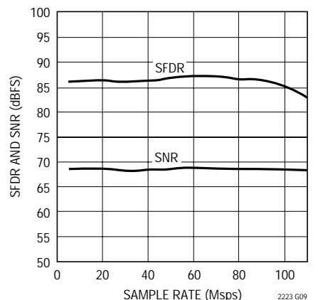
LTC2223 : SFDRおよびSNRと サンプル・レート、2Vレンジ、 f_{IN} = 30\text{MHz} 、 - 1dB
