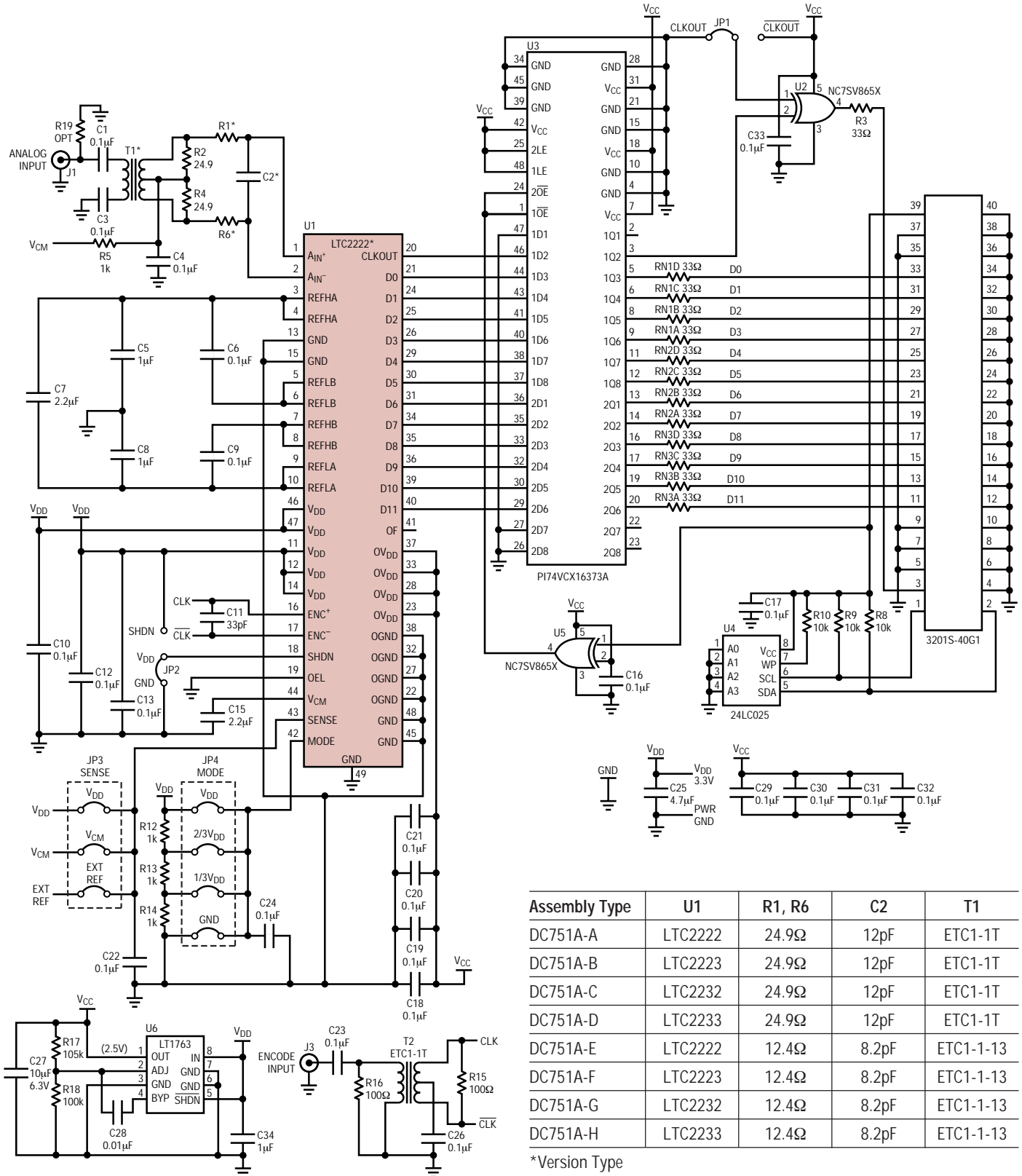
LTC2222の評価回路図
