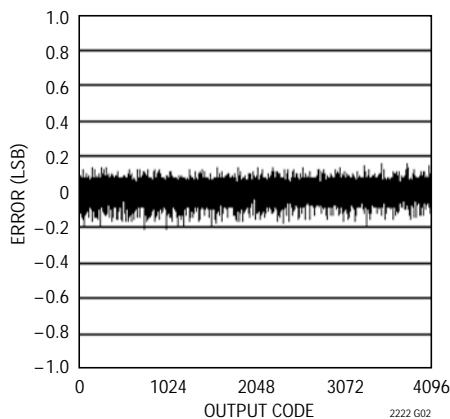
LTC2222 : DNL、2Vレンジ
