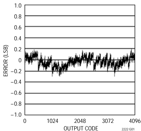
LTC2222 : INL、2Vレンジ
