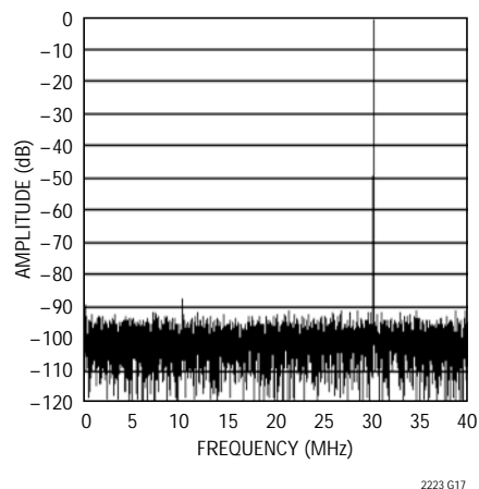
LTC2223 : 8192ポイントの FFT、 f_{IN} = 30\text{MHz} 、 -1\text{dB} 、 1Vレンジ
