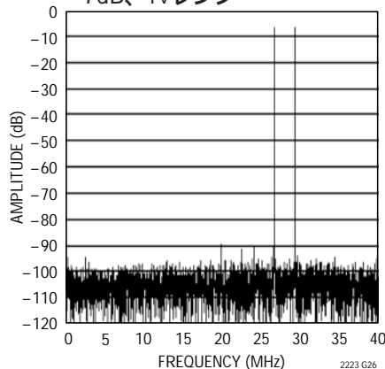
LTC2223 : 8192ポイントの 2トーンFFT、 f_{IN} = 138\text{MHz} および140MHz、それぞれ -7\text{dB} 、1Vレンジ
