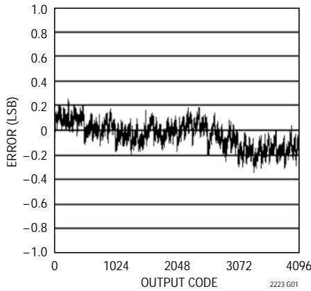
LTC2223 : INL、2Vレンジ
