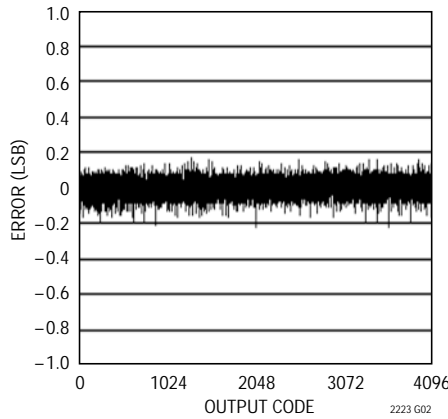
LTC2223 : DNL、2Vレンジ
