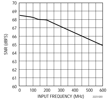
LTC2223 : SNRと入力周波数、 - 1dB、2Vレンジ
