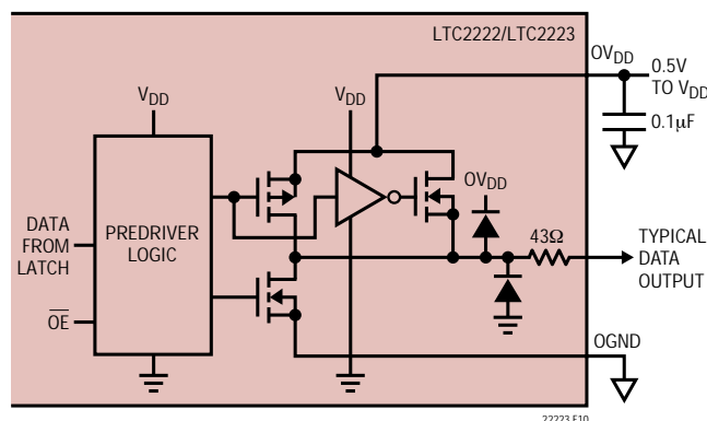
図13 . デジタル出力のバッファ
