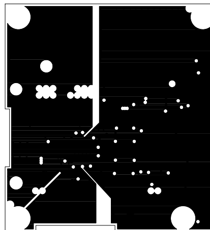
2層 GNDプレーン
