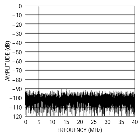
LTC2223 : 8192ポイントの FFT、 f_{IN} = 70\text{MHz} 、 -1\text{dB} 、 2Vレンジ
