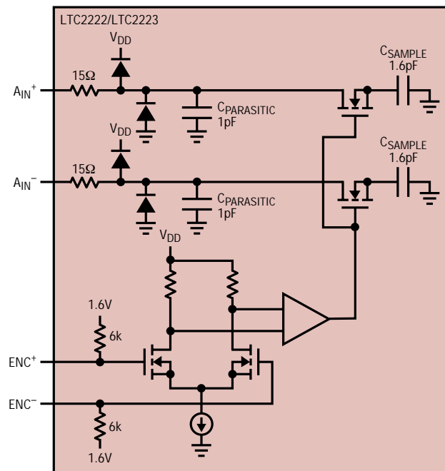
図2 . 等価入力回路
