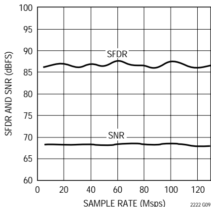
LTC2222 : SFDRおよびSNRと サンプル・レート、2Vレンジ、 f_{IN} = 30\text{MHz} 、- 1dB
