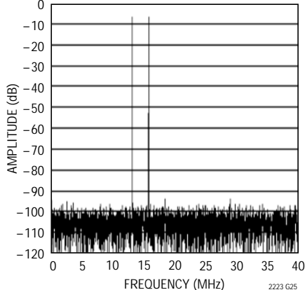
LTC2222 : 8192ポイントの 2トーンFFT、 f_{IN} = 68\text{MHz} および70MHz、それぞれ -7\text{dB} 、2Vレンジ
