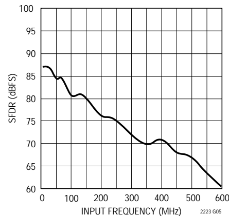
LTC2223 : SFDR (HD2とHD3) と 入力周波数、 - 1dB、2Vレンジ
