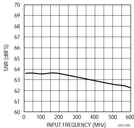
LTC2223 : SNRと入力周波数、 - 1dB、1Vレンジ
