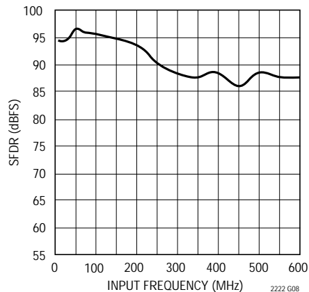
LTC2222 : SFDR (HD4+) と入力 周波数、- 1dB、1Vレンジ
