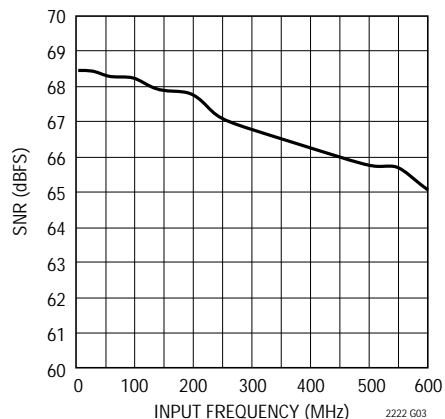
LTC2222 : SNRと入力周波数、 - 1dB、2Vレンジ
