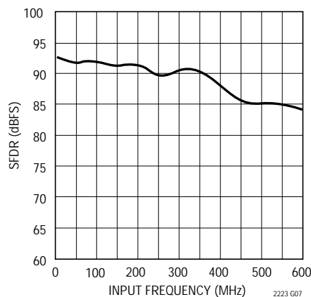
LTC2223 : SFDR (HD4+) と入力 周波数、 - 1dB、2Vレンジ
