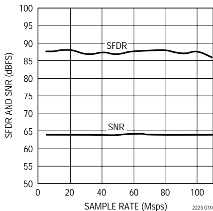
LTC2223 : SFDRおよびSNRと サンプル・レート、1Vレンジ、 f_{IN} = 30\text{MHz} 、 -1\text{dB}
