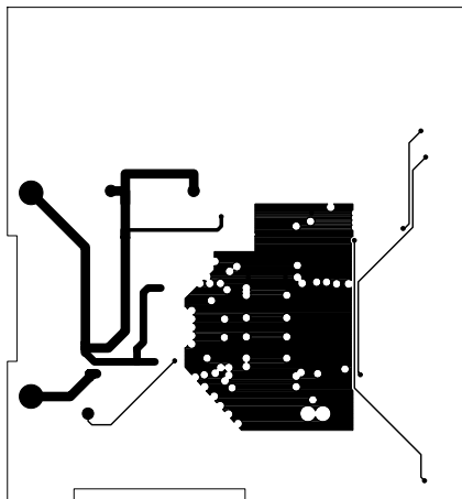
3層 電源プレーン
