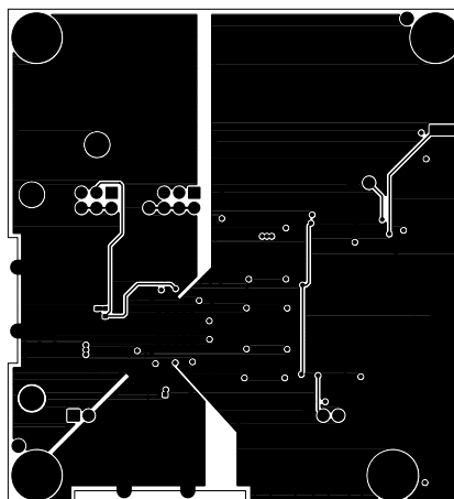
4層 ボトム側
