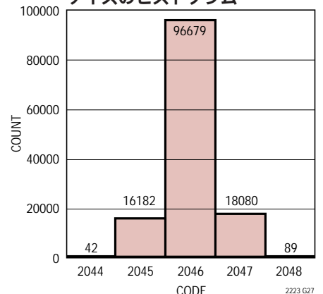
LTC2223 : ノイズのヒストグラム
