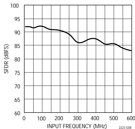
LTC2223 : SFDR (HD4+) と入力 周波数、 - 1dB、1Vレンジ
