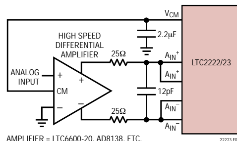
図4. アンプを使った差動ドライブ
