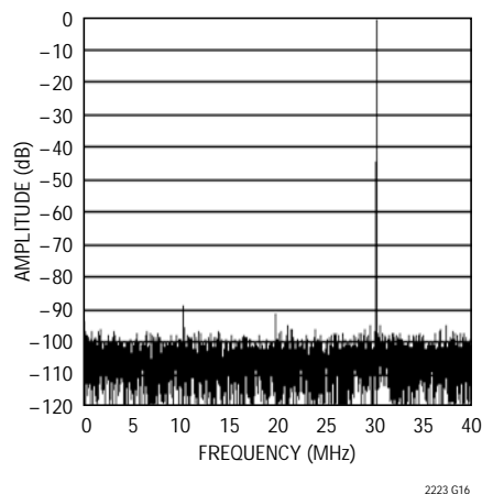
LTC2223 : 8192ポイントの FFT、 f_{IN} = 30\text{MHz} 、 -1\text{dB} 、 2Vレンジ
