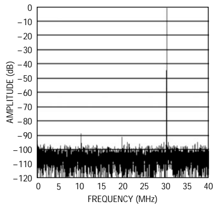
LTC2222 : 8192ポイントの FFT、 f_{IN} = 30\text{MHz} 、 -1\text{dB} 、 2Vレンジ
