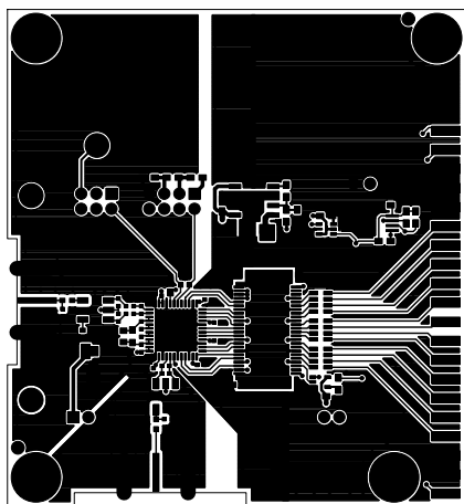
1層 部品側
