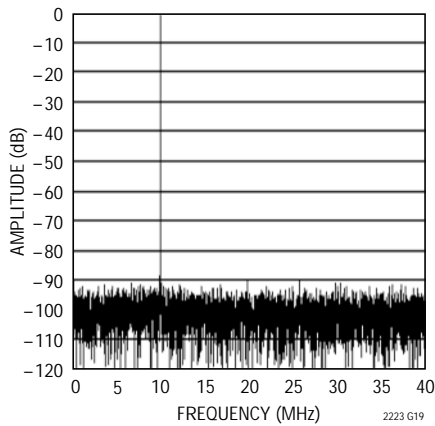
LTC2222 : 8192ポイントの FFT、 f_{IN} = 250\text{MHz} 、 -1\text{dB} 、 2Vレンジ
