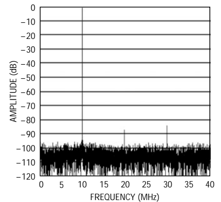
LTC2222 : 8192ポイントの FFT、 f_{IN} = 70\text{MHz} 、 -1\text{dB} 、 2Vレンジ
