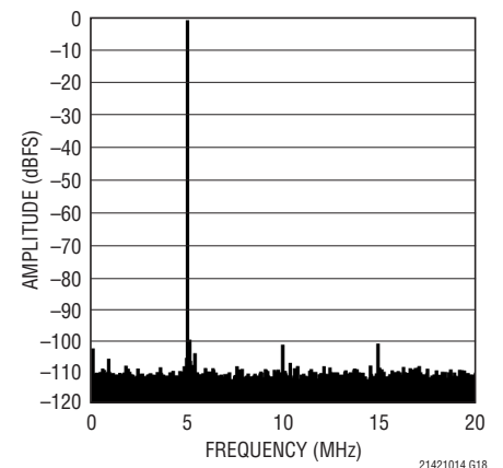
LTC2141-14: 64kポイントのFFT、 f_{IN} = 5\text{MHz} 、-1dBFS、40Mps
