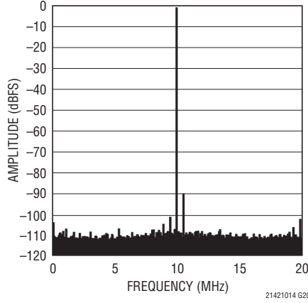
LTC2141-14: 64kポイントのFFT、 f_{IN} = 70\text{MHz} 、 -1\text{dBFS} 、 40\text{Mps}
