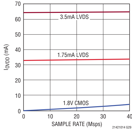
LTC2141-14: I_{OVD} とサンプル・レート、 各チャンネルに5MHz、-1dBFSの 正弦波入力
