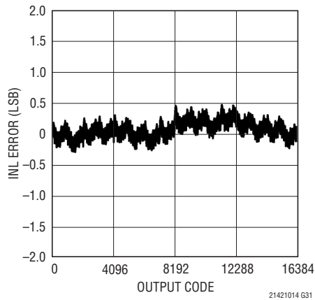
LTC2140-14: 積分非直線性 (INL)
