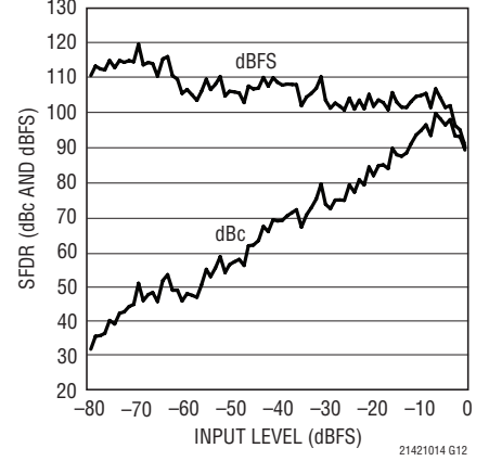
LTC2142-14: SFDRと入力レベル、 f_{IN} = 70\text{MHz} 、65Mps、2V範囲
