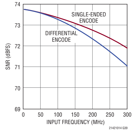
LTC2140-14: SNRと入力周波数、 -1dBFS、25Mpsps、2V範囲
