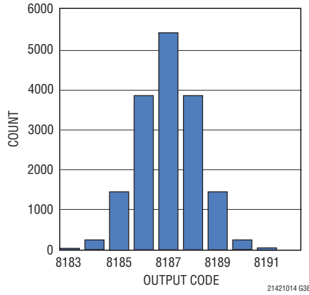
LTC2140-14: 短絡入力 のヒストグラム
