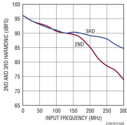
LTC2141-14: 2次および3次高調波と 入力周波数、 -1\text{dBFS} 、 40\text{Mps} 、 1\text{V} 範囲
