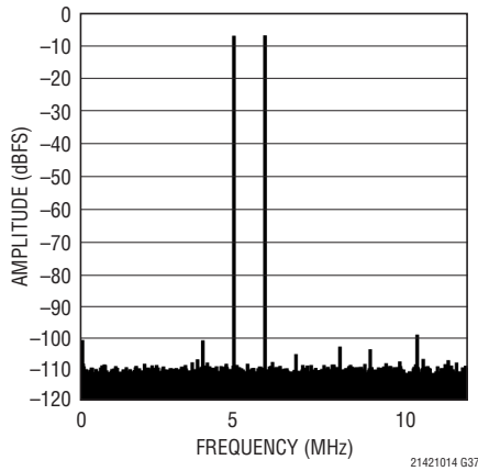
LTC2140-14: 64kポイントの 2トーンFFT、 f_{IN} = 69\text{MHz} 、 70\text{MHz} 、 -7dBFS、25Mpsps
