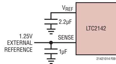
図9. 1.25Vの外部リファレンスを使用する場合
