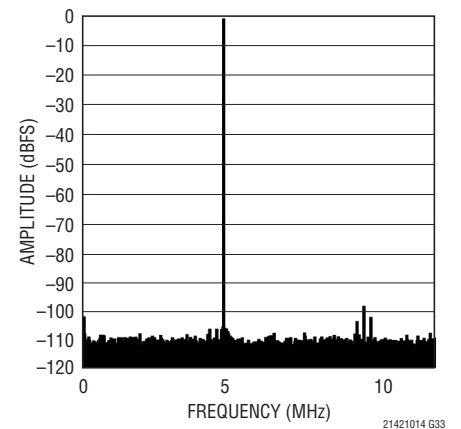
LTC2140-14: 64kポイントのFFT、 f_{IN} = 5\text{MHz} 、-1dBFS、25MSPS
