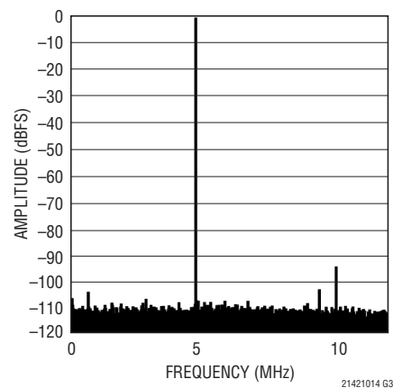
LTC2140-14: 64kポイントのFFT、 f_{IN} = 70\text{MHz} 、-1dBFS、25MSPS
