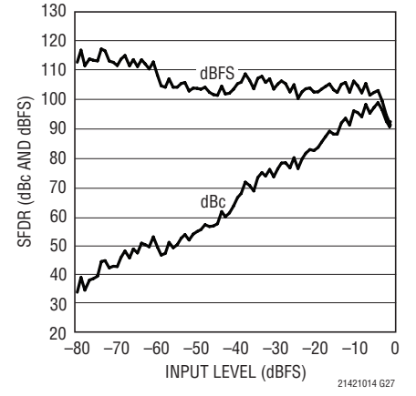
LTC2141-14: SFDRと入力レベル、 f_{IN} = 70\text{MHz} 、 40\text{Mps} 、 2\text{V} 範囲
