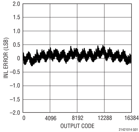
LTC2142-14: 積分非直線性 (INL)
