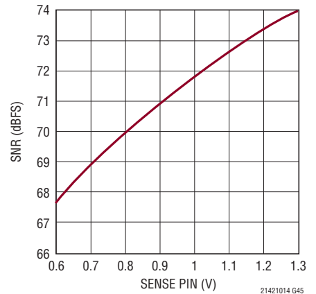
LTC2140-14: SNRとSENSE、 f_{IN} = 5\text{MHz} 、-1dBFS
