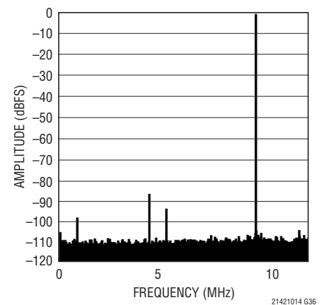
LTC2140-14: 64kポイントのFFT、 f_{IN} = 140\text{MHz} 、-1dBFS、25MSPS
