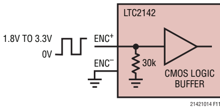
図11. シングルエンド・エンコード・モードでの等価エンコード入力回路
