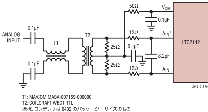
図4. 入力周波数が5MHz～150MHzの場合の推奨フロントエンド回路
