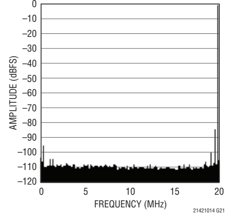
LTC2141-14: 64kポイントのFFT、 f_{IN} = 140\text{MHz} 、 -1\text{dBFS} 、 40\text{Mps}
