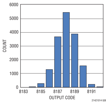
LTC2142-14: 短絡入力 のヒストグラム
