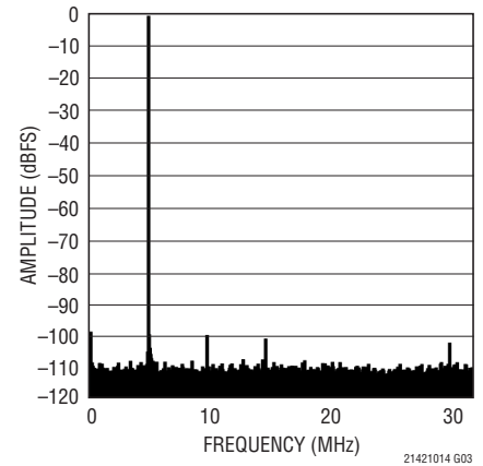
LTC2142-14: 64kポイントのFFT、 f_{IN} = 5\text{MHz} 、 -1\text{dBFS} 、 65\text{Mps}
