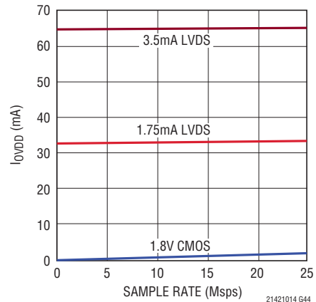
LTC2140-14: I_{OVD} とサンプル・レート、 各入力に5MHz、-1dBFSの正弦波
