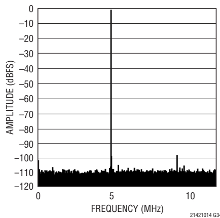
LTC2140-14: 64kポイントのFFT、 f_{IN} = 30\text{MHz} 、-1dBFS、25MSPS
