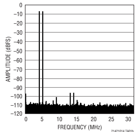
2 トーン FFT、 f_{IN} = 70\text{MHz} および 69\text{MHz}
