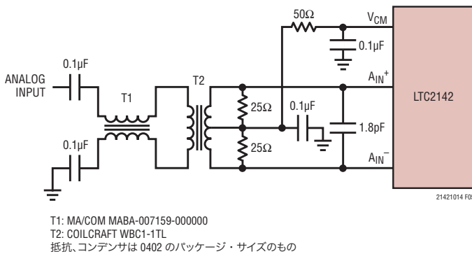
図5. 入力周波数が150MHz～250MHzの場合の推奨フロントエンド回路
