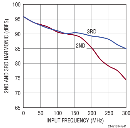
LTC2140-14: 2次および3次高調波と 入力周波数、-1dBFS、25Mpsps、1V範囲
