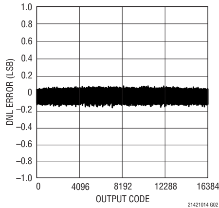
LTC2142-14: 微分非直線性 (DNL)
