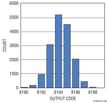
LTC2141-14: 短絡入力 のヒストグラム
