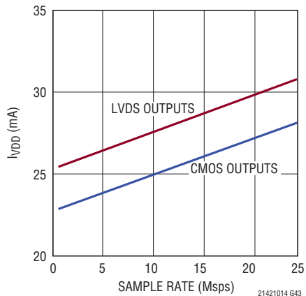
LTC2140-14: I_{VDD} とサンプル・レート、 各チャンネルに5MHz、-1dBFSの 正弦波入力
