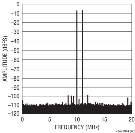
LTC2141-14: 64kポイントの 2トーンFFT、 f_{IN} = 69\text{MHz} 、 70\text{MHz} 、 -7\text{dBFS} 、 40\text{Mps}
