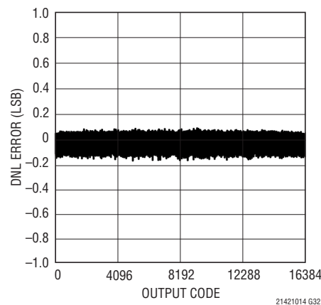
LTC2140-14: 微分非直線性 (DNL)
