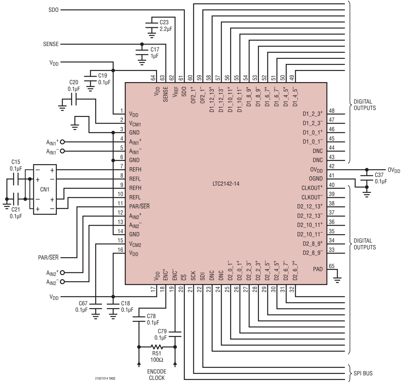
LTC2142 回路図
