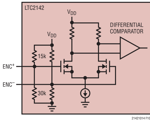
図10. 差動エンコード・モードでの等価エンコード入力回路
