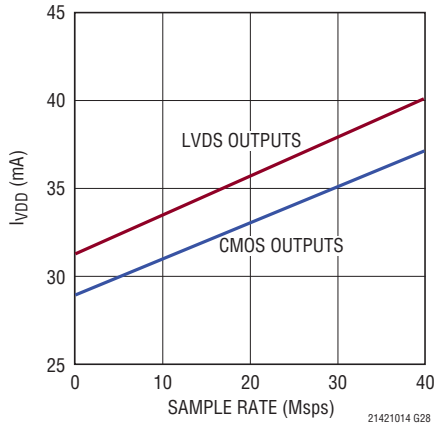
LTC2141-14: I_{VDD} とサンプル・レート、 各チャンネルに5MHz、-1dBFSの 正弦波入力
