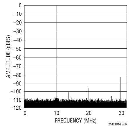
LTC2142-14: 64kポイントのFFT、 f_{IN} = 140\text{MHz} 、 -1\text{dBFS} 、 65\text{Mps}
