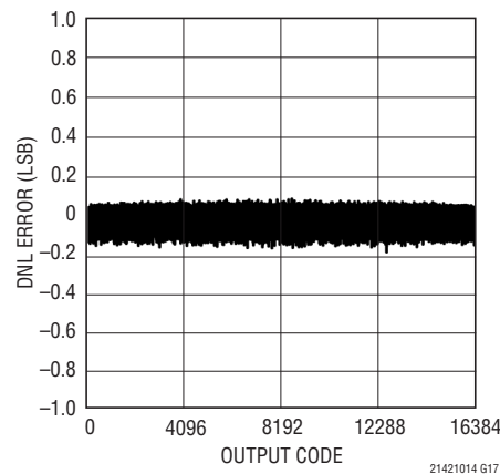
LTC2141-14: 微分非直線性 (DNL)
