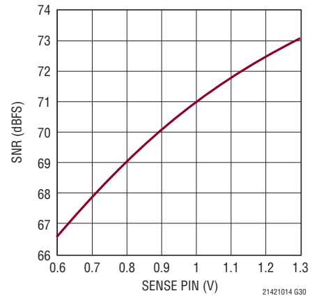
LTC2141-14: SNRと SENSE、 f_{IN} = 5\text{MHz} 、-1dBFS
