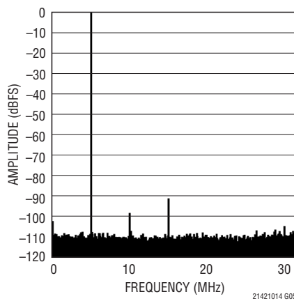
LTC2142-14: 64kポイントのFFT、 f_{IN} = 70\text{MHz} 、 -1\text{dBFS} 、 65\text{Mps}
