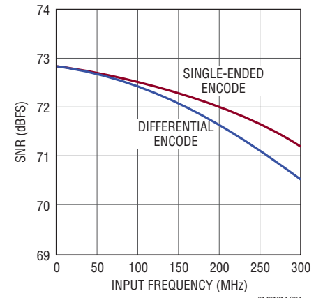
LTC2141-14: SNRと入力周波数、 -1\text{dBFS} 、 105\text{Mps} 、 2\text{V} 範囲
