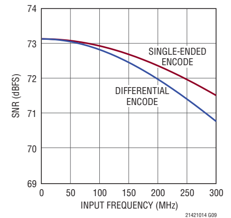
LTC2142-14: SNRと入力周波数、 -1\text{dBFS} 、 65\text{Mps} 、 2\text{V} 範囲
