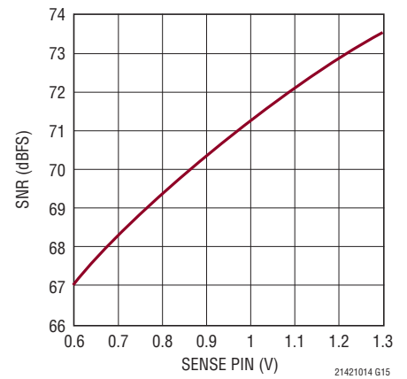
LTC2142-14: SNRとSENSE、 f_{IN} = 5\text{MHz} 、-1dBFS
