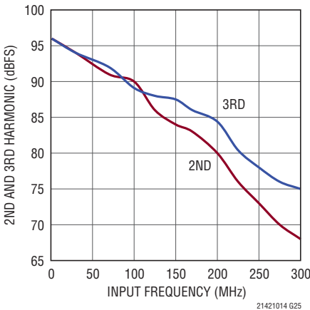
LTC2141-14: 2次および3次高調波と 入力周波数、 -1\text{dBFS} 、 40\text{Mps} 、 2\text{V} 範囲
