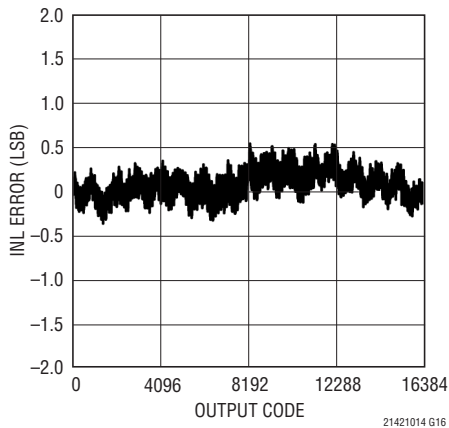
LTC2141-14: 積分非直線性 (INL)
