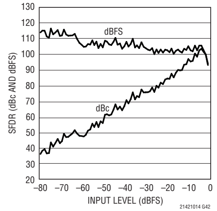
LTC2140-14: SFDRと入力レベル、 f_{IN} = 70\text{MHz} 、25Mpsps、2V範囲
