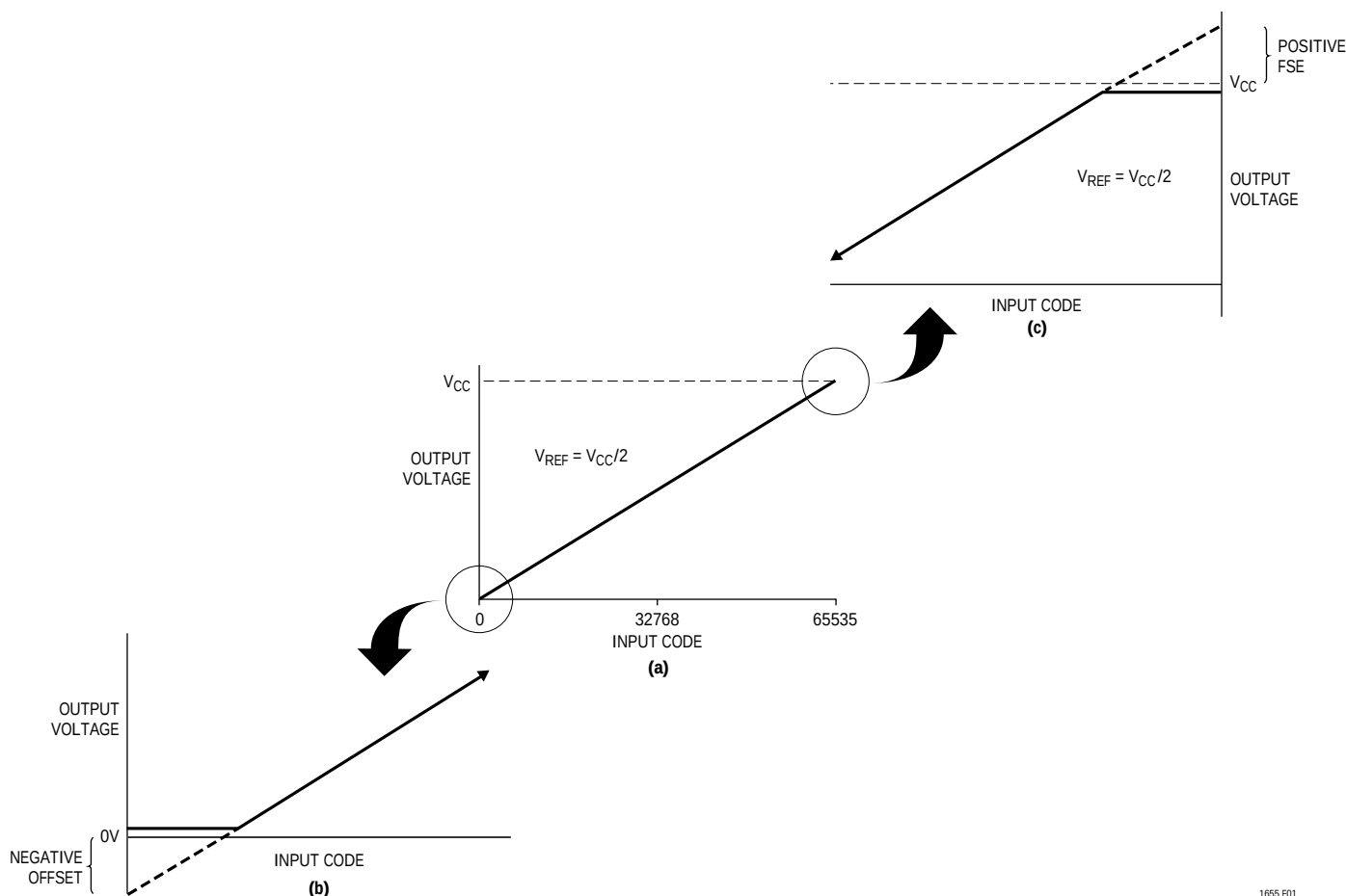
図1. レール・トゥ・レール動作のDAC伝達曲線での影響。(a) 全伝達関数 (b) ゼロ・スケール近くのコードに対する負オフセットの影響 (c) V_{REF} = V_{CC}/2 のときフルスケール近くの入力コードに対する正フルスケール誤差の影響
