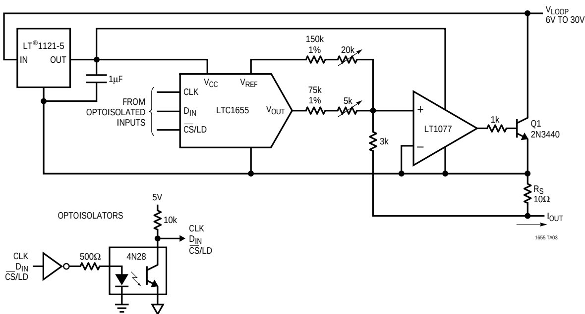
絶縁型4mA–20mAプロセス・コントローラ
