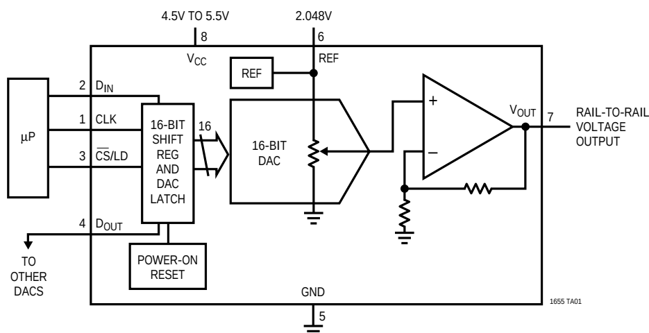
機能ブロック図: 16ビット・レール・トゥ・レールDAC
