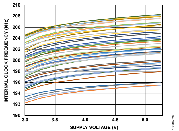
図 19. 内部クロック周波数と電源電圧の関係 (25°C)
