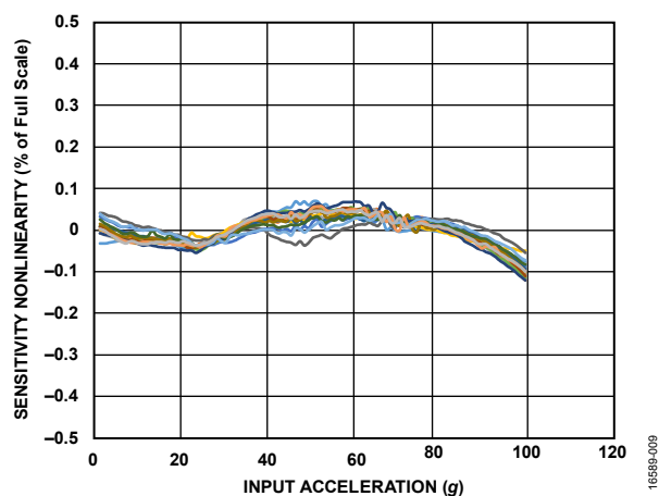
図 9. 感度の非直線性と入力加速度の関係
