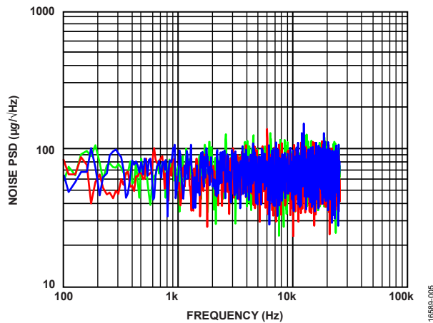
図 8. 100Hz を超えるノイズ PSD
