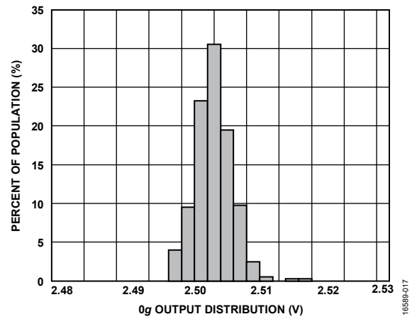
図 13. 0g オフセット・ヒストグラム (25°C)
