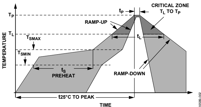
図 2. 推奨のハンダ付けプロファイル
