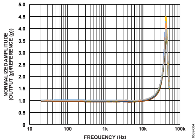
図 4. 周波数応答、高周波 (>5kHz) の振動応答、レーザー振動計コントローラは、正確に使用するために ADXL1005 パッケージを参照
