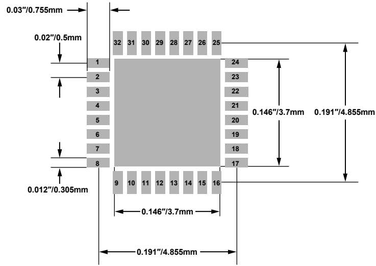
図 25. 推奨される PCB ランド・パターン
