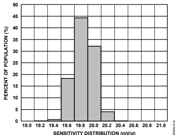
図 7. 感度分布 (25°C)
