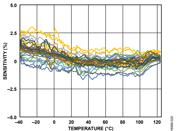
図 6. 感度の温度特性
