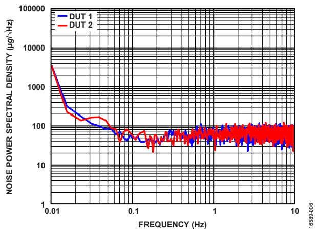
図 5. 10Hz 未満のノイズのパワー・スペクトラム密度 (PSD) の周波数特性
