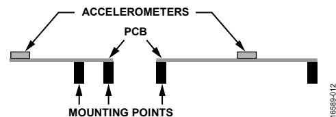
図 24. 加速度センサーの不適切な配置
