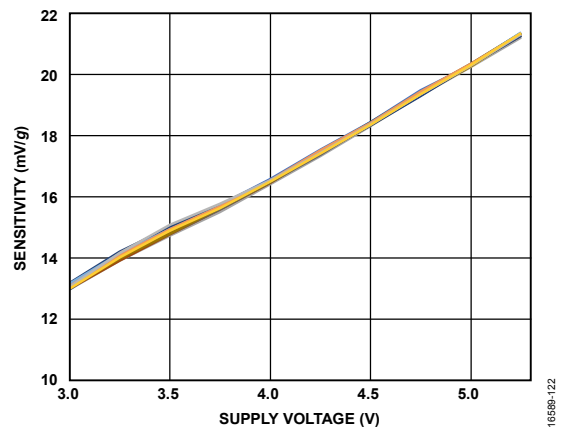
図 22. 感度と電源電圧の関係
