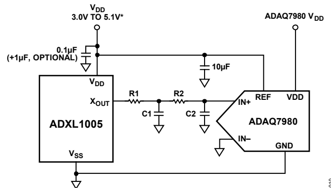
図 23. ADXL1005 のアプリケーション回路
