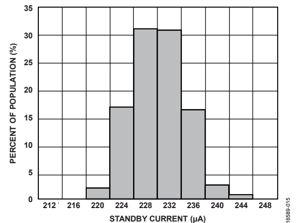
図 15. スタンバイ電流ヒストグラム (25°C)
