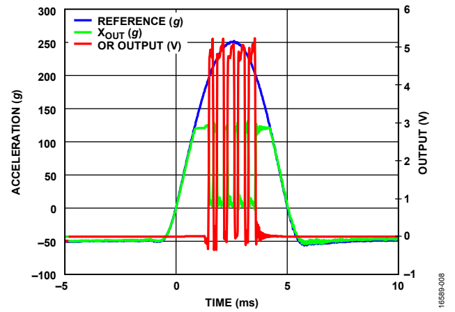
図 18. 負荷条件に対する応答、X OUT デルタは中間点電圧からの差
