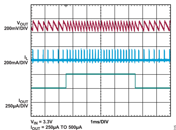
図 15. 250μA～500μA の過渡応答 (図 1 の代表的なアプリケーション回路を参照)
