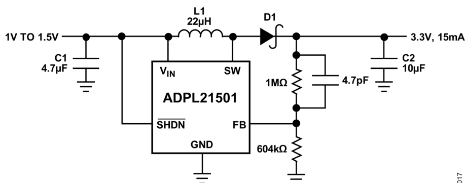
図 17. 1 セル・アルカリ電池入力、3.3V 出力の昇圧コンバータ
