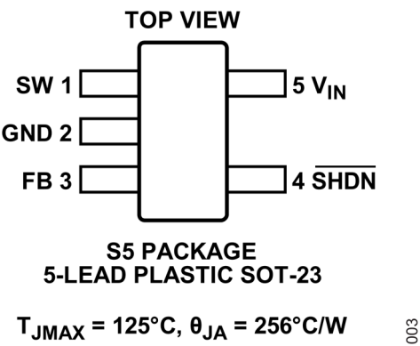
図 3. ピン配置
