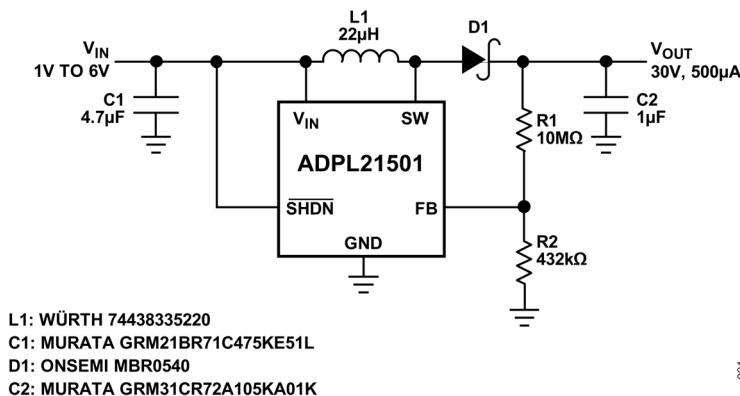
図 1. PIN ダイオード・ドライバ用コンバータ (30V)
