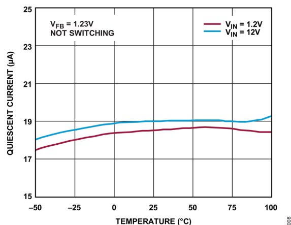
図 8. 静止電流
