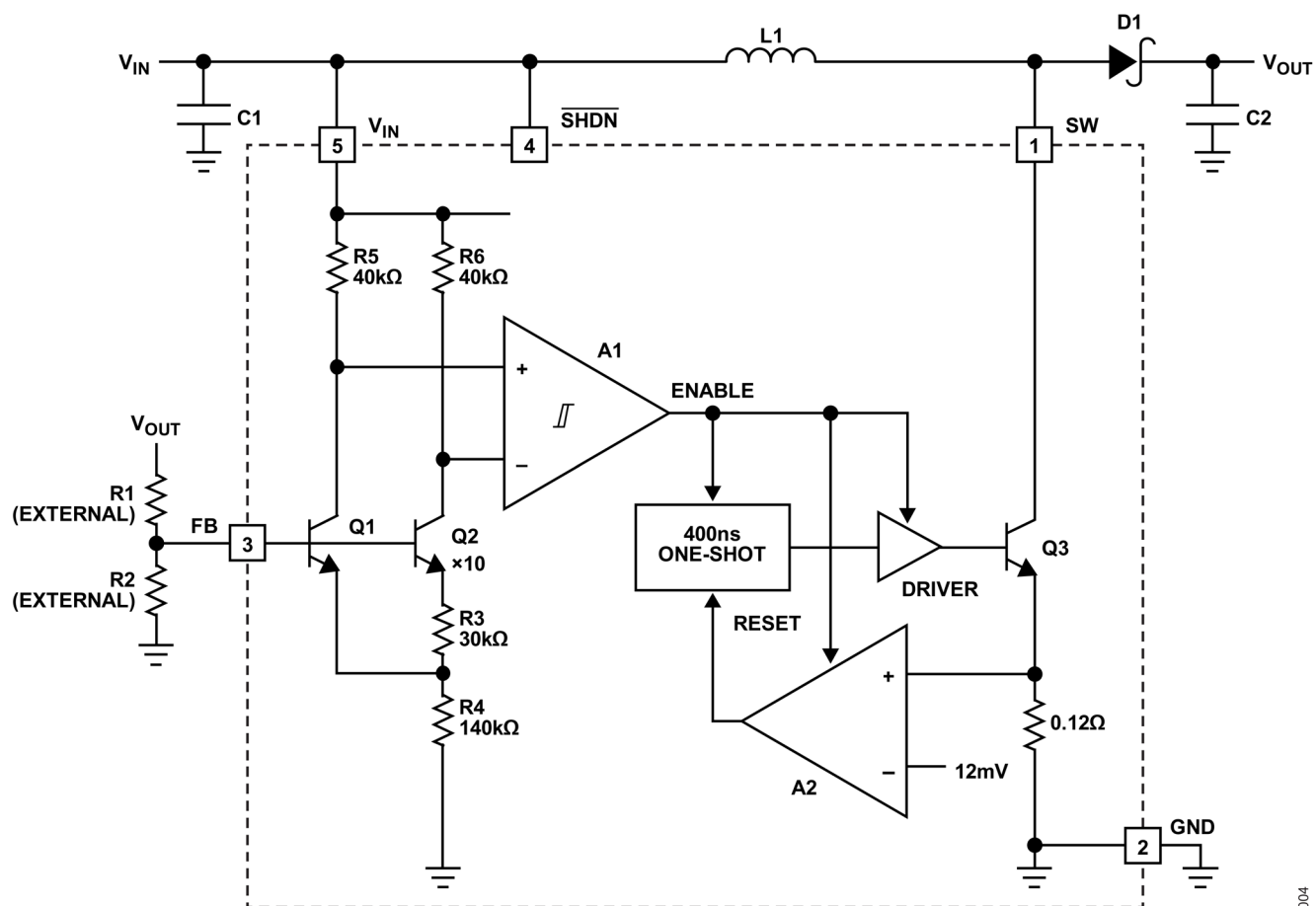
図 4. ADPL21501 のブロック図
