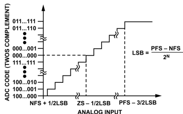
図 49. AD4854 の理想的なバイポーラ入力伝達関数、 N = 20 ビット
