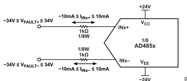
図 54. 外部直列抵抗（AD4854 の通常動作ではトランスペアレント）によるフォルト状態時のラッチアップ電流の制限
