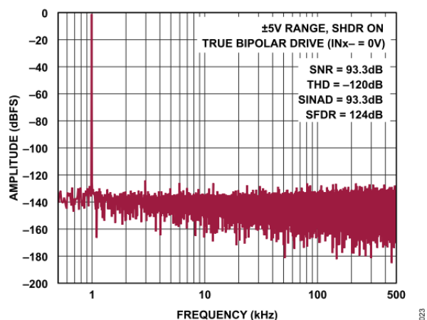
図 22. FFT (1MSPS、 f_{IN} = 1\text{kHz} 、 \pm 5\text{V} レンジ)
