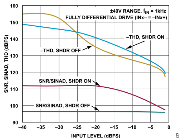
図 23. SNR、SINAD、THD と入力レベルの関係
