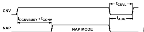
図 62. AD4854 のナップ・モードのタイミング
