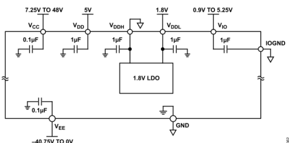
図 61. V_{DDL} が外部給電される場合の AD4854 の電源ピン
