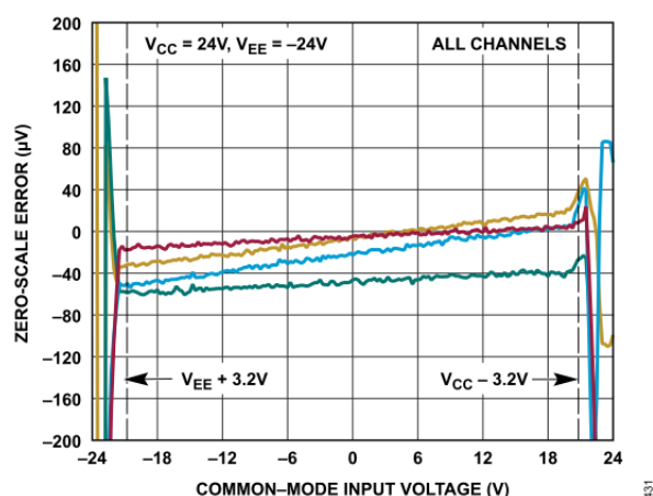
図 31. ゼロスケール誤差と同相入力電圧の関係
