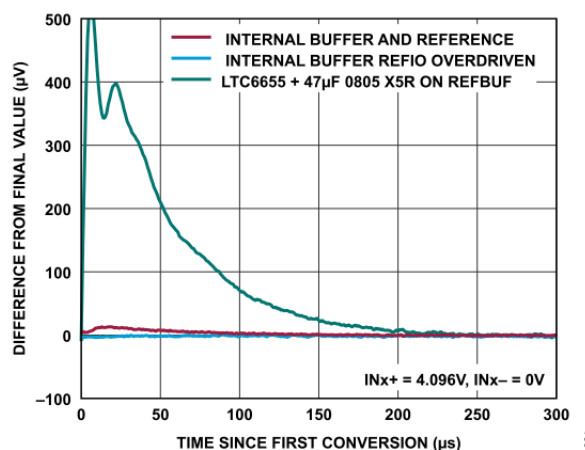
図 60. AD4854 のバースト変換応答 ( f_s = 1MSPS )
