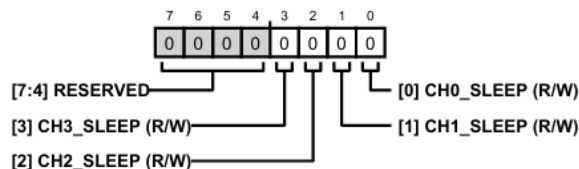
図 99. アドレス : 0x29、リセット : 0x00、レジスタ名 : CH_SLEEP
