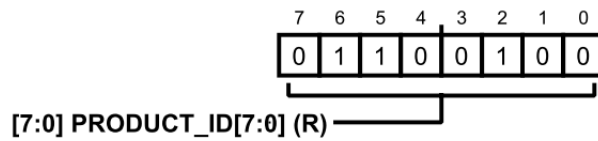
図 79. アドレス : 0x04、リセット : 0x64、レジスタ名 : PRODUCT_ID_L
