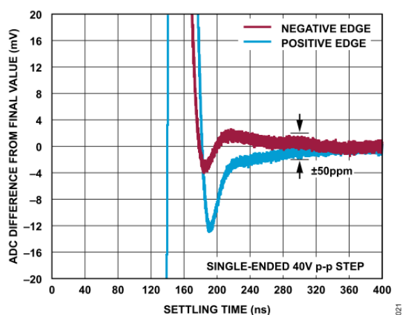
図 20. 入カステップ応答（微細セトリング）
