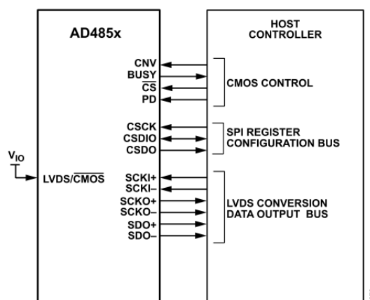
図 67. AD4854 の LVDS 変換データ出力モード
