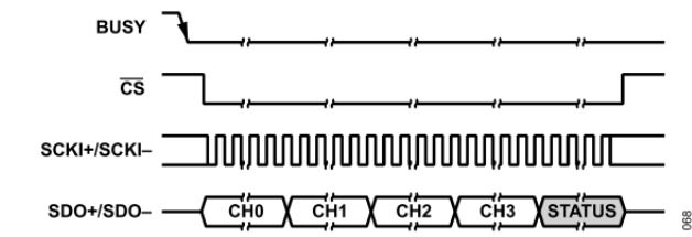
図 68. すべてのパケットが SDO+および SDO-にシーケンシャルに出力
