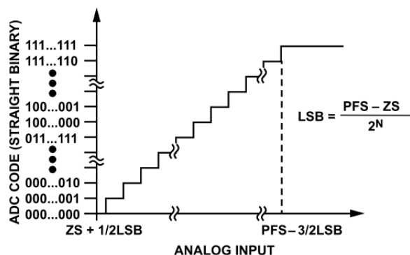
図 50. AD4854 の理想的なユニポーラ入力伝達関数、 N = 20 ビット
