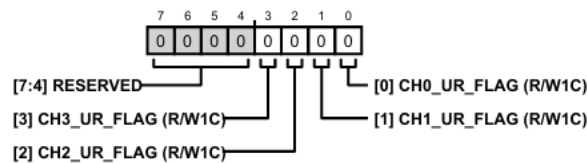
図 93. アドレス : 0x22、リセット : 0x00、レジスタ名 : CH_UR_STATUS
