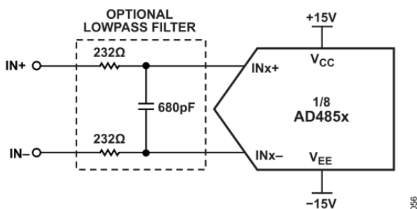
図 55. AD4854 の差動入力フィルタの例
