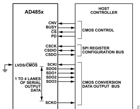
図 65. AD4854 の CMOS 変換データ出力モード
