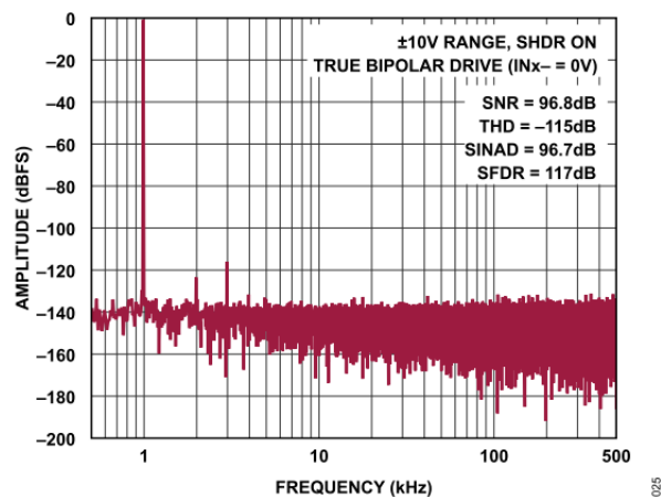
図 24. FFT (1MSPS、 f_{IN} = 1\text{kHz} 、 \pm 10\text{V} レンジ)
