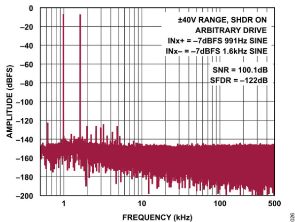
図 25. FFT (1MSPS、 f_{INx+} = 991\text{Hz} 、 f_{INx-} = 1.6\text{kHz} 、 \pm 40\text{V} レンジ)
