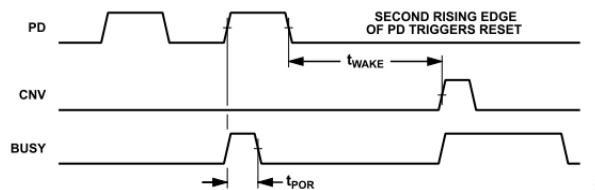
図 63. AD4854 のリセット・タイミング
