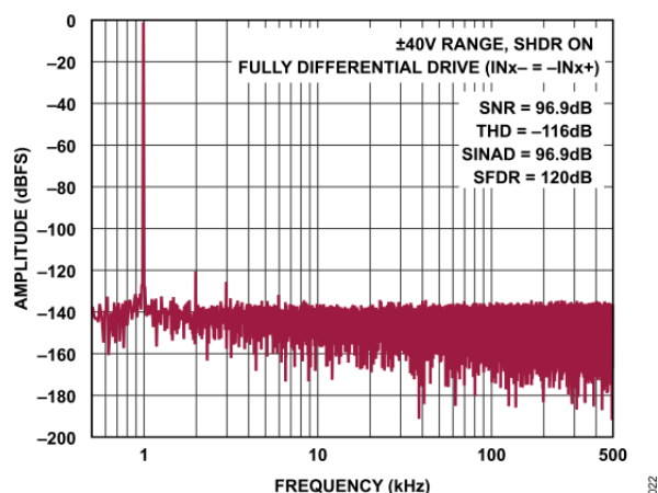
図 21. FFT (1MSPS、 f_{IN} = 1\text{kHz} 、 \pm 40\text{V} レンジ)
