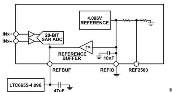
図 58. 外部リファレンスを使用し内部バッファを無効化する構成
