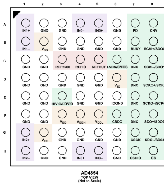
図 8. ピン配置
