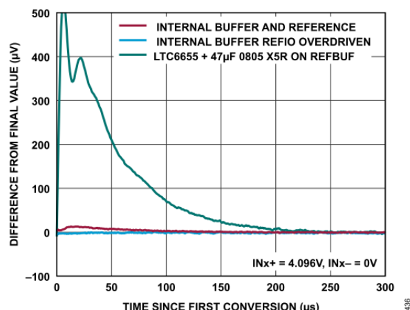
図 36. バースト変換応答 ( f_s = 1\text{MSPS} )
