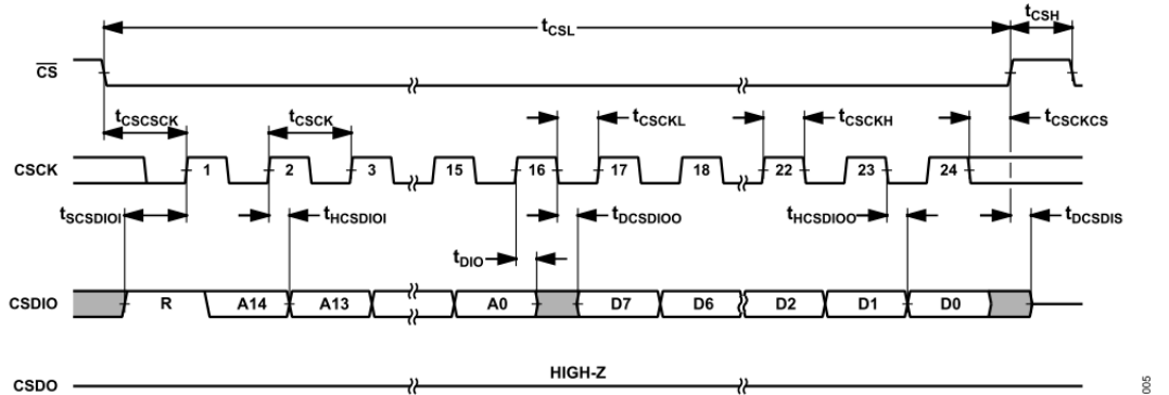
図 4. SPI レジスタ設定バスの 3 線式読出しタイミング
