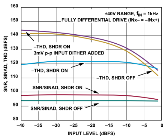
図 23. SNR、SINAD、THD と入力レベルの関係
