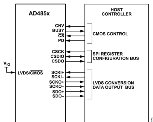
図 67. AD4853 の LVDS 変換データ出力モード
