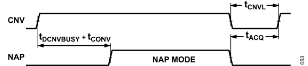
図 62. AD4853 のナップ・モードのタイミング
