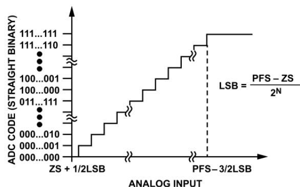
図 50. AD4853 の理想的なユニポーラ入力伝達関数、 N = 16 ビット
