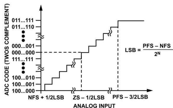
図 49. AD4853 の理想的なバイポーラ入力伝達関数、 N = 16 ビット
