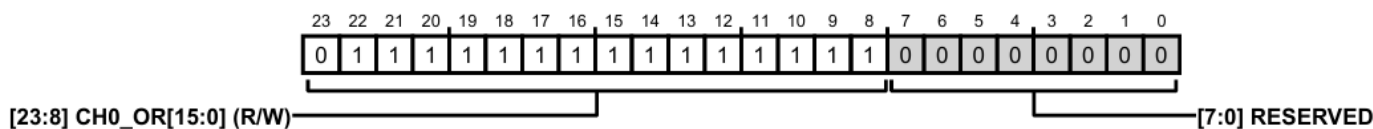
図 104. アドレス : 0x32~0x34、リセット : 0x7FFF00、レジスタ名 : CH0_OR
