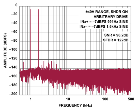
図 25. FFT (1MSPS、 f_{INx+} = 991\text{Hz} 、 f_{INx-} = 1.6\text{kHz} 、 \pm 40\text{V} レンジ)
