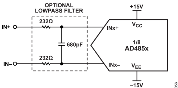
図 55. AD4853 の差動入力フィルタの例
