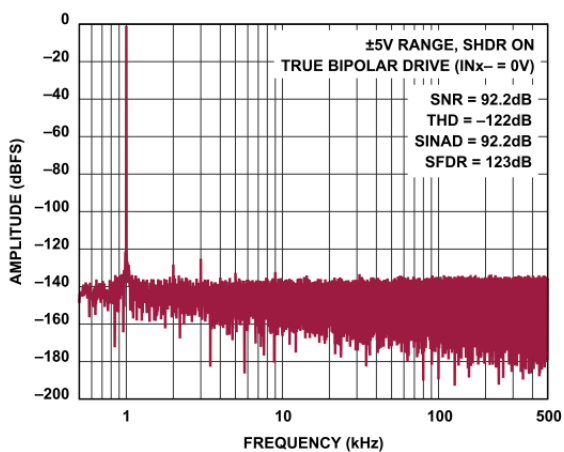
図 22. FFT (1MSPS、 f_{IN} = 1\text{kHz} 、 \pm 5\text{V} レンジ)
