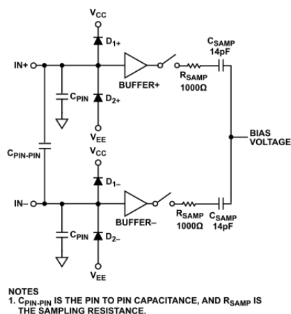
図 53. 差動アナログ入力の等価回路 (シングル・チャンネル)
