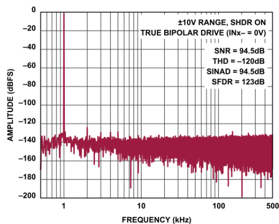
図 24. FFT (1MSPS、 f_{IN} = 1\text{kHz} 、 \pm 10\text{V} レンジ)
