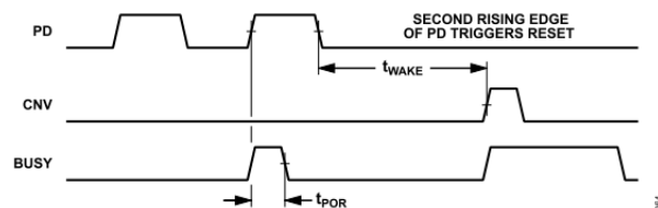
図 63. AD4853 のリセット・タイミング
