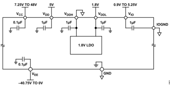
図 61. V_{DDL} が外部給電される場合の AD4853 の電源ピン
