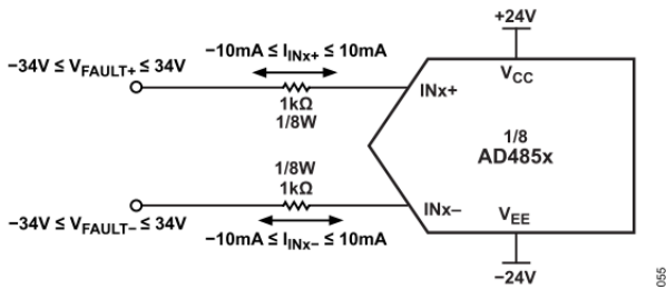
図 54. 外部直列抵抗（AD4853 の通常動作ではトランスペアレント）によるフォルト状態時のラッチアップ電流の制限
