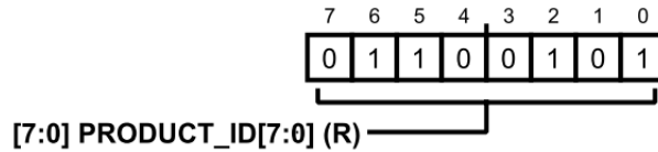
図 79. アドレス : 0x04、リセット : 0x65、レジスタ名 : PRODUCT_ID_L
