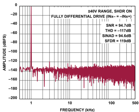
図 21. FFT (1MSPS、 f_{IN} = 1\text{kHz} 、 \pm 40\text{V} レンジ)
