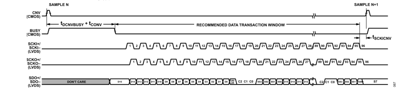
図 69. LVDS シリアル変換データ・バスのタイミング (PACKET_SIZE = 0x1、OS_EN = 0、TEST_PAT = 0)
