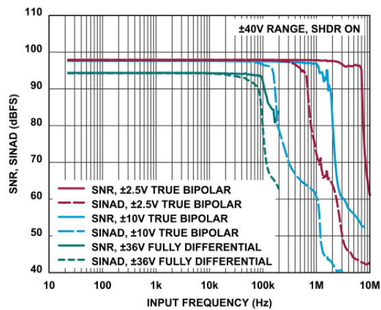
図 26. SNR および SINAD と入力周波数の関係
