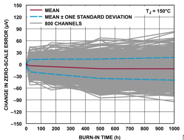
図 38. ゼロスケール誤差の変化とバーンイン時間の関係
