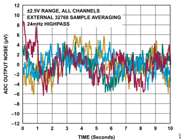
図 37. 10 秒間の低周波ノイズ
