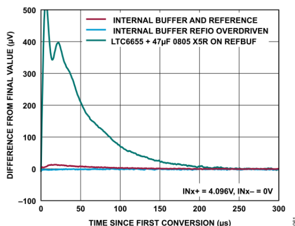
図 60. AD4853 のバースト変換応答 ( f_s = 1MSPS )
