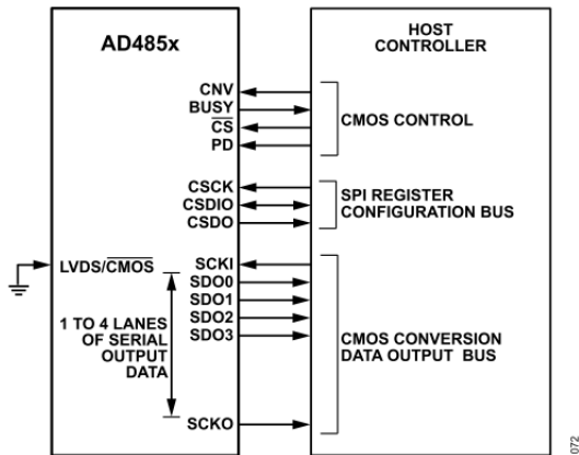
図 65. AD4853 の CMOS 変換データ出力モード
