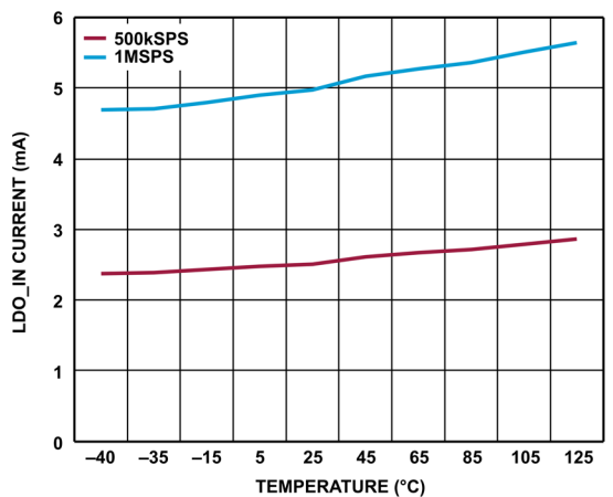
図 35. LDO_IN 電流と温度の関係
