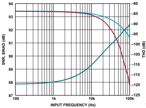
図 12. SNR、SINAD、THD と入力周波数の関係
