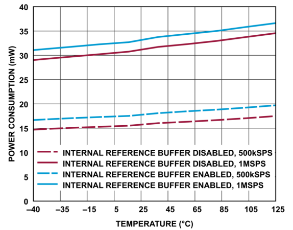
図 46. 消費電力と温度の関係 (内部 LDO をイネーブル)
