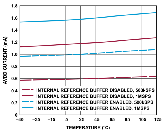
図 32. AVDD 電流と温度の関係
