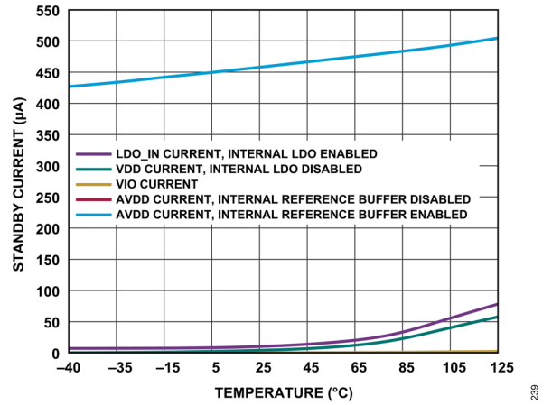
図 39. スタンバイ電流と温度の関係
