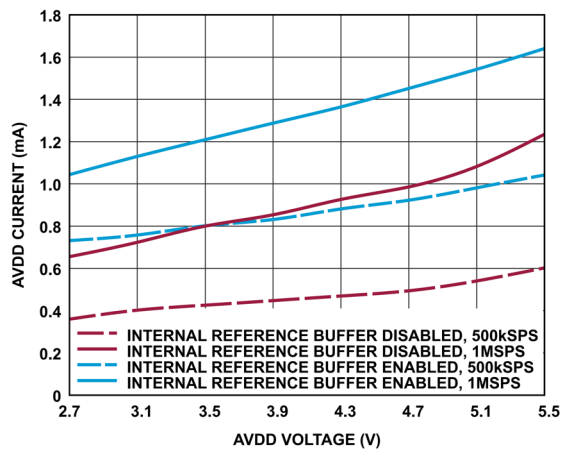
図 31. AVDD 電流と AVDD 電圧の関係
