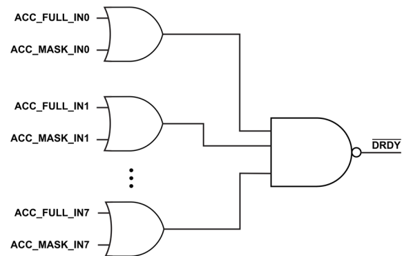
図 61. \overline{\text{DRDY}} マスクのロジック図 (簡略図)
