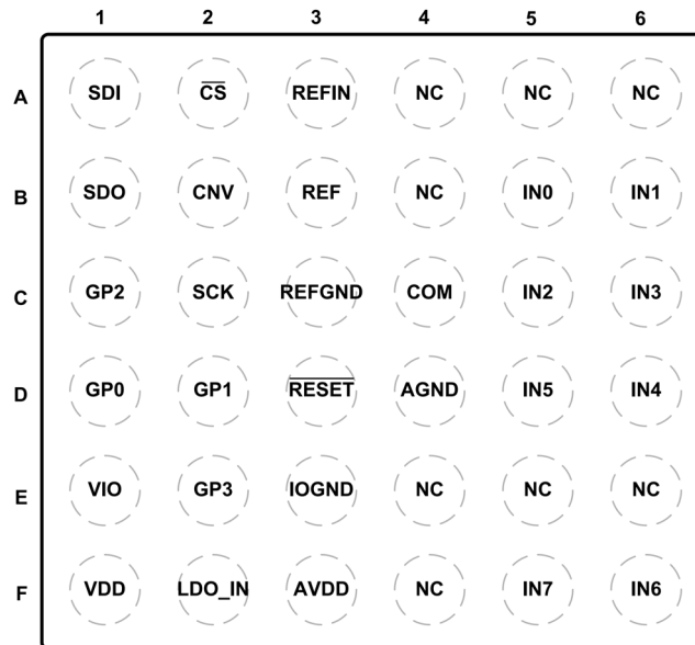
図 5. AD4693/AD4694 WLCSP のピン配置
