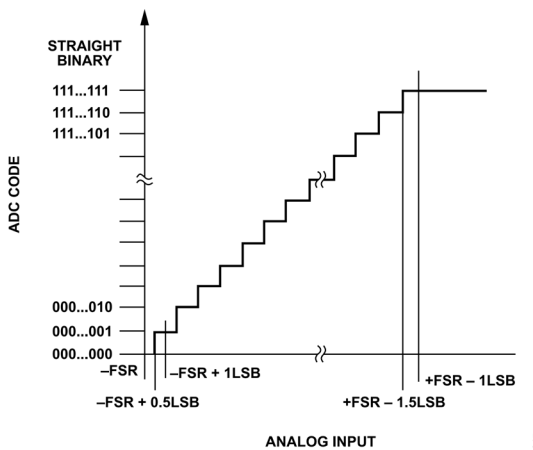
図 48. ADC の理想的な伝達関数 (FSR はフル・スケール範囲)
