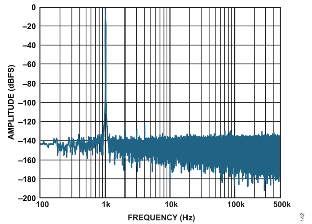
図 22. 高速フーリエ変換 (FFT)、 f_{IN} = 1\text{kHz} 、 V_{REF} = 5\text{V}
