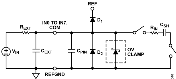
図 49. 等価アナログ入力回路
