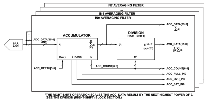
図 60. 平均化フィルタの簡略図
