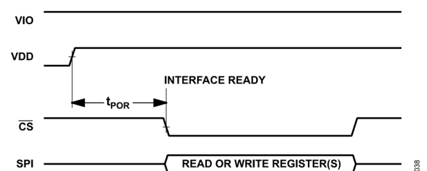
図 79. VDD POR のタイミング図
