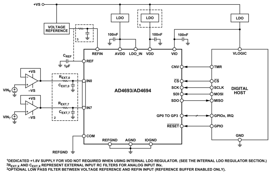
図 84. AD4693/AD4694 の代表的な接続図
