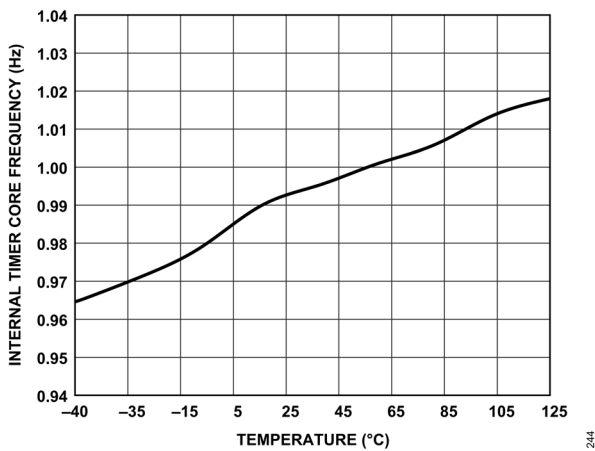
図 44. 内蔵タイマーのコア周波数と温度の関係
