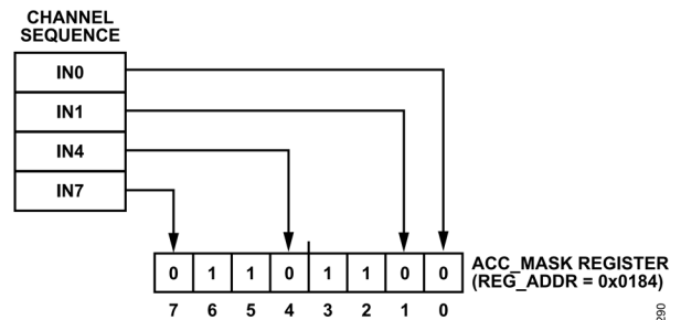
図 90. マスク・ビットの設定とチャンネル・シーケンスの関係を示す例
