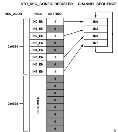
図 56. 標準シーケンサの簡略図
