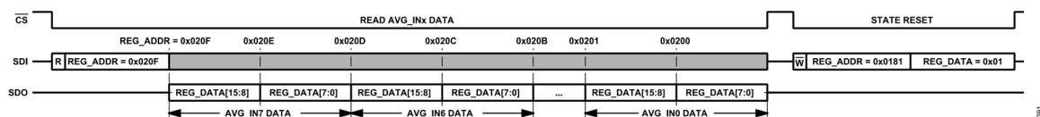
図 91. 自動デクリメント・モードでの隣接チャンネル・データの読出し
