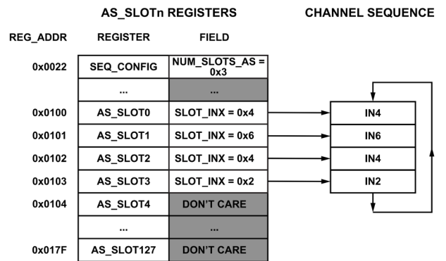
図 58. 詳細シーケンサの簡略図
