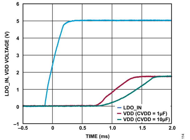
図 40. LDO_IN および VDD の電圧と時間の関係
