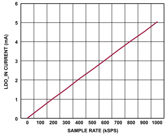
図 33. LDO_IN 電流とサンプル・レートの関係
