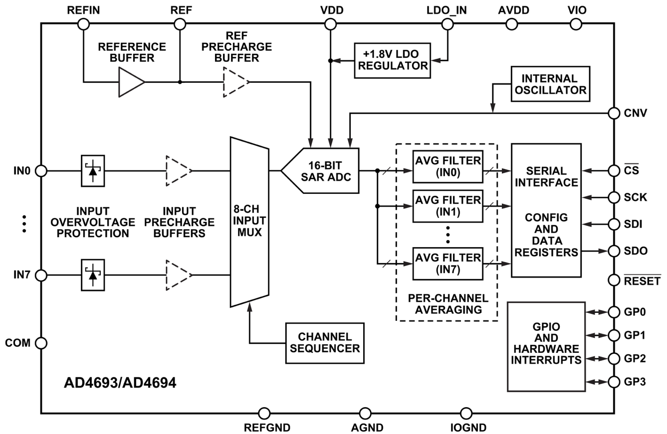
図 1. AD4693/AD4694 の機能ブロック図
