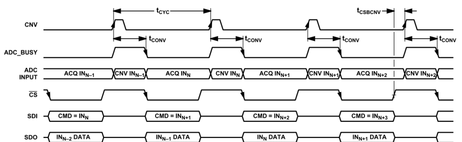
図 71. 手動モードのタイミング図
