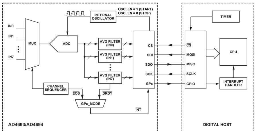
図 68. 自律モードの例示的接続図
