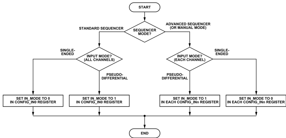
図 98. アナログ入力設定用のデバイス設定フローチャート
