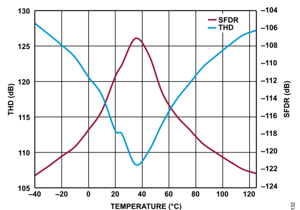
図 17. THD、SFDR の温度特性
