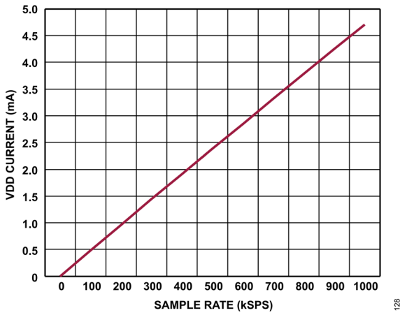
図 36. VDD 電流とサンプル・レートの関係
