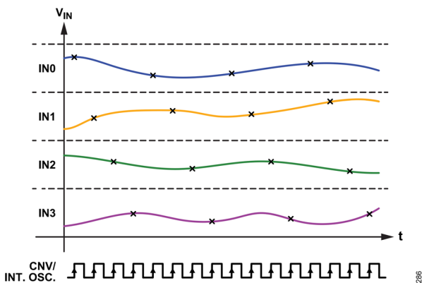
図 86. AD4693/AD4694 のインターリーブ・シーケンス (平均化比率 4)
