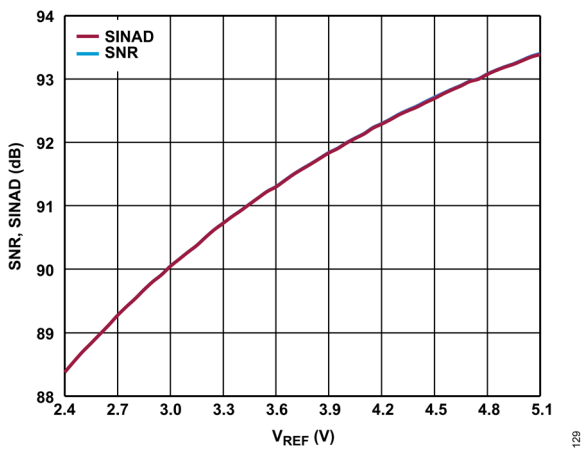
図 13. S/N 比および SINAD と V REF の関係
