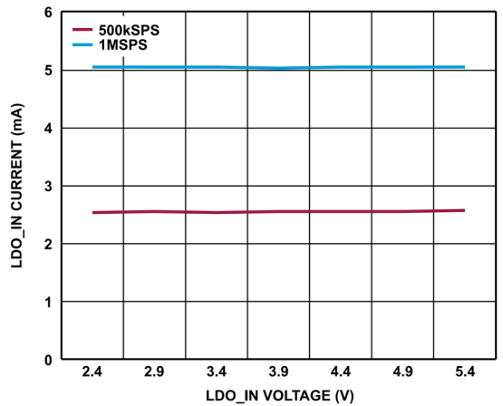
図 34. LDO_IN 電流と LDO_IN 電圧の関係
