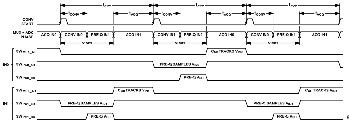
図 52. プリチャージのタイミング図の例
