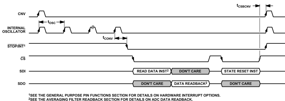
図 65. CNV バースト・モードのタイミング図
