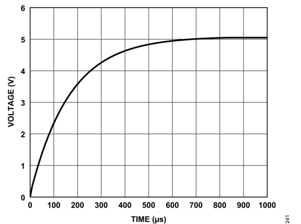
図 41. V_{REF} と時間の関係 (内部リファレンス・バッファをイネーブル)、 C_{REF} = 1\mu F
