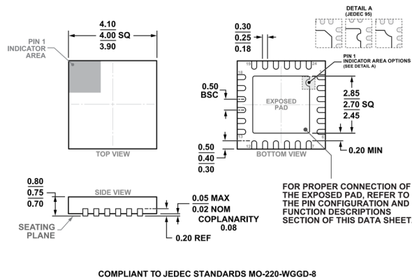
図 102. 24 ピン、リード・フレーム・チップ・スケール・パッケージ [LFCSP] 4mm × 4mm ボディ、0.75mm パッケージ高 (CP-24-8) 寸法：mm
