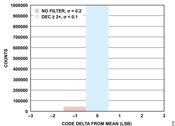
図 18. コードのヒストグラム、sinc5 + 補償、フィルタなし、デシメーション率 ≥ 2x
