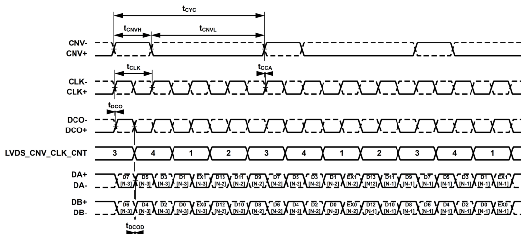
図 107. 拡張分解能パターンの例、デュアル・レーン LVDS、エコー・クロック・モード
