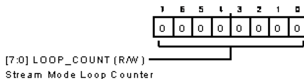
図 121. ストリーム・モード・レジスタ
