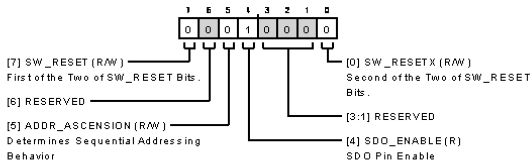
図 110. インターフェース設定 A の設定値
