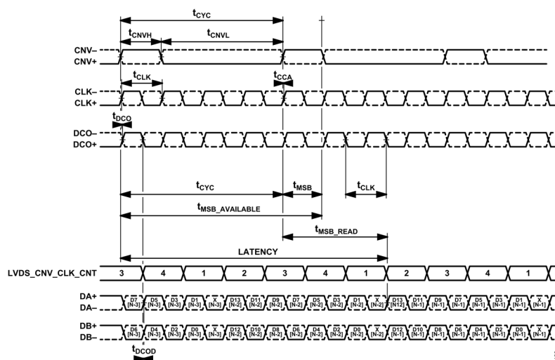
図 79. デュアル・レーン LVDS、エコー・クロック・モードでの LVDS_CNV_CLK_CNT 位置の例
