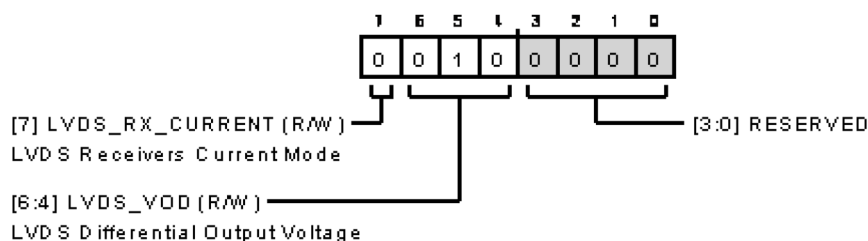
図 128. ADC データ・インターフェース設定 C レジスタ
