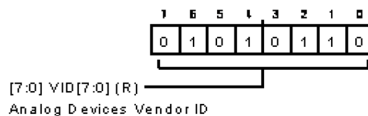
図 119. ベンダ ID ロー・レジスタ
