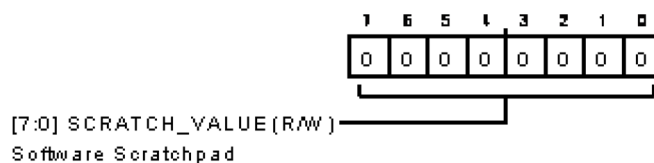
図 117. スクラッチ・パッド・レジスタ
