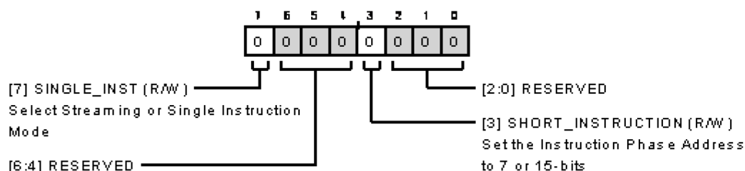
図 111. インターフェース設定 B の追加の設定値
