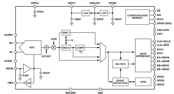
図 1. AD4088 の機能ブロック図
