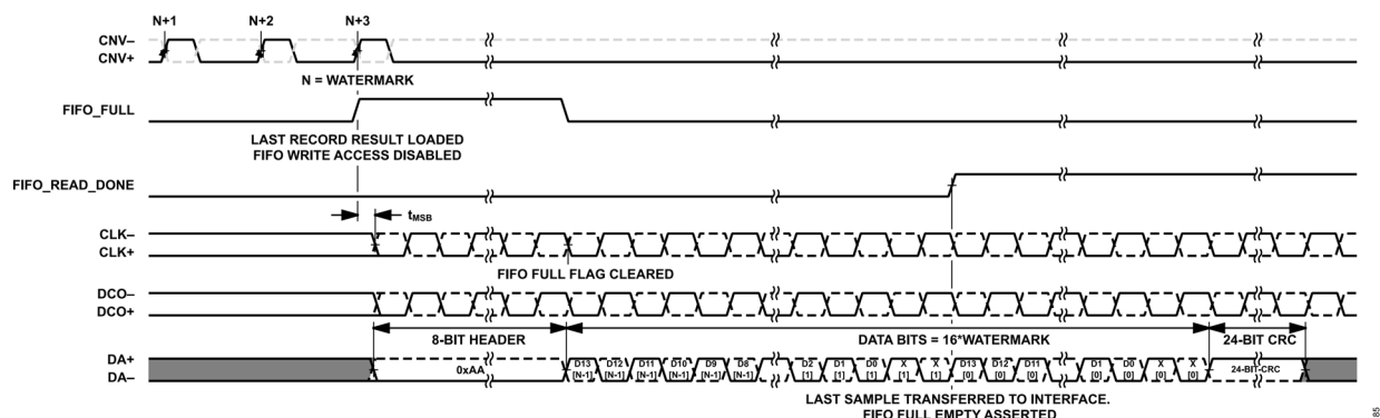
図 88. 非同期読み出しタイミング、データ FIFO イネーブル、LVDS 設定
