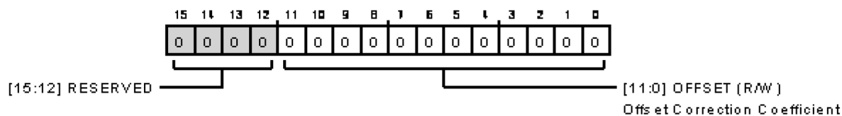
図 138. オフセット補正レジスタ
