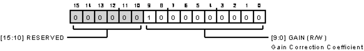
図 139. ゲイン補正レジスタ
