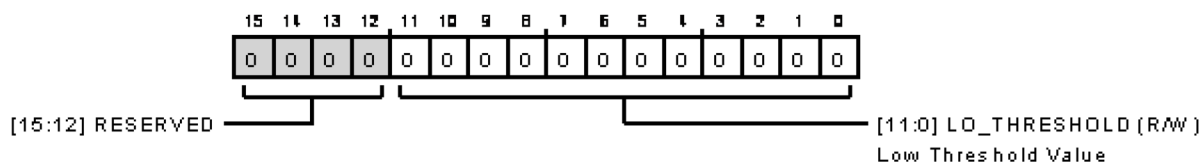
図 137. イベント検出の低閾値設定レジスタ
