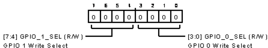
図 131. GPIO 設定 B レジスタ
