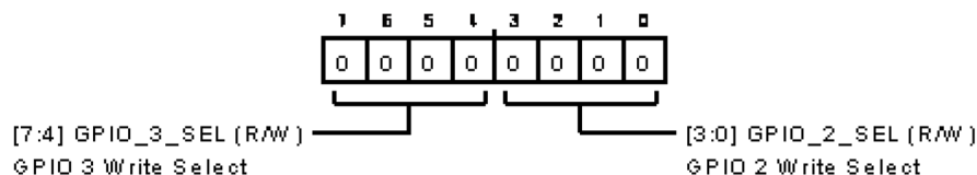
図 132. GPIO 設定 C レジスタ
