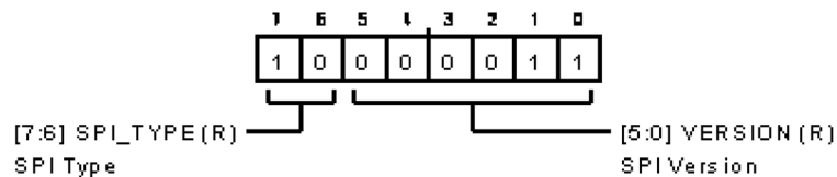
図 118. SPI リビジョン・レジスタ
