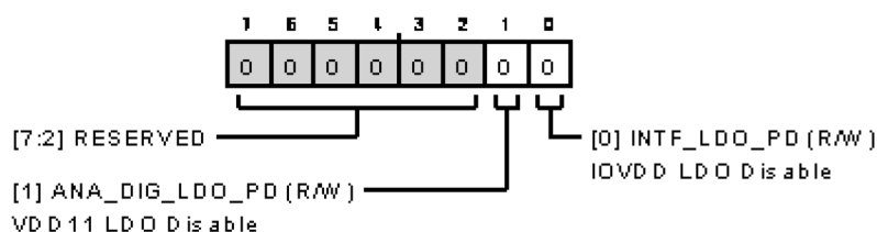
図 129. パワー・コントロール・レジスタ
