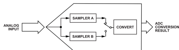
図 30. AD4088 SAR ADC の簡略表示
