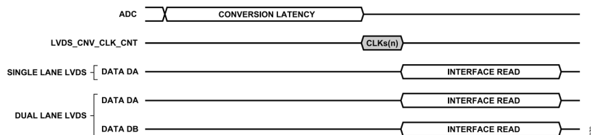
図 80. LVDS データ転送レイテンシ
