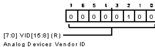
図 120. ベンダ ID ハイ・レジスタ
