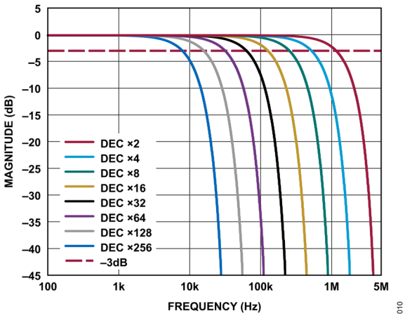
図 10. sinc5 フィルタ応答、 f_s = 10\text{MHz}
