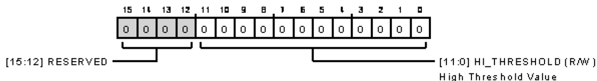
図 136. イベント検出の高閾値設定レジスタ
