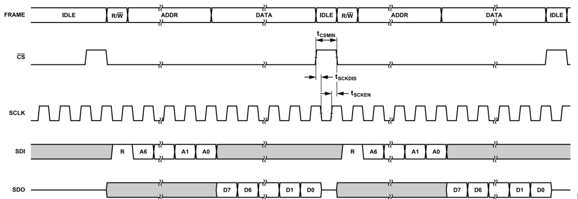
図 72. 設定 SPI タイミング、データ読出しフレーム、連続 SCLK
