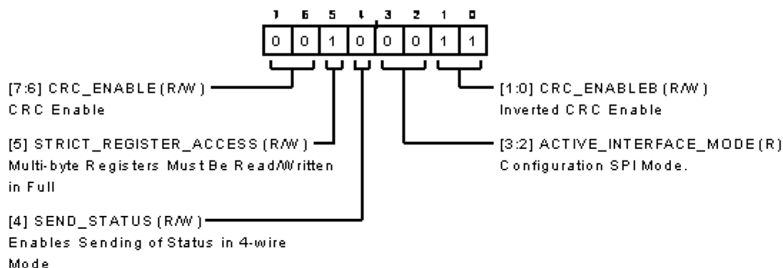
図 123. インターフェース設定 C レジスタ
