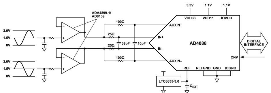
図 45. AD4088 の代表的なアプリケーション図、シングル・オペアンプ・ドライバ
