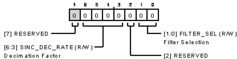
図 140. フィルタ設定レジスタ
