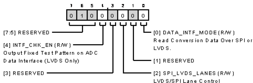
図 126. ADC データ・インターフェース設定 A レジスタ
