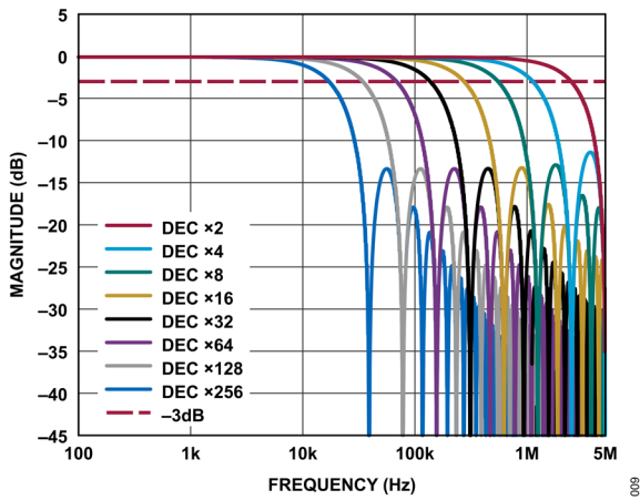
図 9. sinc1 フィルタ応答、 f_s = 10\text{MHz} (DEC \times はデシメーション率)
