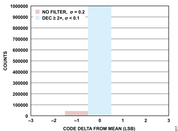
図 17. コードのヒストグラム、sinc5、フィルタなし、デシメーション率 ≥ 2x
