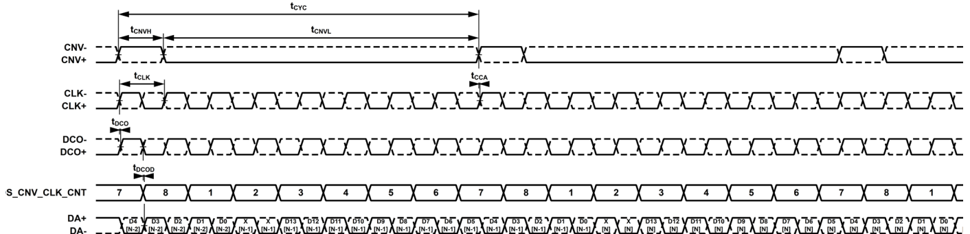
図 106. 拡張分解能パターンの例、シングル・レーン LVDS、エコー・クロック・モード
