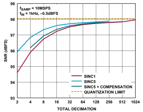
図 12. S/N 比と合計デシメーション係数の関係、 すべてのフィルタ・タイプ
