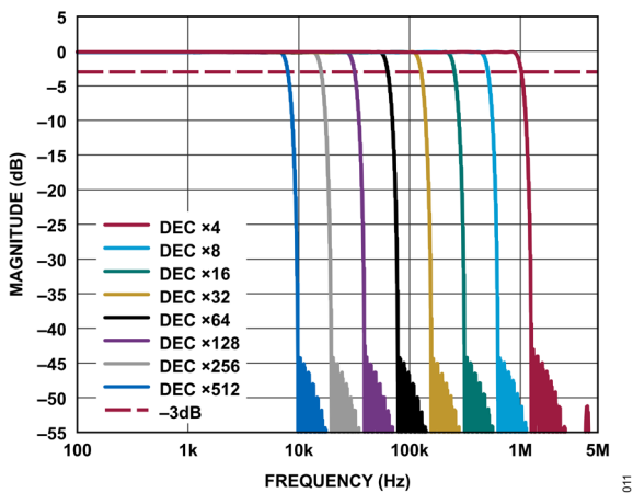
図 11. sinc5 + 補償フィルタ応答、 f_s = 10\text{MHz}
