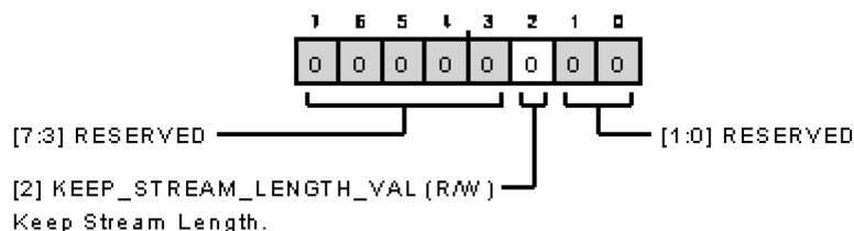
図 122. 転送設定レジスタ
