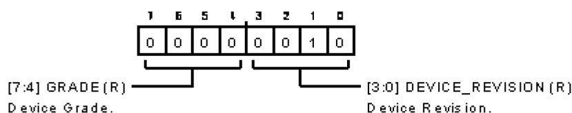
図 116. チップ・グレード・レジスタ
