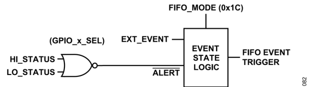
図 84. FIFO イベント検出ロジック
