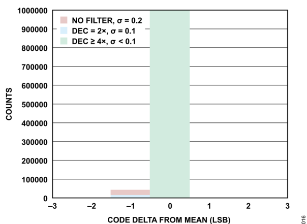
図 16. コードのヒストグラム、sinc1、フィルタなし、デシメーション率 ≥ 2x、デシメーション率 ≥ 4x
