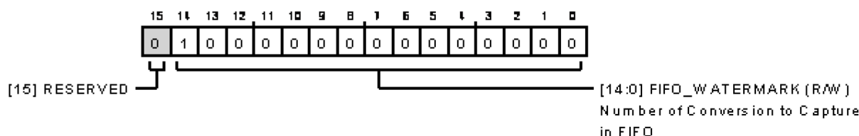
図 134. FIFO ウォーターマーク・レジスタ
