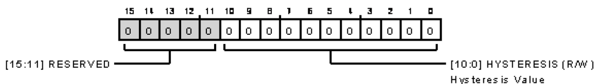
図 135. イベント検出ヒステリシス設定レジスタ
