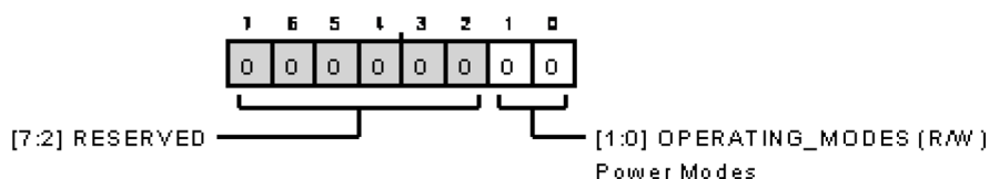
図 112. デバイス設定レジスタ
