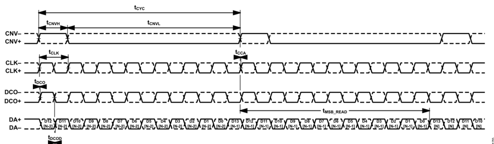
図 73. 連続変換タイミング、LVDS データ・インターフェース、シングル・データ・レーン、エコ・クロック・モード
