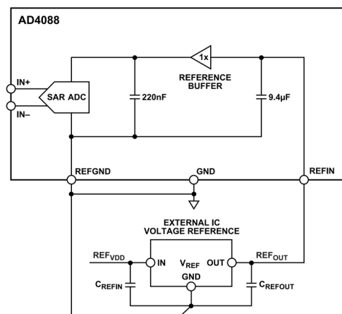
図 46. AD4088 一般的な外部リファレンス設計の機能図
