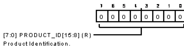
図 115. 製品 ID ハイ・レジスタ
