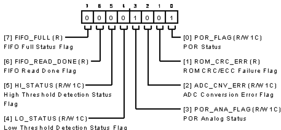
図 125. デバイス・ステータス・レジスタ
