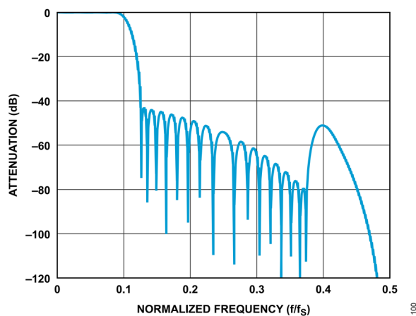
図 103. sinc5 + 補償フィルタの応答、デシメーション率 2
