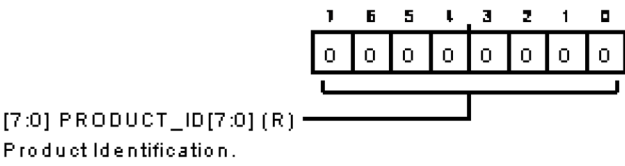
図 114. 製品 ID ロー・レジスタ
