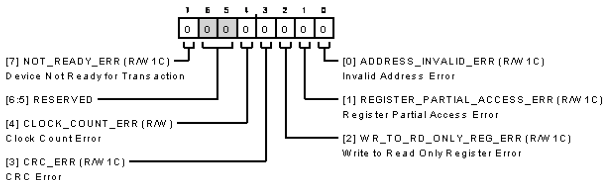
図 124. インターフェース・ステータス A レジスタ
