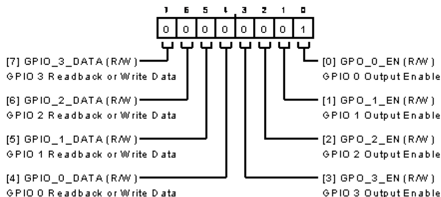
図 130. GPIO 設定 A レジスタ
