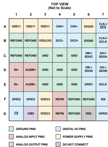
図 2. ピン配置
