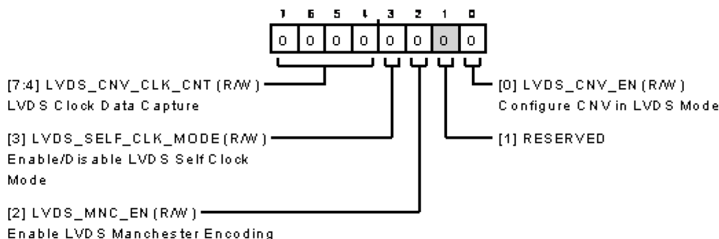
図 127. ADC データ・インターフェース設定 B レジスタ
