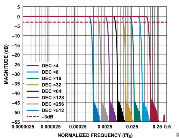
図 105. sinc5 + 補償フィルタの応答
