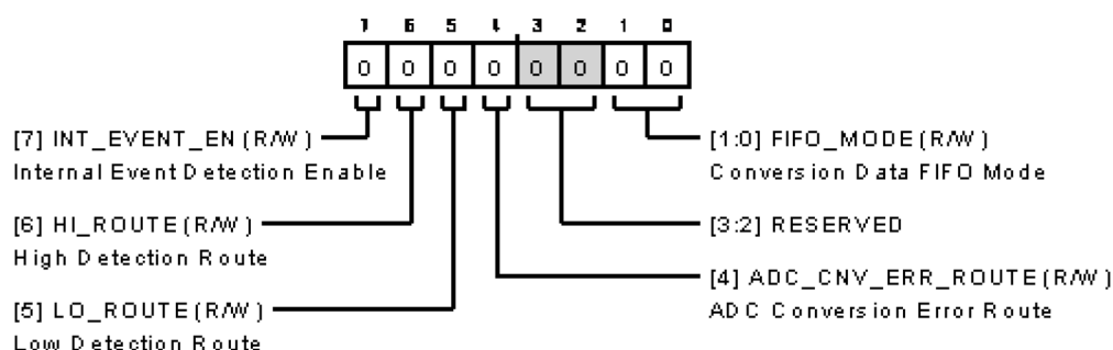
図 133. 全般的な設定レジスタ
