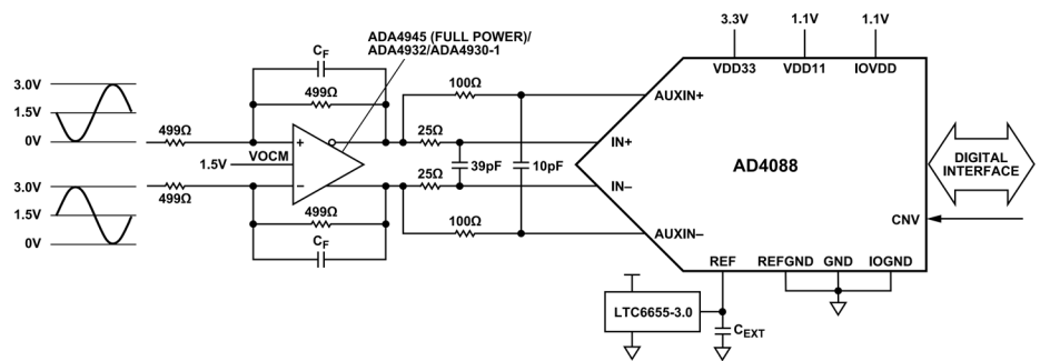
図 44. AD4088 の代表的なアプリケーション図、完全差動アンプ
