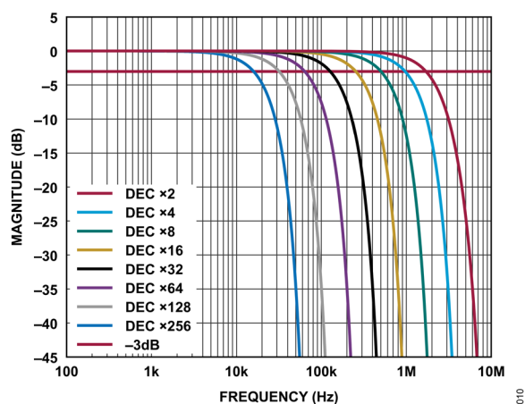
図 10. sinc5 フィルタ応答、 f_s = 20\text{MHz}
