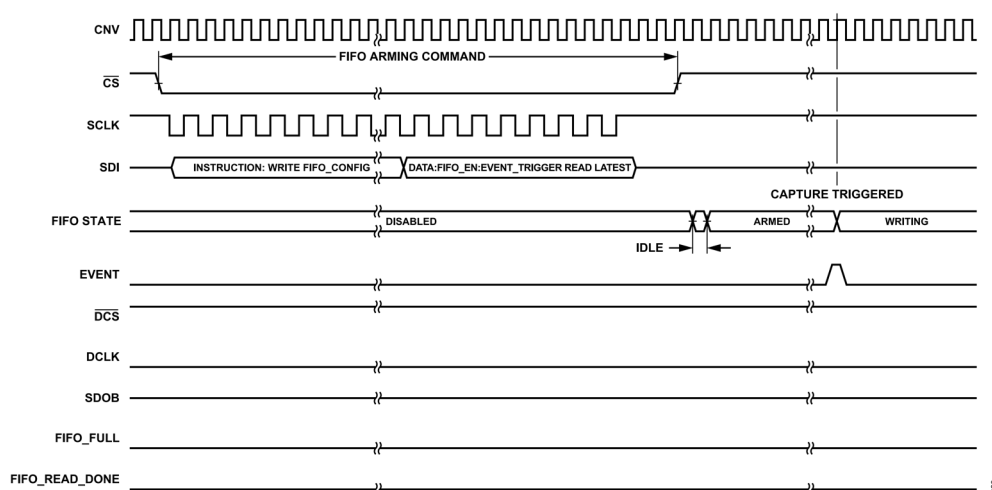
図 93. イベント・トリガされた取り込み、最新のウォーターマークの読出しの作動
