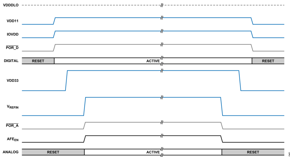
図 43. 電源シーケンス、外部生成化 IOVDD、VDD11
