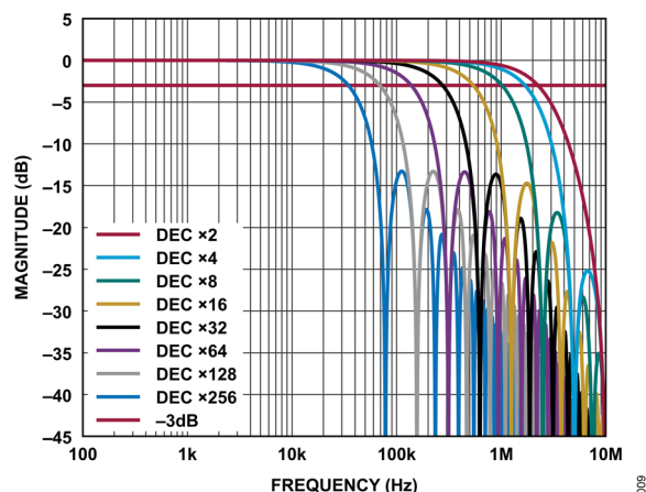
図 9. sinc1 フィルタ応答、 f_s = 20\text{MHz} (DEC \times はデシメーション率)
