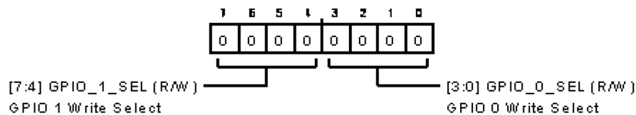
図 132. GPIO 設定 B レジスタ
