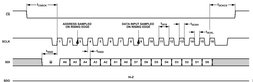
図 69. 設定 SPI タイミング、データ書き込みフレーム、8 ビット命令モード、シングル 8 ビット・レジスタ
