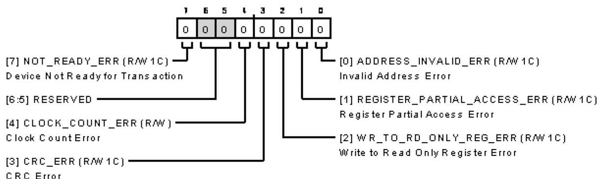
図 125. インターフェース・ステータス A レジスタ
