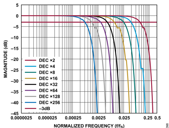
図 105. sinc5 フィルタの応答、全デシメーション率
