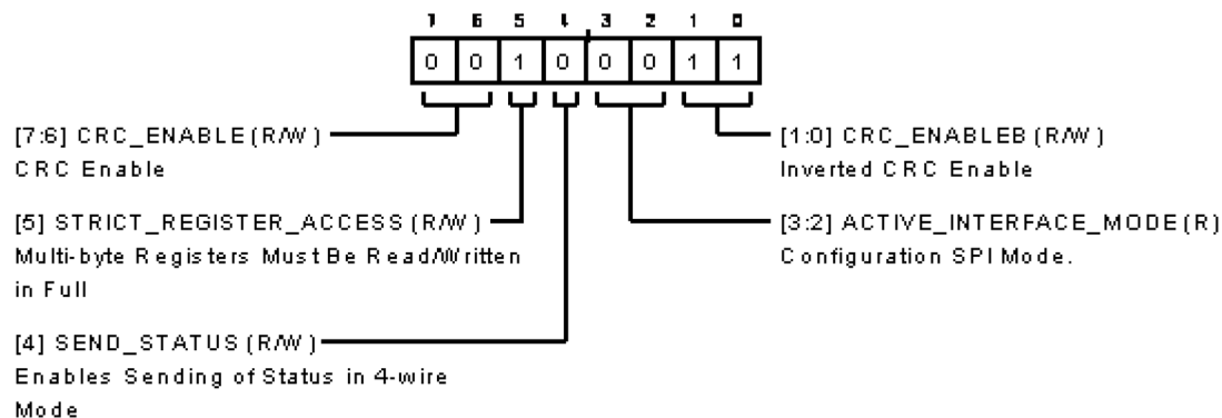
図 124. インターフェース設定 C レジスタ
