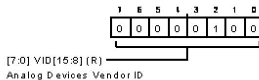
図 121. ベンダ ID ハイ・レジスタ
