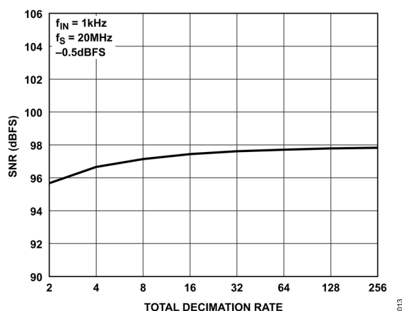
図 13. SNR と合計デシメーション率の関係、sinc5
