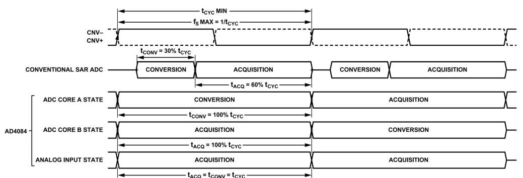
図 33. 従来の SAR と比較した変換サイクル
