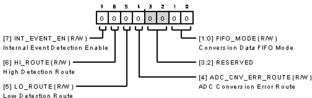
図 134. 全般的な設定レジスタ
