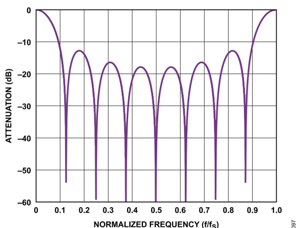
図 103. sinc1 フィルタの応答、デシメーション率 8
