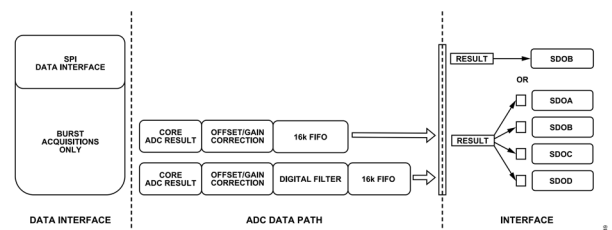
図 53. SPI データ・インターフェースのデータ経路のオプション
