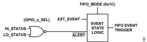
図 86. FIFO イベント検出ロジック
