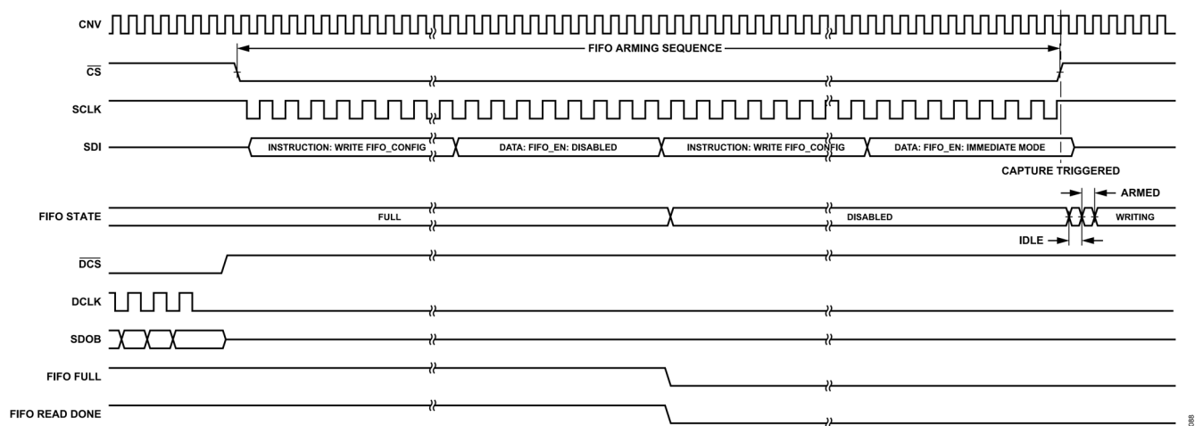
図 92. 即時トリガ・モードの再作動
