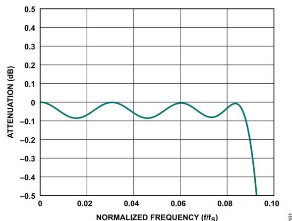
図 107. sinc5 + 補償フィルタの応答、デシメーション率 2、通過帯域リップル
