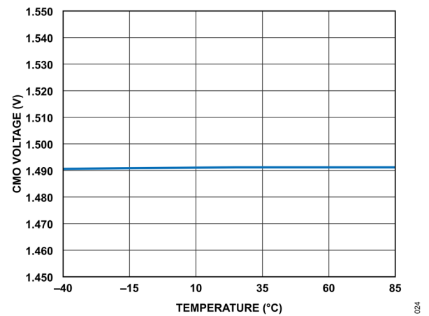
図 25. CMO 電圧と温度の関係
