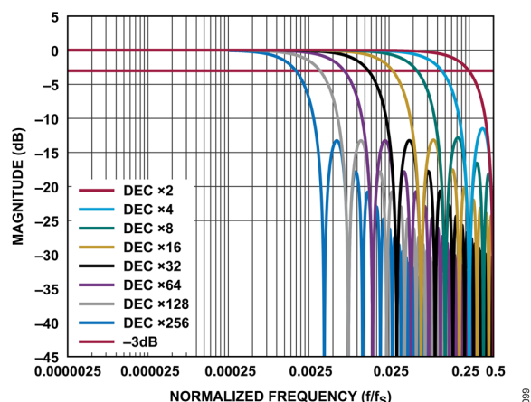
図 104. sinc1 フィルタの応答、全デシメーション率
