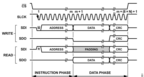
図 55. 汎用 SPI 設定の書き込み操作、CRC イネーブル済み
