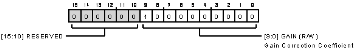
図 140. ゲイン補正レジスタ
