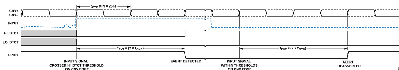
図 84. イベント検出のタイミング
