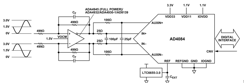
図 46. AD4084 の代表的なアプリケーション図、完全差動アンプ
