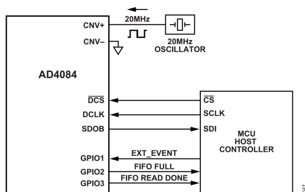
図 51. SPI データ・インターフェースのクロッキングの例
