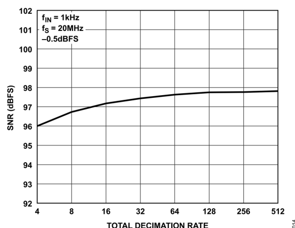
図 14. SNR と合計デシメーション率の関係、sinc5 + 補償
