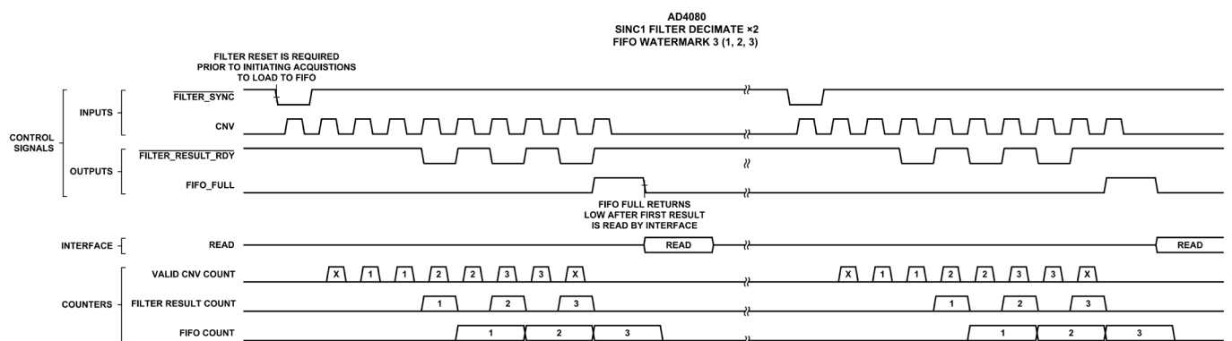
図 100. FIFO を用いたフィルタ・タイミングの説明
