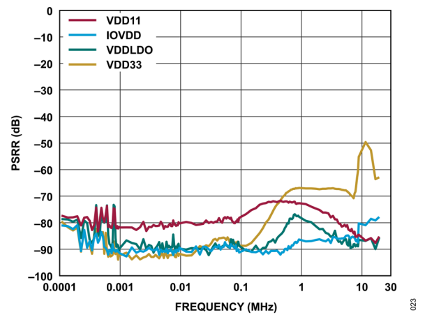
図 24. PSRR と周波数の関係
