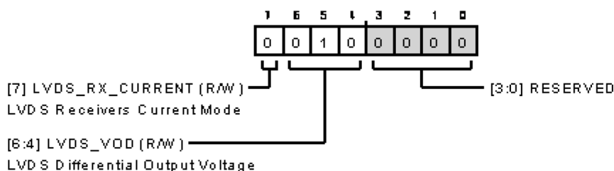
図 129. ADC データ・インターフェース設定 C レジスタ
