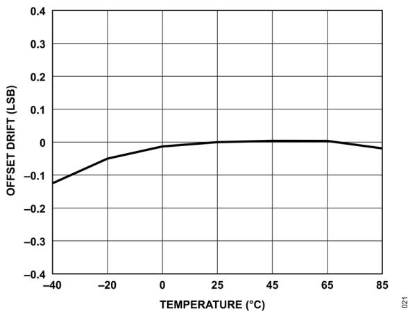
図 22. オフセット・ドリフトと温度の関係
