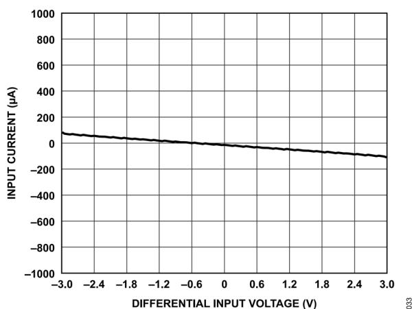
図 36. 代表値入力電流と差動入力電圧の関係
