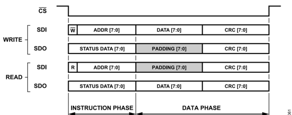
図 65. ショート命令モード、データ・ステータスをイネーブル、 CRC をイネーブル
