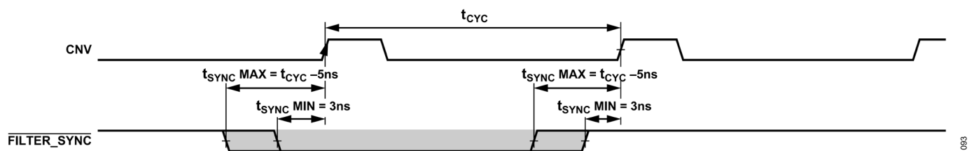
図 99. フィルタ・リセットのタイミング
