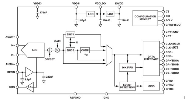
図 1. AD4084 の機能ブロック図
