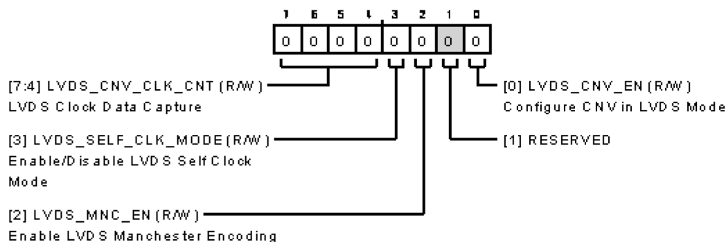
図 128. ADC データ・インターフェース設定 B レジスタ
