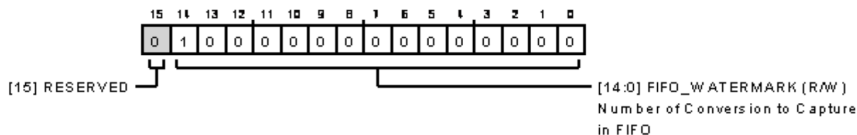
図 135. FIFO ウォーターマーク・レジスタ
