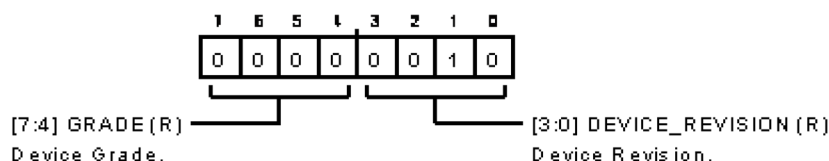
図 117. チップ・グレード・レジスタ
