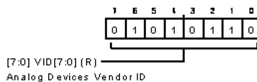
図 120. ベンダ ID ロー・レジスタ
