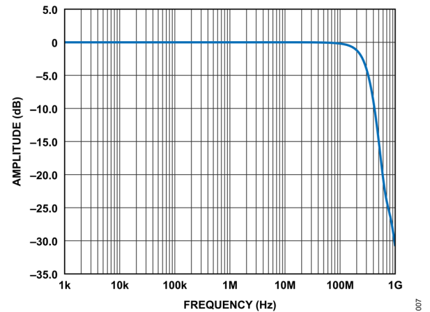
図 7. 20MSPS で小信号-3dB の帯域幅
