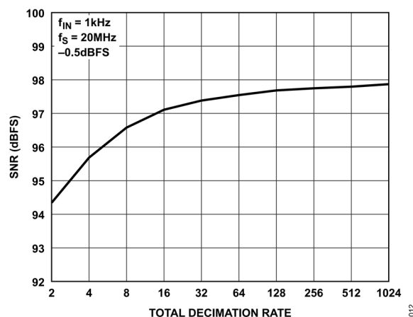
図 12. SNR と合計デシメーション率の関係、sinc1
