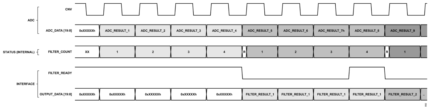
図 98. デジタル・フィルタのデシメーション率 4 のフレームの概要
