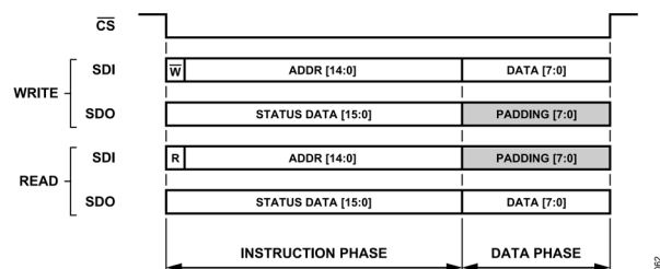
図 66. ロング命令モード、データ・ステータスをイネーブル、 CRC をディスエーブル
