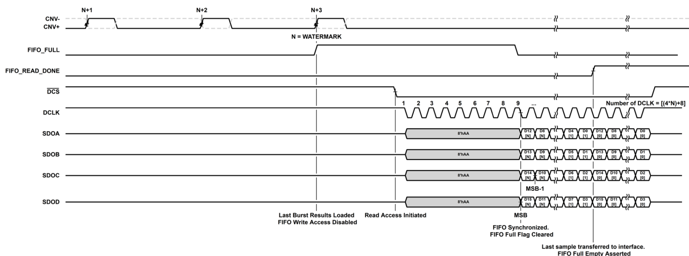
図 89. 非同期取り込み読み出しタイミング、データ FIFO をイネーブル済み、クワッド・データ・レーン設定
