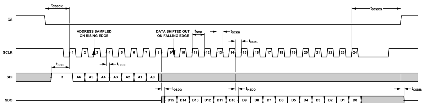
図 73. 設定 SPI タイミング、データ読出しフレーム、8 ビット命令モード、スチーミング・モード、マルチバイト・レジスタ
