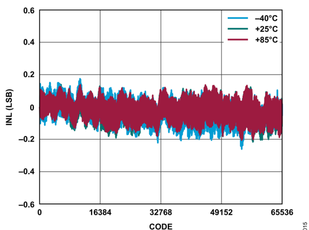
図 15. 様々な温度での INL とコードの関係、20MSPS
