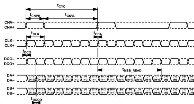
図 76. 連続変換タイミング、LVDS データ・インターフェース、デュアル・データ・レーン、エコ・クロック・モード
