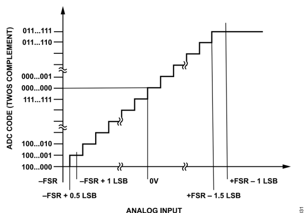
図 34. 差動出力コードに対する ADC の理想的な伝達関数 (FSR はフルスケール範囲)
