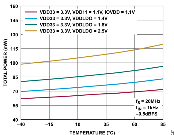
図 29. 20MSPS での総電力と温度の関係
