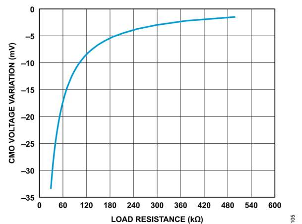
図 26. CMO 電圧変動と負荷抵抗の関係
