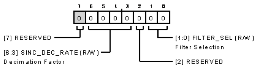
図 141. フィルタ設定レジスタ
