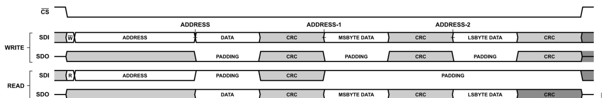
図 63. CRC をイネーブルにしたストリーミング・モードの設定、 STRICT_REGISTER_ACCESS = 0（ディスエーブル）、ADDR_ASCENSION = 0
