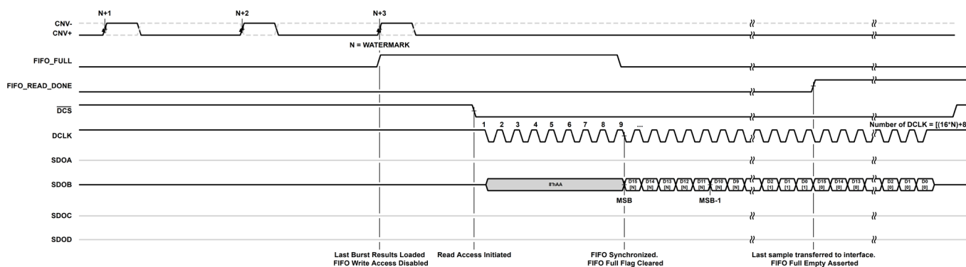
図 88. 非同期取り込み読出しタイミング、データ FIFO をイネーブル済み、シングル・データ・レーン
