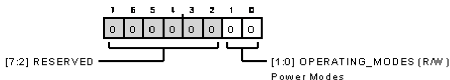
図 113. デバイス設定レジスタ
