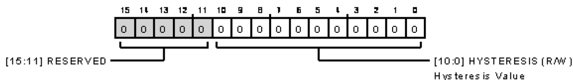
図 136. イベント検出ヒステリシス設定レジスタ
