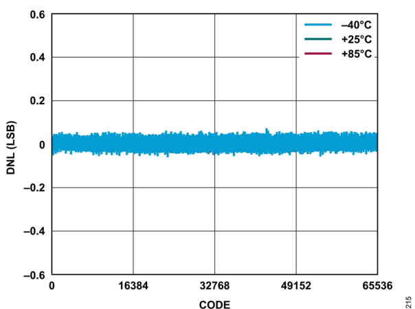
図 16. 様々な温度での DNL とコードの関係、20MSPS
