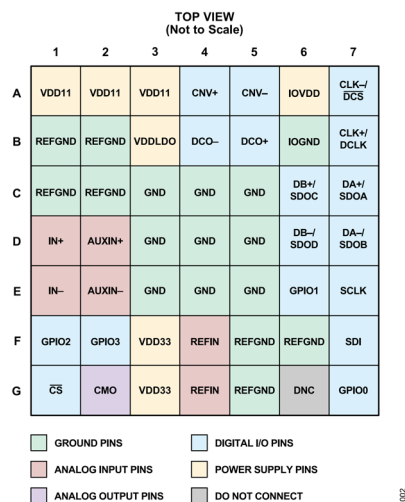
図 2. ピン配置
