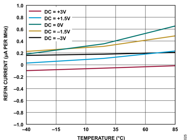
図 27. ダイナミック REFIN 電流と温度の関係
