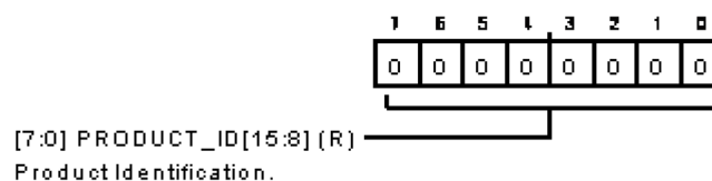
図 116. 製品 ID ハイ・レジスタ
