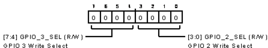
図 133. GPIO 設定 C レジスタ
