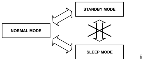
図 44. 動作モードの遷移
