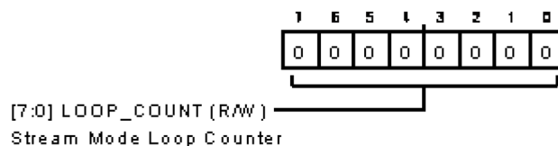
図 122. ストリーム・モード・レジスタ
