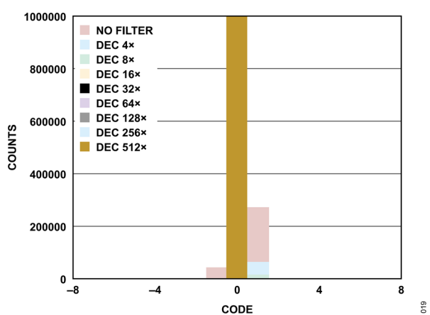
図 20. コードのヒストグラム、sinc5 + 補償、フィルタなし、デシメーション率 2、4～512
