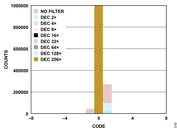
図 19. コードのヒストグラム、sinc5、フィルタなし、デシメーション率 2、4～256
