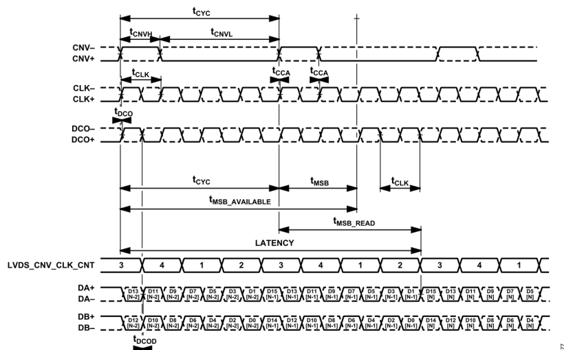
図 81. デュアル・レーン LVDS、エコー・クロック・モード、LVDS_CNV_CLK_CNT 位置の例
