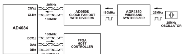
図 50. デュアル・レーン、LVDS データ・インターフェースのクロッキングの例
