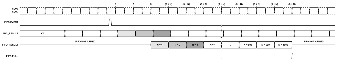
図 87. FIFO データ取り込みの例、WATERMARK = 1000
