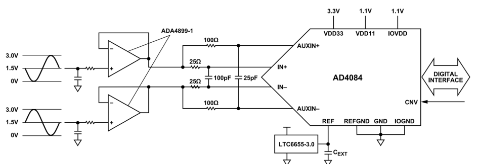
図 47. AD4084 の代表的なアプリケーション図、シングル・オペアンプ・ドライバ
