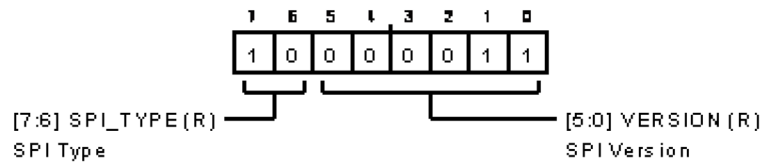
図 119. SPI リビジョン・レジスタ
