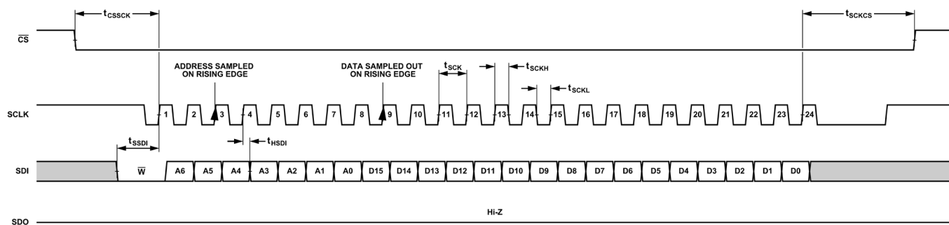
図 70. 設定 SPI タイミング、データ書き込みフレーム、8 ビット命令モード、ストリーミング・モード、マルチバイト・レジスタ
