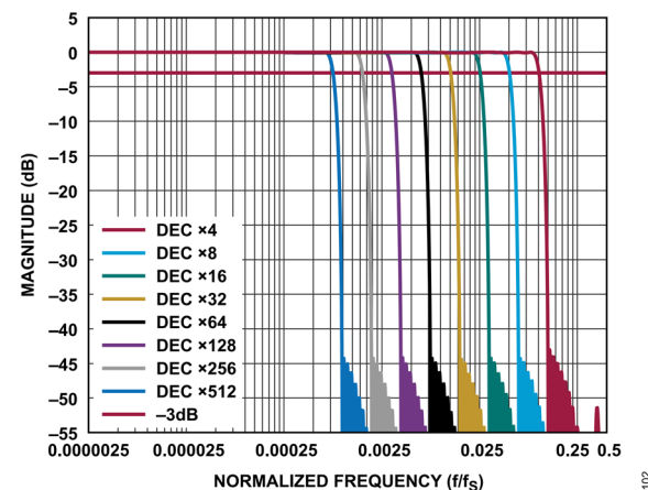
図 108. sinc5 + 補償フィルタの応答
