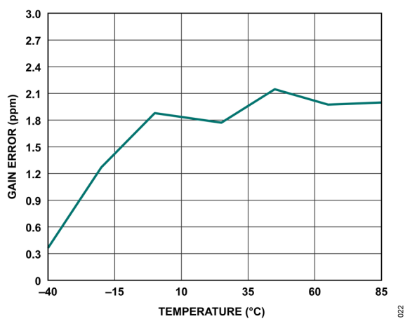
図 23. ゲイン誤差と温度の関係
