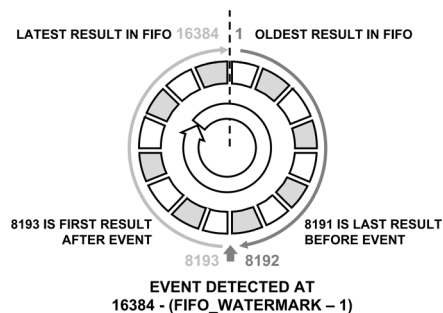
図 94. イベント取り込みモードのすべての FIFO の読出しモードの例、FIFO フィリング
