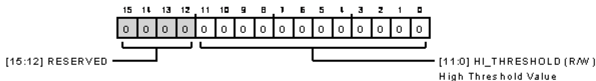
図 137. イベント検出の高閾値設定レジスタ
