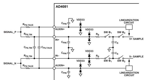
図 35. アナログ入力の等価回路モデル
