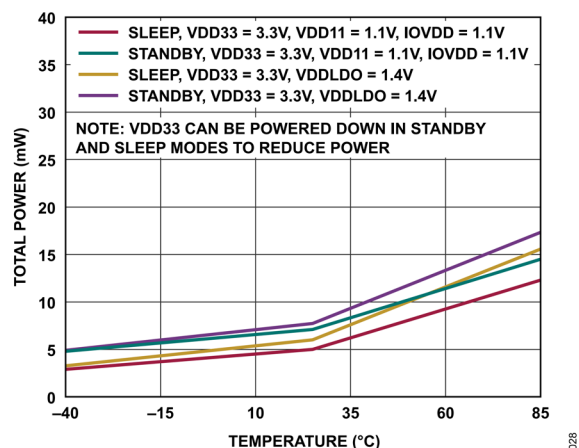
図 30. スリープ・モードおよびスタンバイ・モードでの総電力と温度の関係
