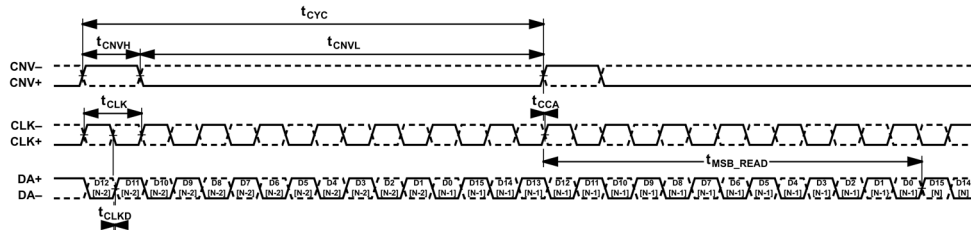
図 77. 連続変換タイミング、LVDS データ・インターフェース、シングル・データ・レーン、セルフ・クロック・モード
