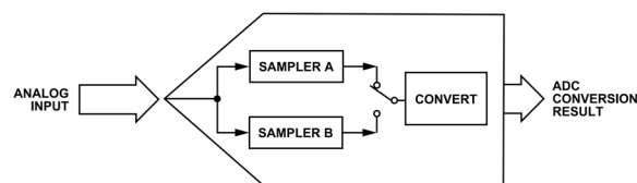
図 32. AD4084 SAR ADC の簡略表示
