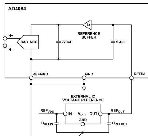
図 48. サンプル・モードの例示的接続図
