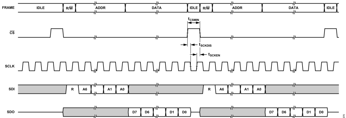
図 74. 設定 SPI タイミング、データ読出しフレーム、連続 SCLK
