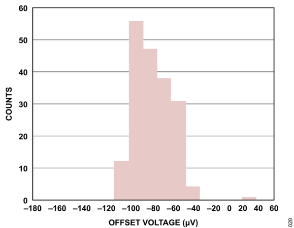
図 21. オフセット電圧のヒストグラム
