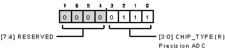
図 114. チップ・タイプ・レジスタ
