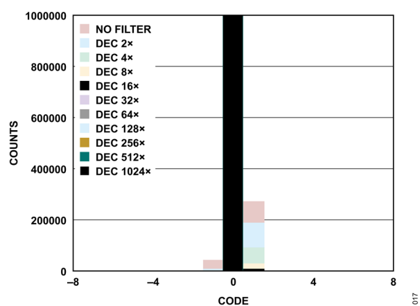
図 18. コードのヒストグラム、sinc1、フィルタなし、デシメーション率 2、4～1024
