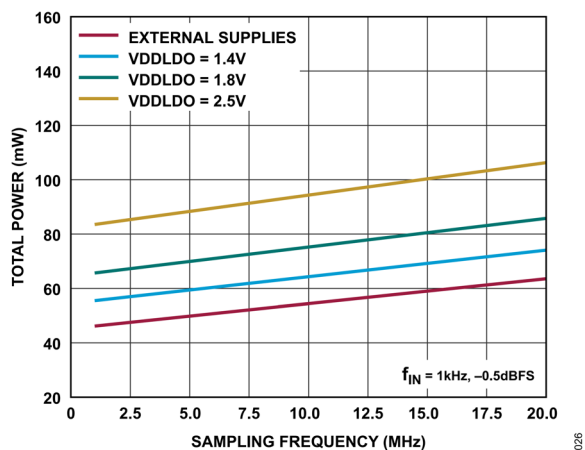
図 28. 総電力とサンプリング周波数の関係
