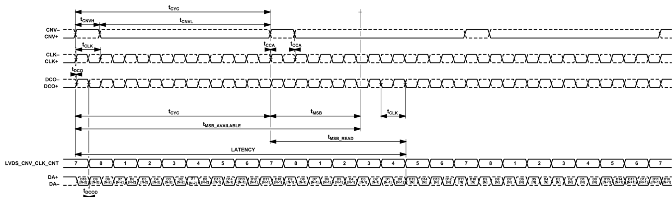
図 80. シングル・レーン LVDS、エコー・クロック・モード、LVDS_CNV_CLK_CNT 位置の例
