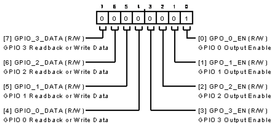
図 131. GPIO 設定 A レジスタ
