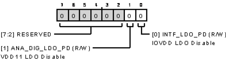
図 130. パワー・コントロール・レジスタ
