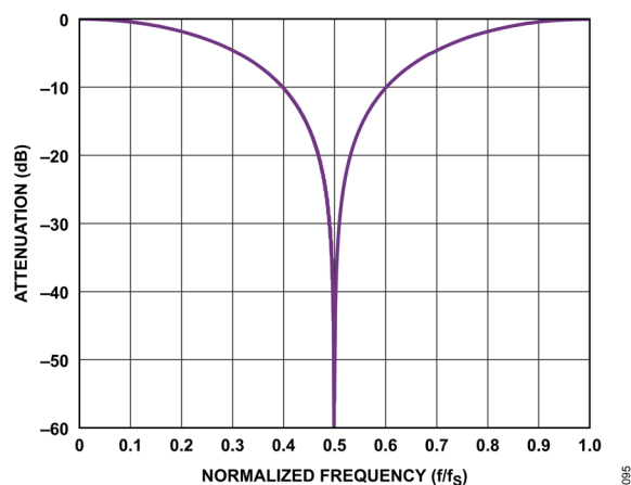
図 101. sinc1 フィルタの応答、デシメーション率 2
