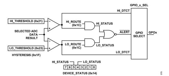
図 83. 内部生成化イベント検出信号経路
