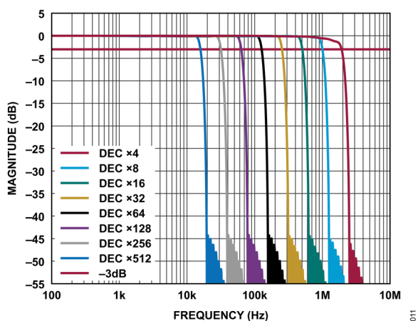
図 11. sinc5 + 補償フィルタ応答、 f_s = 20\text{MHz}
