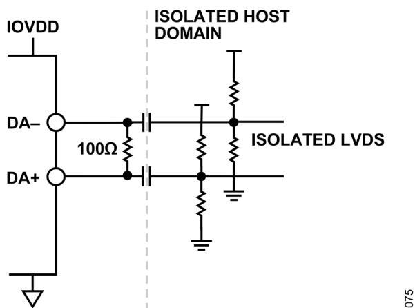
図 79. 絶縁型 LVDS
