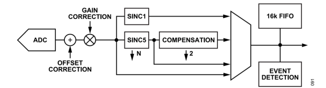
図 97. デジタル・フィルタの選択オプション
