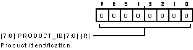
図 115. 製品 ID ロー・レジスタ
