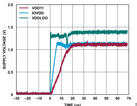
図 38. 代表的なレギュレータの起動トランジェント、コンバータがアイドル中
