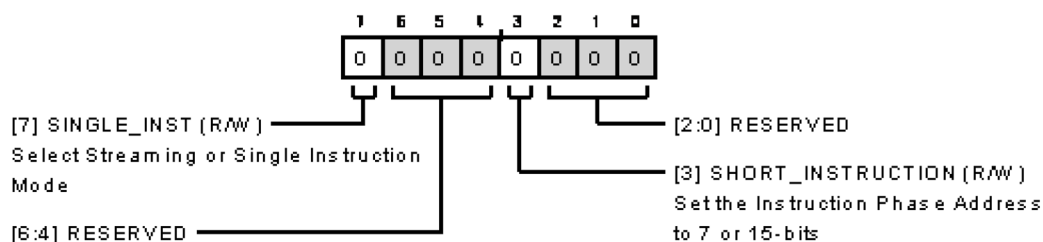
図 112. インターフェース設定 B の追加の設定値
