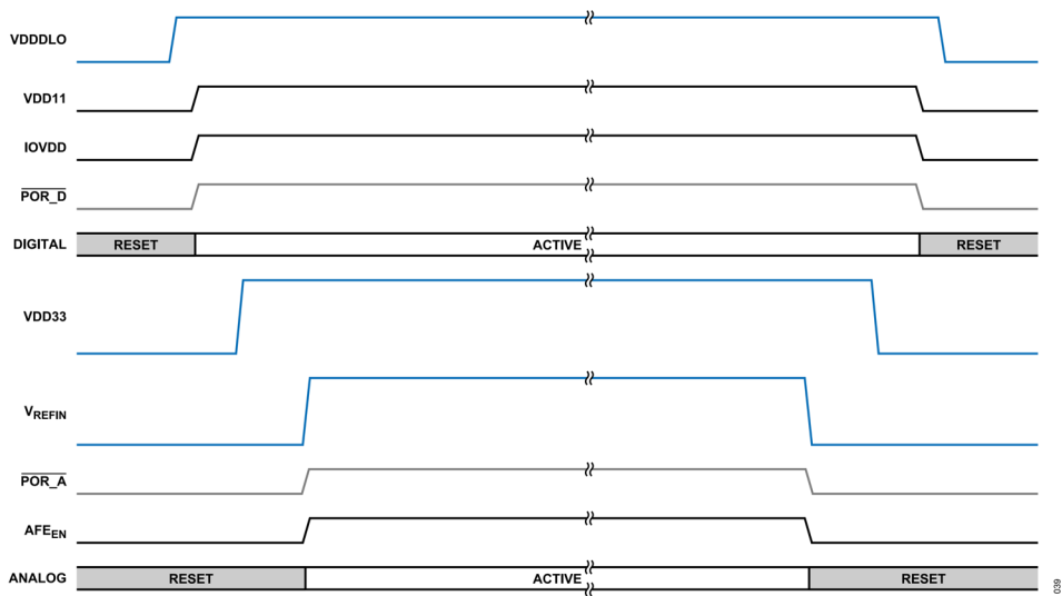
図 42. 電源シーケンス、内部生成化 IOVDD、VDD11
