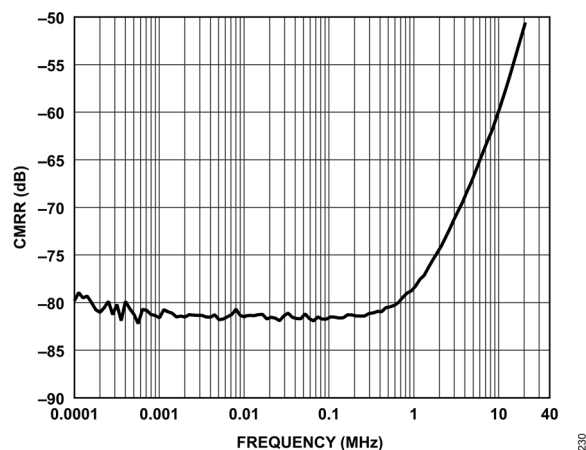
図 31. AC 同相モード除去比 (CMRR) と入力周波数の関係
