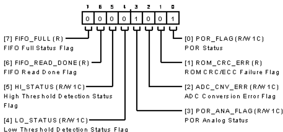
図 126. デバイス・ステータス・レジスタ
