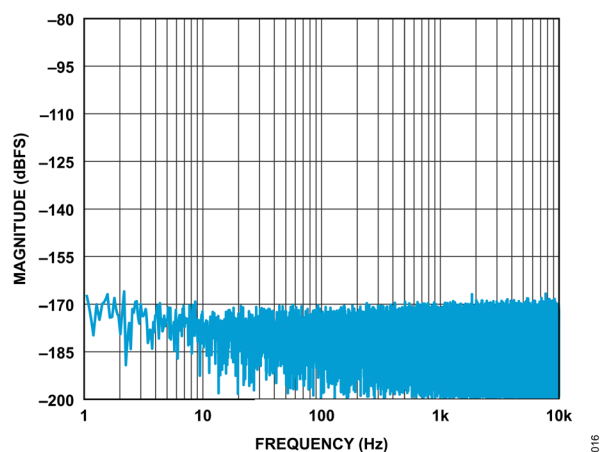
図 17. 低周波ノイズ、入力を短絡
