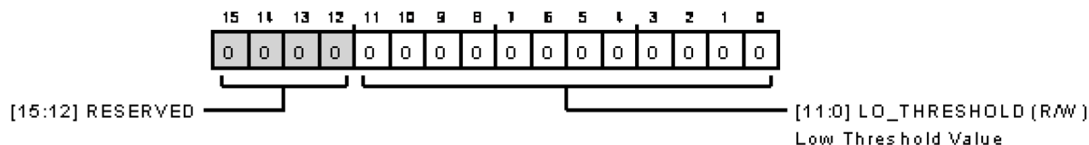
図 138. イベント検出の低閾値設定レジスタ
