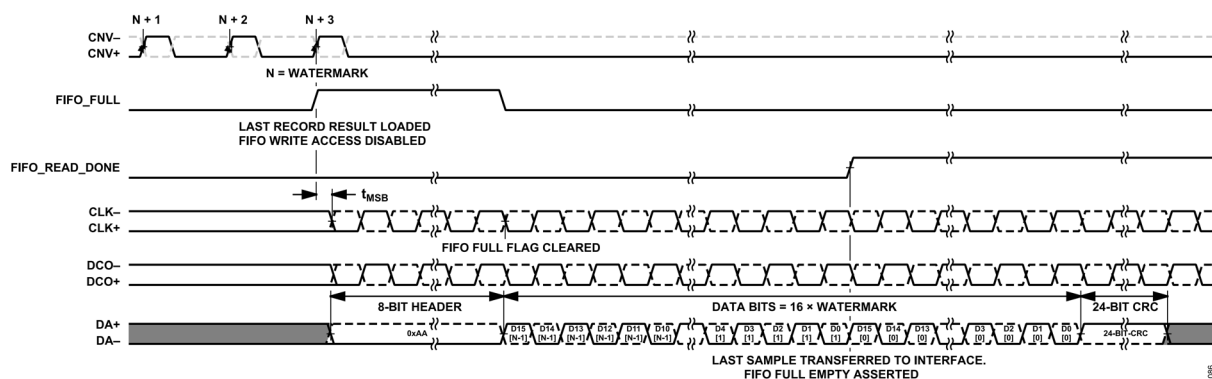
図 90. 非同期取り込み読出しタイミング、データ FIFO をイネーブル済み、LVDS 設定
