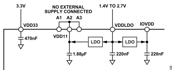
図 39. 内部安定化（1.1V）電源の構成
