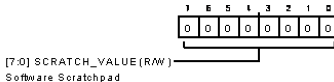
図 118. スクラッチ・パッド・レジスタ
