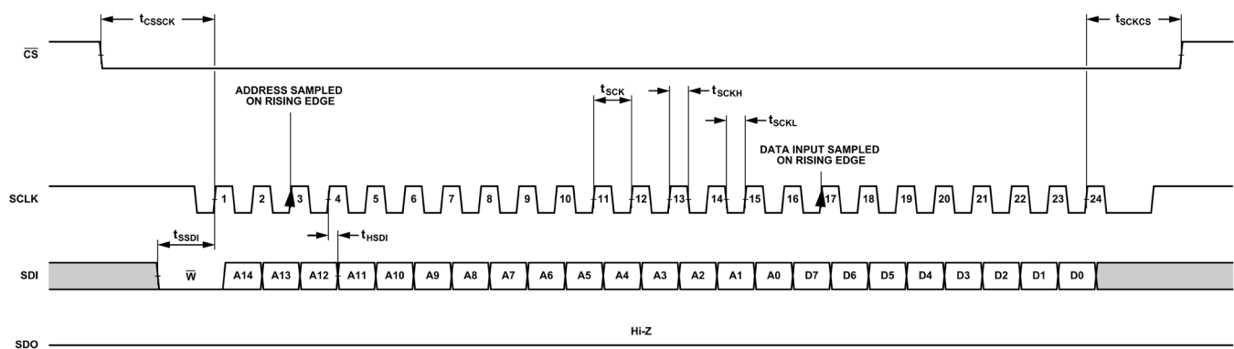
図 68. 設定 SPI タイミング、データ書き込みフレーム、16 ビット命令モード（デフォルト）
