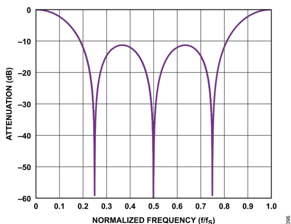
図 102. sinc1 フィルタの応答、デシメーション率 4
