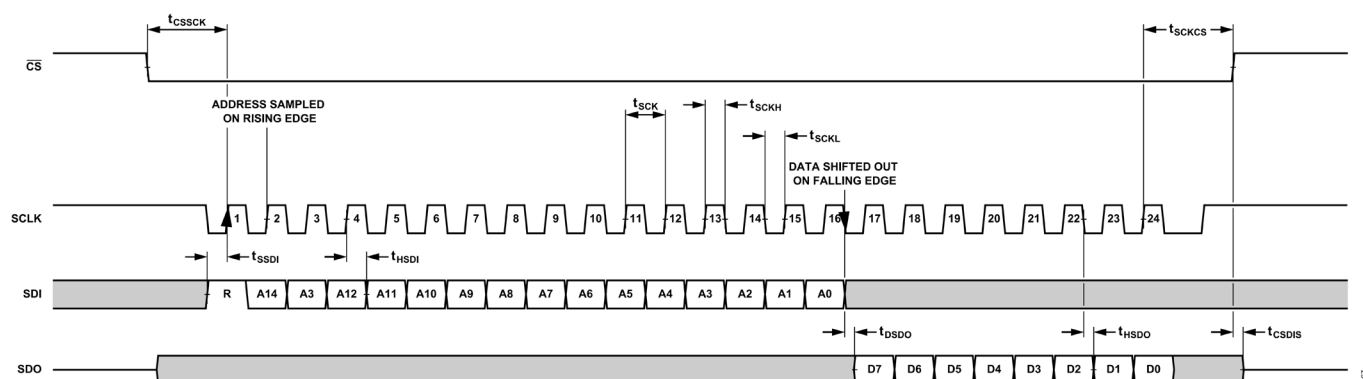
図 71. 設定 SPI タイミング、データ読出しフレーム、16 ビット命令モード（デフォルト）
