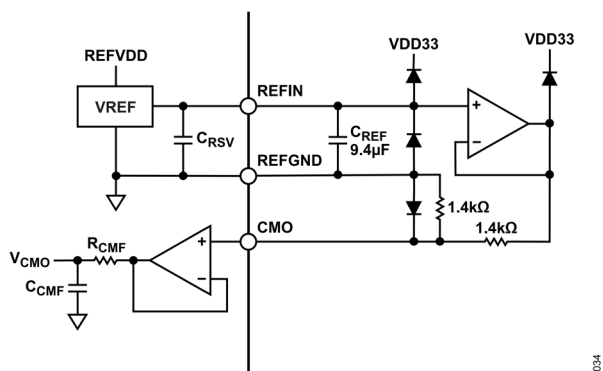
図 37. REFIN および CMO 内部等価回路と代表的な応用例
