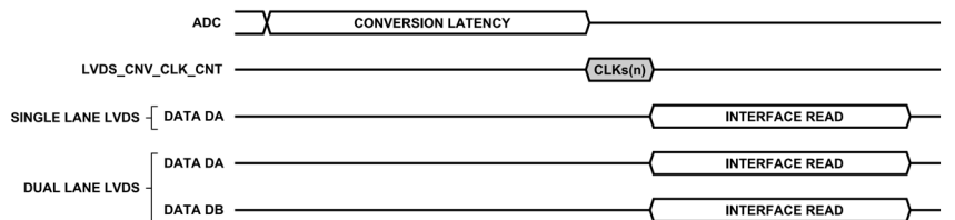
図 82. LVDS データ転送レイテンシ
