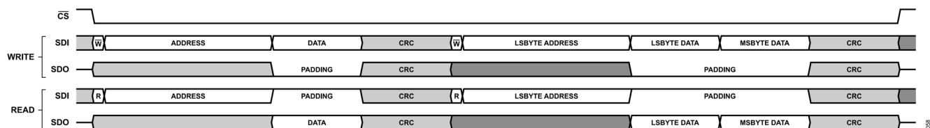
図 62. CRC をイネーブルにした単一命令モードの設定、ADDR_ASCENSION = 1
