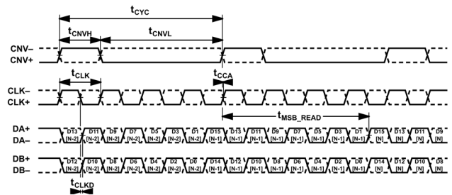
図 78. 連続変換タイミング、LVDS データ・インターフェース、デュアル・データ・レーン、セルフ・クロック・モード
