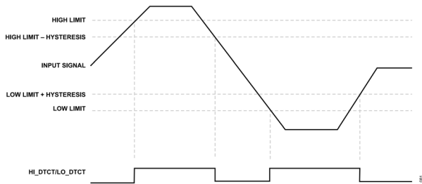
図 85. 閾値検出レベル
