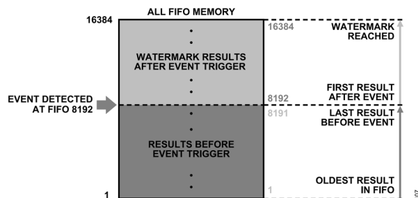
図 95. FIFO イベント取り込みモードのすべての FIFO の読出しモードの例、FIFO 内のイベント位置の特定
