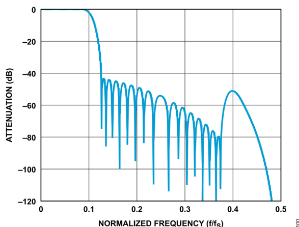
図 106. sinc5 + 補償フィルタの応答、デシメーション率 2
