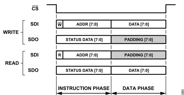
図 64. ショート命令モード、データ・ステータスをイネーブル、 CRC をディスエーブル
