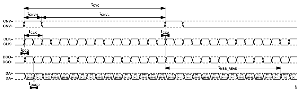
図 75. 連続変換タイミング、LVDS データ・インターフェース、シングル・データ・レーン、エコ・クロック・モード
