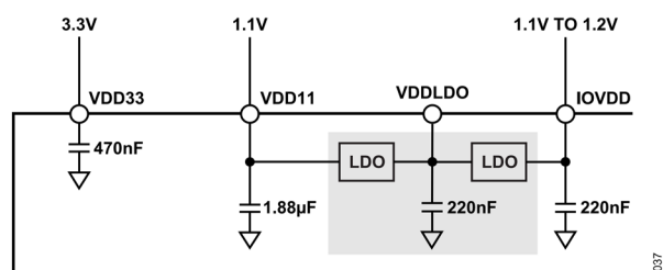
図 40. 外部電圧源の構成
