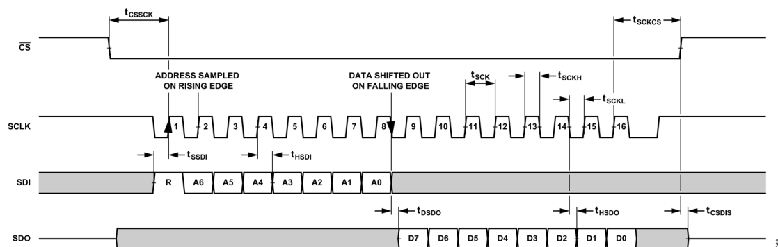
図 72. 設定 SPI タイミング、データ読出しフレーム、8 ビット命令モード
