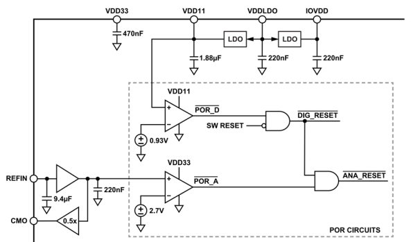
図 41. POR 回路の簡略図
