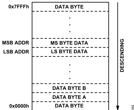
図 58. 汎用バイト幅メモリ、マルチバイト・レジスタの例
