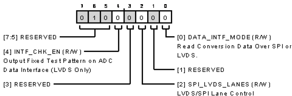
図 127. ADC データ・インターフェース設定 A レジスタ
