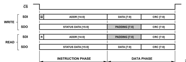
図 67. ロング命令モード、データ・ステータスをイネーブル、 CRC をイネーブル
