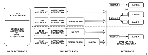
図 52. LVDS データ・インターフェースのオプション
