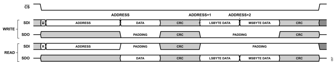
図 61. CRC をイネーブルにしたストリーミング・モードの設定、ADDR_ASCENSION = 1
