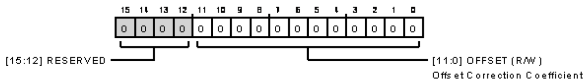
図 139. オフセット補正レジスタ
