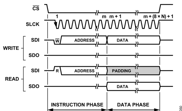
図 54. 汎用 SPI 設定フレーム、CRC ディスエーブル
