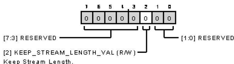
図 123. 転送設定レジスタ
