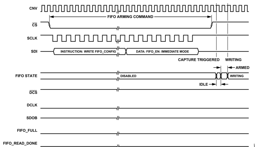
図 91. 即時トリガ・モードの作動
