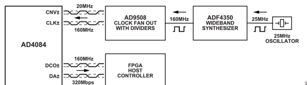
図 49. シングル・レーン、LVDS データ・インターフェースのクロッキングの例
