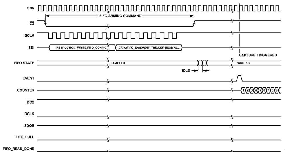
図 96. イベント・トリガ取り込みモード、すべての FIFO の読出しの再作動
