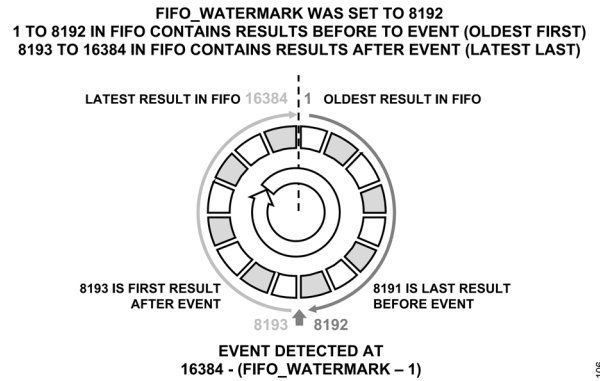
図 92. イベント取り込みモードのすべての FIFO 読出しモード例、FIFO フィリング
