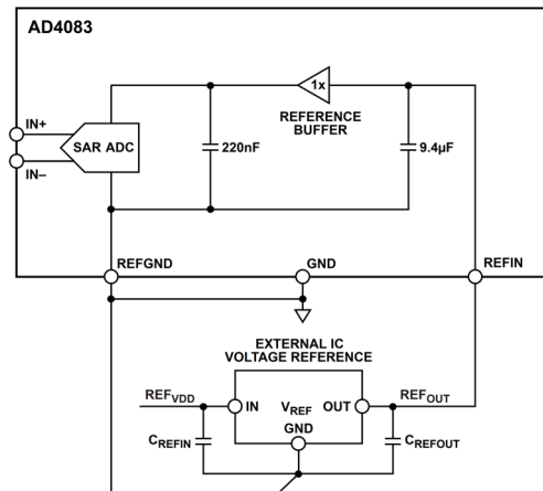
図 46. AD4083 一般的な外部リファレンス設計の機能図
