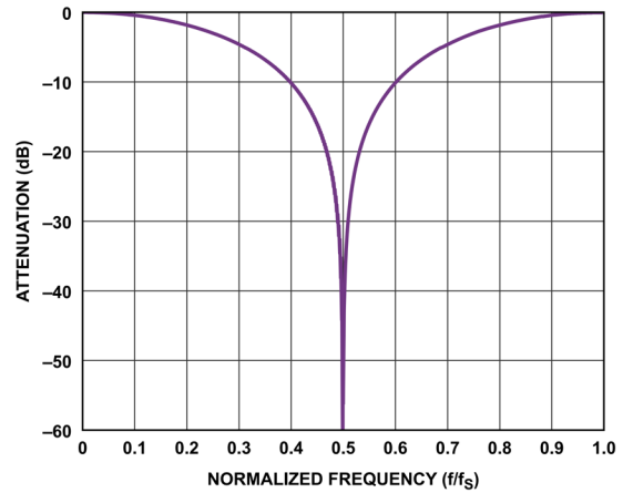
図 99. sinc1 フィルタの応答、デシメーション率 2
