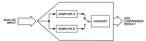
図 30. AD4083 SAR ADC の簡略表示
