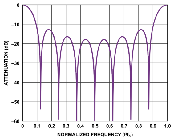
図 101. sinc1 フィルタの応答、デシメーション率 8
