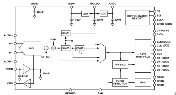
図 1. AD4083 の機能ブロック図
