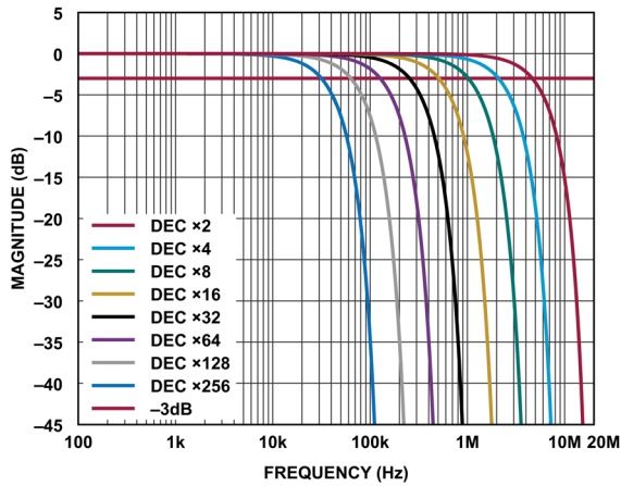
図 9. sinc1 フィルタ応答、 f_s = 40\text{MHz} (DEC \times はデシメーション率)
