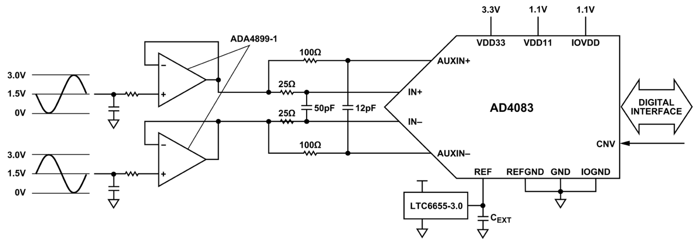
図 45. AD4083 の代表的なアプリケーション図、シングル・オペアンプ・ドライバ
