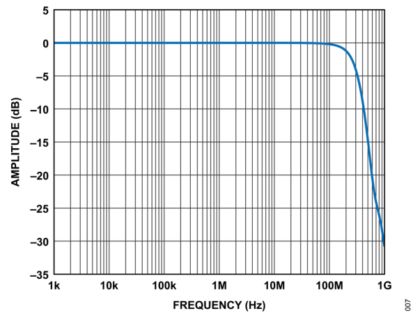
図 7. 40MSPS で小信号-3dB の帯域幅
