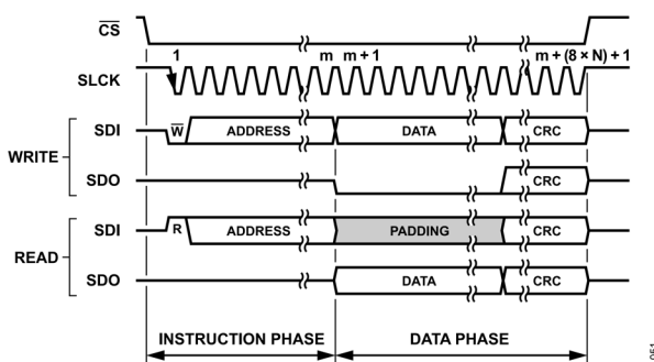
図 53. 一般的な SPI 設定の書込み操作、CRC イネーブル
