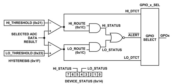
図 81. 内部発生イベント検出信号経路
