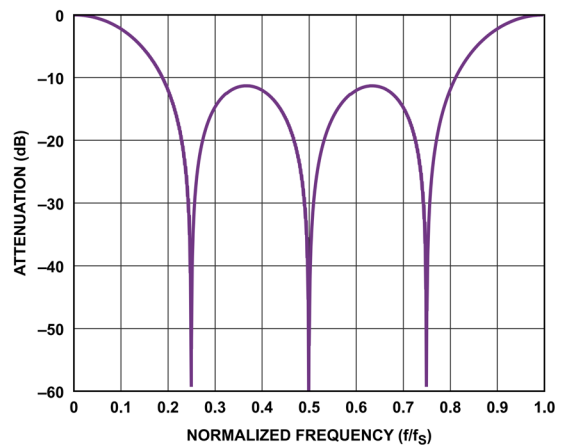
図 100. sinc1 フィルタの応答、デシメーション率 4
