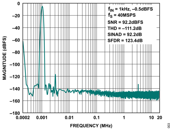
図 3. 高速フーリエ変換 (FFT) 40MSPS、 f_{IN} = 1\text{kHz} 、 -0.5\text{dBFS}
