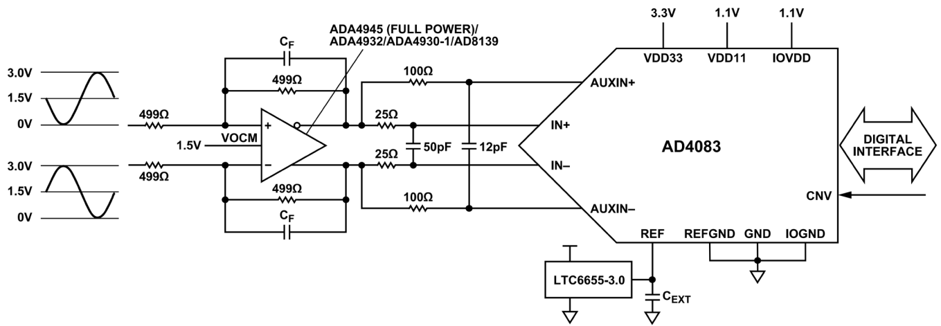
図 44. AD4083 の代表的なアプリケーション図、完全差動アンプ
