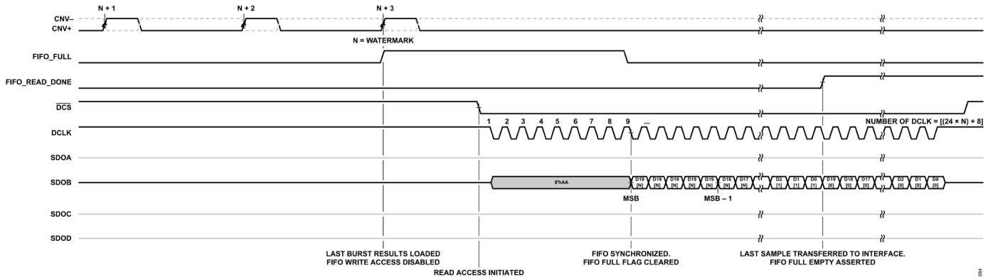
図 86. 非同期取り込み読出しタイミング、データ FIFO イネーブル、シングル・データ・レーン
