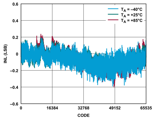
図 14. 様々な温度での INL とコードの関係、40MSPS
