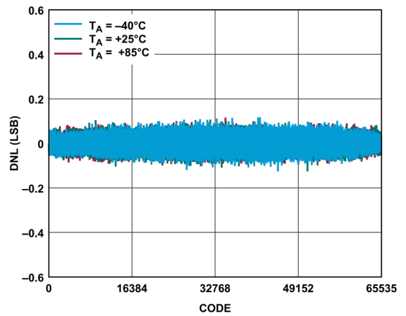
図 13. 様々な温度での DNL とコードの関係、40MSPS
