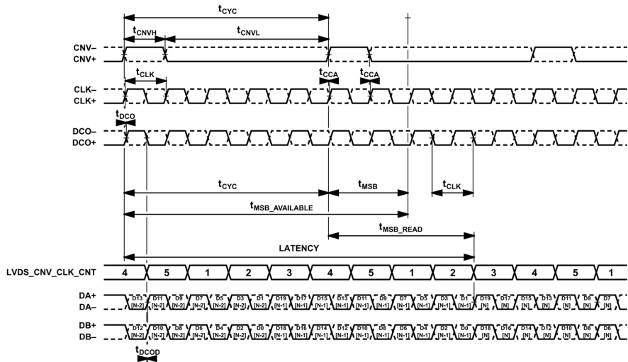
図 79. デュアル・レーン LVDS、エコー・クロック・モードでの LVDS_CNV_CLK_CNT 位置の例
