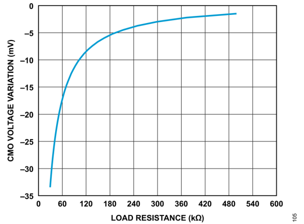
図 24. CMO 電圧変動と負荷抵抗の関係
