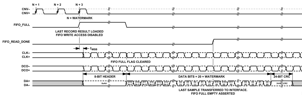
図 88. 非同期取り込み読出しタイミング、データ FIFO イネーブル、LVDS 設定
