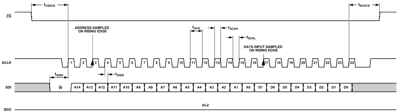
図 66. 設定 SPI タイミング、データ書き込みフレーム、16 ビット命令モード (デフォルト)
