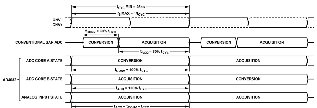
図 31. 従来の SAR と比較した変換サイクル
