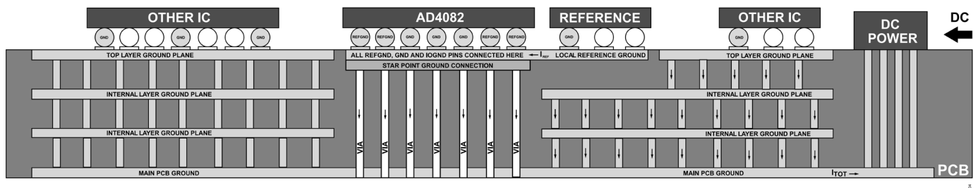
図 108. PCB グラウンド・プレーンの推奨レイアウト
