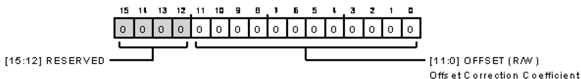
図 137. オフセット補正レジスタ
