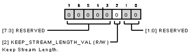
図 121. 転送設定レジスタ
