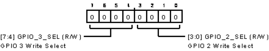
図 131. GPIO 設定 C レジスタ
