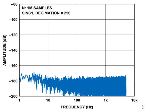
図 15. 入力短絡時のノイズ・フロア
