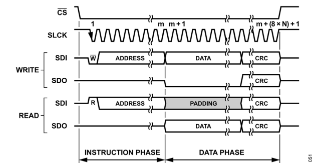
図 53. 一般的な SPI 設定の書込み操作、CRC イネーブル
