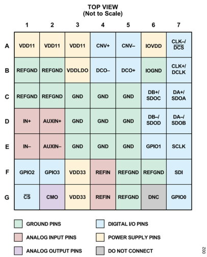
図 2. ピン配置
