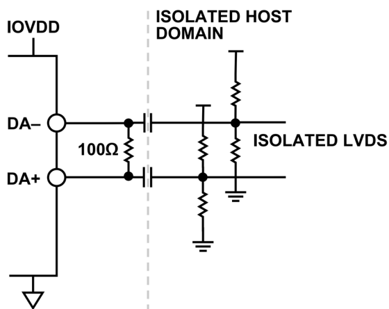
図 77. 絶縁型 LVDS
