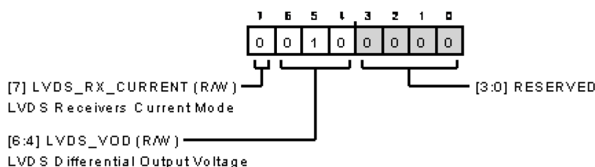
図 127. ADC データ・インターフェース設定 C レジスタ
