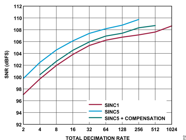
図 12. すべてのフィルタについて合計の S/N 比と 合計デシメーションの関係
