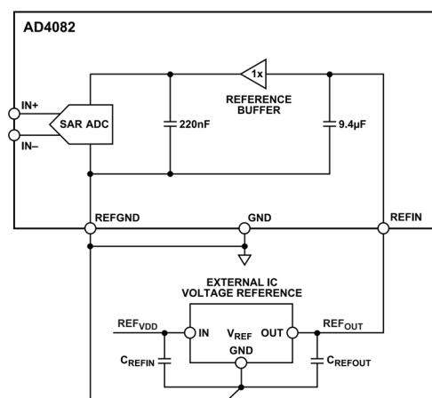
図 46. AD4082 一般的な外部リファレンス設計の機能図
