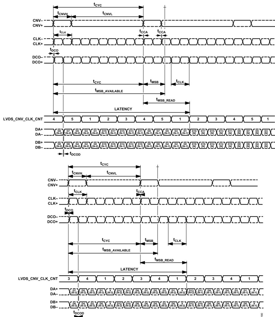
図 79. デュアル・レーン LVDS、エコー・クロック・モードでの LVDS_CNV_CLK_CNT 位置の例
