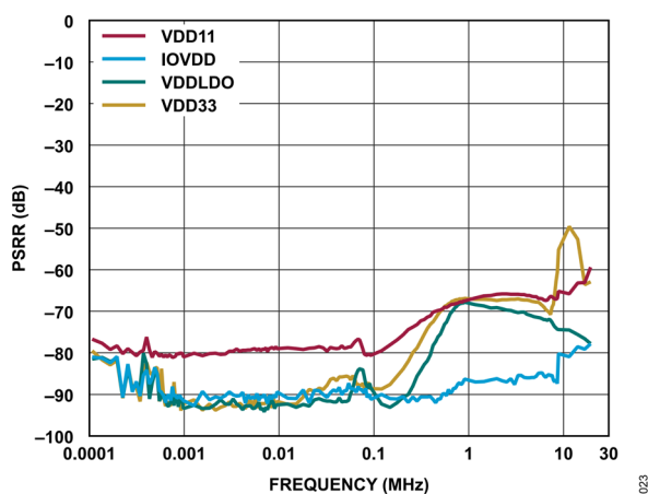
図 22. 電源電圧変動除去比 (PSRR) と周波数の関係
