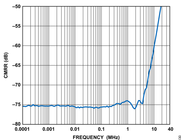
図 29. AC 同相モード除去比 (CMRR) と入力周波数の関係
