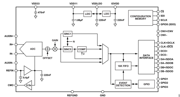
図 1. AD4082 の機能ブロック図
