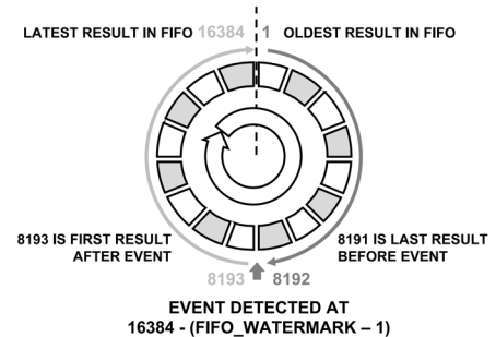
図 92. イベント取り込みモードのすべての FIFO 読出しモード例、FIFO フィリング
