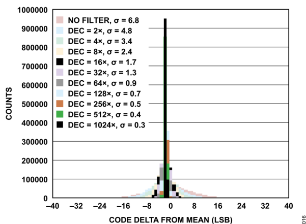
図 16. コードのヒストグラム、sinc1 フィルタとデシメーション・レートの関係
