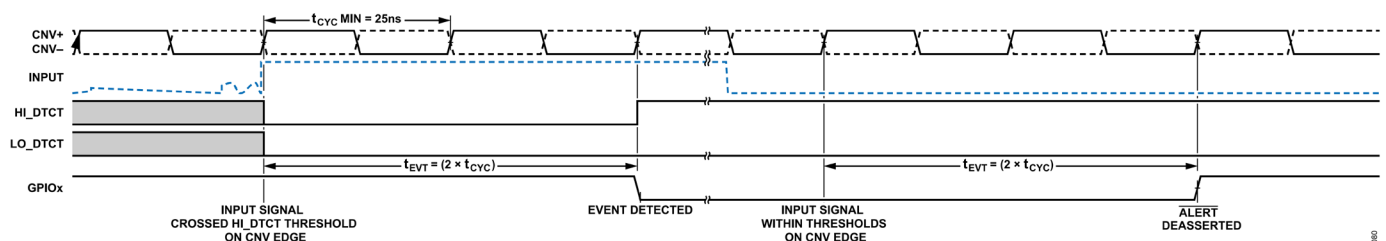
図 82. イベント検出のタイミング
