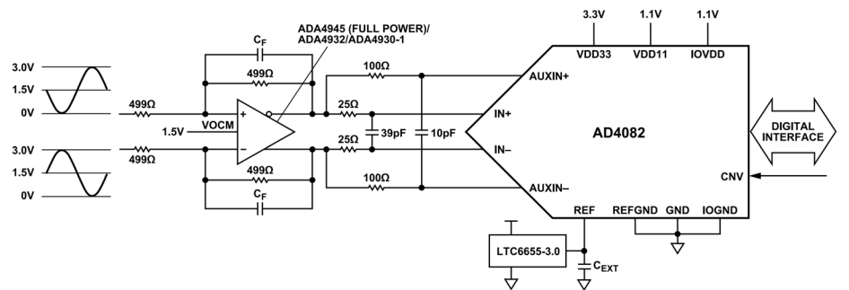
図 44. AD4082 の代表的なアプリケーション図、完全差動アンプ
