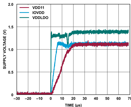
図 36. 代表的なレギュレータの起動トランジェント、コンバータがアイドリング
