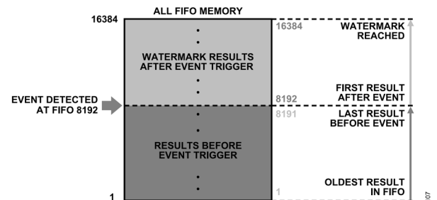
図 93. FIFO イベント取り込みモードのすべての FIFO 読出しモード例、FIFO 内のイベント位置の特定
