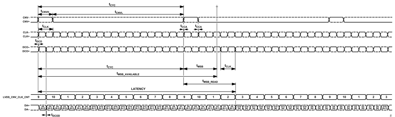
図 78. シングル・レーン LVDS、エコー・クロック・モードでの LVDS_CNV_CLK_CNT 位置の例
