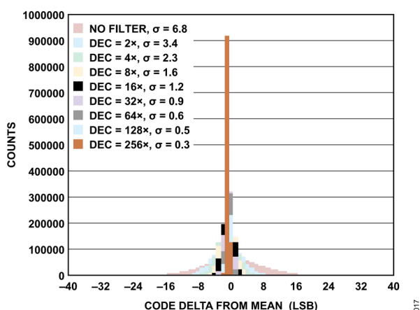
図 17. コードのヒストグラム、sinc1、フィルタなし、デシメーション率 2、4～1024
