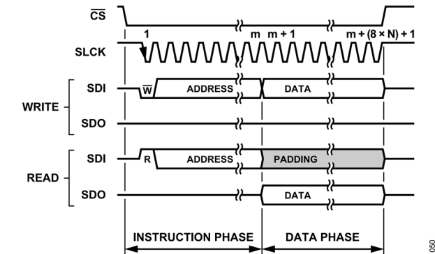
図 52. 一般的な SPI 設定フレーム、CRC ディスエーブル
