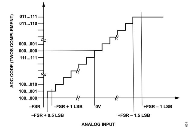
図 32. 差動出力コードに対する ADC の理想的な伝達関数 (FSR はフルスケール範囲)
