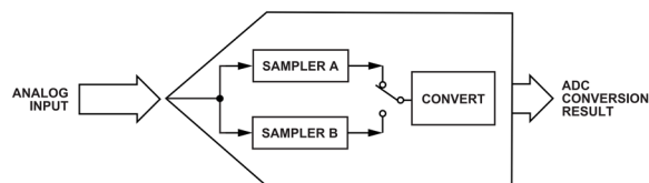
図 30. AD4082 SAR ADC の簡略表示
