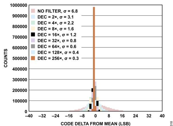
図 18. コードのヒストグラム、sinc5、フィルタなし、デシメーション率 2、4～256
