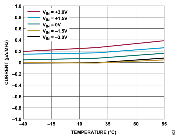
図 25. ダイナミック REFIN 電流と温度の関係
