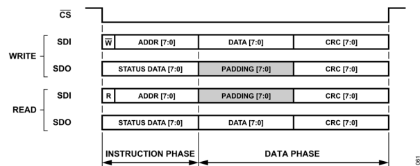
図 63. ショート命令モード、データ・ステータスをイネーブル、CRC をイネーブル
