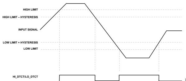
図 83. 閾値検出レベル
