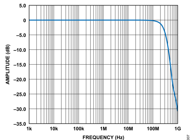
図 7. 10MSPS で小信号-3dB の帯域幅
