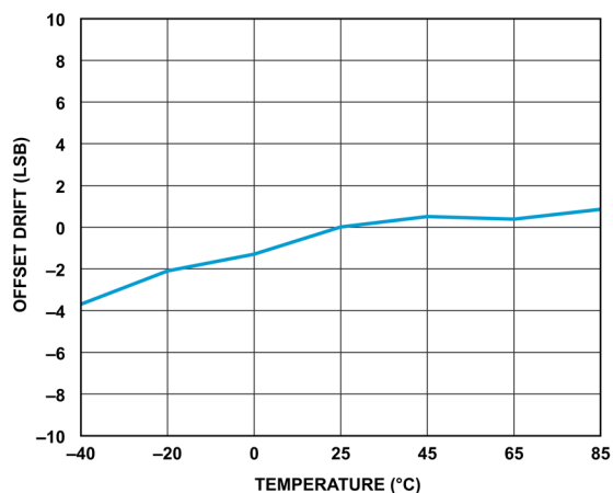
図 21. オフセット・ドリフトと温度の関係
