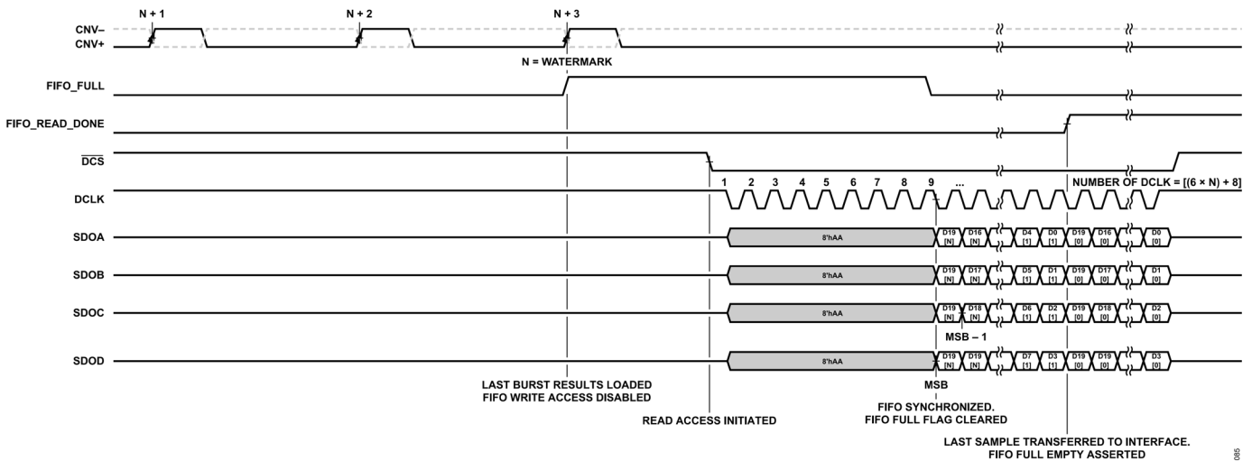
図 86. 非同期読み出しタイミング、データ FIFO をイネーブル済み、クワッドデータ・レーン設定
