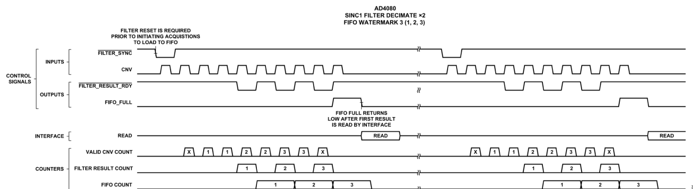
図 97. FIFO を用いたフィルタ・タイミングの説明
