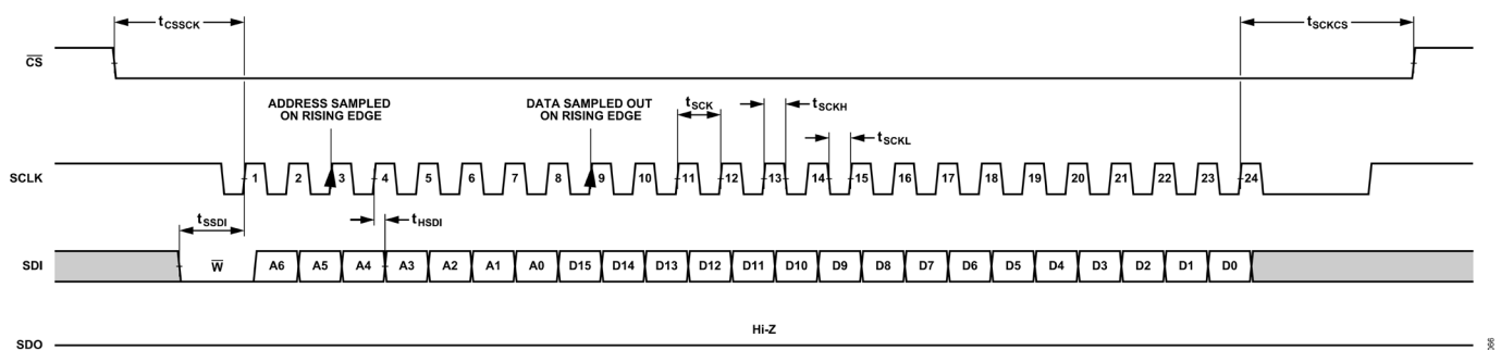
図 67. 設定 SPI タイミング、データ書き込みフレーム、8 ビット命令モード、ストリーミング・モード、マルチバイト・レジスタ
