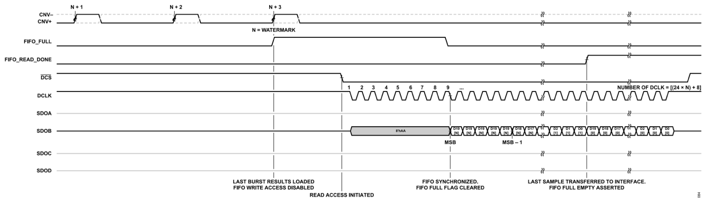
図 85. 非同期読み出しタイミング、データ FIFO をイネーブル済み、シングル・データ・レーン
