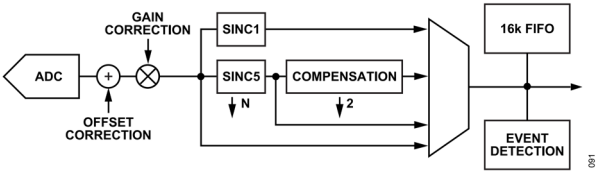
図 94. デジタル・フィルタの選択オプション
