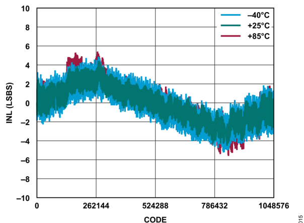
図 15. 様々な温度での INL とコードの関係、40MSPS
