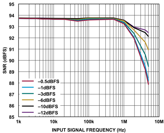
図 5. SNR と入力信号周波数の関係 (振幅 = -0.5\text{dBFS} 、 -1\text{dBFS} 、 -3\text{dBFS} 、 -6\text{dBFS} 、 -10\text{dBFS} 、 -12\text{dBFS} )
