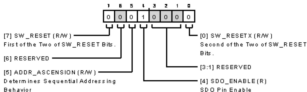
図 108. インターフェース設定 A の設定値
