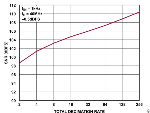
図 13. SNR と合計デシメーション率の関係、Sinc5
