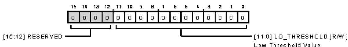
図 135. イベント検出の低閾値設定レジスタ
