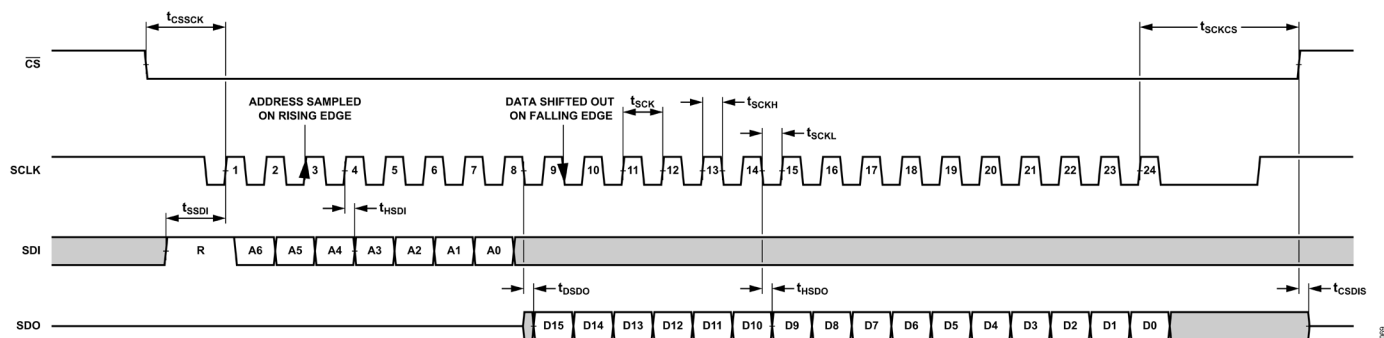
図 70. 設定 SPI タイミング、データ読出しフレーム、8 ビット命令モード、スレーミング・モード、マルチバイト・レジスタ
