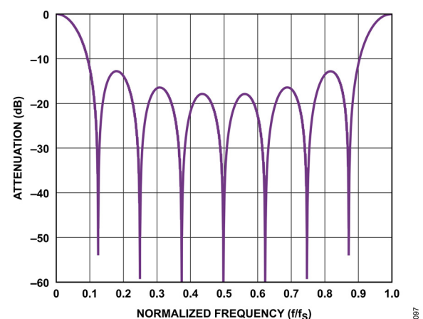
図 100. Sinc1 フィルタの応答、デシメーション率 8
