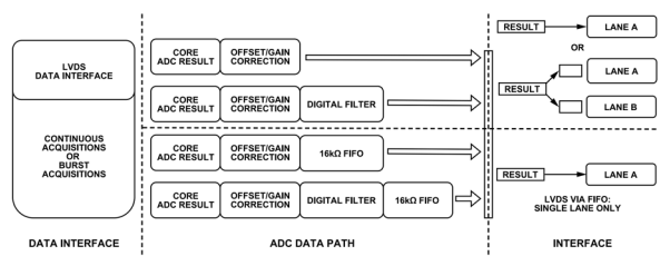
図 49. LVDS データ・インターフェースのオプション
