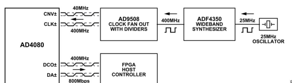
図 46. シングル・レーン、LVDS データ・インターフェースのクロッキングの例
