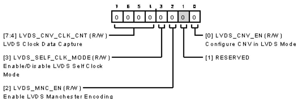
図 125. ADC データ・インターフェース設定 B レジスタ
