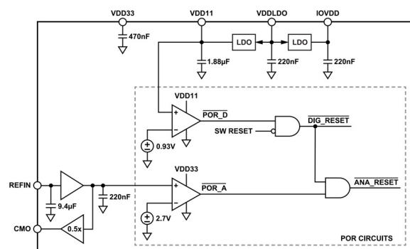
図 39. POR 回路の簡略図
