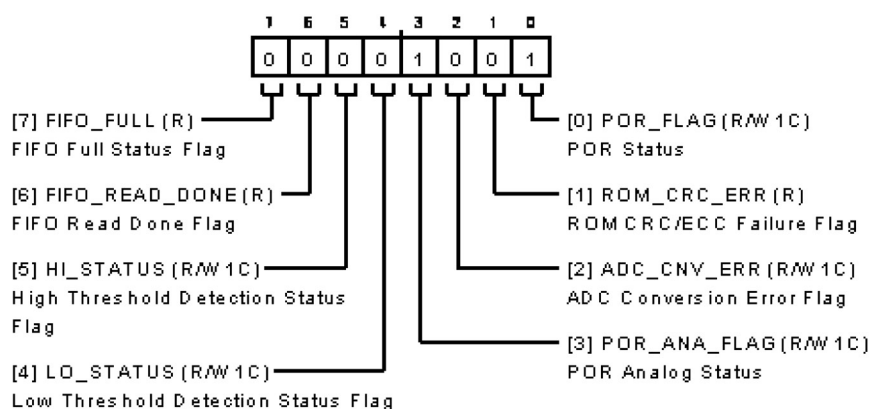
図 123. デバイス・ステータス・レジスタ
