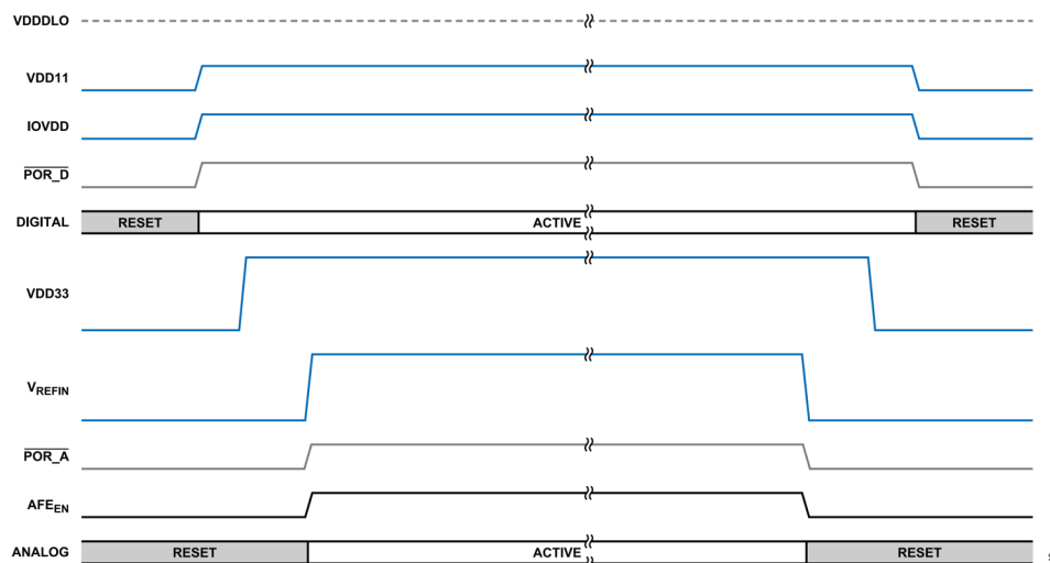
図 41. 電源シーケンス、外部生成化 IOVDD、VDD11
