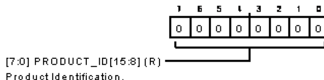
図 113. 製品 ID ハイ・レジスタ
