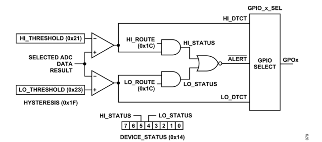
図 80. 内部生成化イベント検出信号経路
