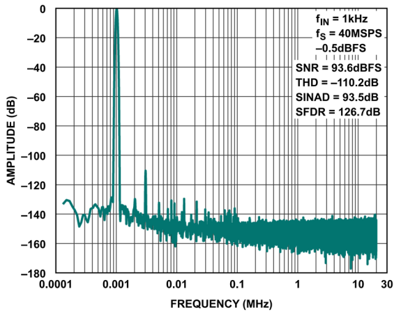
図 3. FFT 40MSPS、 f_{IN} = 1\text{kHz} 、 -0.5\text{dBFS}
