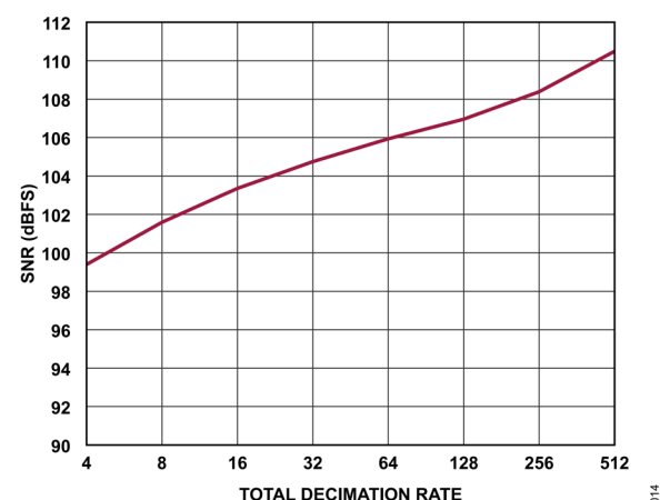
図 14. SNR と合計デシメーション率の関係、Sinc5 + 補償
