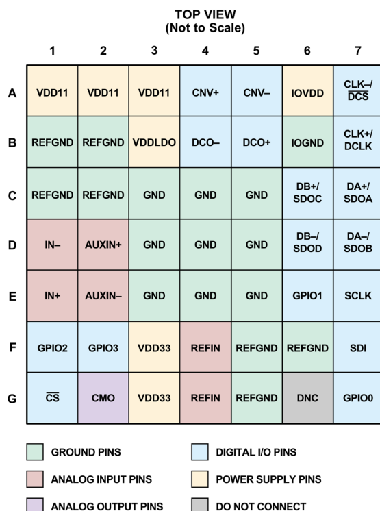
図 2. ピン配置
