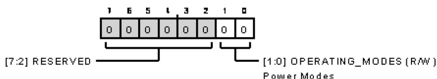
図 110. デバイス設定レジスタ
