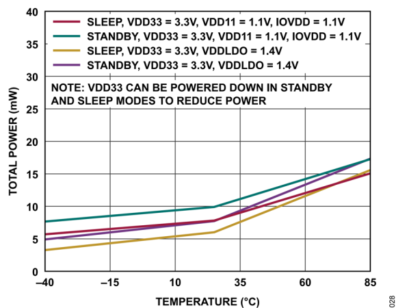
図 29. スリープ・モードおよびスタンバイ・モードでの総電力と温度の関係
