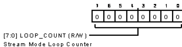
図 119. ストリーム・モード・レジスタ
