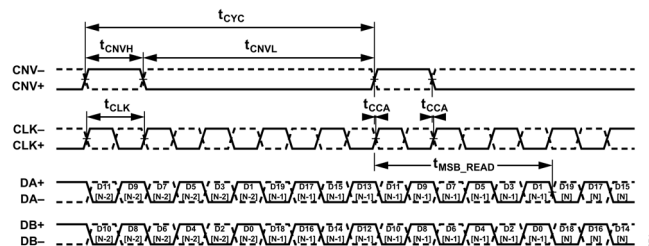
図 75. 連続変換タイミング、LVDS データ・インターフェース、デュアル・データ・レーン、セルフ・クロック・モード
