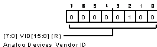
図 118. ベンダ ID ハイ・レジスタ
