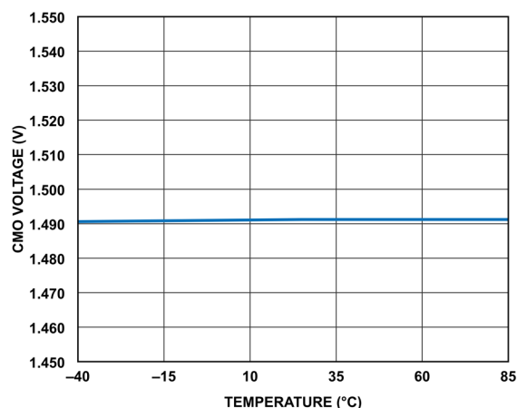
図 24. CMO 電圧と温度の関係
