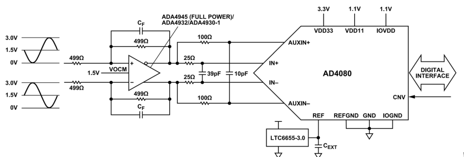
図 43. AD4080 の代表的なアプリケーション図、完全差動アンプ
