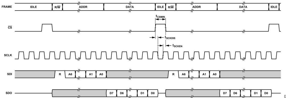
図 71. 設定 SPI タイミング、データ読み出しフレーム、連続 SCLK
