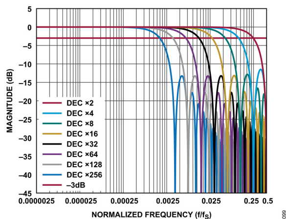
図 102. Sinc5 フィルタの応答、全デシメーション率
