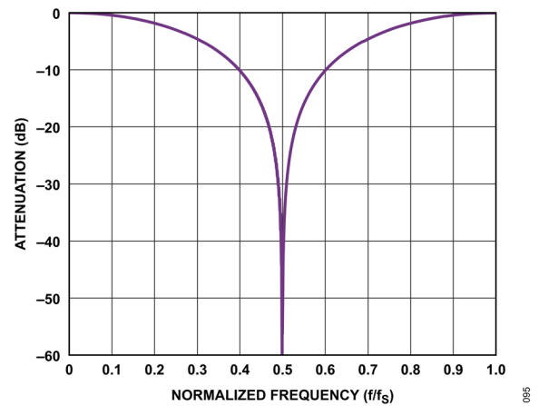
図 98. Sinc1 フィルタの応答、デシメーション率 2
