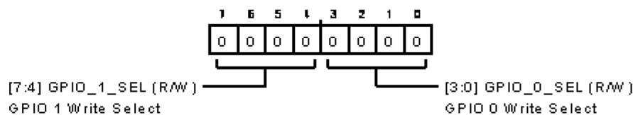
図 129. GPIO 設定 B レジスタ
