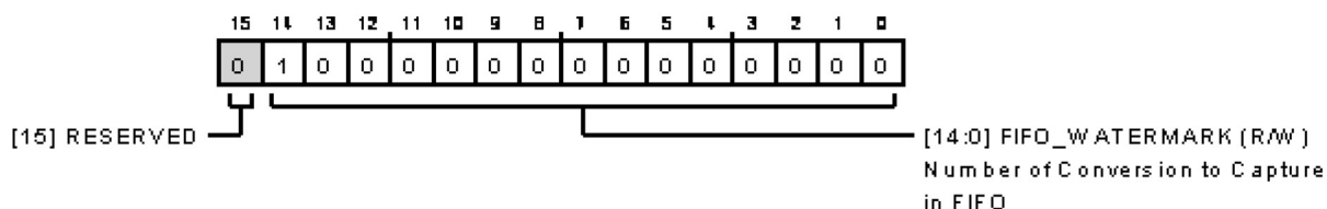
図 132. FIFO ウォーターマーク・レジスタ
