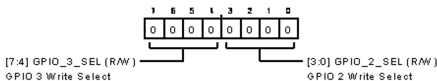
図 130. GPIO 設定 C レジスタ
