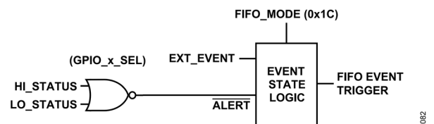
図 83. FIFO イベント検出ロジック
