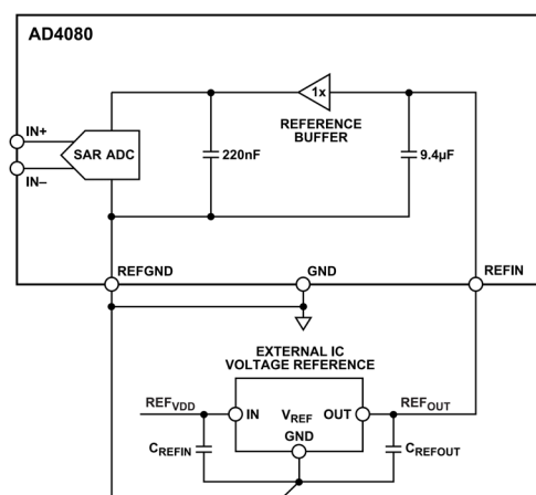
図 45. AD4080 一般的な外部リファレンス設計の機能図
