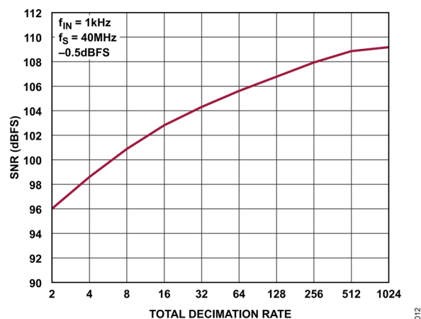
図 12. SNR と合計デシメーション率の関係、Sinc1
