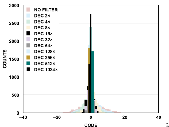
図 17. コードのヒストグラム、Sinc1、デシメーション率 2、デシメーション率 4～デシメーション率 1024
