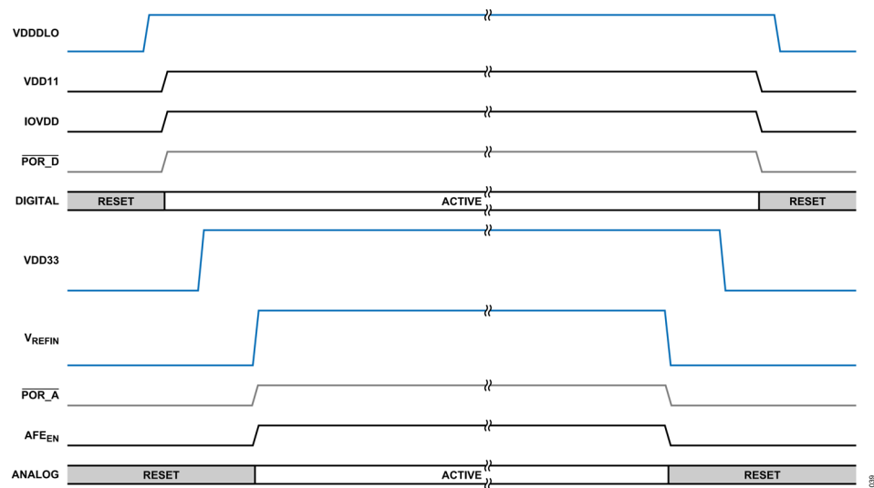
図 40. 電源シーケンス、内部生成化 IOVDD 、 VDD11
