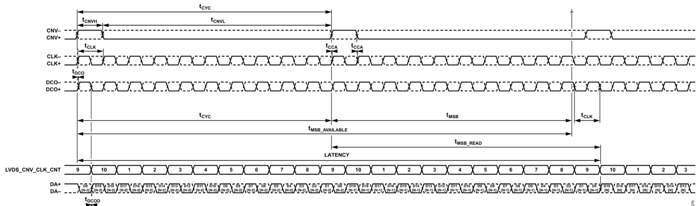
図 77. シングル・レーン LVDS、エコー・クロック・モード、LVDS_CNV_CLK_CNT 位置の例
