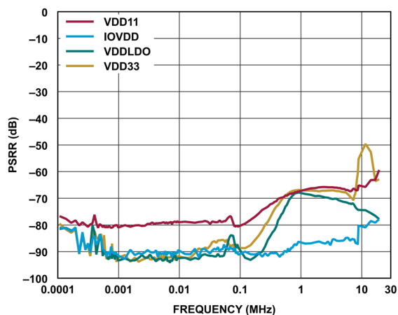
図 23. PSRR と周波数の関係
