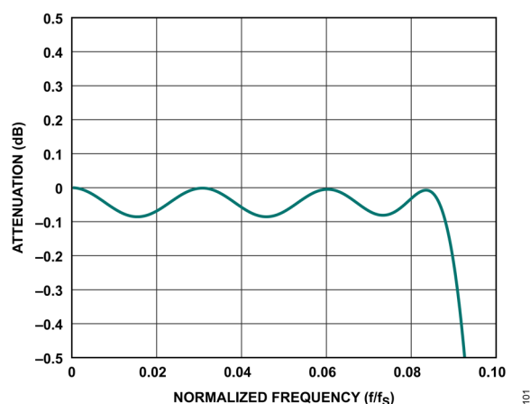
図 104. Sinc5 + 補償フィルタの応答、デシメーション率 2、通過帯域リップル
