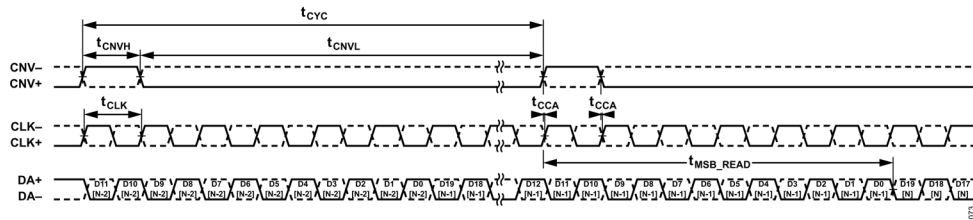
図 74. 連続変換タイミング、LVDS データ・インターフェース、シングル・データ・レーン、セルフ・クロック・モード
