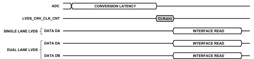
図 79. LVDS データ転送レイテンシ
