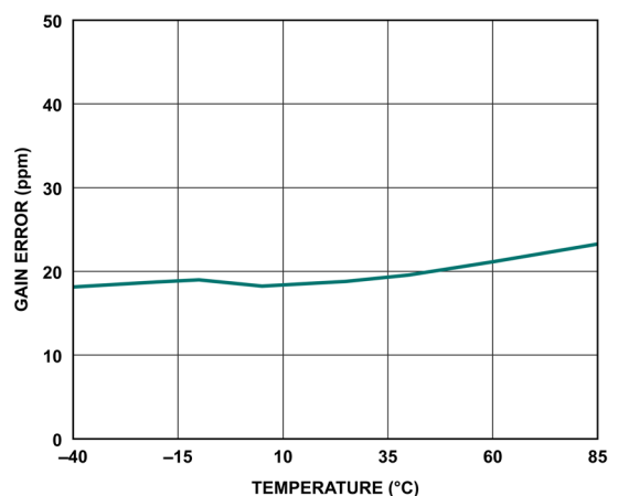
図 22. ゲイン誤差と温度の関係
