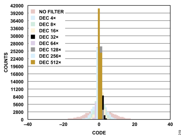
図 19. コードのヒストグラム、Sinc5 + 補償、デシメーション率 2、デシメーション率 4～デシメーション率 512
