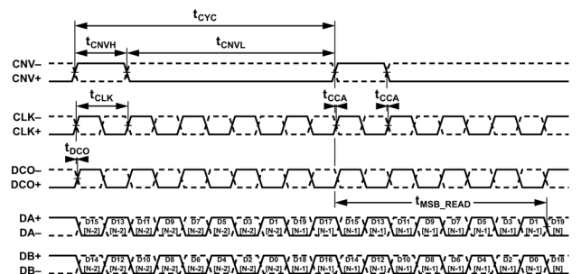
図 73. 連続変換タイミング、LVDS データ・インターフェース、デュアル・データ・レーン、エコ・クロック・モード
