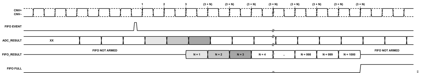
図 84. FIFO データ取り込みの例、WATERMARK = 1000
