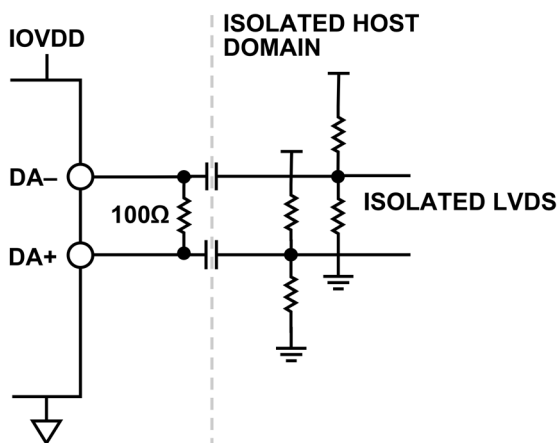
図 76. 絶縁型 LVDS
