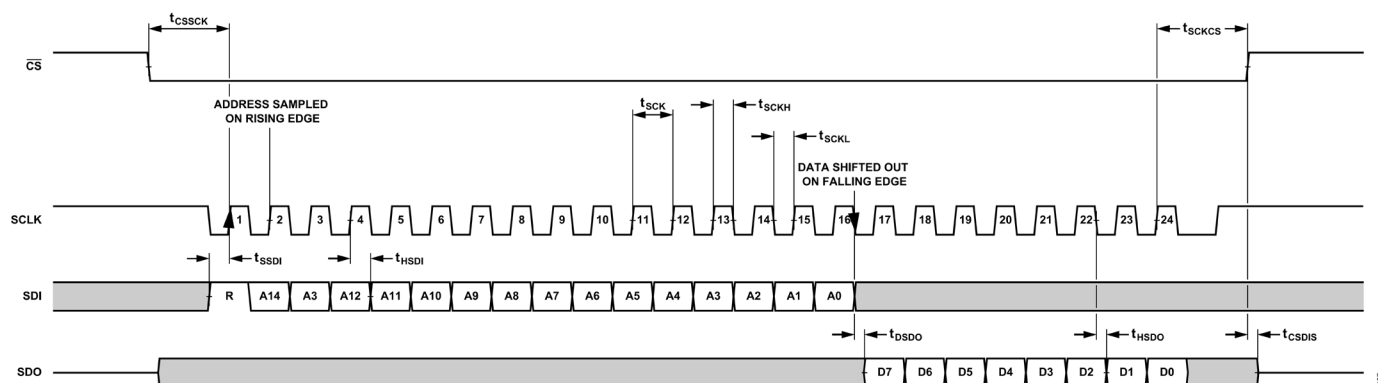
図 68. 設定 SPI タイミング、データ読出しフレーム、16 ビット命令モード（デフォルト）
