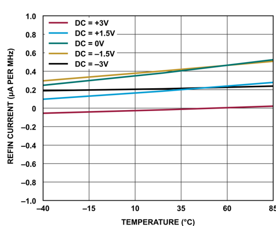
図 26. ダイナミック REFIN 電流と温度の関係
