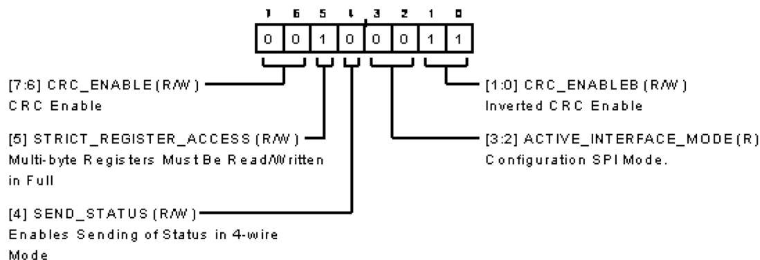
図 121. インターフェース設定 C レジスタ
