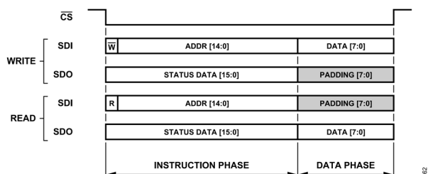
図 63. ロング命令モード、データ・ステータスをイネーブル済み、 CRC をディスエーブル済み
