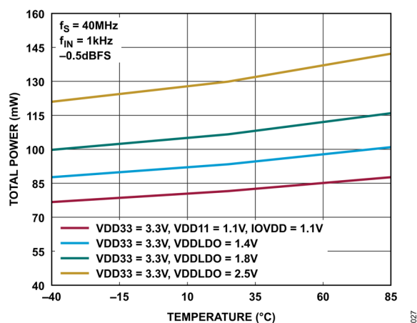
図 28. 40MSPS での総電力と温度の関係
