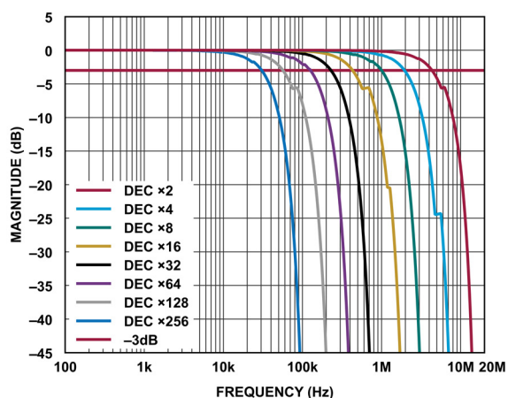
図 9. Sinc1 フィルタ応答、 f_s = 40\text{MHz} (DEC x はデシメーション率)
