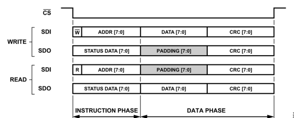
図 62. ショート命令モード、データ・ステータスを イネーブル済み、CRC をイネーブル済み
