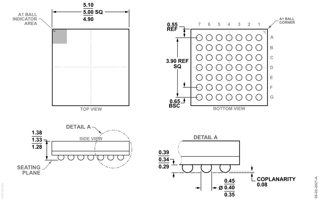
図 139. 49 ボール・チップ・スケール・パッケージ、ボール・グリッド・アレイ [CSP_BGA] (BC-49-8) 単位：mm
