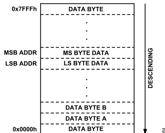
図 55. 汎用バイト幅メモリ、マルチバイト・レジスタの例
