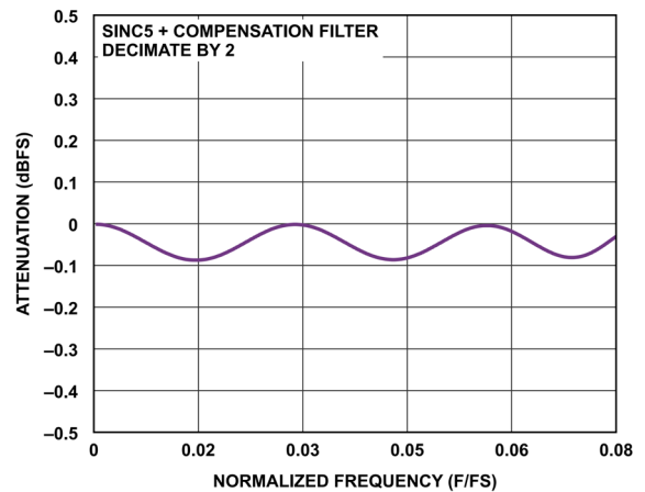
図 8. Sinc5 + 補償フィルタ、パス・バンドの平坦性
