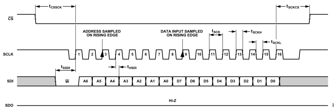
図 66. 設定 SPI タイミング、データ書き込みフレーム、8 ビット命令モード、シングル 8 ビット・レジスタ
