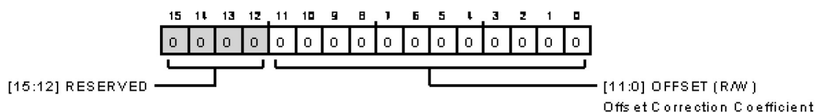
図 136. オフセット補正レジスタ
