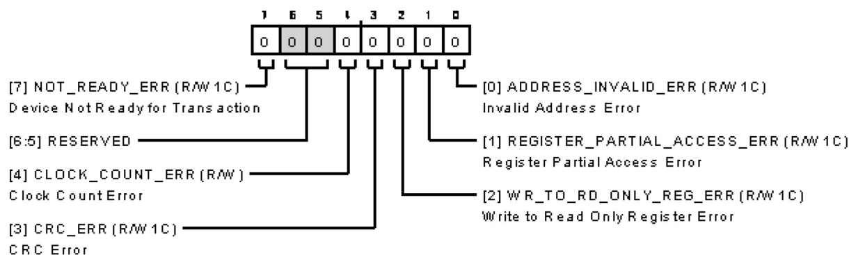
図 122. インターフェース・ステータス A レジスタ
