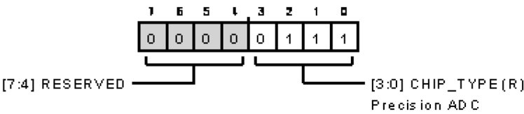
図 111. チップ・タイプ・レジスタ
