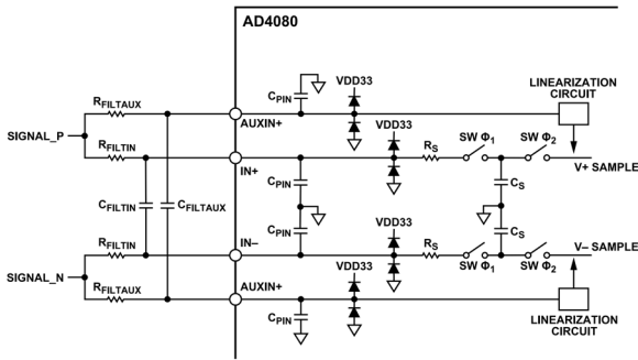
図 33. アナログ入力の等価回路モデル
