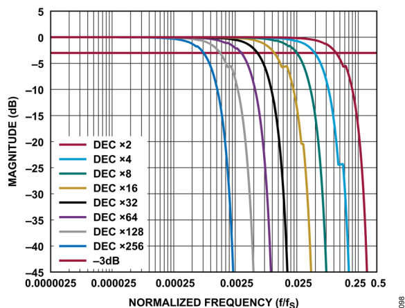
図 101. Sinc1 フィルタの応答、全デシメーション率
