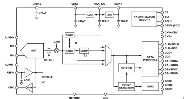
図 1. AD4080 の機能ブロック図
