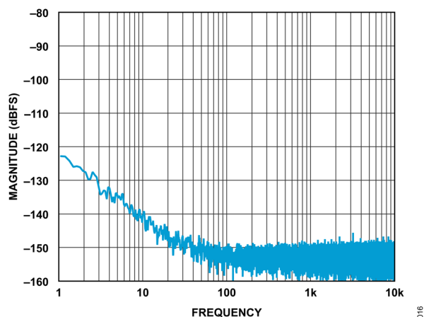
図 16. 低周波ノイズ、入力を短絡
