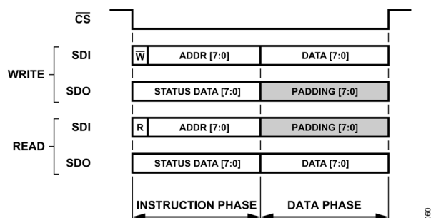
図 61. ショート命令モード、データ・ステータスを イネーブル済み、CRC をディスエーブル済み
