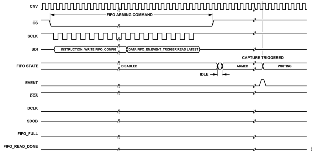
図 90. イベント・トリガされた取り込み、最新のウォーターマークの読出しの作動
