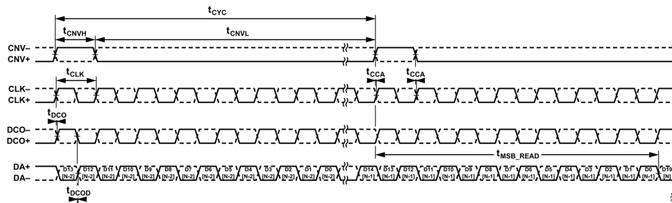
図 72. 連続変換タイミング、LVDS データ・インターフェース、シングル・データ・レーン、エコ・クロック・モード
