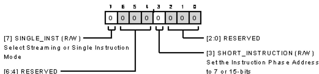
図 109. インターフェース設定 B の追加の設定値
