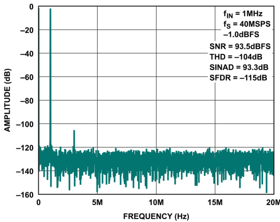
図 4. FFT 40MSPS、 f_{IN} = 1\text{MHz} 、 -1.0\text{dBFS}
