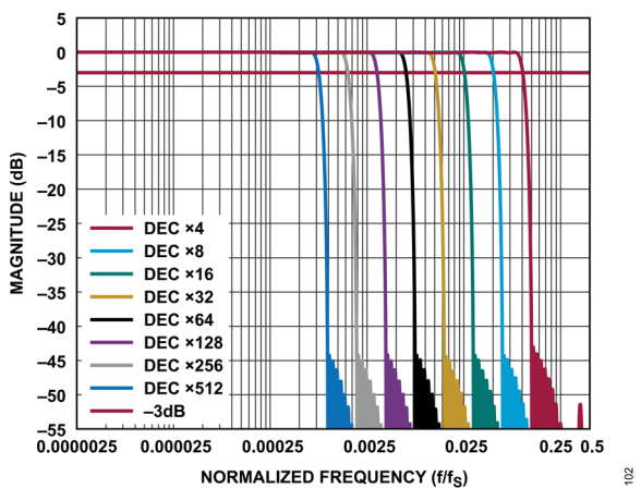
図 105. Sinc5 + 補償フィルタの応答
