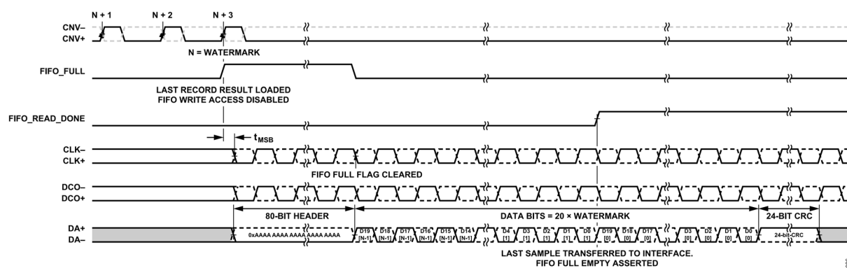
図 87. 非同期取り込み読み出しタイミング、データ FIFO をイネーブル済み、LVDS 設定
