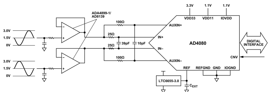
図 44. AD4080 の代表的なアプリケーション図、シングル・オペアンプ・ドライバ
