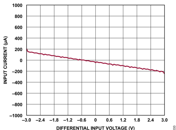
図 34. 代表的な入力電流と差動入力電圧の関係
