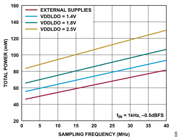
図 27. 総電力とサンプリング周波数の関係
