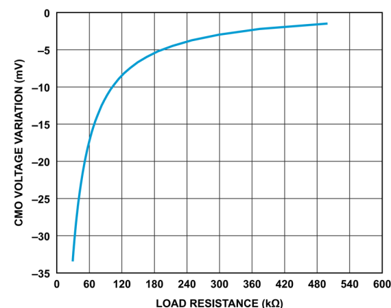
図 25. CMO 電圧変動と負荷抵抗の関係
