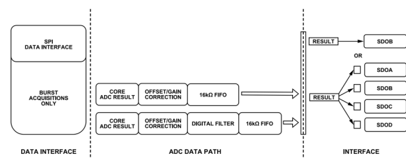
図 50. SPI データ・インターフェースのデータ経路のオプション
