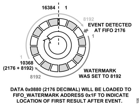
図 91. イベント取り込みモードのすべての FIFO の読み出しモードの例、FIFO フィリング
