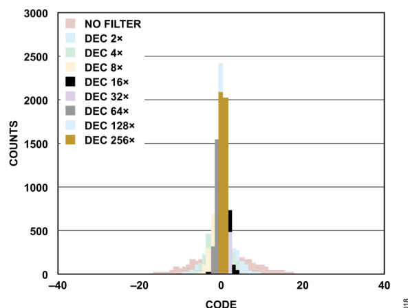
図 18. コードのヒストグラム、Sinc5、デシメーション率 2、デシメーション率 4～デシメーション率
