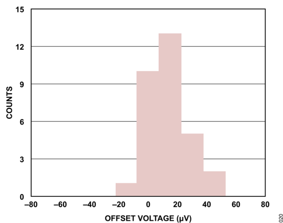
図 20. オffset 電圧のヒストグラム
