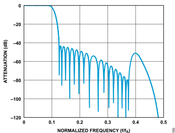
図 103. Sinc5 + 補償フィルタの応答、デシメーション率 2
