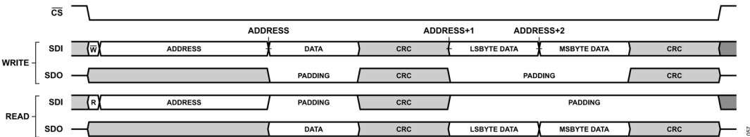
図 58. CRC をイネーブルにしたストリーミング・モードの設定、ADDR_ASCENSION = 1
