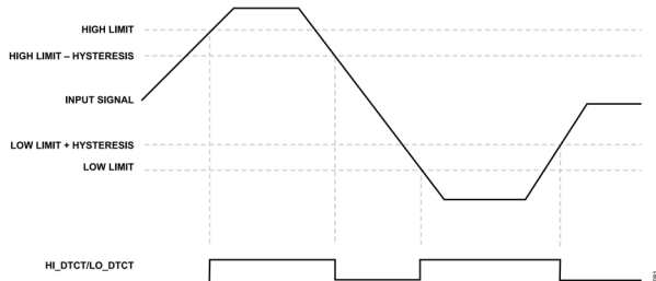
図 82. 閾値検出レベル
