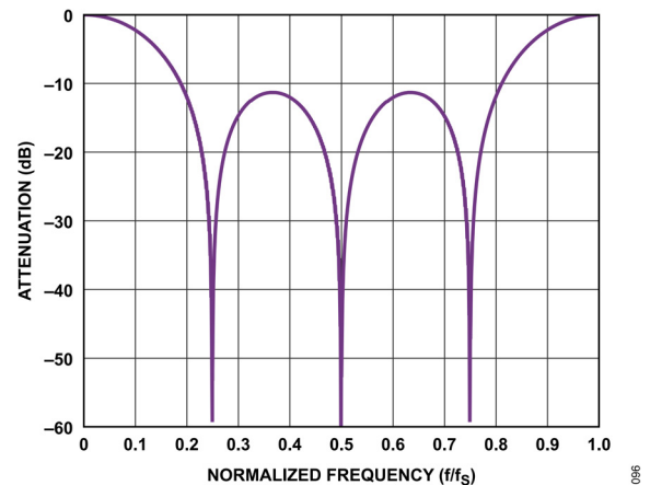
図 99. Sinc1 フィルタの応答、デシメーション率 4
