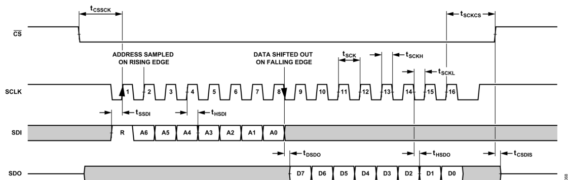
図 69. 設定 SPI タイミング、データ読出しフレーム、8 ビット命令モード
