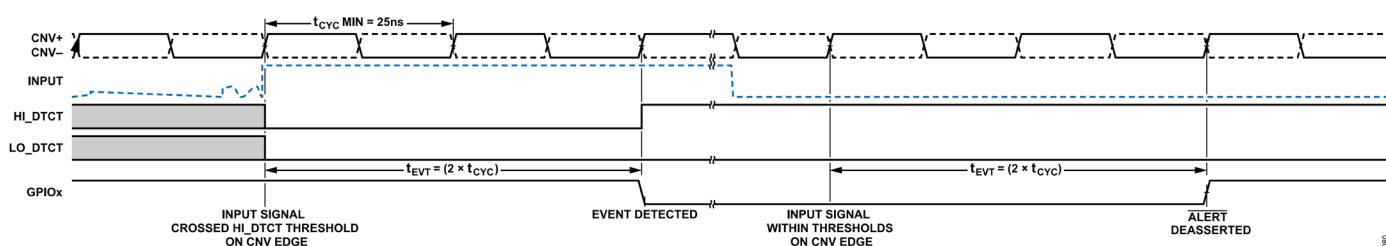
図 81. イベント検出のタイミング
