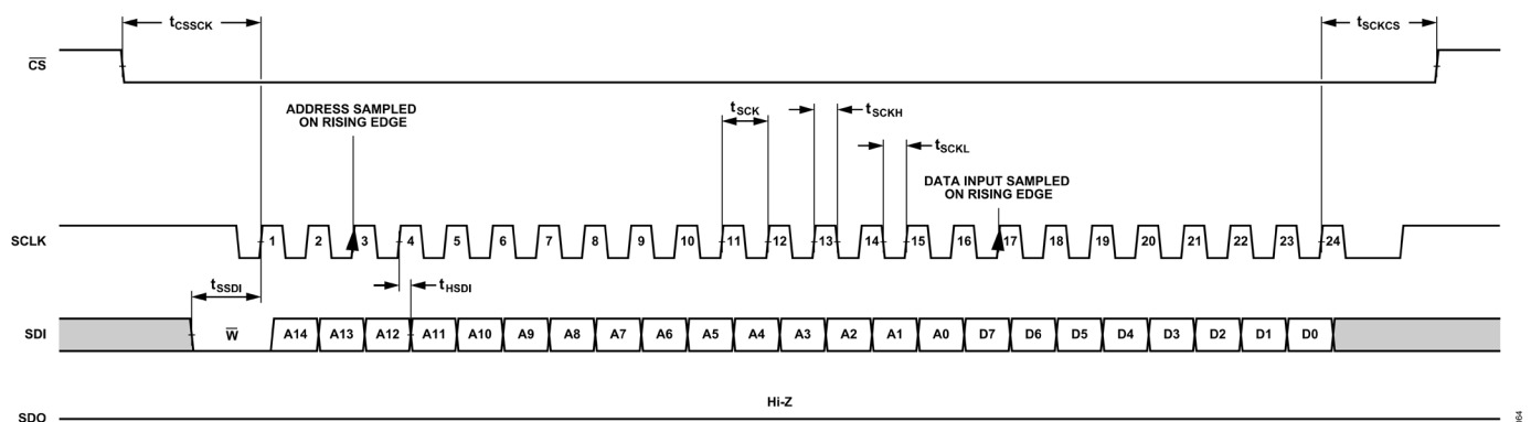
図 65. 設定 SPI タイミング、データ書き込みフレーム、16 ビット命令モード（デフォルト）
