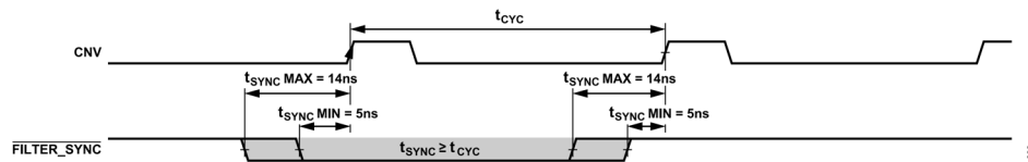
図 96. フィルタ・リセットのタイミング
