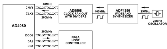
図 47. デュアル・レーン、LVDS データ・インターフェースのクロッキングの例
