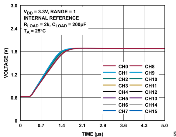
図 26. セトリング時間
