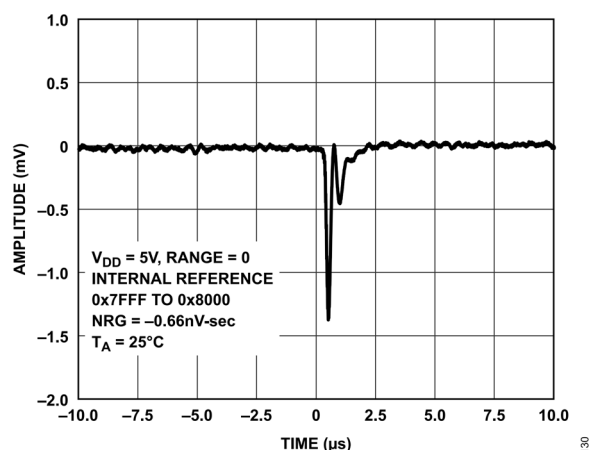
図 30. デジタル/アナログ・グリッチ・インパルス、5V
