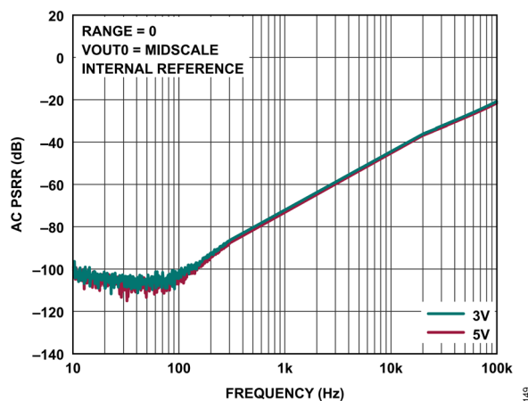
図 49. V OUT AC PSRR と周波数の関係
