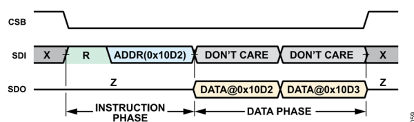
図 64. 昇順アドレス指定によるマルチバイト読み出し
