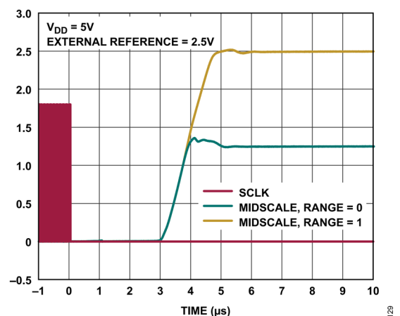
図 29. パワーダウン終了時のミッドスケール出力
