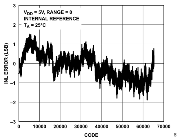
図 6. INL 誤差とコードの関係
