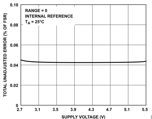
図 14. TUE と電源電圧の関係
