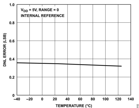
図 10. DNL 誤差と温度の関係
