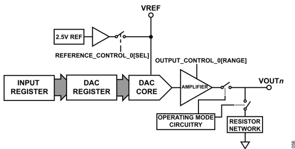
図 61. DAC チャンネルのブロック図
