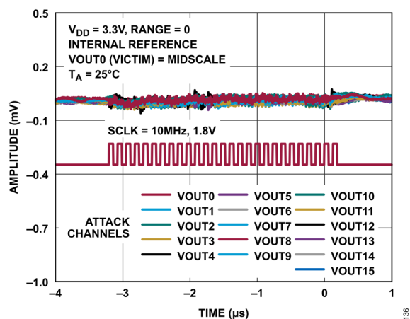
図 36. デジタル・フィードスルー
