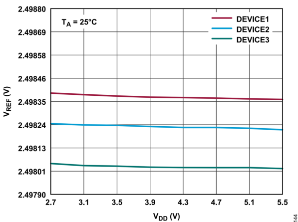
図 44. VREF と VDD の関係
