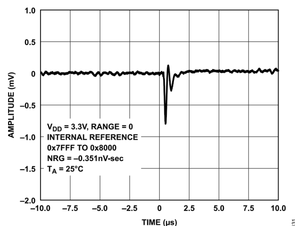
図 31. デジタル/アナログ・グリッチ・インパルス、3.3V
