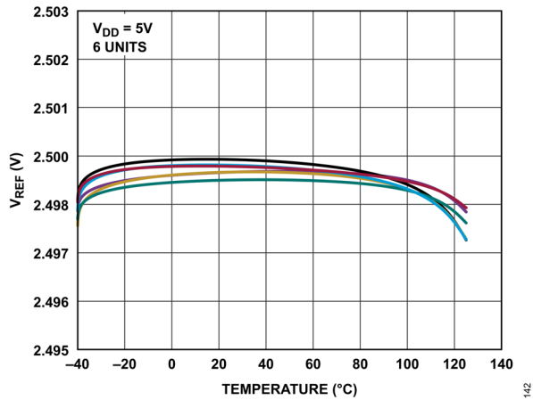
図 42. VREF と温度の関係
