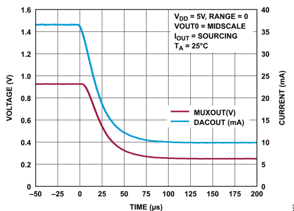
図 56. MUX_OUT と出力電流トランジェントの関係、立下がり
