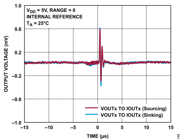
図 48. MUX_OUT から VOUTx へのグリッチ
