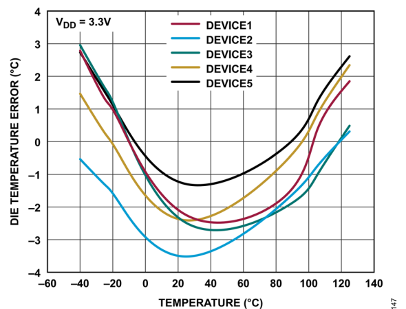
図 47. MUX_OUT 誤差と内部ダイ温度の関係
