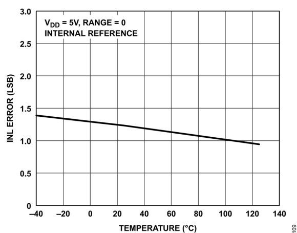
図 9. INL 誤差と温度の関係
