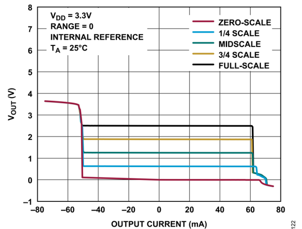
図 22. VDD = 3.3V でのソース能力とシンク能力
