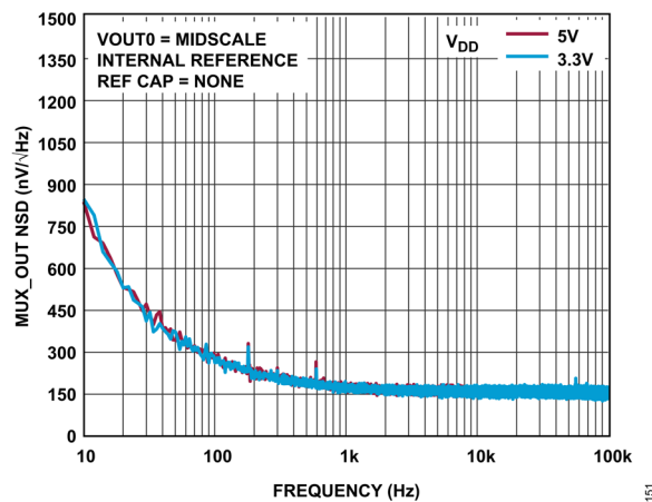
図 51. MUX_OUT の NSD
