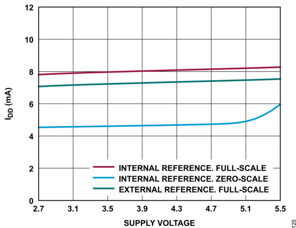
図 25. I_{DD} と電源電圧の関係
