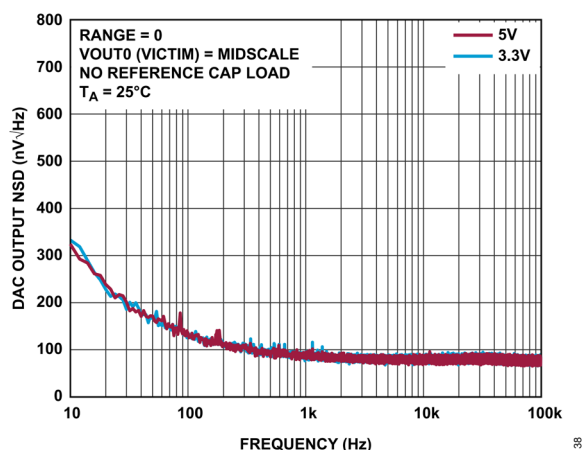
図 38. ノイズ・スペクトル密度 (NSD)
