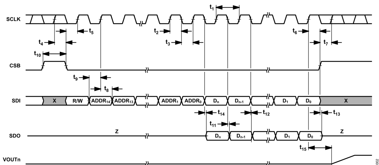
図 2. シリアル読出し動作と書き込み動作
