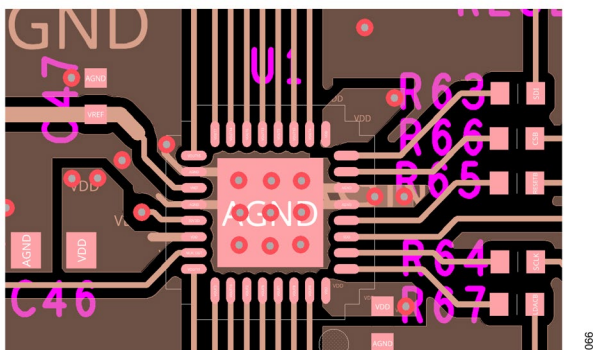
図 71. 評価用ボードのレイアウト
