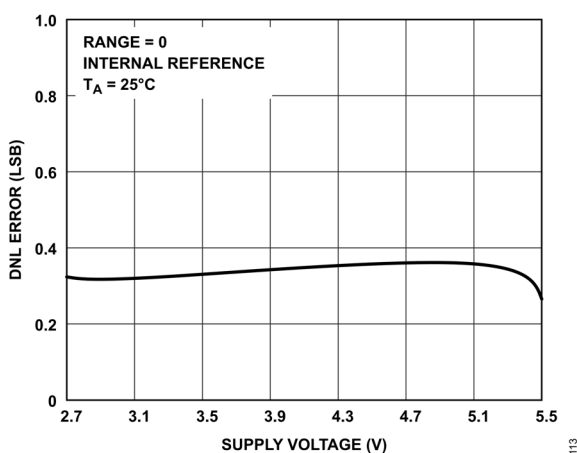
図 13. DNL 誤差と電源電圧の関係
