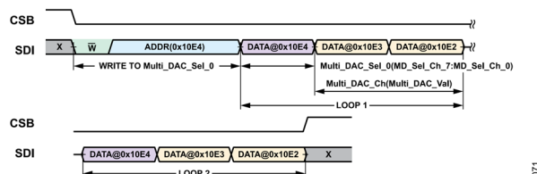
図 76. オプション 4 の例：MULTI_DAC_CHn レジスタへの書込み・ストリーム・モード（ループ）、降順アドレス
