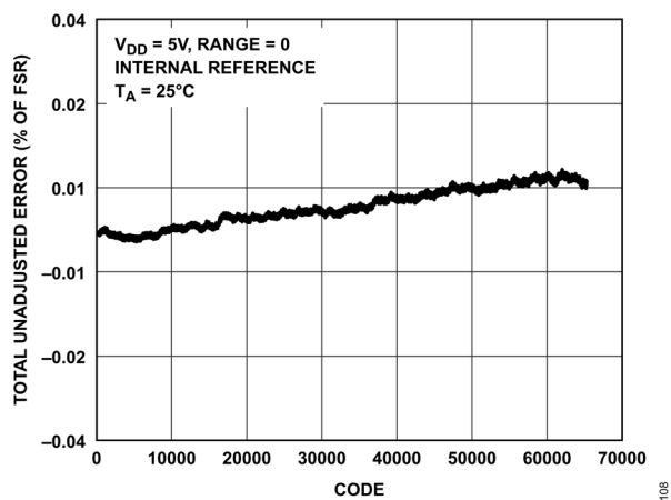
図 8. 総合未調整誤差 (TUE) とコードの関係
