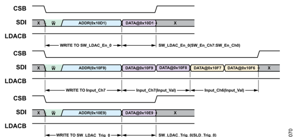
図 75. オプション 3 の例：INPUT_CH7 と INPUT_CH6 レジスタへの書き込み - ソフトウェア LDAC、ストリーム・モード、降順アドレス
