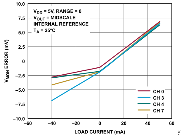
図 46. MUX_OUT 誤差と出力電圧の関係、5V
