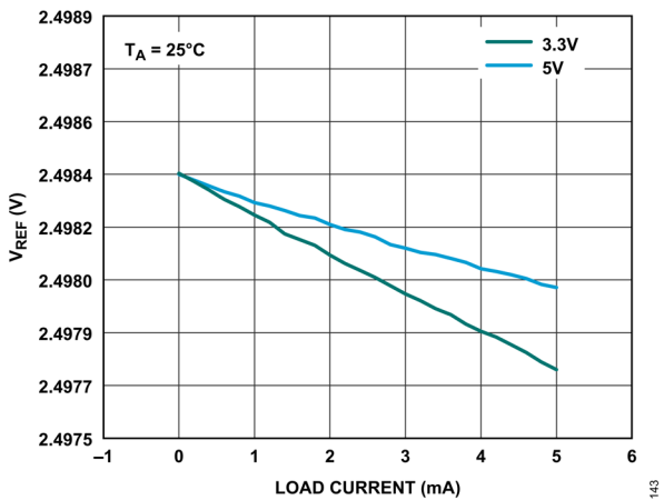
図 43. VREF と負荷電流の関係
