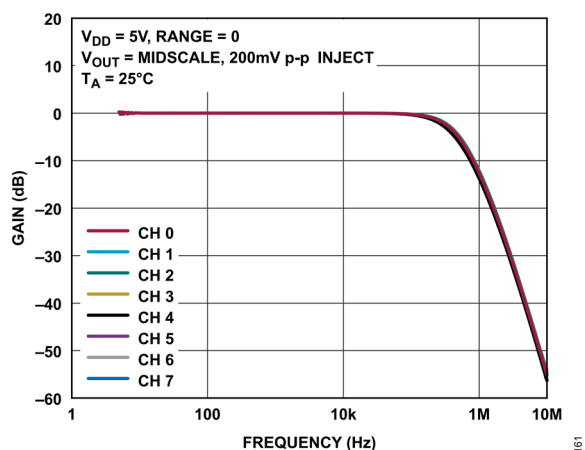
図 60. MUX_OUT 電圧モニタリングの周波数応答
