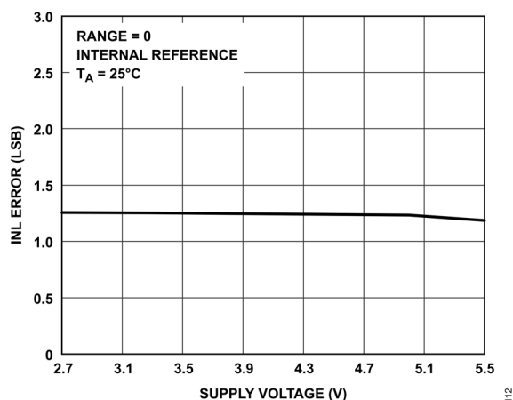
図 12. INL 誤差と電源電圧の関係
