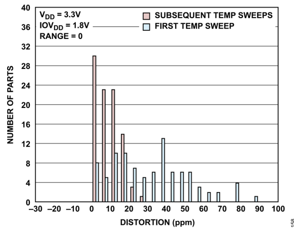
図 58. リファレンスの熱ヒステリシス
