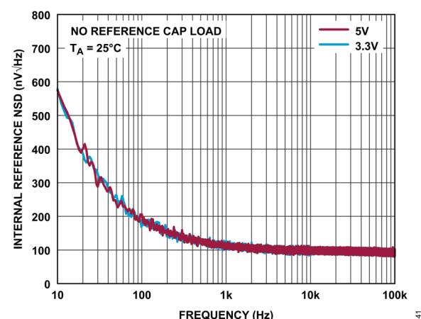
図 41. 内部リファレンスの NSD と周波数の関係
