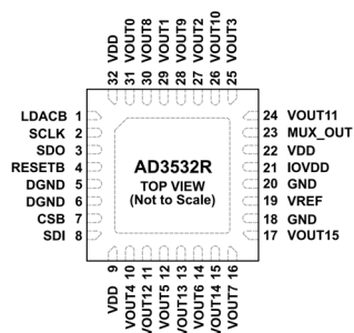
図 5. LFCSP のピン配置
