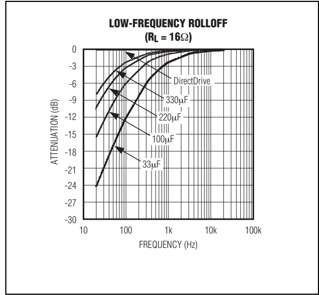
図3. 標準的な出力コンデンサ値に対する低周波での減衰度
