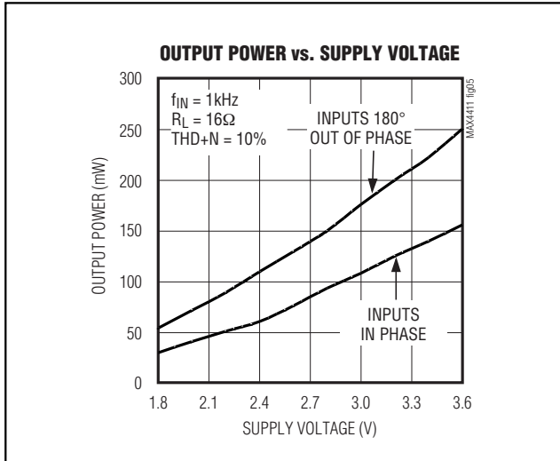
図5. 出力電力対入力電源電圧(入力が同相/逆相の場合)
