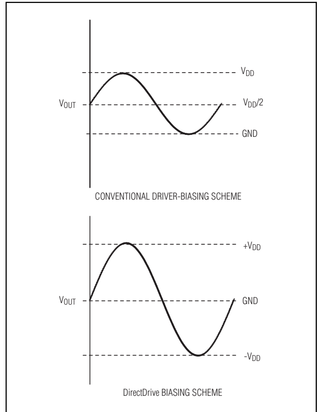
図1. 従来のドライバの出力波形対MAX4411の出力波形
