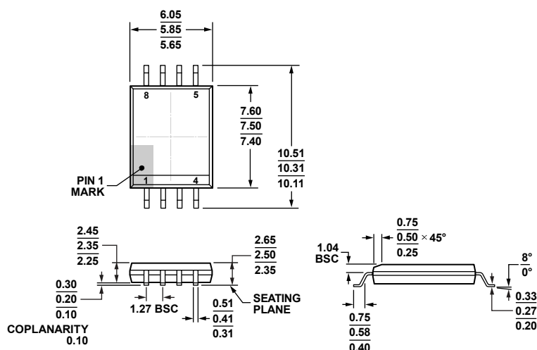
図 28. 16 ピン、標準 SOP (スモール・アウトライン・パッケージ) [SOIC_W] ワイド・ボディ (RW-16) 寸法単位: mm (括弧内はインチ)
