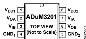
図 5.ADuM3201 のピン配置
