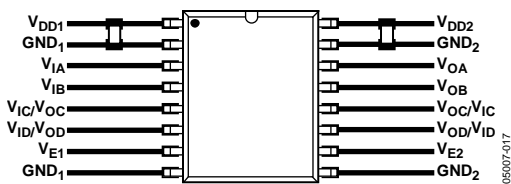
図 17. プリント回路ボードの推奨レイアウト
