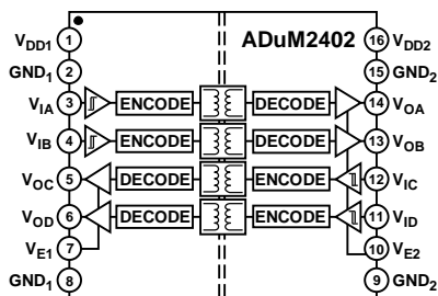
図 3. ADuM2402
