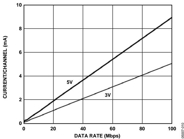
図 10. 5 V および 3 V 動作でのデータレート対チャンネルあたりの出力電源電流(15 pF 出力無負荷)
