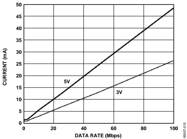
図 15. 5 V および 3 V 動作でのデータレート対 ADuM2402 の V_{DD1} または V_{DD2} 電源電流
