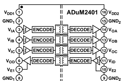
図 2. ADuM2401
