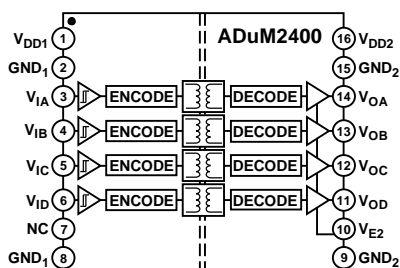
図 1. ADuM2400
