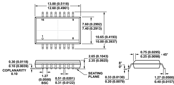
図 24.16 ピン標準スモール・アウトライン・パッケージ[SOIC_W] ワイドボディ(RW-16) 寸法: mm (インチ)
