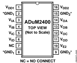
図 5.ADuM2400 のピン配置
