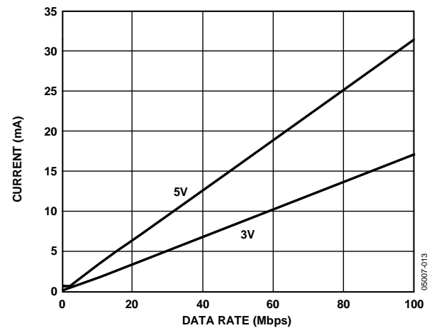
図 13. 5 V および 3 V 動作でのデータレート対 ADuM2401 V DD1 電源電流
