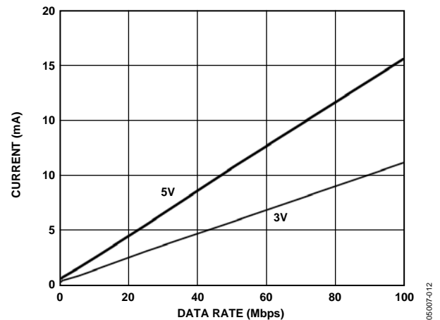
図 12. 5 V および 3 V 動作でのデータレート対 ADuM2400 V DD2 電源電流(Typ)
