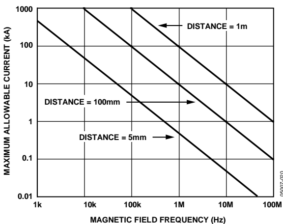
図 20.様々な電流値と ADuM240x までの距離に対する最大許容電流
