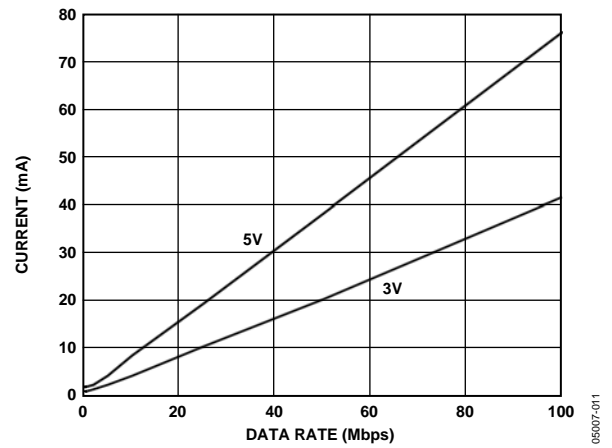
図 11. 5 V および 3 V 動作でのデータレート対 ADuM2400 V DD1 電源電流
