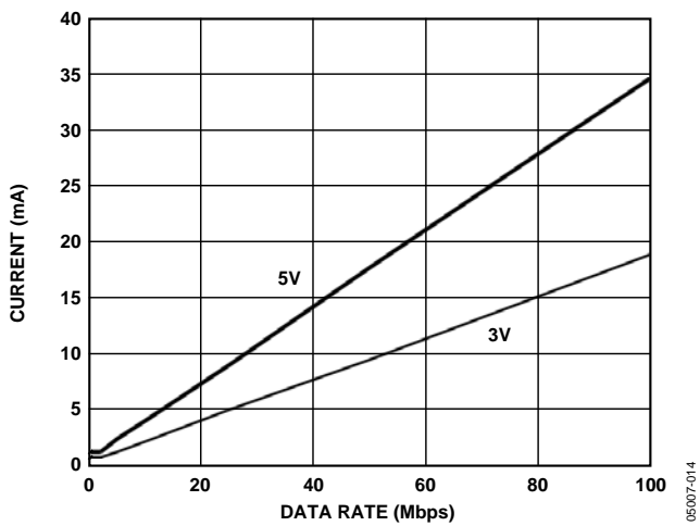
図 14. 5 V および 3 V 動作でのデータレート対 ADuM2401 V_{DD2} 電源電流(Typ)
