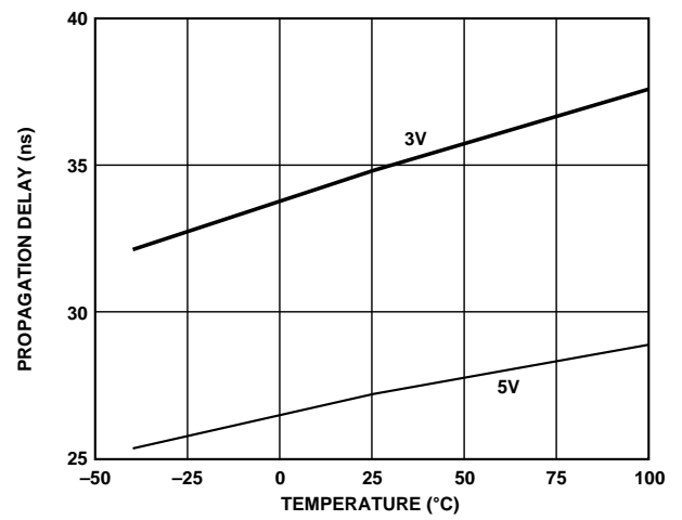
図 16. 伝搬遅延の温度特性、C グレード
