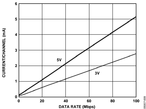
図 9. 5 V および 3 V 動作でのデータレート対チャンネルあたりの出力電源電流(出力無負荷)
