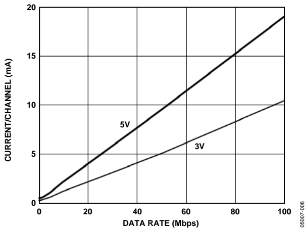
図 8. 5 V および 3 V 動作でのデータレート対チャンネルあたりの入力電源電流((出力無負荷)
