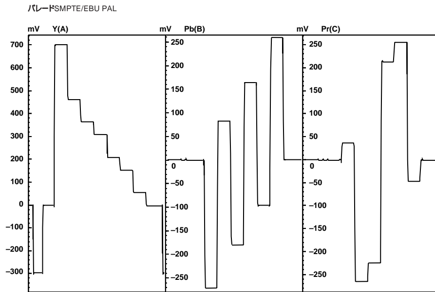
図99 . PAL YUV パレード・プロット
