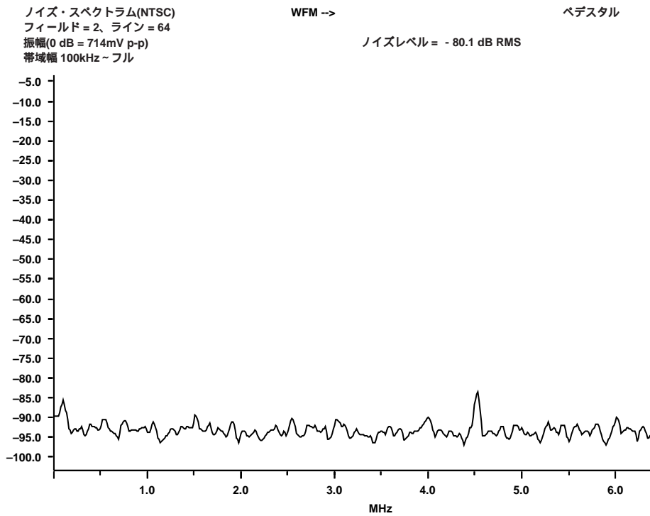
図97 . NTSC S/N比ベデスタル測定
