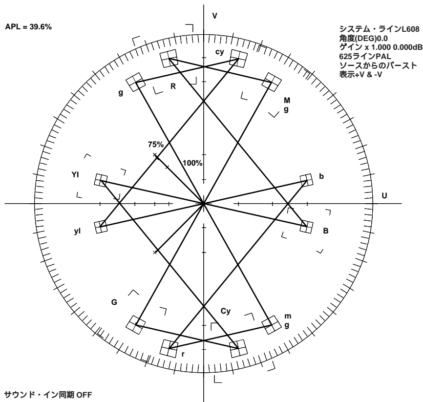
図91 . PALベクトル・プロット
