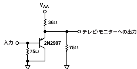
図84 . 推奨出力D/ACバッファ
