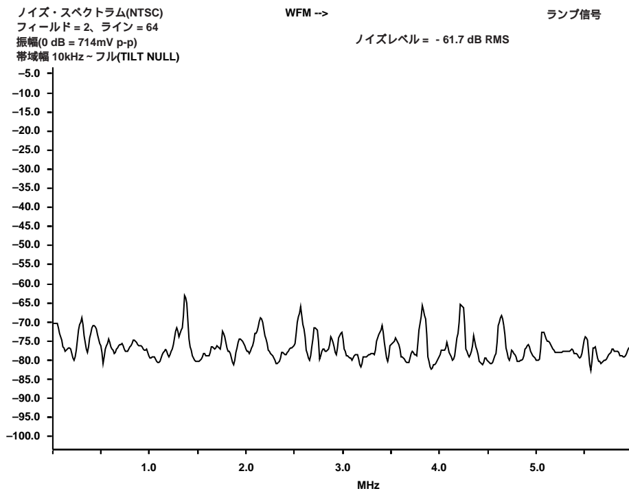
図98 . NTSC S/N比ランプ測定
