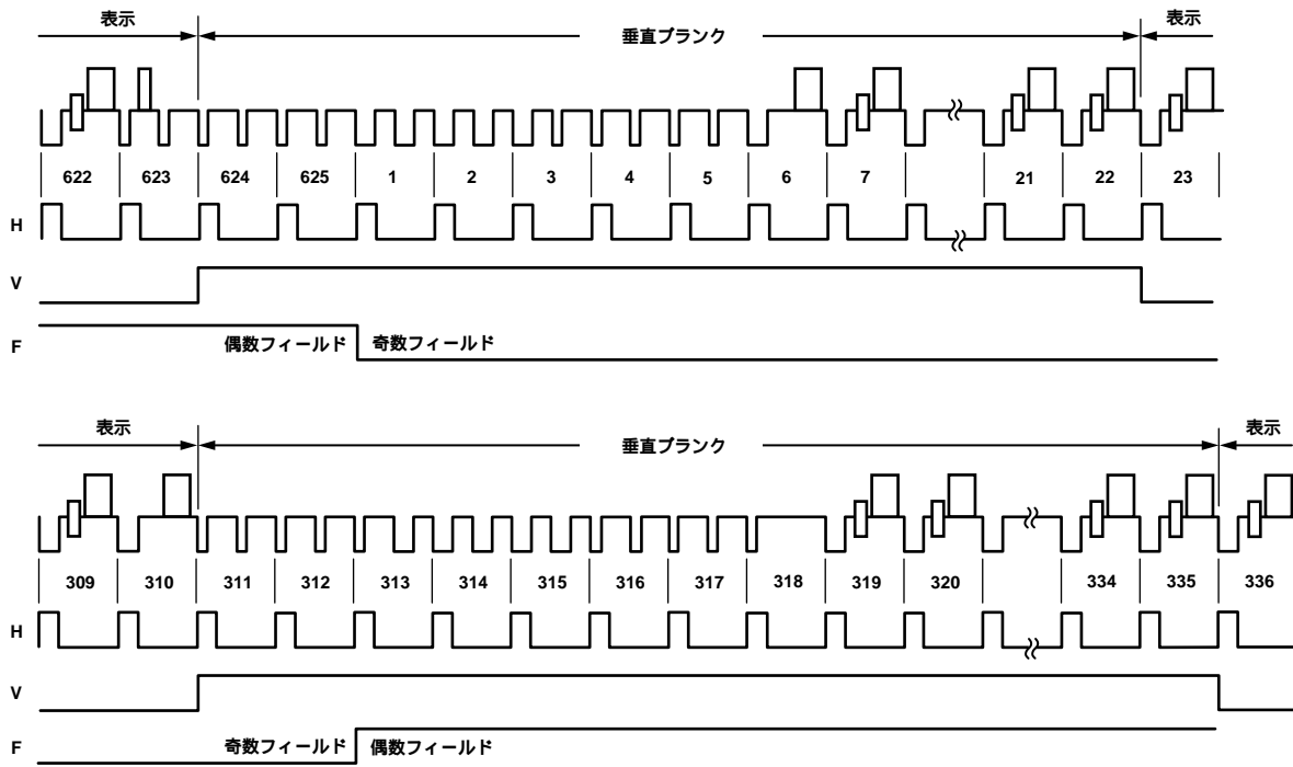
図22. タイミング・モード0(PALマスター・モード)
