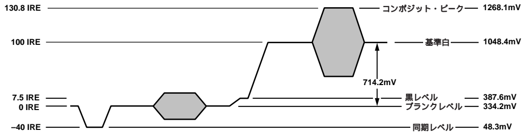
図61 . NTSCコンボジット・ビデオ・レベル
