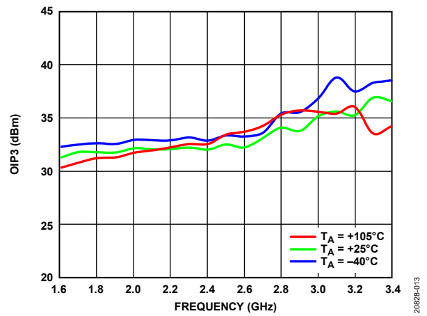
図 13. OIP3 の周波数特性 (出力トーン電力: 8dBm)
