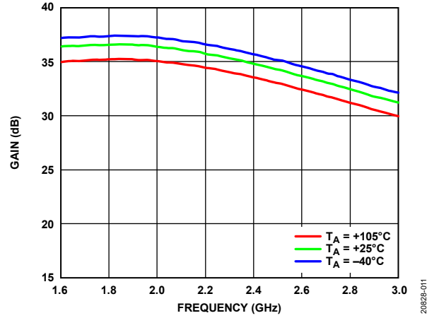
図 11. 様々な温度でのゲインの周波数特性 (1.6GHz~3.0GHz)
