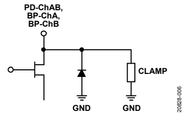
図 6. PD-ChAB および BP-Chx のインターフェース回路図
