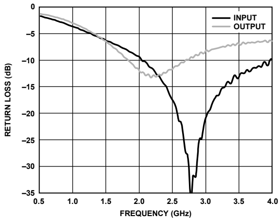
図 17. リターン・ロスの周波数特性
