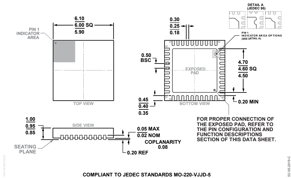
図 29. 40 ピン・リードフレーム・チップスケール・パッケージ [LFCSP] 6mm × 6mm ボディ、0.95mm パッケージ高 (CP-40-15) 寸法：mm
