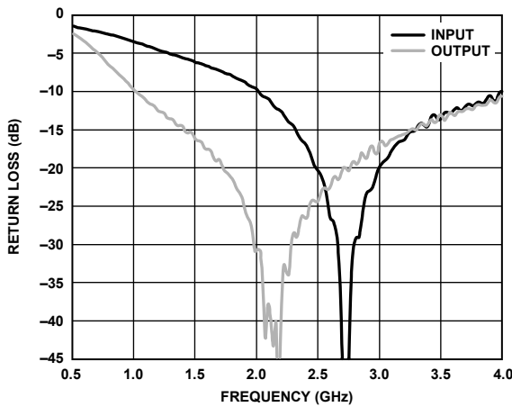
図 9. リターン・ロスの周波数特性
