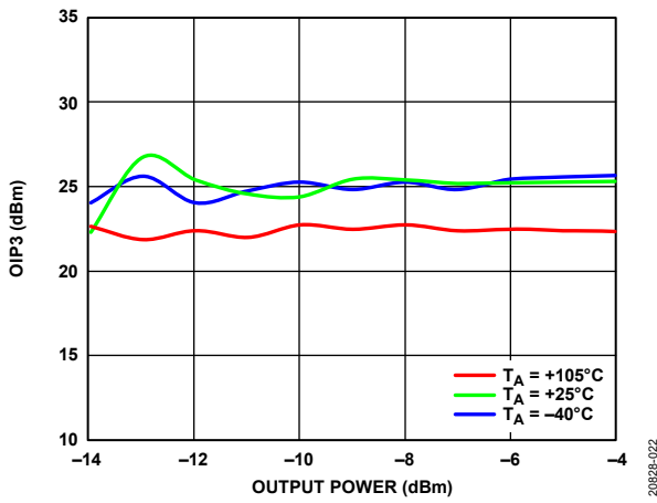
図 22. OIP3 と出力電力の関係 (2.3GHz)
