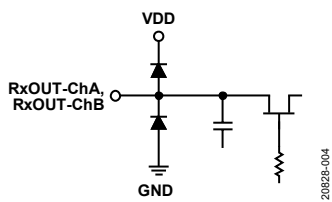
図 4. RxOUT-Chx のインターフェース回路図
