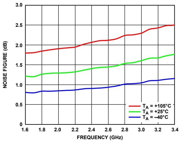
図 18. 様々な温度でのノイズ指数の周波数特性
