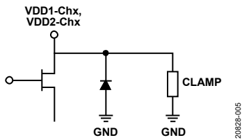
図 5. VDD1-Chx および VDD2-Chx のインターフェース回路図
