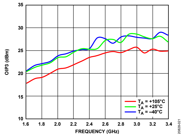
図 21. OIP3 の周波数特性 (出力トーン電力: 8dBm)
