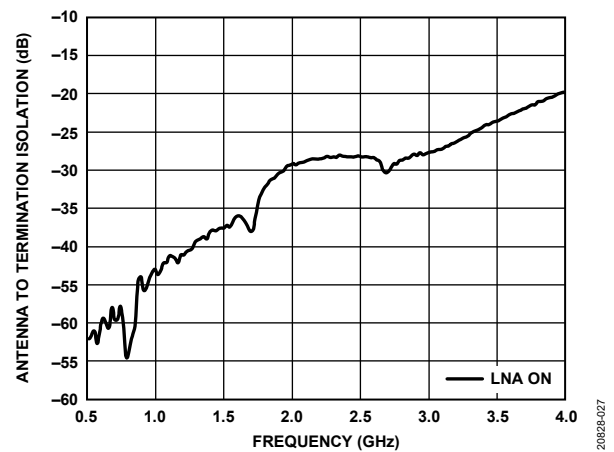
図 27. アンテナと終端間のアイソレーションの周波数特性 (LNA オン)
