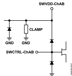
図 7. SWCTRL-ChAB および SWVDD-ChAB のインターフェース回路図
