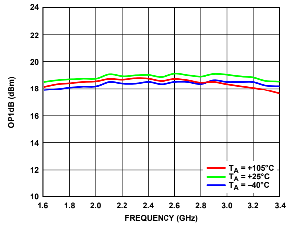
図 15. 様々な温度での OP1dB の周波数特性
