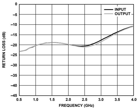
図 25. リターン・ロスの周波数特性
