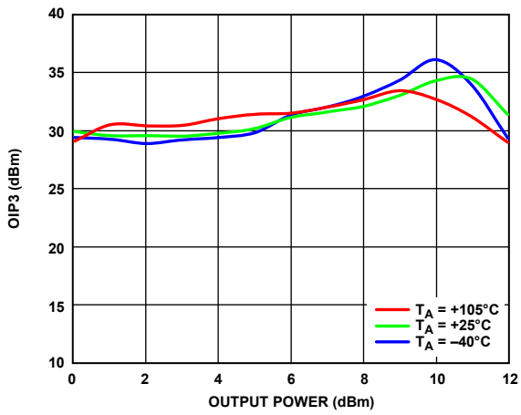
図 14. OIP3 と出力電力の関係 (2.3GHz)
