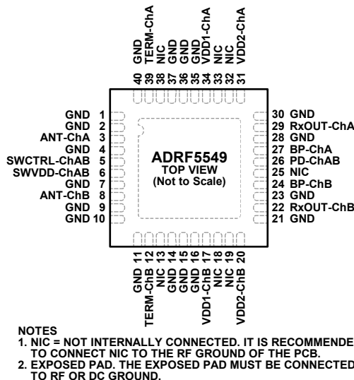
図 2. ピン配置
