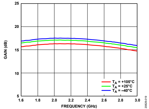
図 19. 様々な温度でのゲインの周波数特性 (1.6GHz~3.0GHz)
