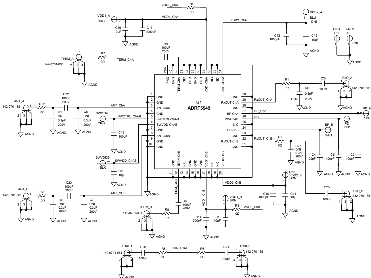
図 28. 代表的なアプリケーション回路
