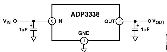
図2. 代表的なアプリケーション回路
