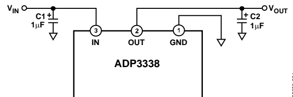
図20. 代表的なアプリケーション回路
