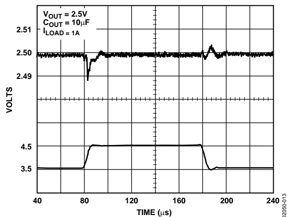
図13. ライン過渡応答
