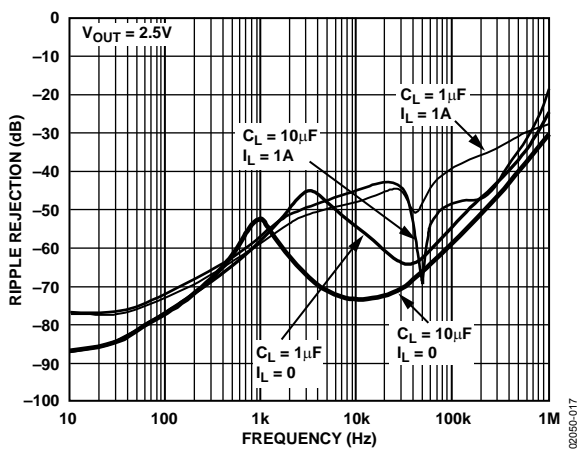
図17.電源リップル除去比
