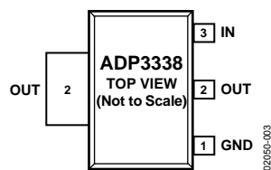
図3. ピン配置
