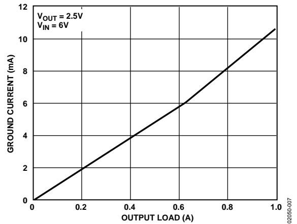
図7.負荷電流対グラウンド電流
