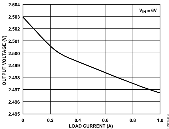
図5.負荷電流対出力電圧
