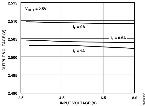
図4.入力電圧対ライン・レギュレーション出力電圧
