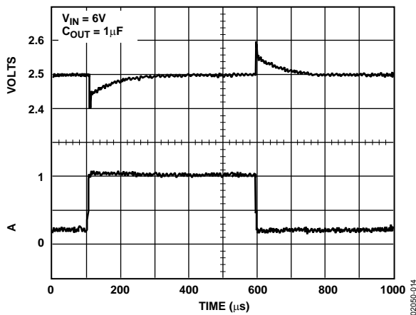
図14. 負荷過渡応答
