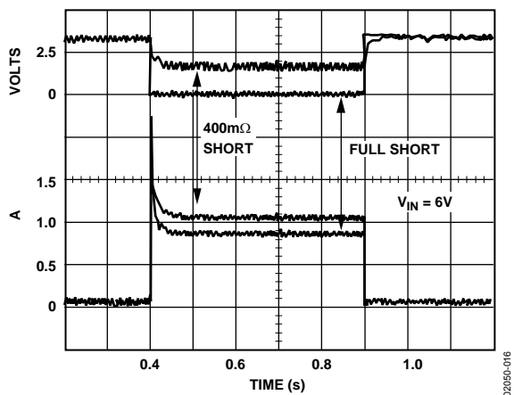
図16.短絡電流
