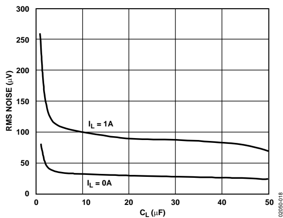
図18. C_L 対 RMS ノイズ
