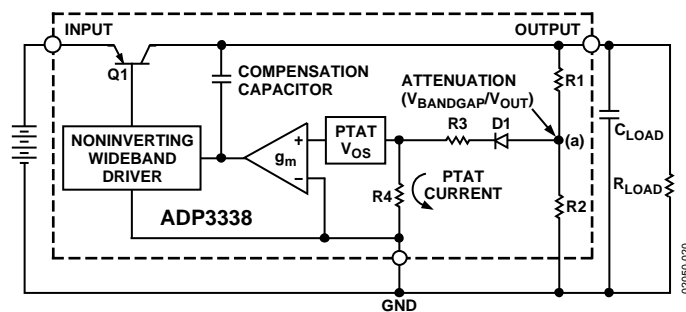
図21. 機能ブロック図
