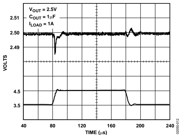
図12. ライン過渡応答
