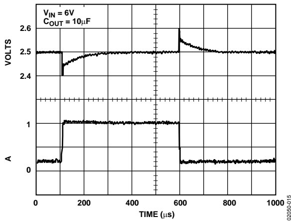
図15. 負荷過渡応答
