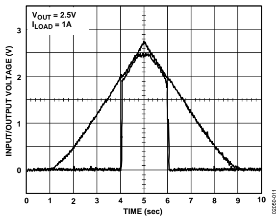
図11. パワーアップ/パワーダウン
