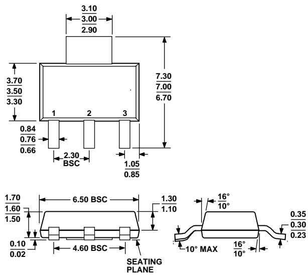
図23.3 ピン・スモール・アウトライン・トランジスタ・パッケージ[SOT-223] (KC-3) 寸法: mm
