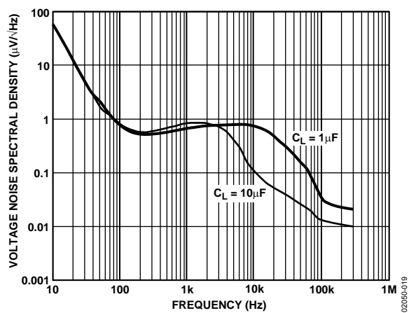
図19.出力ノイズ密度 (10 Hz~100 kHz)
