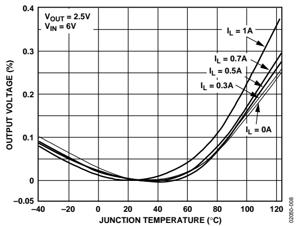
図8.ジャンクション温度対出力電圧変動%
