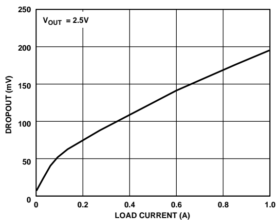
図10. 負荷電流対ドロップアウト電圧
