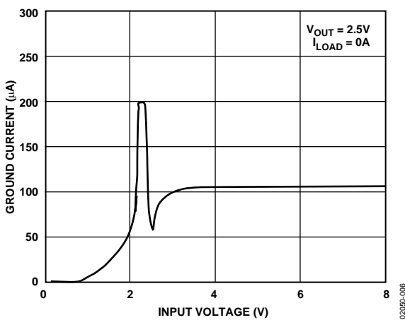
図6.電源電圧対グラウンド電流
