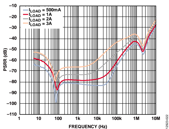
図 22. 各種入力電圧での電源電圧変動除去比 (PSRR) の周波数特性、 V_{OUT} = 1.3 \text{ V} 、 V_{IN} = 1.7 \text{ V}
