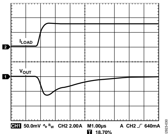
図 31. 出力過渡応答、C OUT = 10 μF
