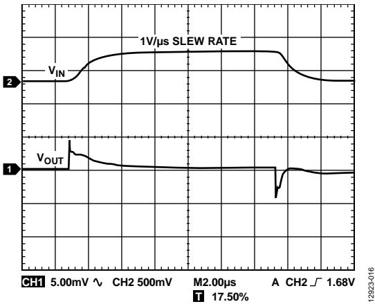
図 16. ライン過渡応答、負荷電流 = 3 A、 V_{IN} = 1.5\text{ V} \sim 1.98\text{ V} のステップ、 V_{OUT} = 1.3\text{ V}
