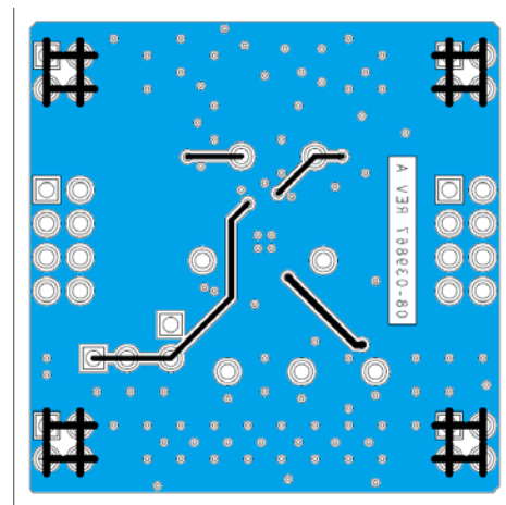
図 48. 代表値なボード・レイアウト、底面
