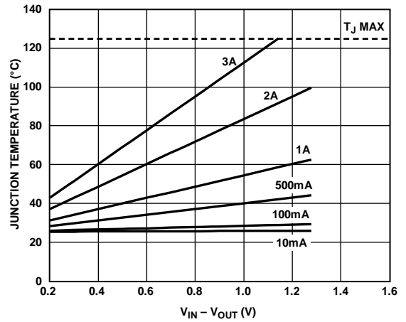
図 41. 500 mm 2 の PCB 銅箔、T B = 25°C
