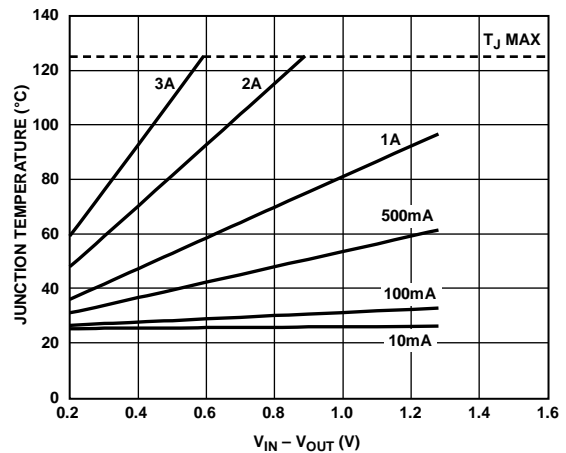
図 35. 6400 mm 2 の PCB 銅箔、 T_A = 25^\circ\text{C}
