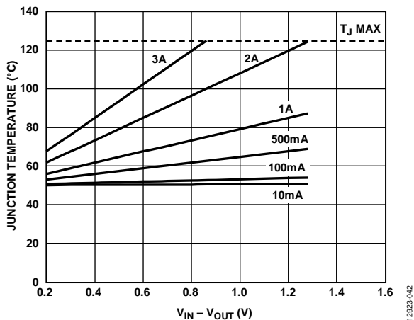
図 44. 1000 mm 2 の PCB 銅箔、 T_B = 50^\circ\text{C} 、LFCSP パッケージ
