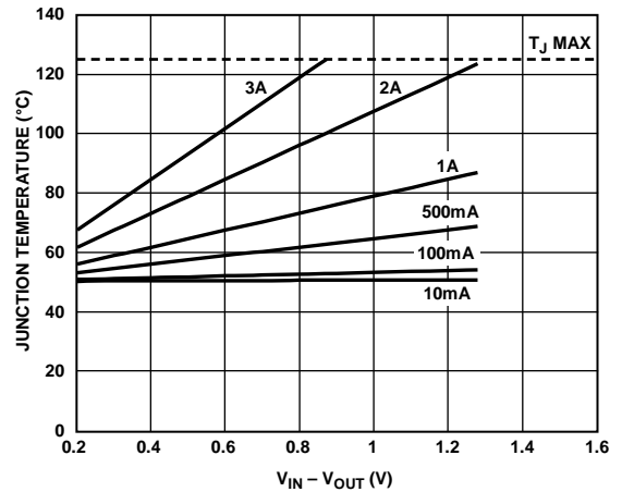
図 42. 500 mm 2 の PCB 銅箔、T B = 50°C
