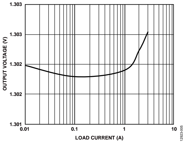
図 5. 負荷電流対出力電圧 ( V_{OUT} )
