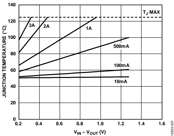
図 39. 500 mm 2 の PCB 銅箔、T A = 50°C
