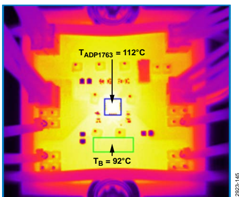
図 45. ADP1763 評価用ボードの熱画像 ( I_{LOAD} = 3 \text{ A} 、 V_{IN} = 1.5 \text{ V} 、 V_{OUT} = 1.3 \text{ V} 、 T_B = 92^\circ\text{C} )
