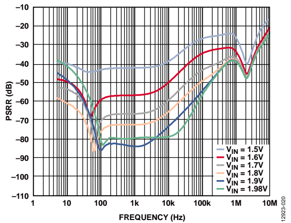
図 20. 各種負荷での電源電圧変動除去比 (PSRR) の周波数特性、 V_{OUT} = 1.3\text{ V} 、負荷電流 = 3 A
