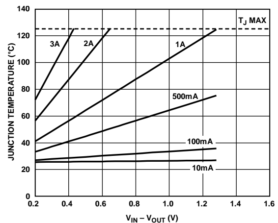
図 36. 500 mm 2 の PCB 銅箔、 T_A = 25^\circ\text{C}
