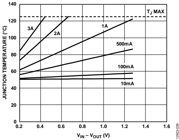
図 38. 6400 mm 2 の PCB 銅箔、T A = 50°C
