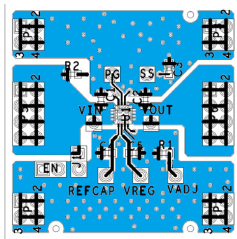
図 47. 代表値なボード・レイアウト、上面
