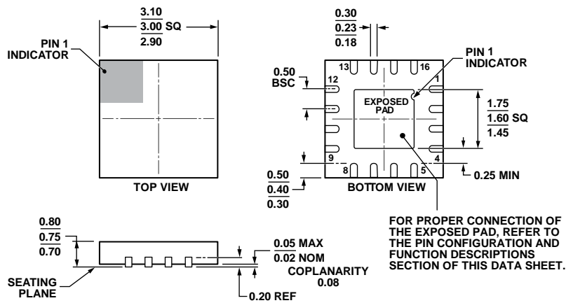
図 49. 16 ピン・リードフレーム・チップスケール・パッケージ [LFCSP] 3 mm × 3 mm ボディ、0.75 mm パッケージ高 (CP-16-22) 寸法: mm
