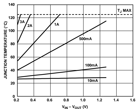
図 37. 25 mm 2 の PCB 銅箔、 T_A = 25^\circ\text{C}
