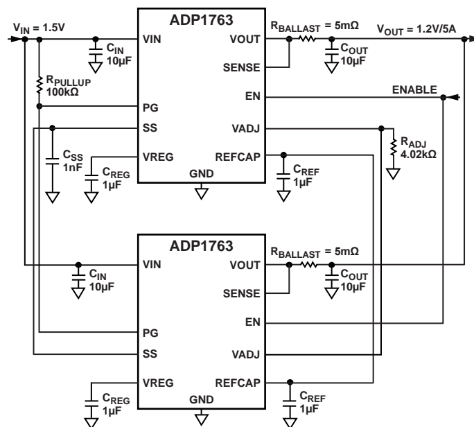
図 34. 大電流出力を実現する 2 個の ADP1763 デバイスの並列接続
