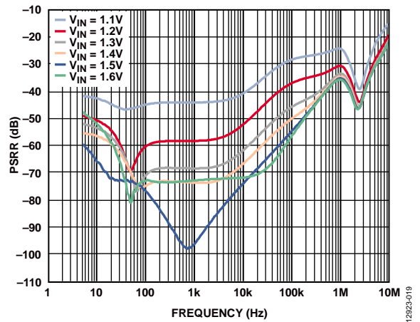
図 19. 各種負荷での電源電圧変動除去比 (PSRR) の周波数特性、 V_{OUT} = 0.9\text{ V} 、負荷電流 = 3 A
