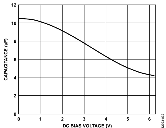
図 33. DC バイアス電圧対容量
