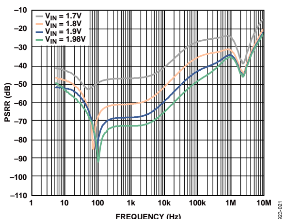
図 21. 各種負荷での電源電圧変動除去比 (PSRR) の周波数特性、 V_{OUT} = 1.5\text{ V} 、負荷電流 = 3 A
