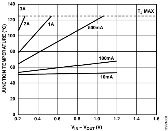
図 40. 25 mm 2 の PCB 銅箔、T A = 50°C
