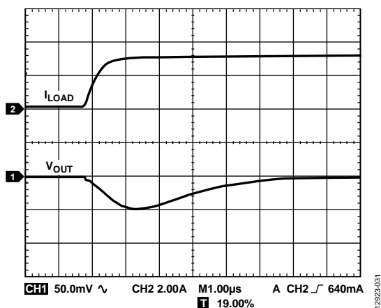
図 32. 出力過渡応答、C OUT = 47 μF
