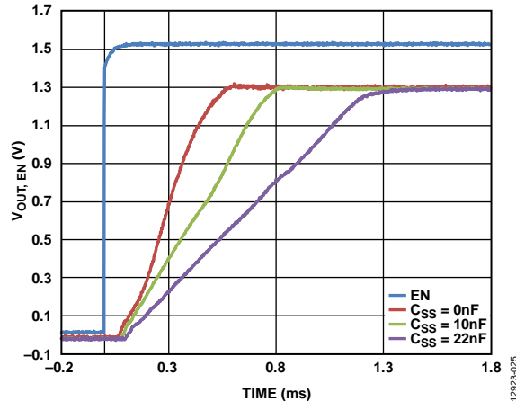
図 25. 固定 VOUT の外付けソフト・スタート・コンデンサによるランプアップ時間 (VOUT, EN)
