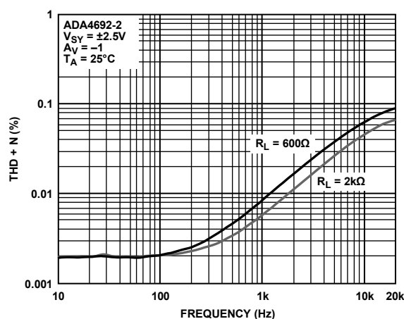
図 1. THD + ノイズの周波数特性
