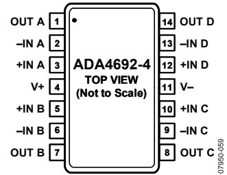
図 8. 14 ピン TSSOP (RU-14)
