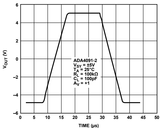
図 14.大信号過渡応答
