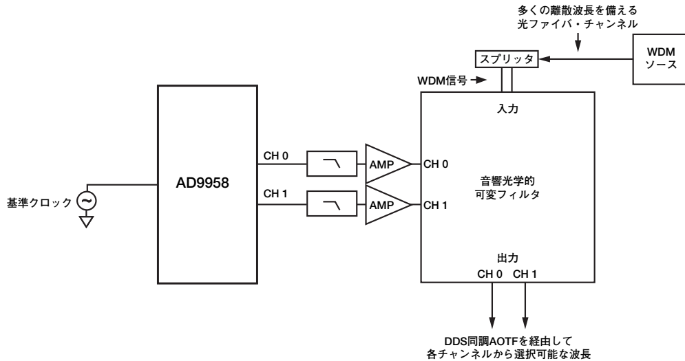
図28. DDSから音響光学的可変フィルタにスティミュラスを供給する回路
