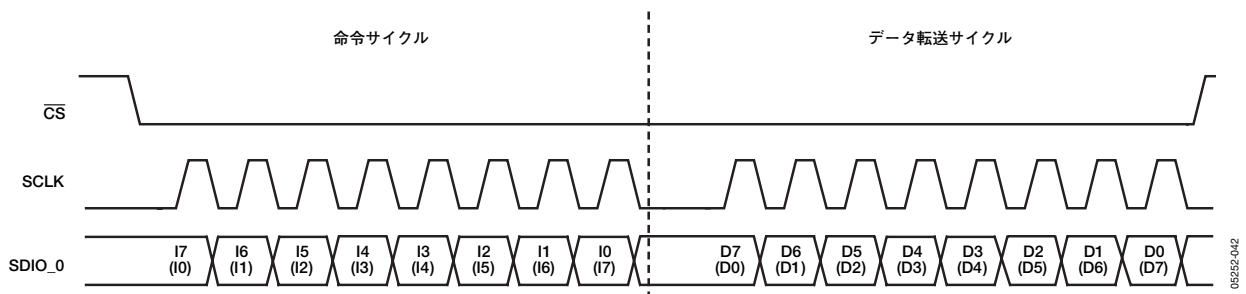
図42. シングル・ビットのシリアル・モードの書き込みタイミングクロックをローレベルにストール
