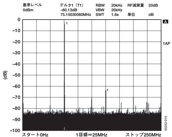
図10. f_{OUT}=75.1\text{MHz} 、 f_{CLK}=500\text{MSPS} 、 ワイドバンドSFDR
