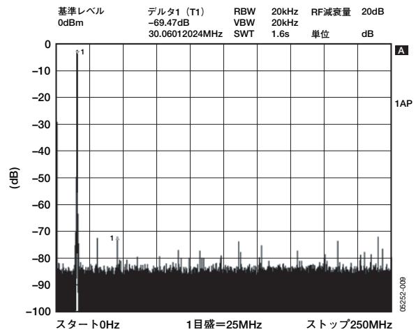
図9. f_{OUT}=15.1\text{MHz} 、 f_{CLK}=500\text{MSPS} 、 ワイドバンドSFDR
