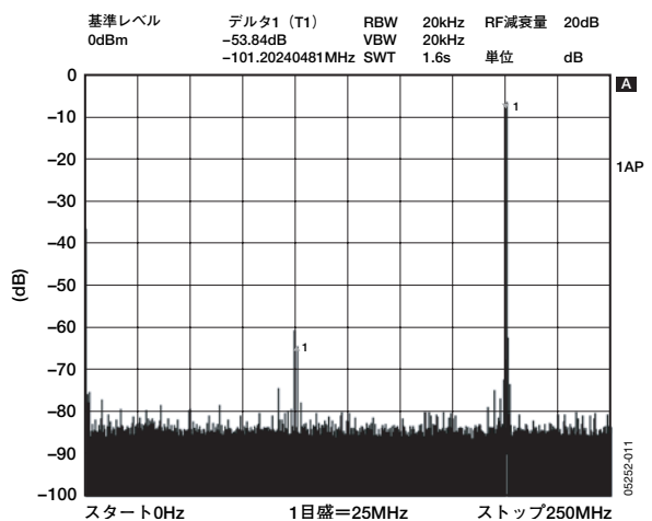
図11. f_{OUT}=200.3\text{MHz} 、 f_{CLK}=500\text{MSPS} 、 ワイドバンドSFDR
