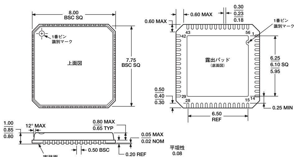
図49. 56ピン・リード・フレーム・チップ・スケール・パッケージ [LFCSP_VQ]
