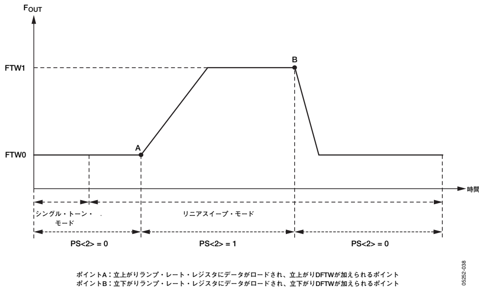
図38. ノードウェル機能をディスエーブルにしたときのリニアスイープ
