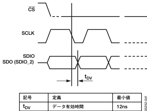
図41. シリアルI/Oポートからのデータ読み出しタイミング図
