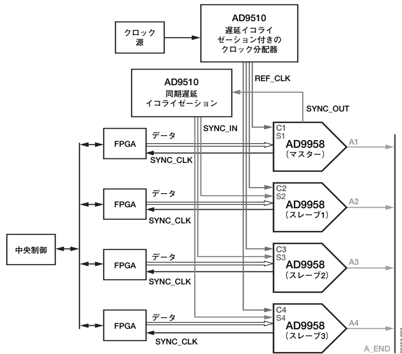
図27. 複数のAD9958を同期化し、AD9510を基準クロックとSYNCクロックのクロック分配器として使用して、チャンネル容量を増加する回路
