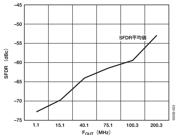
図23. f_{OUT} 対 チャンネルのSFDR平均値
