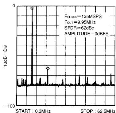
図36 . 1波のSFDR
