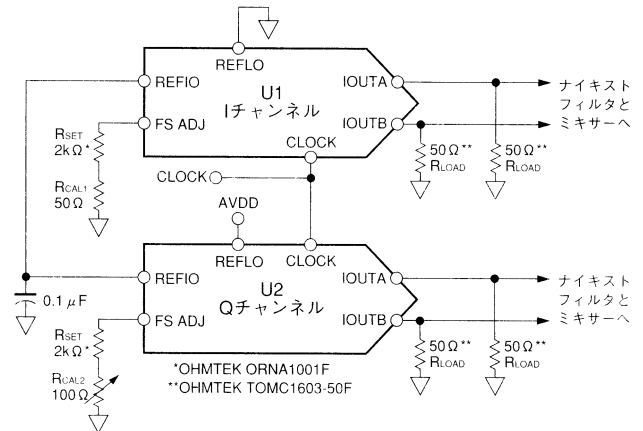
図57 . 2個のAD9760を使用したベースバンドQAM構成
