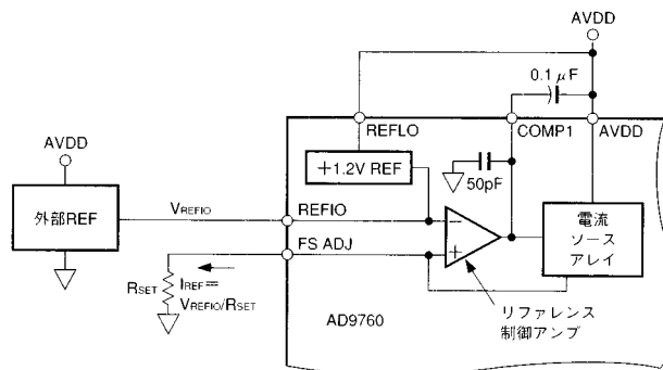
図41．外部リファレンス構成
