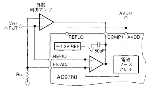
図45．外部リファレンス制御アンプを構成
