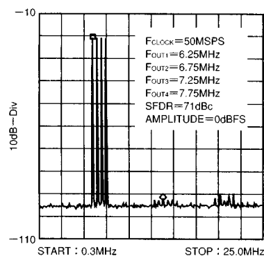
図38 . 4波のSFDR
