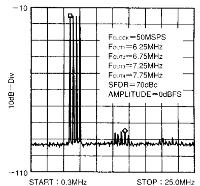
図20. 4波のSFDR
