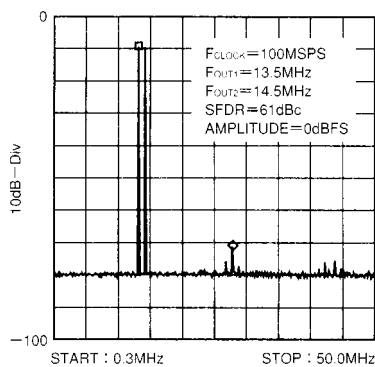
図19. 2波のSFDR
