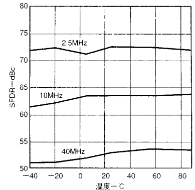
図17. SFDRと温度 @ 100MSPS、0dBFS
