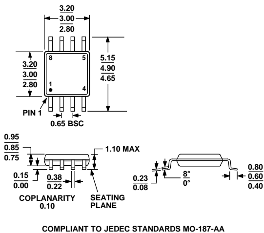
図52.8 ピン・ミニ・スモール・アウトライン・パッケージ[MSOP] (RM-8) 寸法: mm
