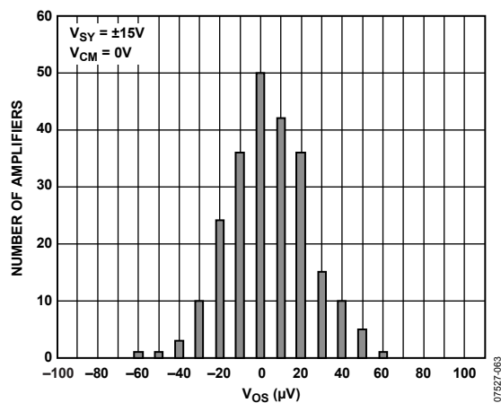
図 8. 入力オフセット電圧の分布
