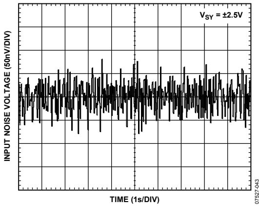
図 47. 0.1~10 Hz でのノイズ
