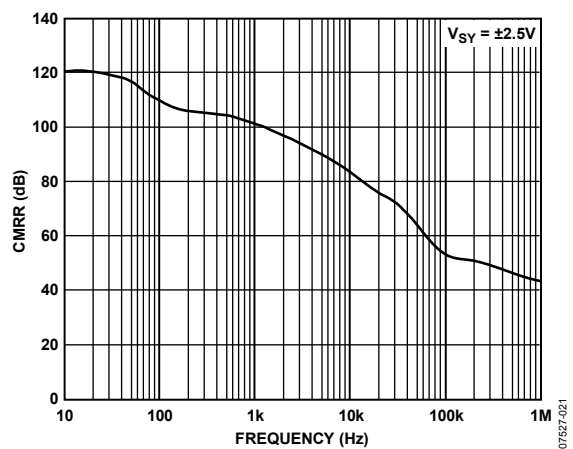
図 25.CMRR の周波数特性
