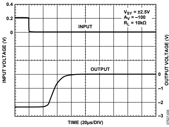
图 36. 负侧过负荷回復
