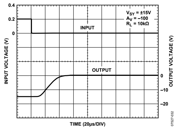
图 39. 负侧过负荷回復
