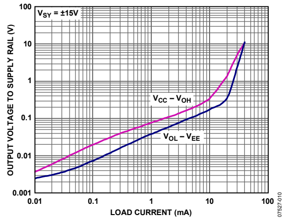
図 16. 負荷電流対電源レールまで近づく出力電圧
