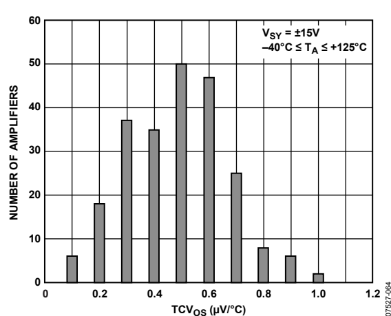
図 9. 入力オフセット電圧ドリフトの分布
