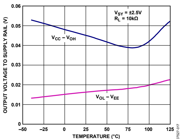
図 17.電源レールまで近づく出力電圧の温度特性
