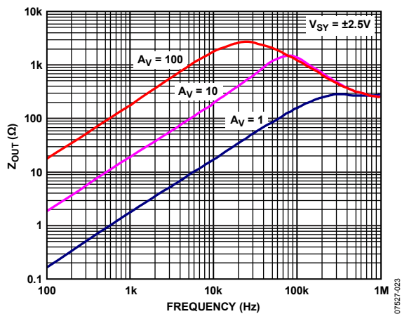
図 24.出カインピーダンスの周波数特性
