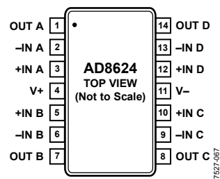
図 3.14 ピン TSSOP
