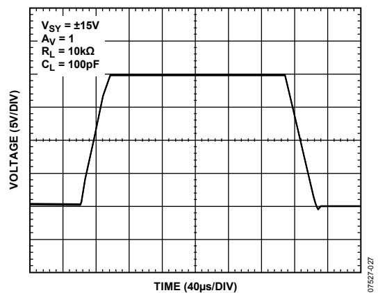
図 34.大信号過渡応答
