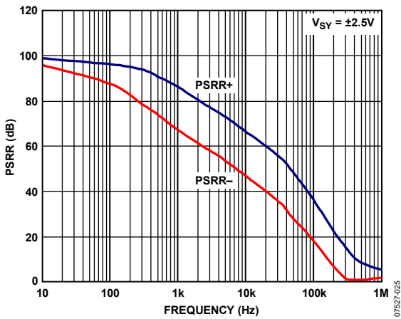
図 29.PSRR の周波数特性
