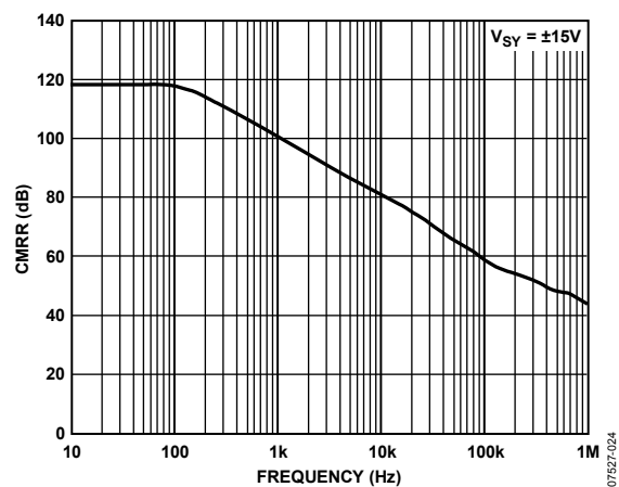
図 28.CMRR の周波数特性
