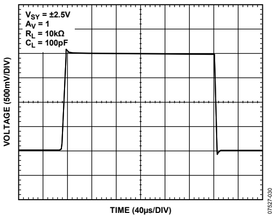
図 31.大信号過渡応答
