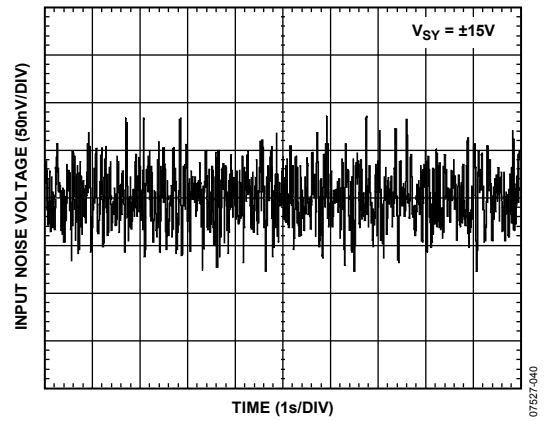
図 49. 0.1~10 Hz でのノイズ
