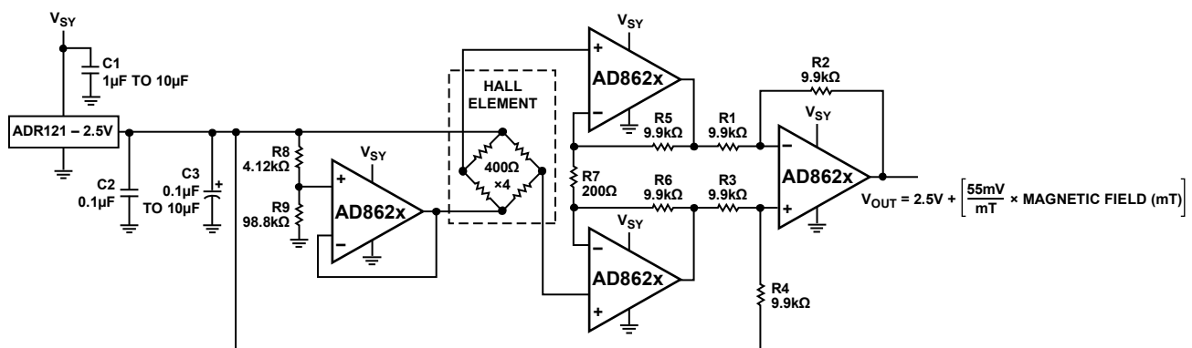
図 57.ホール・センサーのシグナル・コンデショニング
