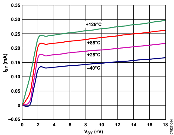
図 18.電源電圧対電源電流
