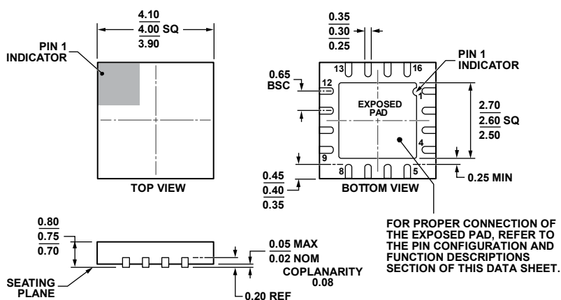
図 61.16 ピン・リードフレーム・チップ・スケール・パッケージ[LFCSP_WQ] 4 mm x 4mm ボディ、極薄クワッド (CP-16-17) 寸法: mm
