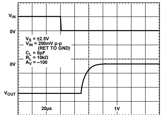
図30.負の過電圧回復時間
