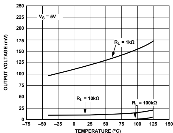
図49.電源レールまで近づく出力電圧の温度特性
