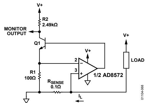
図68.ローサイド負荷電流モニター
