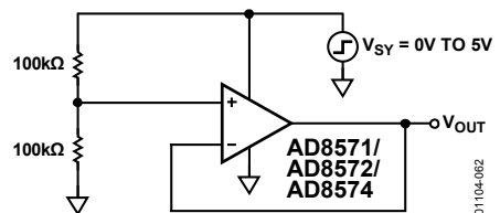
図62.AD857x パワーアップ時間のテスト回路
