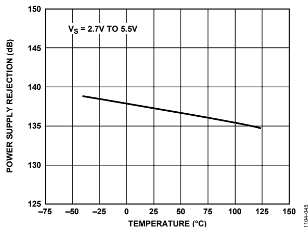
図45.電源除去比の温度特性
