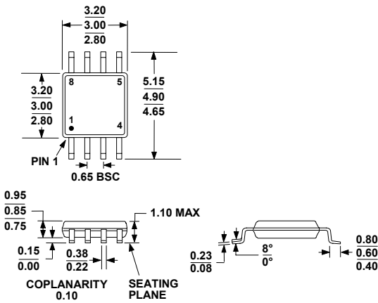
図69.8 ピン・ミニ・スモール・アウトライン パッケージ[MSOP] (RM-8) 寸法: mm
