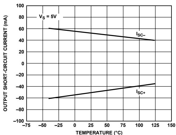
図47.出力短絡電流の温度特性
