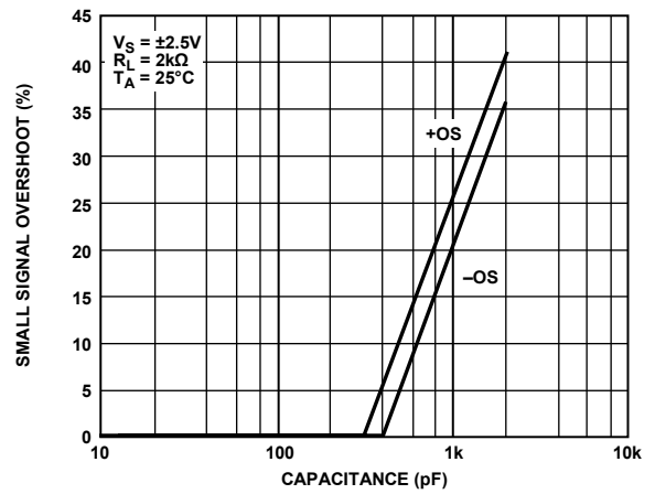
図28.小信号オーバーシュート対負荷容量
