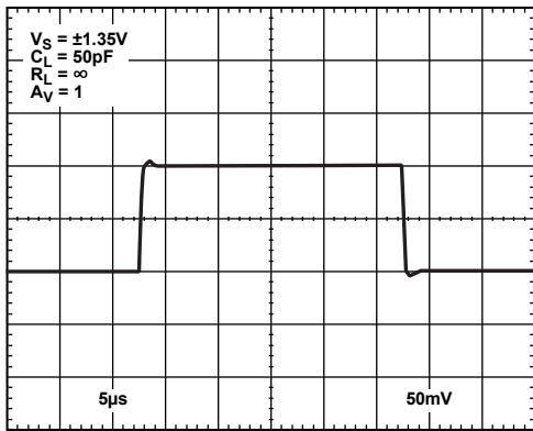
図25.小信号過渡応答
