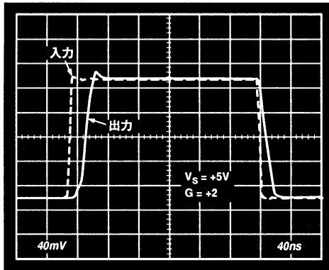
図33. オーバードライブから回復
