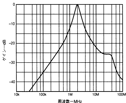
図39. バイクワッド型の2 MHzバンドパス・フィルタの周波数特性
