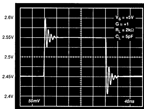
図30. 100mVステップ・パルス応答、 V_S = +5V 、 G = +1
