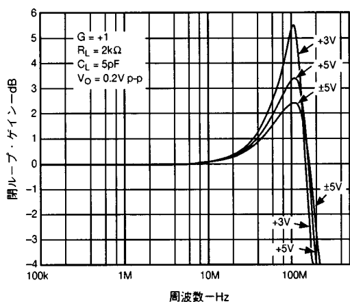
図17. クローズドループ周波数特性と電源
