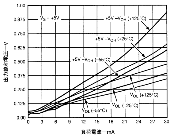
図21. 出力飽和電圧と負荷電流
