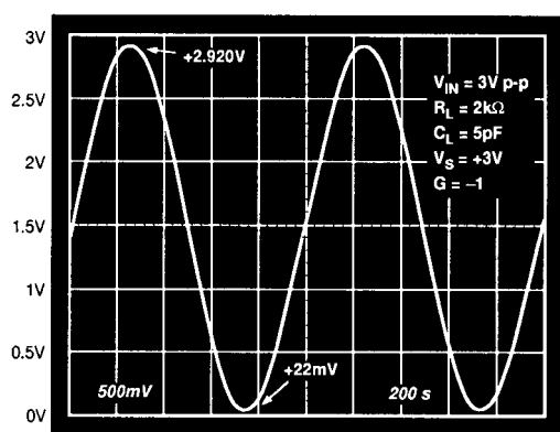
図31. 出力振幅特性、 V_S = +3V
