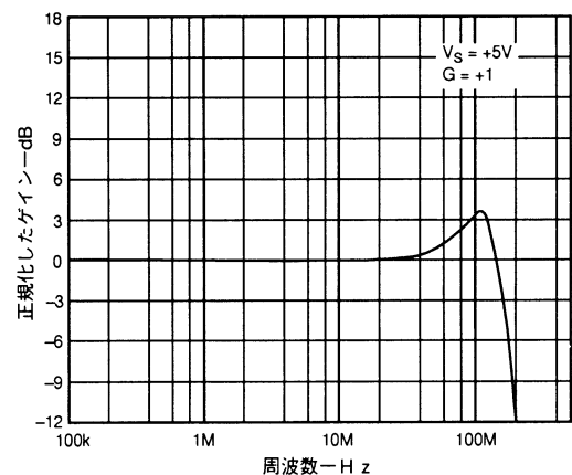
図2. 周波数応答: ゲイン = +1、 V_S = +5 V
