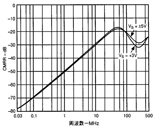
図20. CMRRの周波数特性
