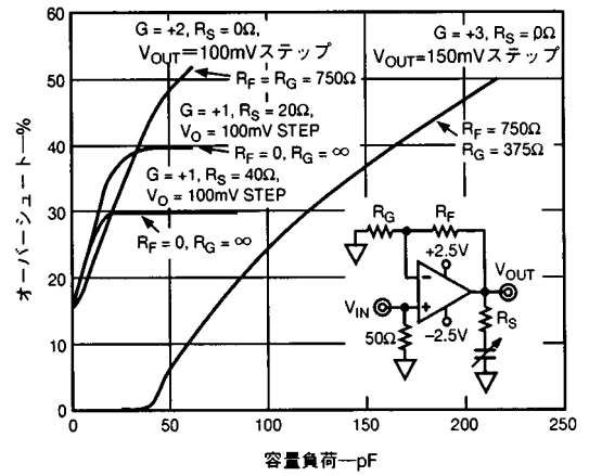
図25. オーバーシュート(%)と容量負荷
