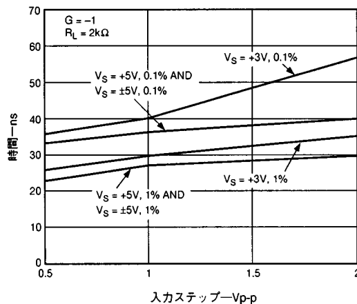
図19. ステップ入力のセトリング時間
