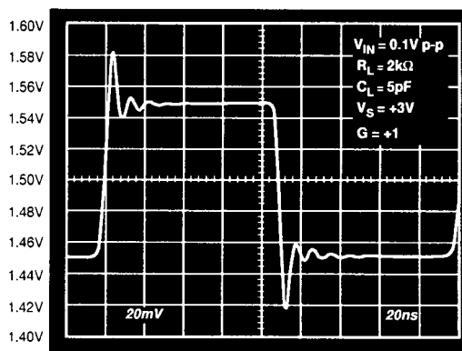
図32. ステップ・パルス応答、 G = +1 、 V_{IN} = 100mV
