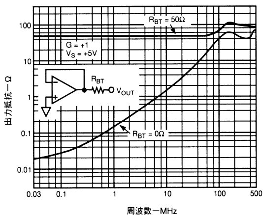
図18. 出力抵抗の周波数特性
