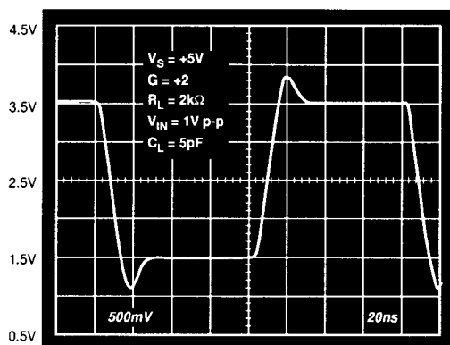
図29. 1Vステップ・パルス応答、 V_S = +5V 、 G = +2
