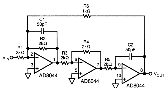
図38. AD8044を使用したバイクワッド型の2 MHzバンドパス・フィルタ
