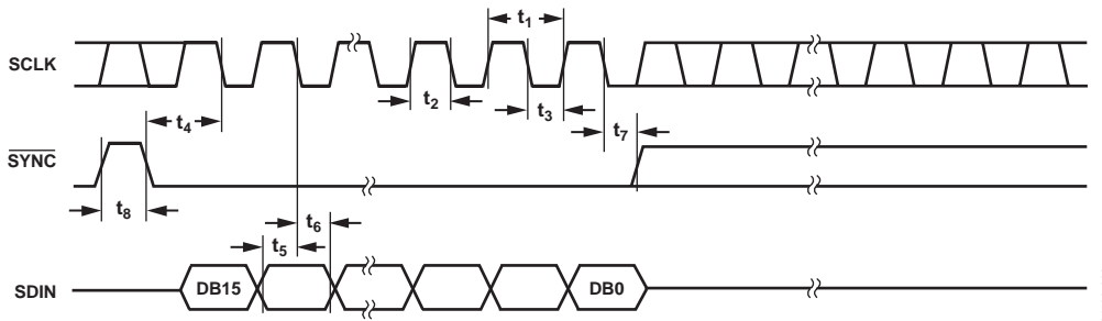
図2. スタンドアロン・タイミング図
