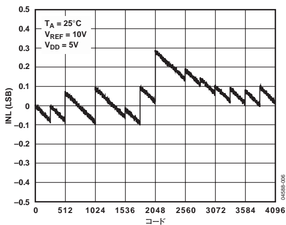
図6. コード対 INL
