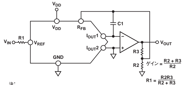
図39. 電流出力DACゲインの増加
