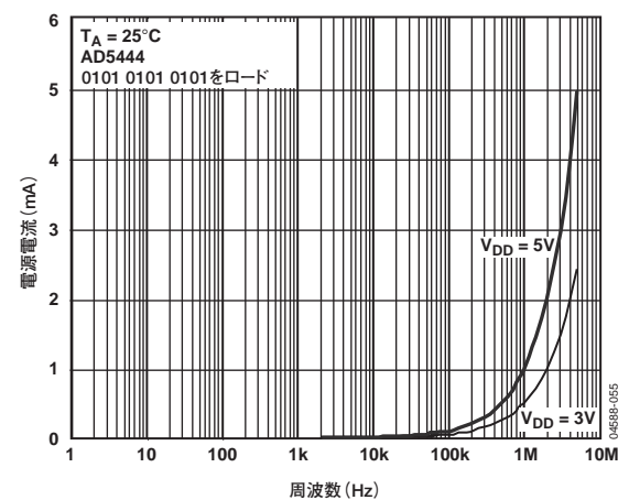
図17. 更新レート 対 電源電流
