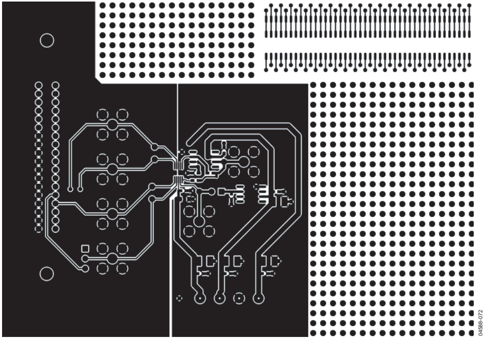
図51. 部品面のアートワーク
