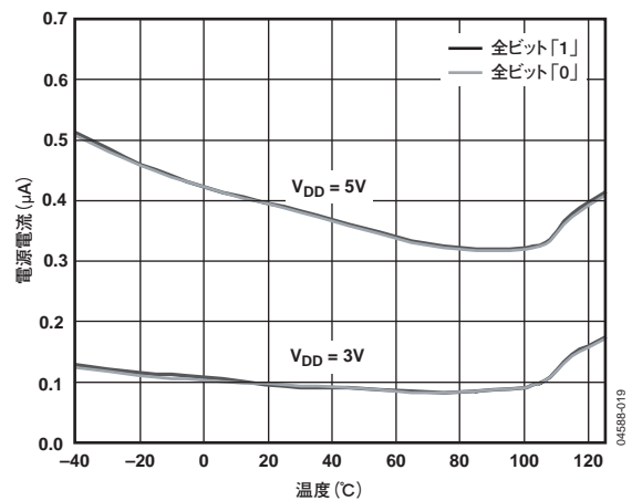
図16. 電源電流の温度特性
