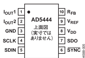
図5. MSOP( RM-10 )のピン配置
