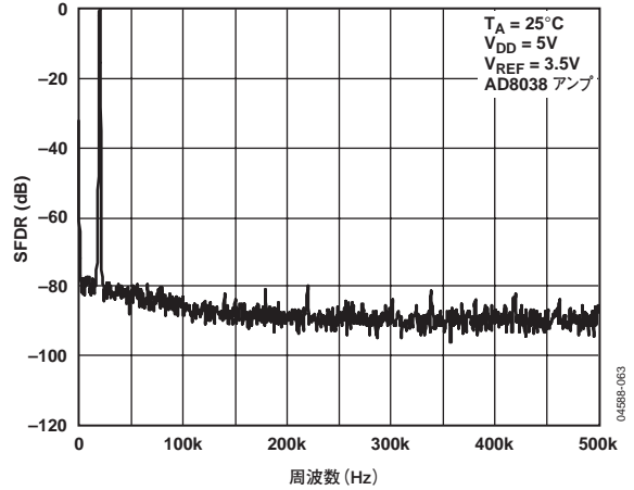
図27. ワイドバンドSFDR( f_{OUT} = 20\text{kHz} 、クロック = 1MHz )
