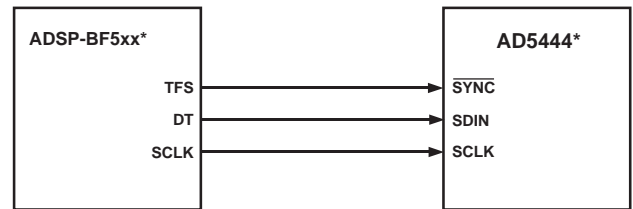
図45. ADSP-BF5xxとAD5444とのインターフェース
