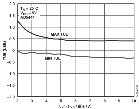
図11. リファレンス電圧対 TUE
