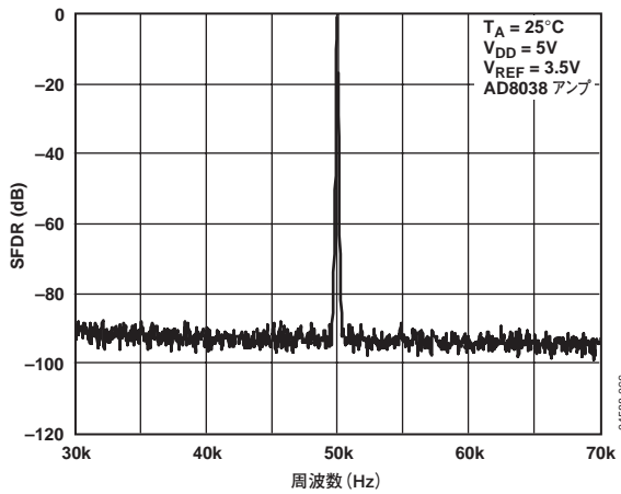
図30. ナローバンドSFDR( f_{OUT} = 50\text{kHz} , クロック = 1MHz)
