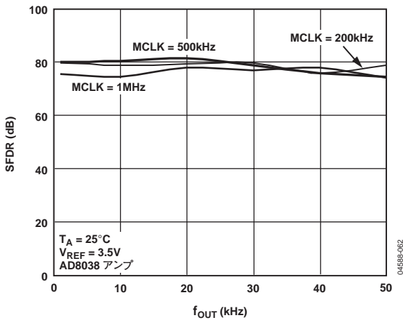
図26. f_{OUT} 周波数 対 ワイドバンドSFDR
