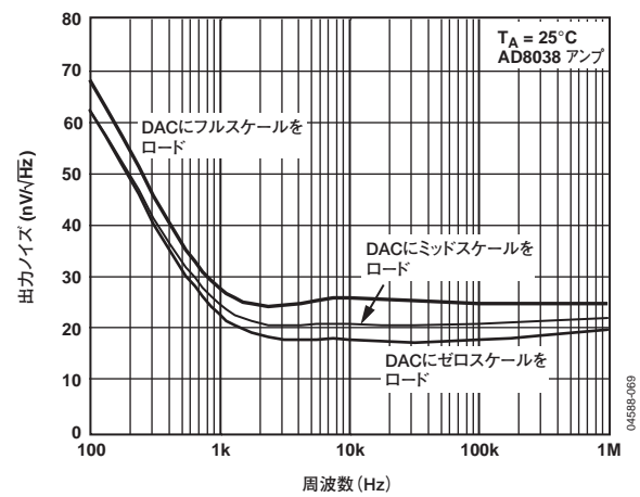
図33. 出力ノイズ・スペクトル密度
