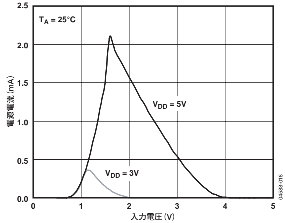
図15. ロジック入力電圧 対 電源電流
