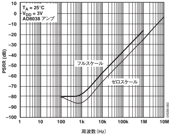
図24. 電源電圧変動除去比の周波数特性
