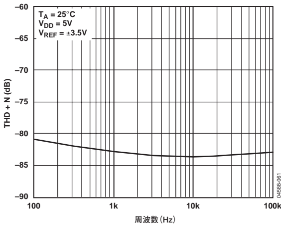
図25. THD + ノイズの周波数特性
