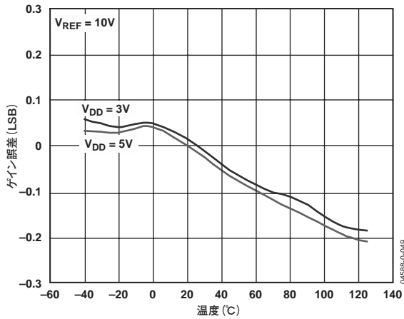
図12. ゲイン誤差 (LSB) の温度特性
