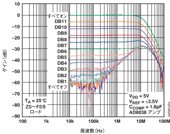
図19. 各コードに対するリファレンス乗算帯域幅の周波数特性
