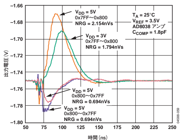
図23. ミッドスケール遷移 ( V_{REF} = 3.5V )
