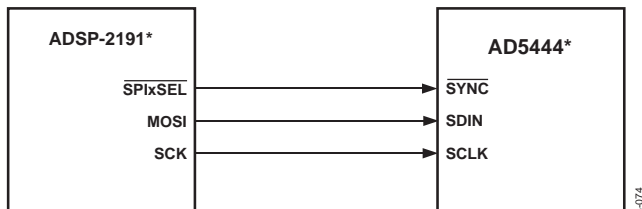
図42. ADSP-2191のSPIとAD5444とのインターフェース
