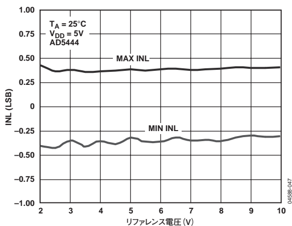
図8. リファレンス電圧対 INL
