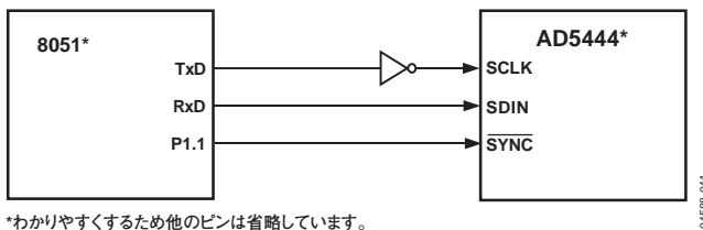
図46. 80C51/80L51とAD5444とのインターフェース
