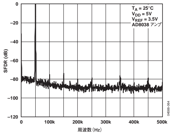
図28. ワイドバンドSFDR( f_{OUT} = 50\text{kHz} 、クロック = 1MHz )
