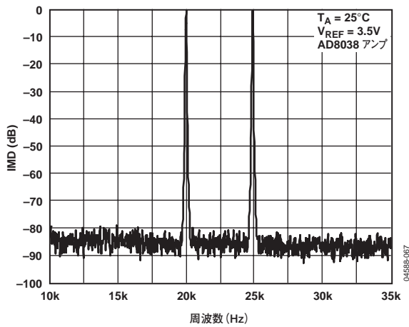
図31. ナローバンドIMD( f_{OUT} = 20\text{kHz} , 25kHz, クロック = 1MHz)
