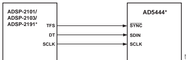
図43. ADSP-2101/ADSP-2103/ADSP-2191のSPORTとAD5444とのインターフェース
