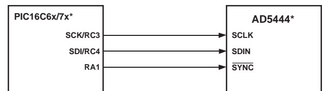
図49. PIC16C6x/7xとAD5444とのインターフェース
