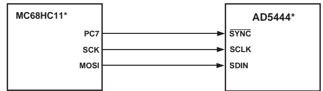
図47. 68HC11/68L11とAD5444とのインターフェース
