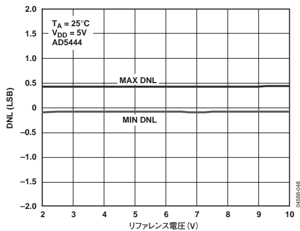
図9. リファレンス電圧対 DNL
