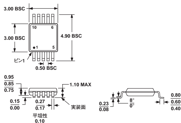
図54. 10ピン・ミニ・スモール・アウトライン・パッケージ[MSOP] (RM-10) 寸法単位:mm
