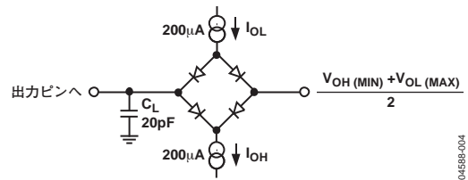
図4. SDOタイミング仕様に対する負荷回路
