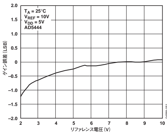
図13. リファレンス電圧 対 ゲイン誤差 (LSB)
