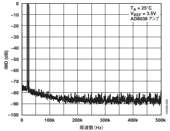
図32. ワイドバンドIMD( f_{OUT} = 20\text{kHz} , 25kHz, クロック = 1MHz)
