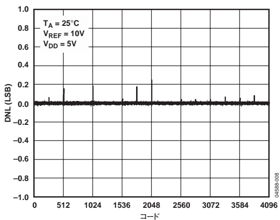
図7. コード対 DNL
