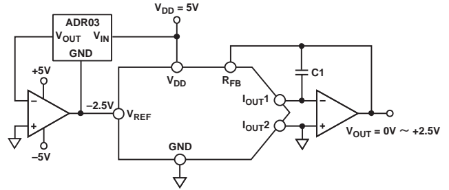
図38. 最小の部品による正の電圧出力
