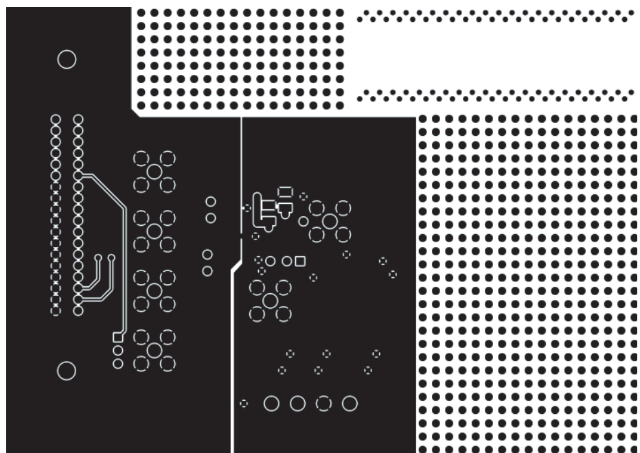
図53. ハンダ面のアートワーク
