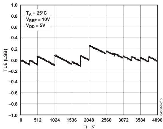
図10. コード対 TUE
