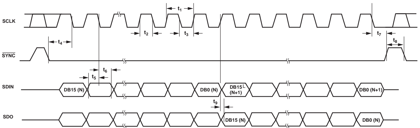
図3. デイジーチェーン・タイミング図
