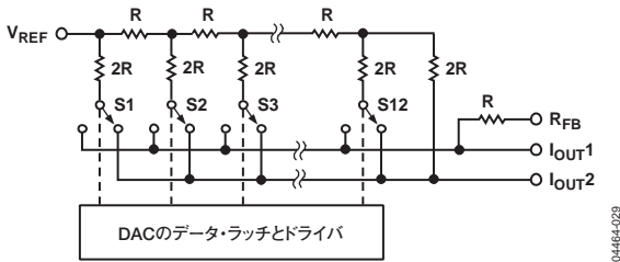
図34. 簡略回路図
