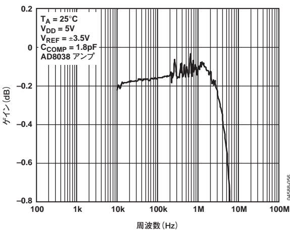
図20. リファレンス乗算帯域幅 (全ビット「1」をロード)
