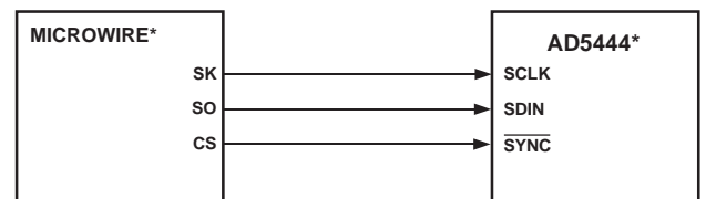
図48. MICROWIREとAD5444とのインターフェース
