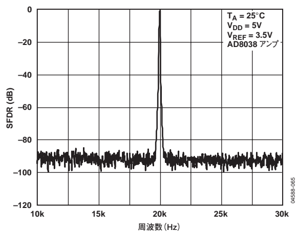
図29. ナローバンドSFDR( f_{OUT} = 20\text{kHz} 、クロック = 1MHz )
