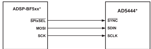
図44. ADSP-BF5xxとAD5444とのインターフェース
