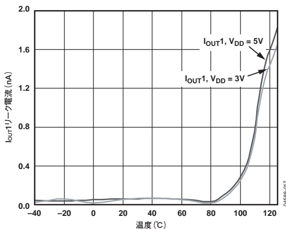
図14. IOUT1リーク電流の温度特性
