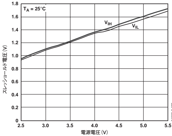
図18. 電源電圧 対 スレッシュホールド電圧
