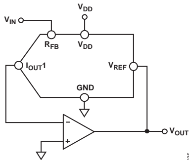
図40. デバイダまたはプログラマブルなゲイン素子として使用した電流切替え型DAC
