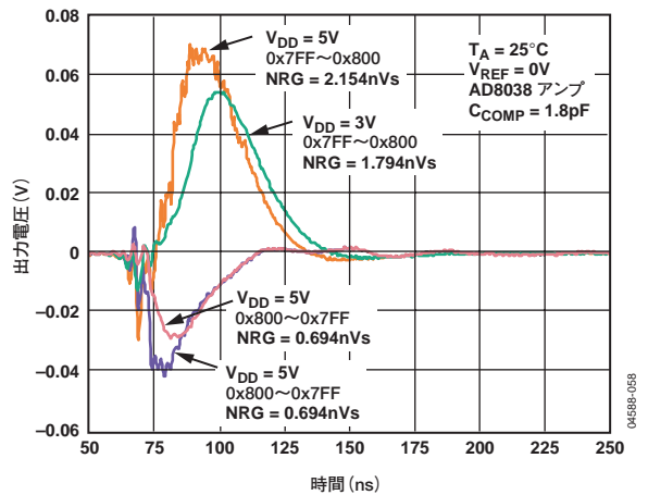
図22. ミッドスケール遷移 ( V_{REF} = 0V )
