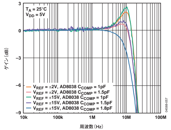
図21. 各補償コンデンサに対するリファレンス乗算帯域幅の周波数特性
