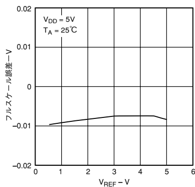
特性22 フルスケール誤差 対 V_{REF}
