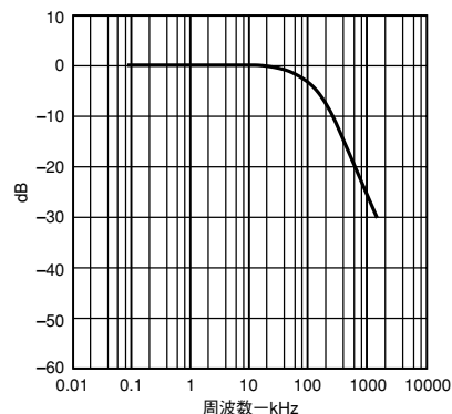
特性21 マルチプライヤ帯域幅 (小信号周波数応答性)
