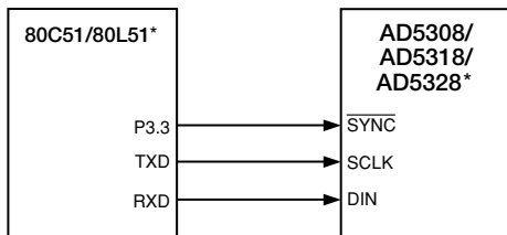
図13 80C51/80L51とAD5308/AD5318/AD5328とのインターフェース
