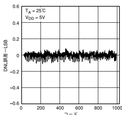
特性5 AD5318の代表的なDNLプロット
