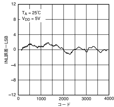
特性3 AD5328の代表的なINLプロット
