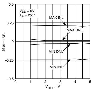
特性7 AD5308のINLおよび DNL誤差 対 V_{REF}
