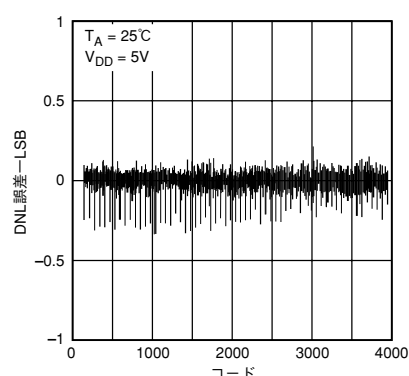
特性6 AD5328の代表的なDNLプロット
