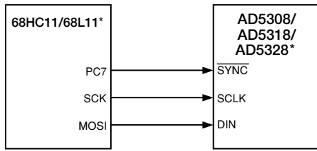
図12 68HC11/68L11とAD5308/AD5318/AD5328とのインターフェース
