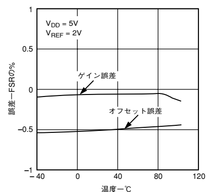
特性9 AD5308のオフセットおよび ゲイン誤差 対 温度
