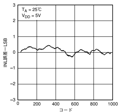
特性2 AD5318の代表的なINLプロット
