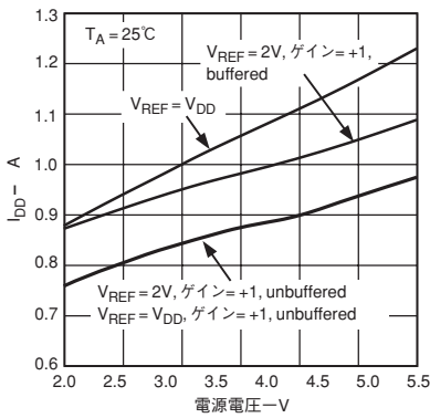
特性13 電源電流 対 電源電圧
