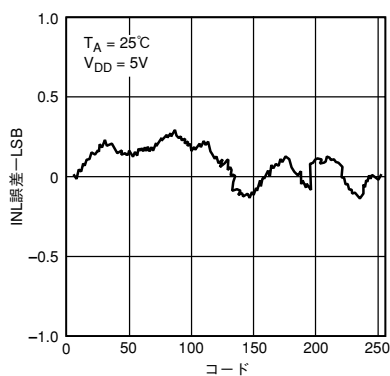
特性1 AD5308の代表的なINLプロット
