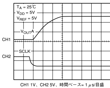
特性16 ハーフスケール・セトリング (1/4から3/4スケールのコード変化)
