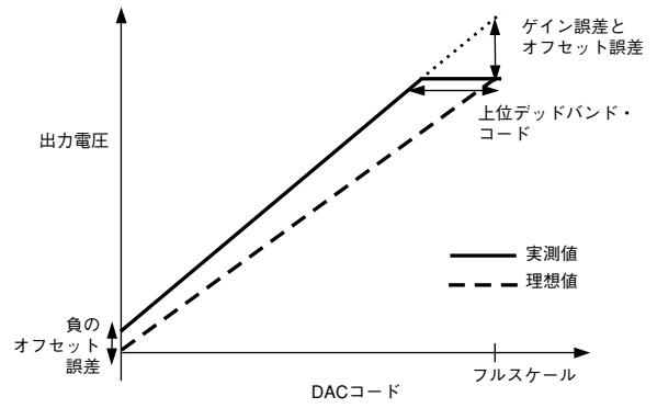
図3 正のオフセットを含む伝達関数
