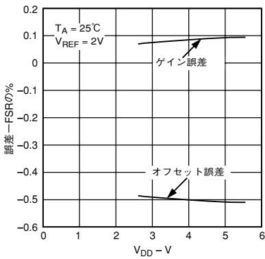
特性10 オフセットおよびゲイン誤差 対 V_{DD}
