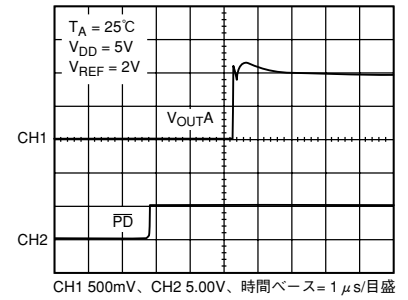
特性18 ミッドスケールへのパワーダウン終了
