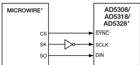
図14 MICROWIREとAD5308/AD5318/AD5328とのインターフェース
