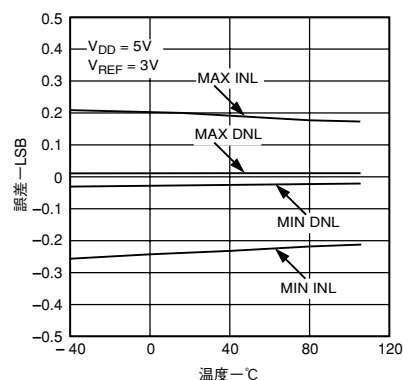
特性8 AD5308のINLおよび DNL誤差 対 温度
