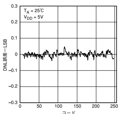
特性4 AD5308の代表的なDNLプロット
