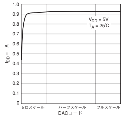
特性12 電源電流 対 DACコード
