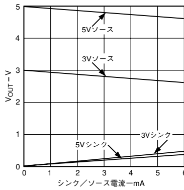
特性11 V_{OUT} ソースおよびシンク電流能力
