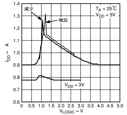
特性15 電源電流 対 SCLKおよびDINロジック入力電圧の増減
