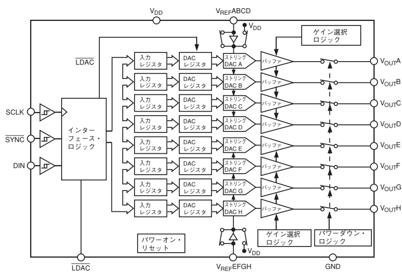
機能ブロック図
