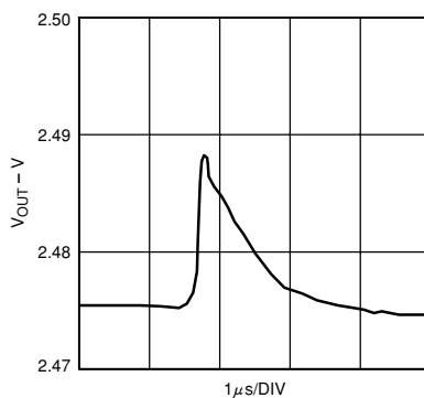
特性20 AD5328のメジャー・コード遷移時グリッチ・エネルギー
