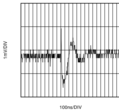
特性23 DAC間クロストーク
