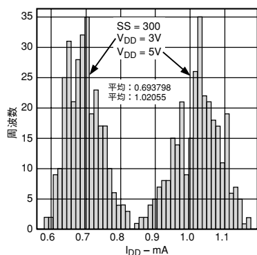
特性19 V_{DD} = 3V および V_{DD} = 5V 時の I_{DD} ヒストグラム
