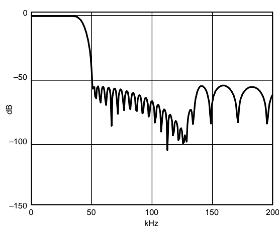
特性6 DAC総合フィルタ応答、 f_s = 96\text{kHz}
