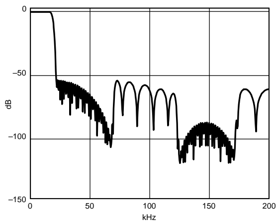
特性5 DAC総合フィルタ応答、 f_s = 48\text{kHz}
