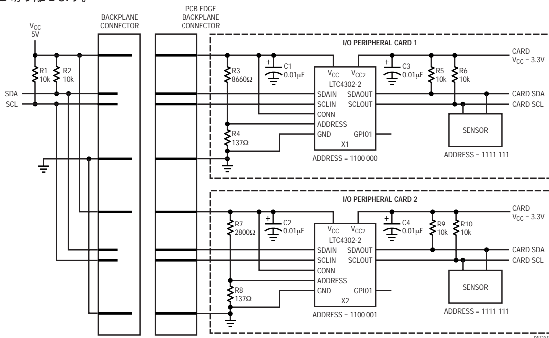
図3 . ネストされたアドレス指定と5Vから3.3Vへのレベル変換のアプリケーションでの使用
