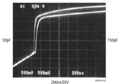
図2 . C BUS = 50pF、C BUS = 150pFでの立上り時間を短縮する立上り時間アクセラレータ
